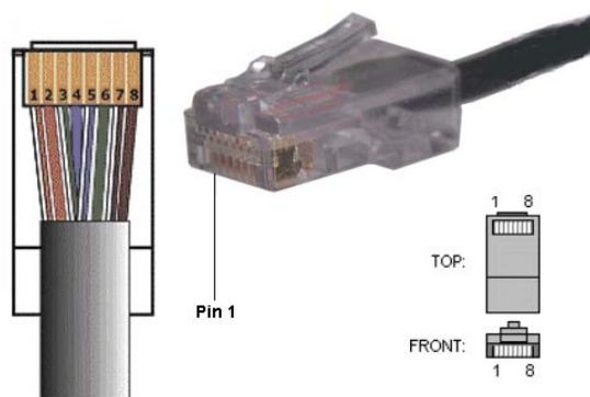
Figura 39. RJ45 macho
