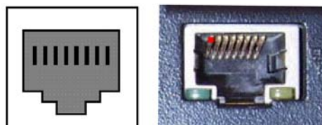
Figura 40. RJ45 hembra
