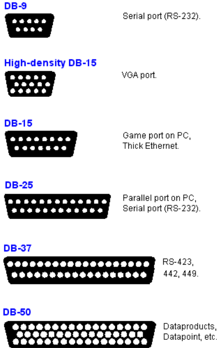
Figura 43. Conectores tipo D-Sub
