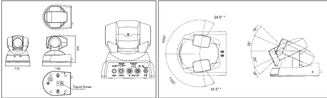
Figura 24. Videocámara Robótica EVI-D100
