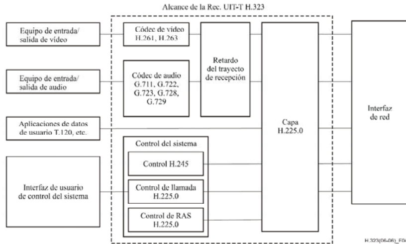
Figura 6. Diagrama de un equipo terminal H.323
