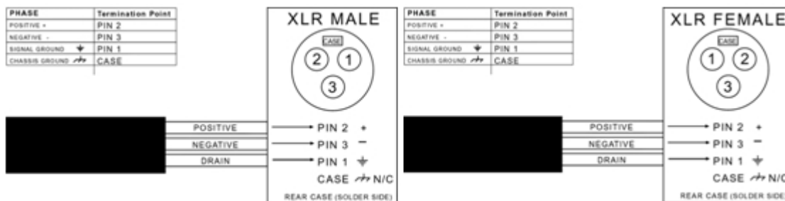
Figura 38. Conectores XLR “Cannon”
