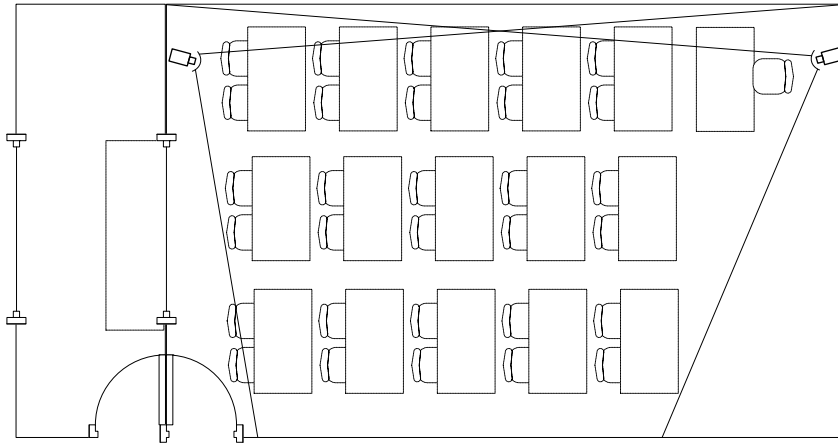
Figura 12. Dispositivos de entrada de video en el Aula de Videoconferencias
