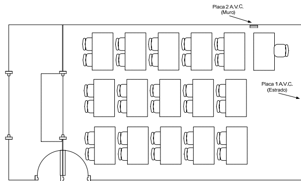
Figura 15. Ubicación de placas de conexión en el Aula de Usos Múltiples
