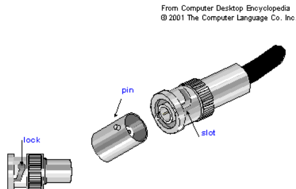
Figura 42. Conector BNC
