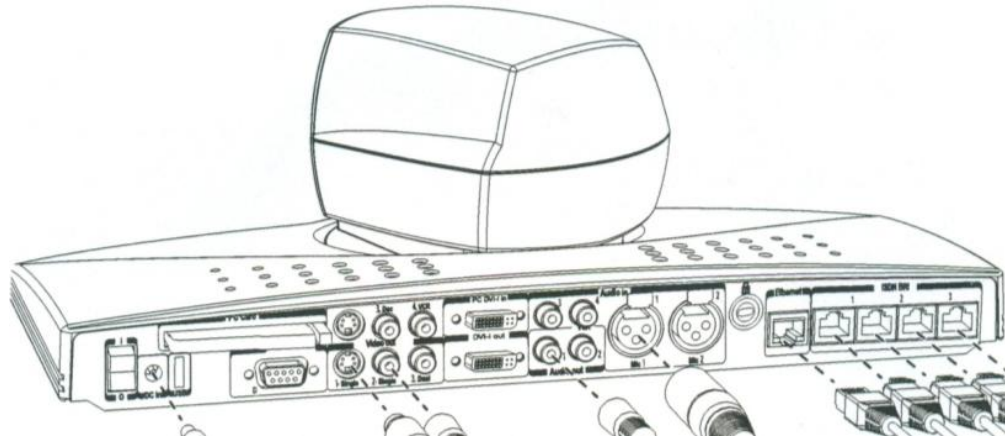
Figura 10. CoDec de videoconferencia 880 MXP
