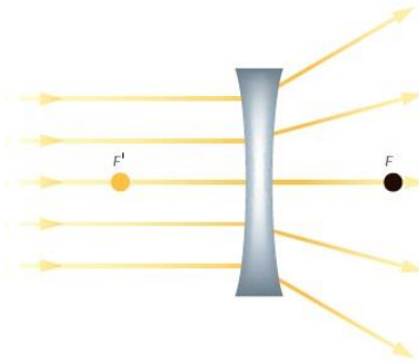
Figura 7: Lente divergente.
