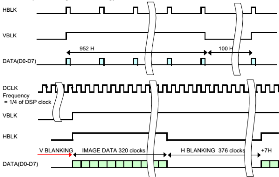
Figura 56: Diagrama de Lectura de datos de la cámara.
