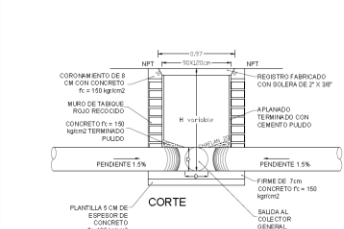
DETALLE DE REGISTRO (R-5) PLUVIAL 90X120 cm (INTERIOR)
