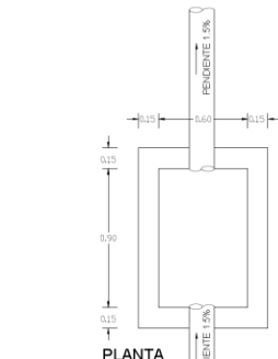
DETALLE DE REGISTRO PLUVIAL 90X60 cm (INTERIOR) REGISTROS: 1, 2, 3, 4, 6, 7, 8 y 9
