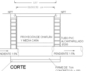
DETALLE DE REGISTRO PLUVIAL 90X60 cm (INTERIOR) REGISTROS: 1, 2, 3, 4, 6, 7, 8 y 9
