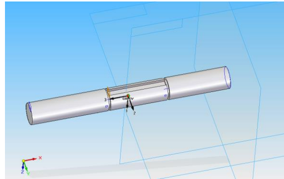
Fig 3.18. Eje motriz para primer paso de transmisión
