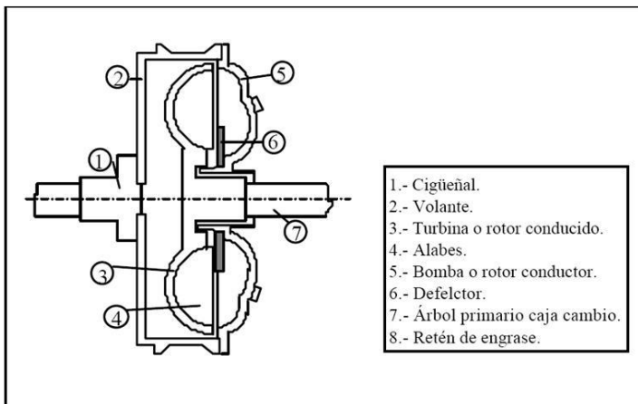
Fig. 2.13 Embrague hidráulico [11]
