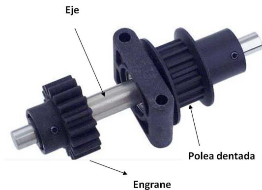
Fig. 2.20 Ejemplo de ensamble de un engrane y una polea dentada en un eje
