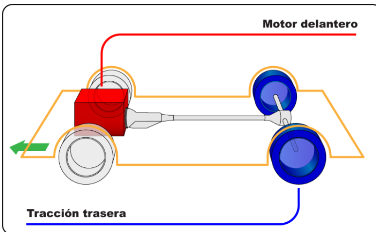
Fig. 2.3 Configuración de motor delantero con tracción trasera [8]
