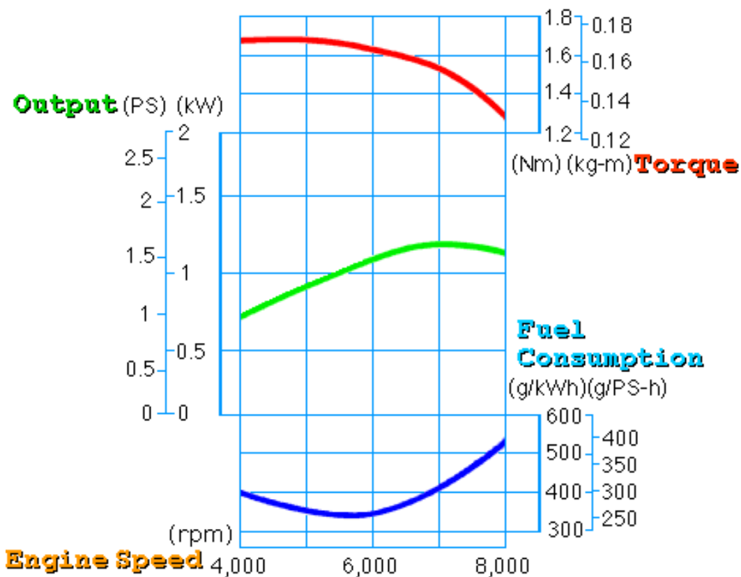
Fig. 3.9 Curva de rendimiento del motor GX31.
