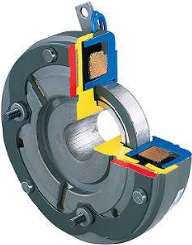
Fig. 2.14 Clutch industrial de 2 polos [11].
