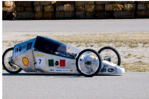
Fig.1.5 Prototipo "Ahuicyani" participante en 2009.
