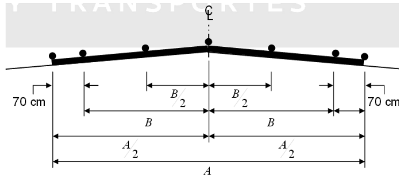
FIGURA 4.29.- Ubicación de los puntos por nivelar
