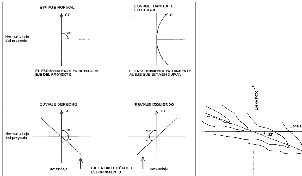
Imagen 4.31 Croquis de esvajes
