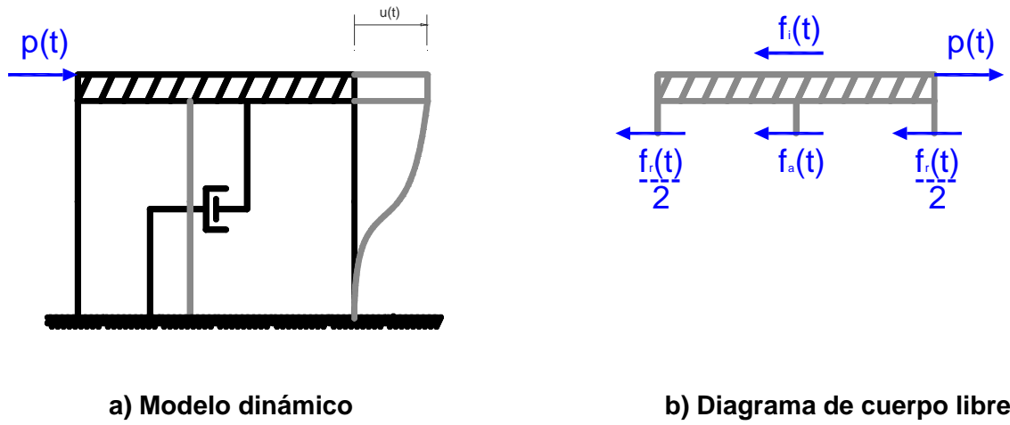
Fig 2.3.- Sistema de un grado de libertad
