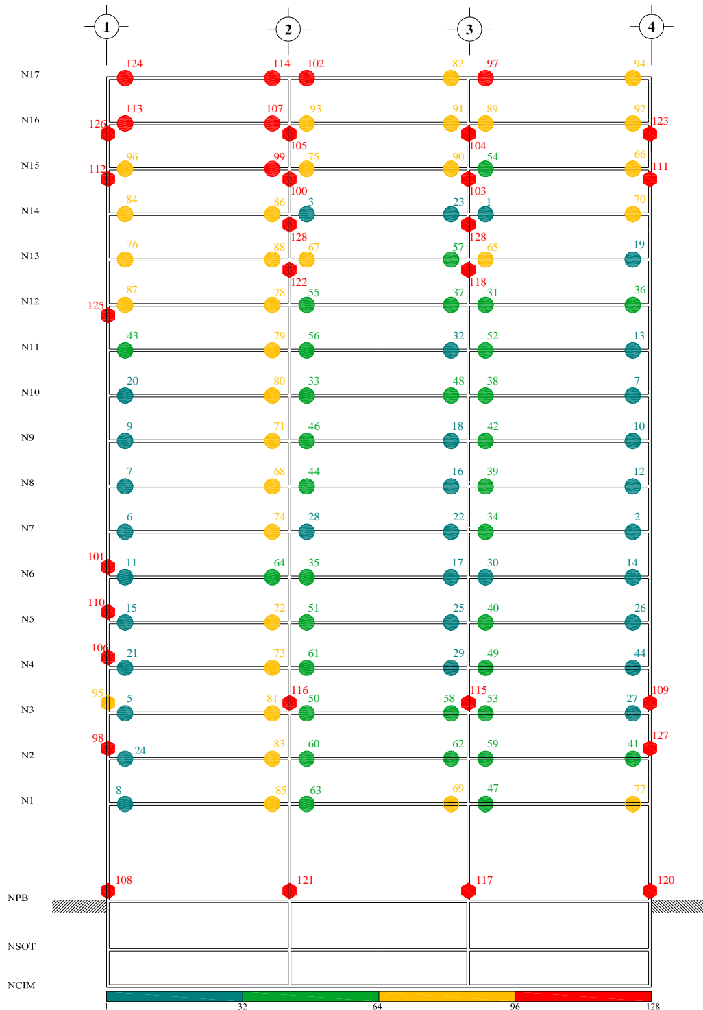
Fig 4.123.- Mecanismo de falla y secuencia de formación de articulaciones plásticas, edificio 17 niveles, caso A (Cuerpo Principal) con resistencias nominales, distribución de fuerzas laterales del análisis dinámico modal espectral
