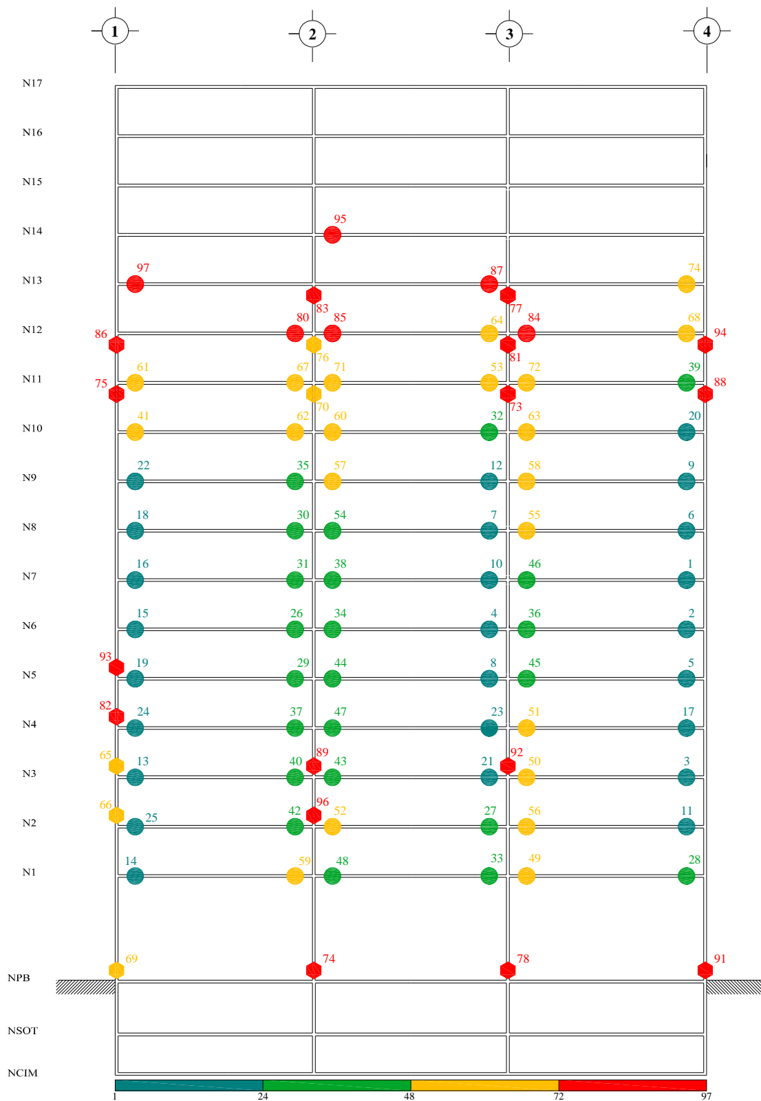
Fig A.25.- Secuencia de formación de articulaciones plásticas, análisis estático no-lineal (Push-over) con distribución de cargas laterales de análisis paso a paso inelástico, sobre-resistencias, edificio 17 niveles, caso A (Cuerpo Principal)
