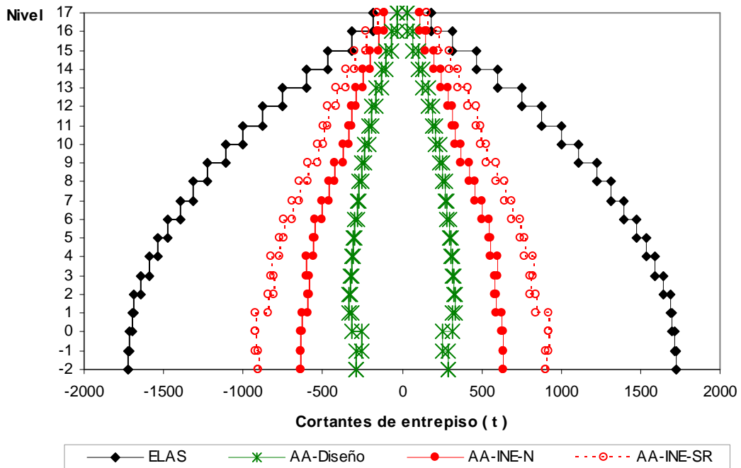
Fig 4.60.- Distribución en elevación de las fuerzas cortantes de entrepiso, edificio 17 niveles, caso B (Apéndice A)
