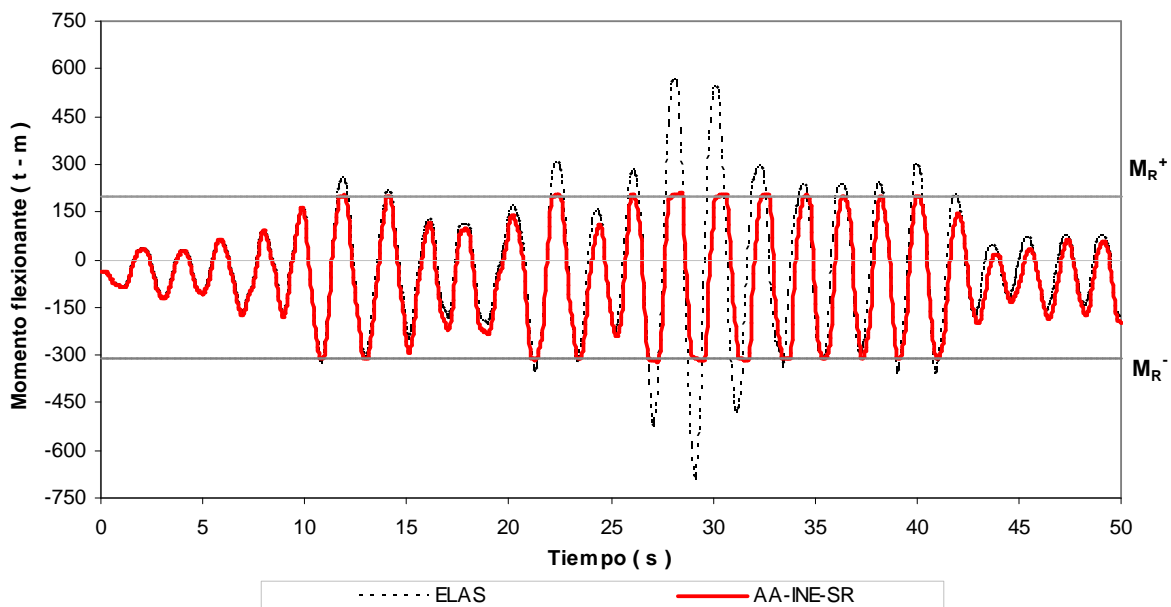
Fig 4.82.- Historias de momentos flexionantes en el extremo izquierdo de la viga 1, edificio 17 niveles, caso B (Apéndice A) con sobre-resistencias
