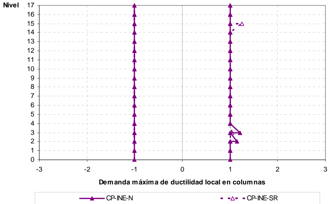
Fig 4.95.- Demandas máximas de ductilidad local en columnas, edificio 17 niveles, caso A (Cuerpo Principal) con resistencias nominales y con sobre-resistencias
