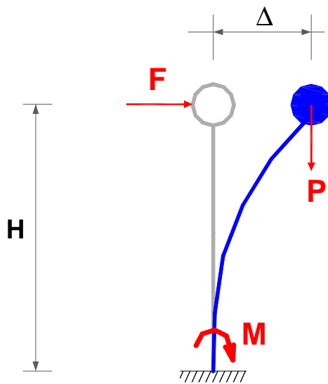
Fig 2.6.- Efectos P-Δ
