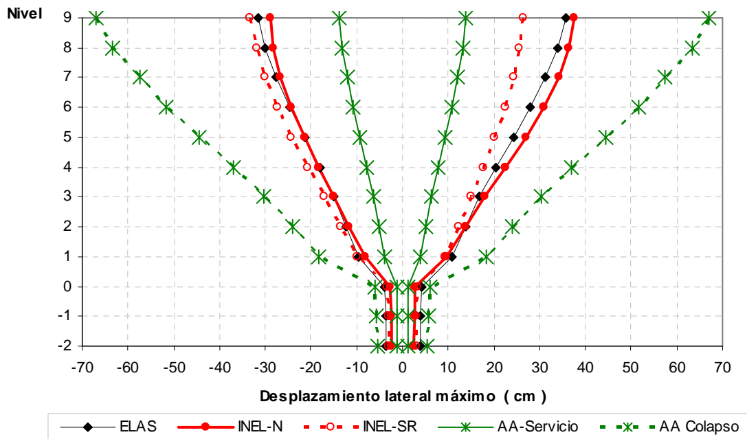
Fig 4.4.- Desplazamientos horizontales máximos, edificio 9 niveles, caso B
