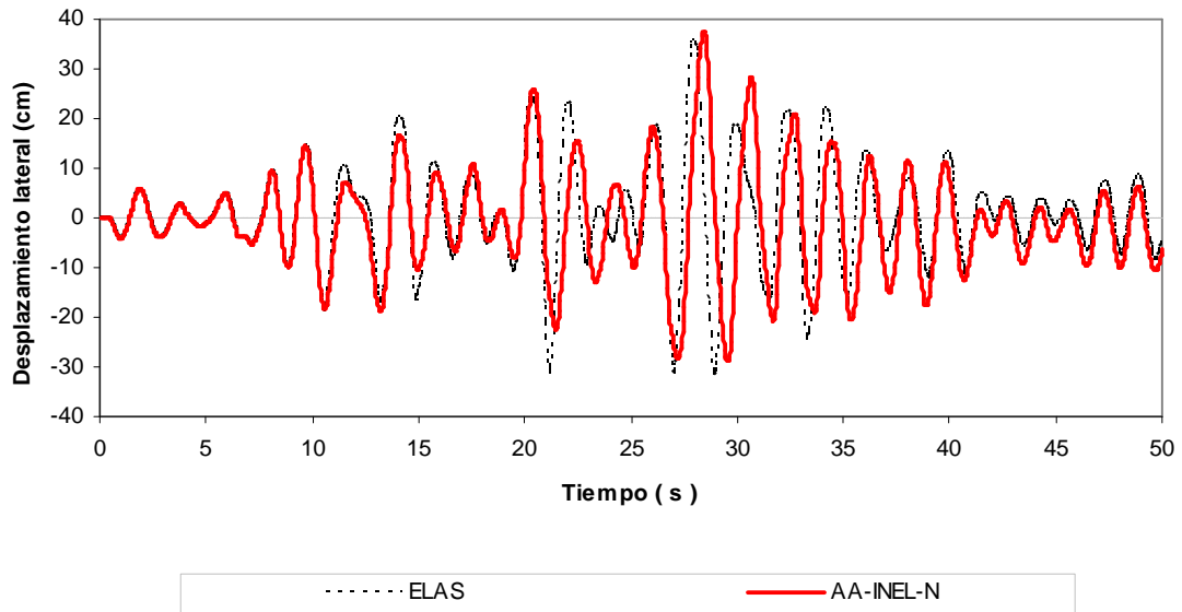
Fig 4.7.- Historia de desplazamientos de azotea, edificio 9 niveles, caso B (Apéndice A) con resistencias nominales
