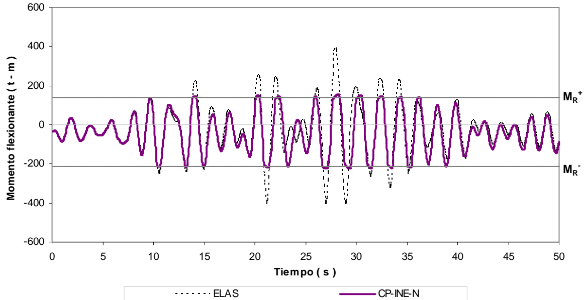
Fig 4.31.- Historias de momentos flexionantes en el extremo izquierdo de la viga 1, edificio 9 niveles, caso A (Cuerpo Principal) con resistencias nominales
