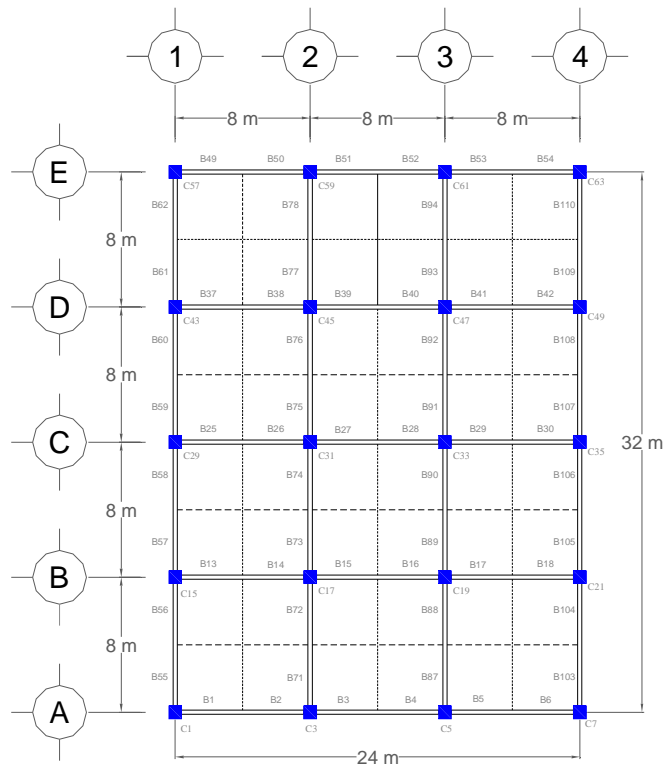
Fig 3.2b.- Planta tipo del edificio de 9 niveles
