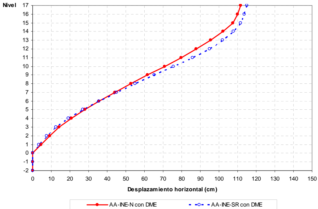
Fig 4.120.- Desplazamientos horizontales máximos, edificio 17 niveles, caso B con resistencias nominales y sobre-resistencias, distribución de fuerzas laterales del análisis dinámico modal espectral
