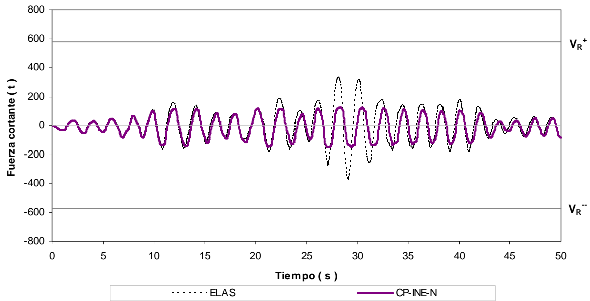
Fig 4.75.- Historias de fuerzas cortantes en el extremo inferior de la columna 1, edificio 17 niveles, caso A (Cuerpo Principal) con resistencias nominales
