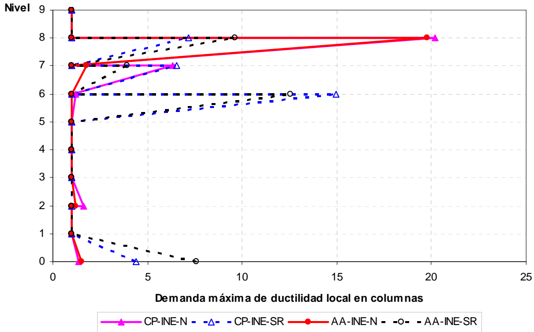
Fig 5.48.- Comparación de demandas máximas de ductilidad local en columnas, análisis estático no-lineal (Push-over), edificio de 9 niveles con resistencias nominales y sobre-resistencias, caso A (Cuerpo Principal) y B (Apéndice A)
