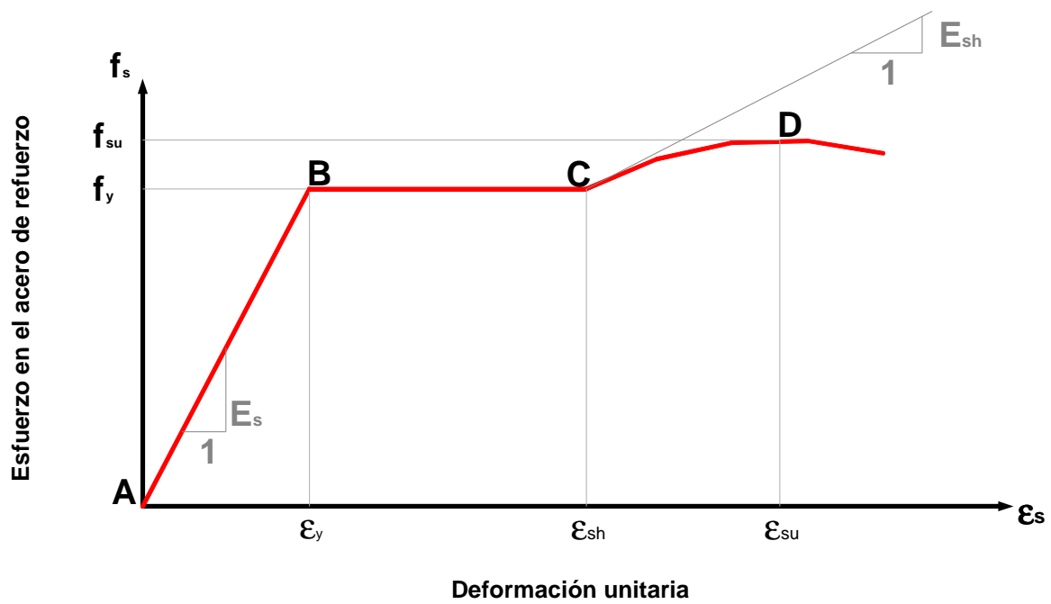
Fig 2.20.- Curva esfuerzo-deformación para el acero, considerando la etapa del endurecimiento por deformación
