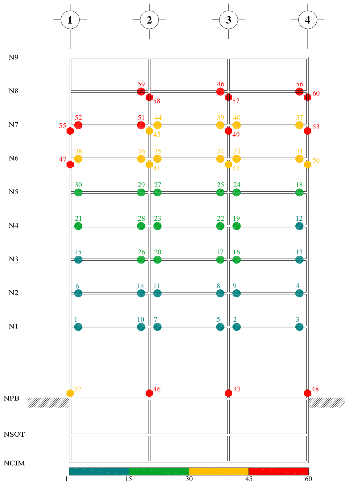
Fig A.10.- Secuencia de formación de articulaciones plásticas, análisis estático no-lineal (Push-over) con distribución de cargas laterales de análisis paso a paso elástico, resistencias nominales, edificio 9 niveles, caso A (Cuerpo Principal)
