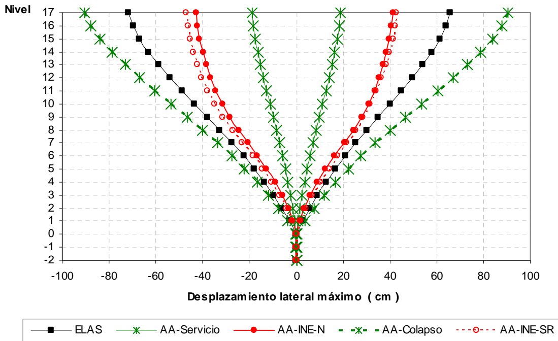
Fig 4.52.- Desplazamientos horizontales máximos, edificio 17 niveles, caso B
