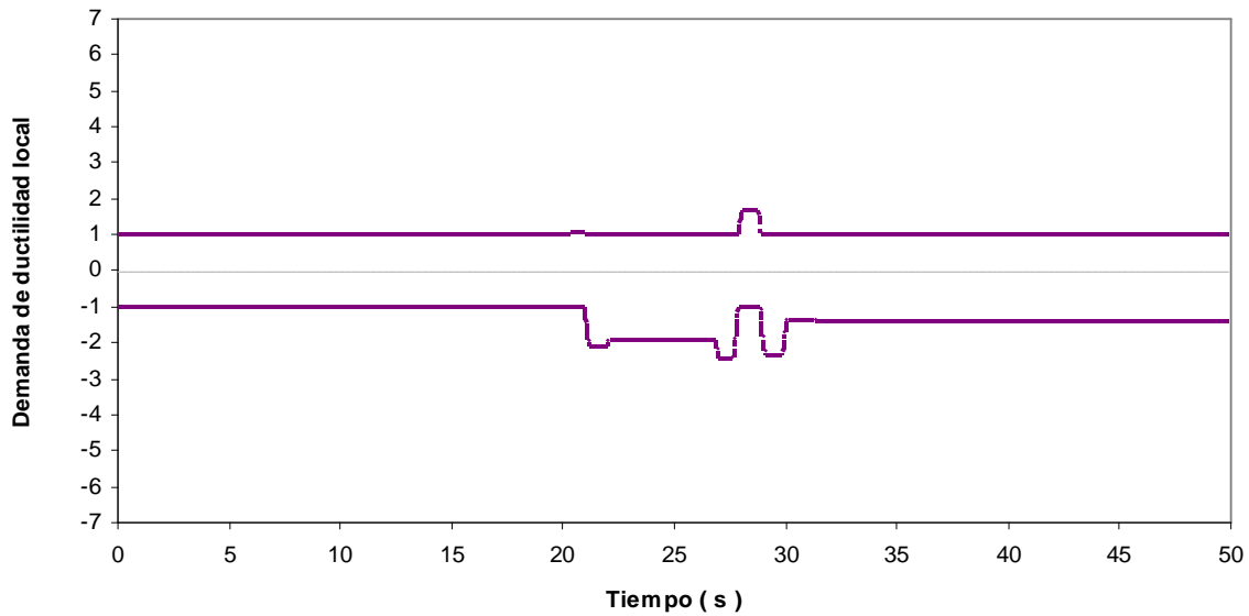
Fig 4.40.- Historias de demandas de ductilidad el extremo izquierdo de la viga 1, edificio 9 niveles, caso A (Cuerpo Principal) con sobre-resistencias
