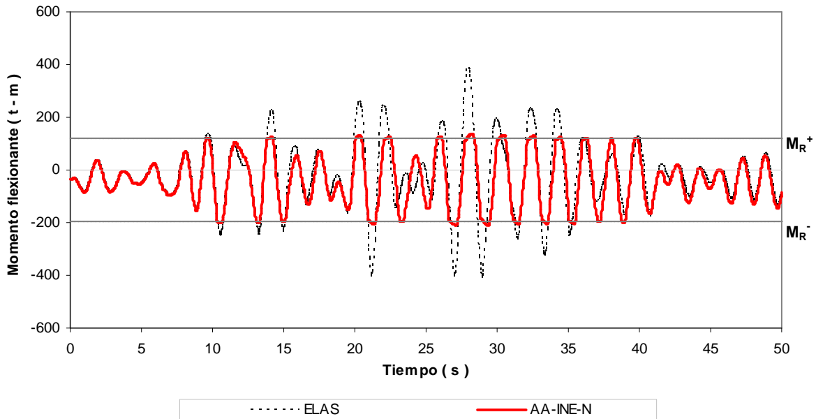
Fig 4.33.- Historias de momentos flexionantes en el extremo izquierdo de la viga 1, edificio 9 niveles, caso B (Apéndice A) con resistencias nominales
