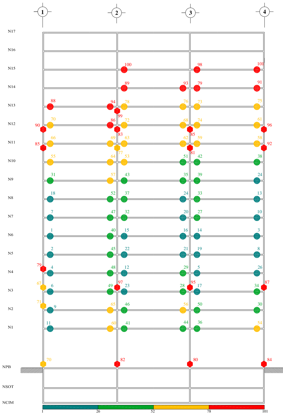
Fig A.28.- Secuencia de formación de articulaciones plásticas, análisis estático no-lineal (Push-over) con distribución de cargas laterales de análisis paso a paso inelástico, resistencias nominales, edificio 17 niveles, caso B (Apéndice A)
