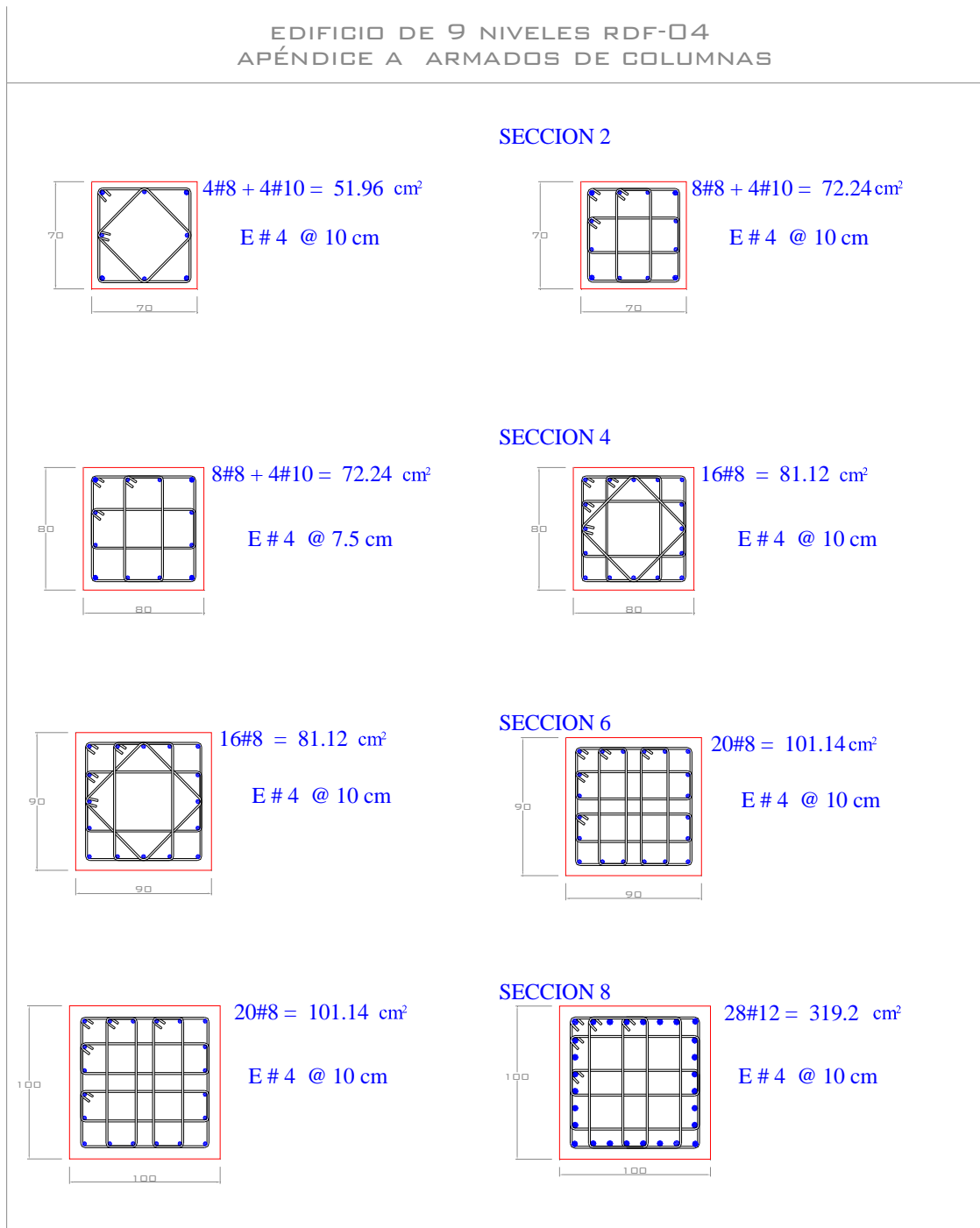
Fig 3.19.- Armados de acero longitudinal y transversal propuestos en columnas del eje C, edificio 9 niveles, Apéndice A (caso B) de las NTC-Sismo, RDF-04
