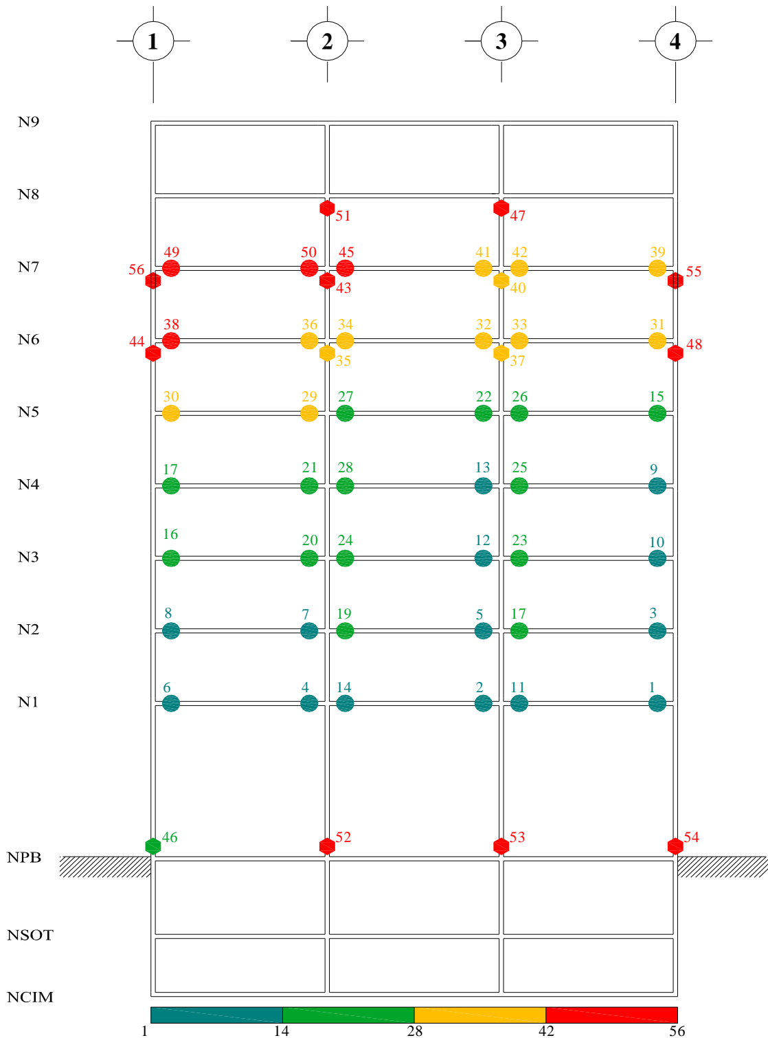
Fig 4.108.- Mecanismo de falla y secuencia de formación de articulaciones plásticas, edificio 9 niveles, caso A (Cuerpo Principal) con sobre-resistencias, distribución de fuerzas laterales del análisis paso a paso inelástico para \Delta_{máx}
