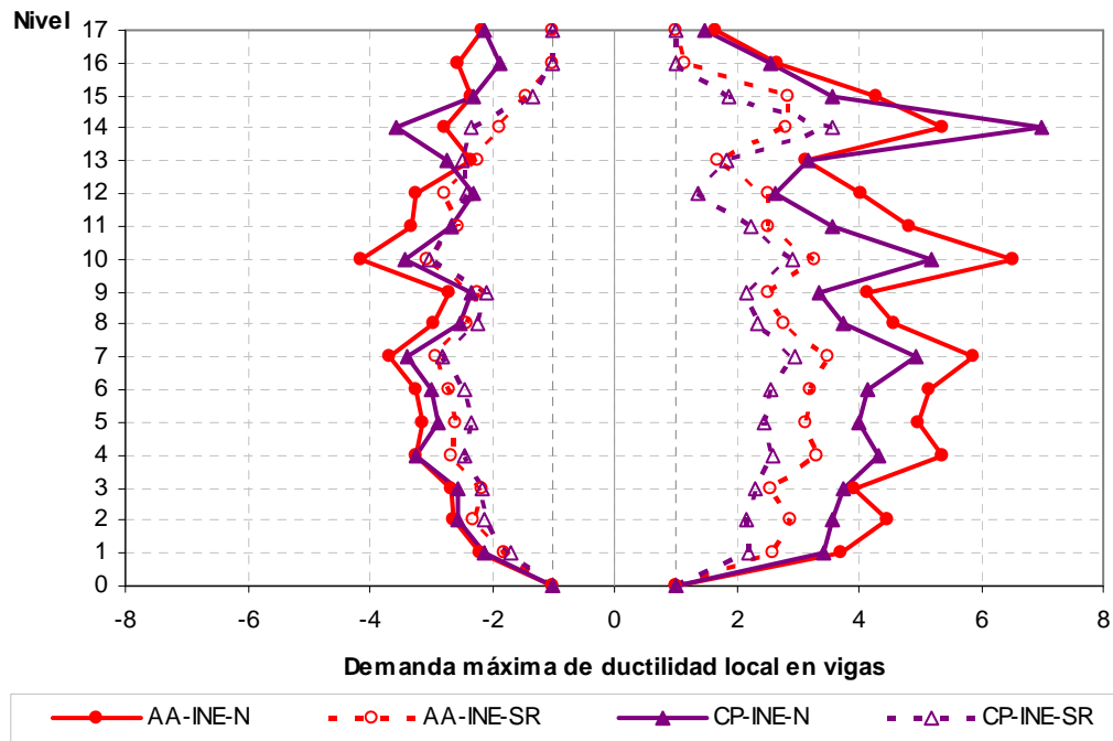
Fig 5.29.- Comparación de demandas máximas de ductilidad local en vigas, análisis paso a paso inelástico (resistencias nominales y sobre-resistencias), edificio de 17 niveles, casos A (Cuerpo Principal) y B (Apéndice A)
