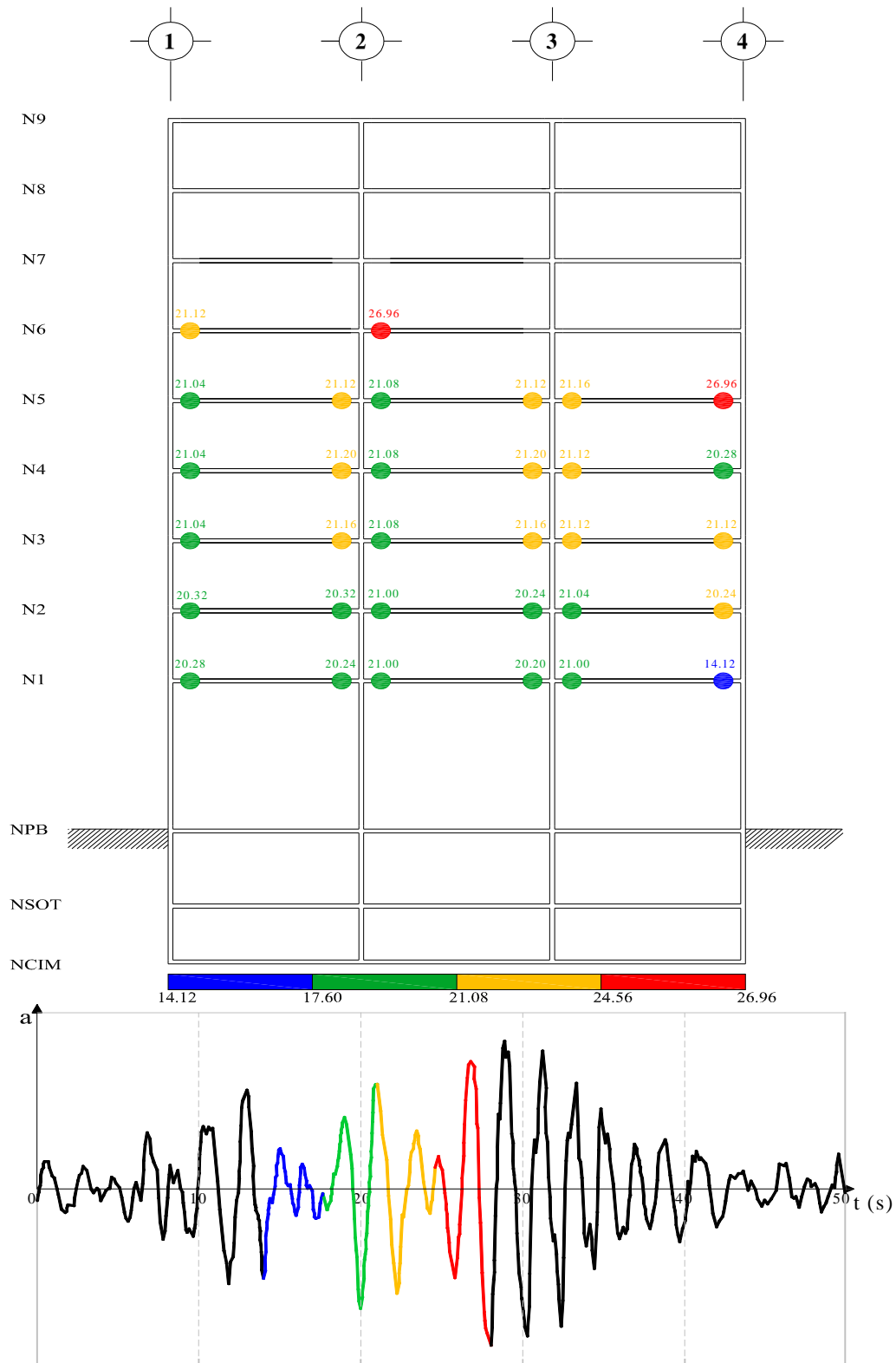
Fig 4.44.- Secuencia de formación y distribución global de articulaciones plásticas, edificio 9 niveles, caso A con sobre-resistencias
