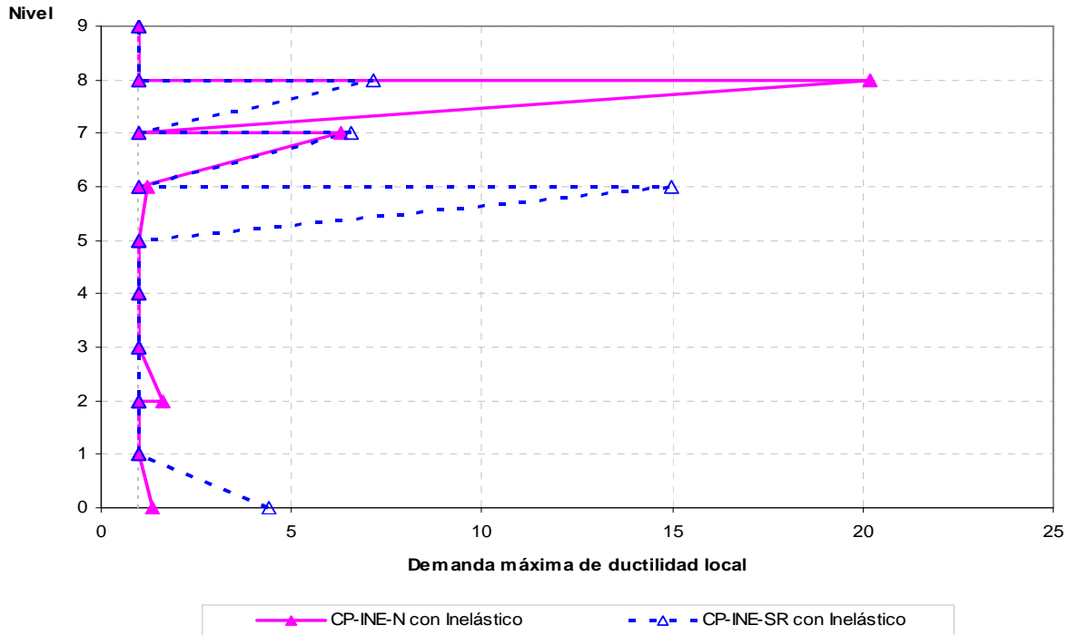
Fig 4.113.- Demandas máximas de ductilidad local en columnas, edificio 9 niveles, caso A (Cuerpo Principal) con resistencias nominales y sobre-resistencias, distribución de fuerzas laterales del análisis paso a paso inelástico para \Delta_{m\acute{a}x}
