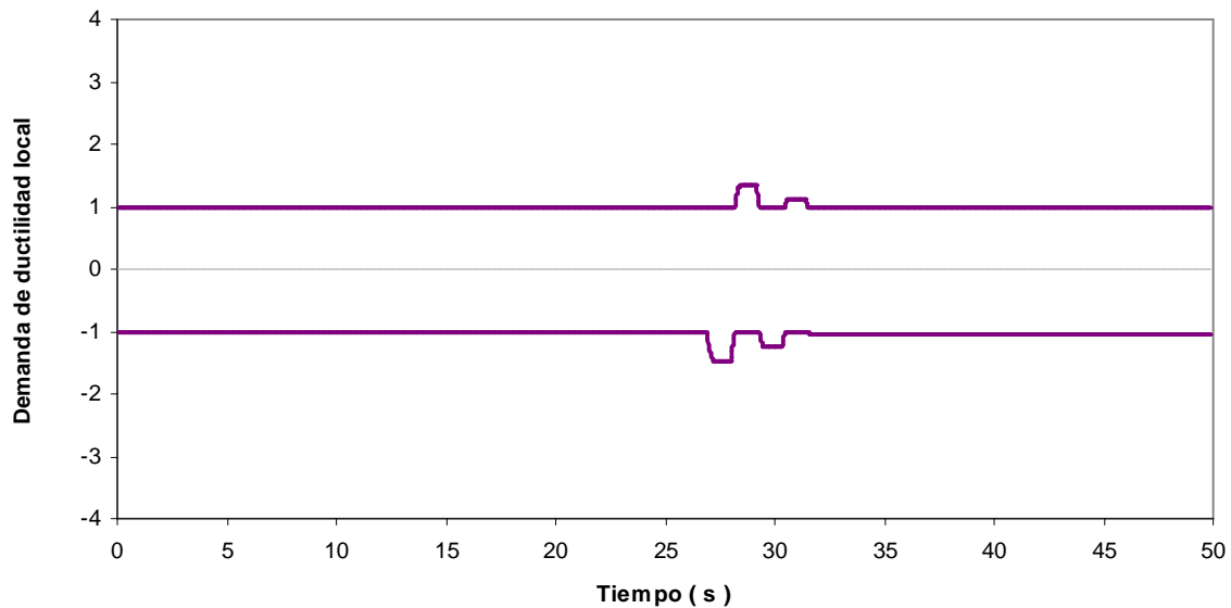
Fig 4.88.- Historias de demandas de ductilidad en el extremo izquierdo de la viga 1, edificio 17 niveles, caso A (Cuerpo Principal) con sobre-resistencias
