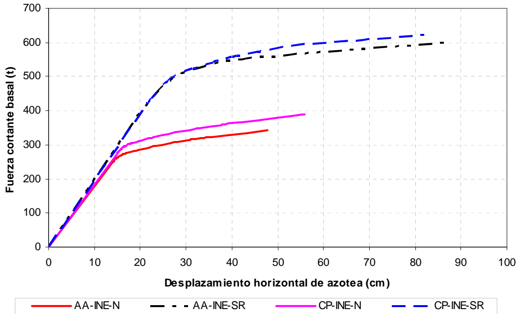
Fig 5.32.- Comparación de relaciones fuerza cortante basal-desplazamiento horizontal de azotea, análisis estático no-lineal (Push-over) con resistencias nominales y sobre-resistencias, edificio de 9 niveles, casos A (Cuerpo Principal) y B (Apéndice A)
