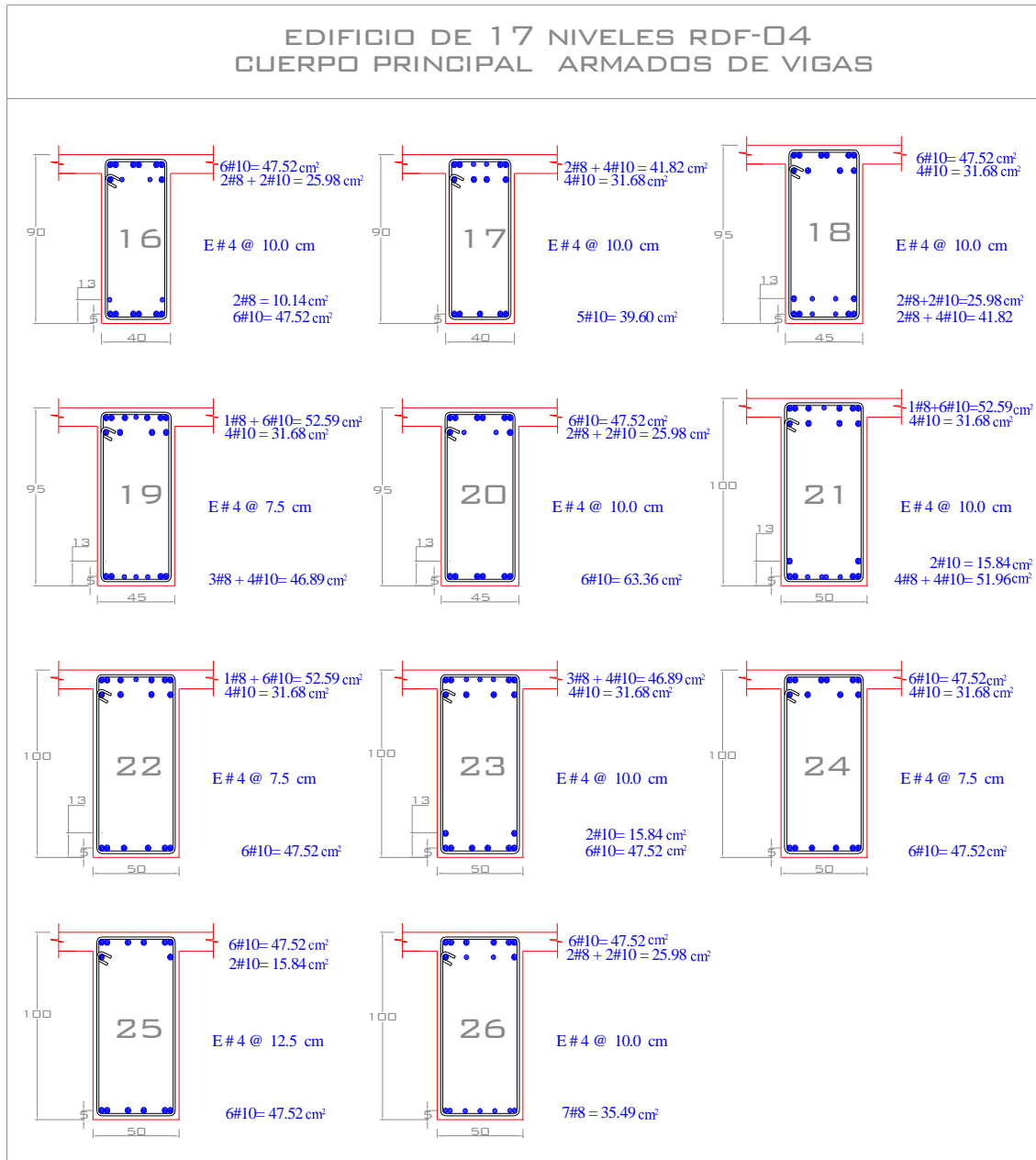
Fig 3.29b.- Armados longitudinal y transversal propuestos de vigas, edificio 17 niveles, Cuerpo Principal (caso A) de las NTC-Sismo, RDF-04
