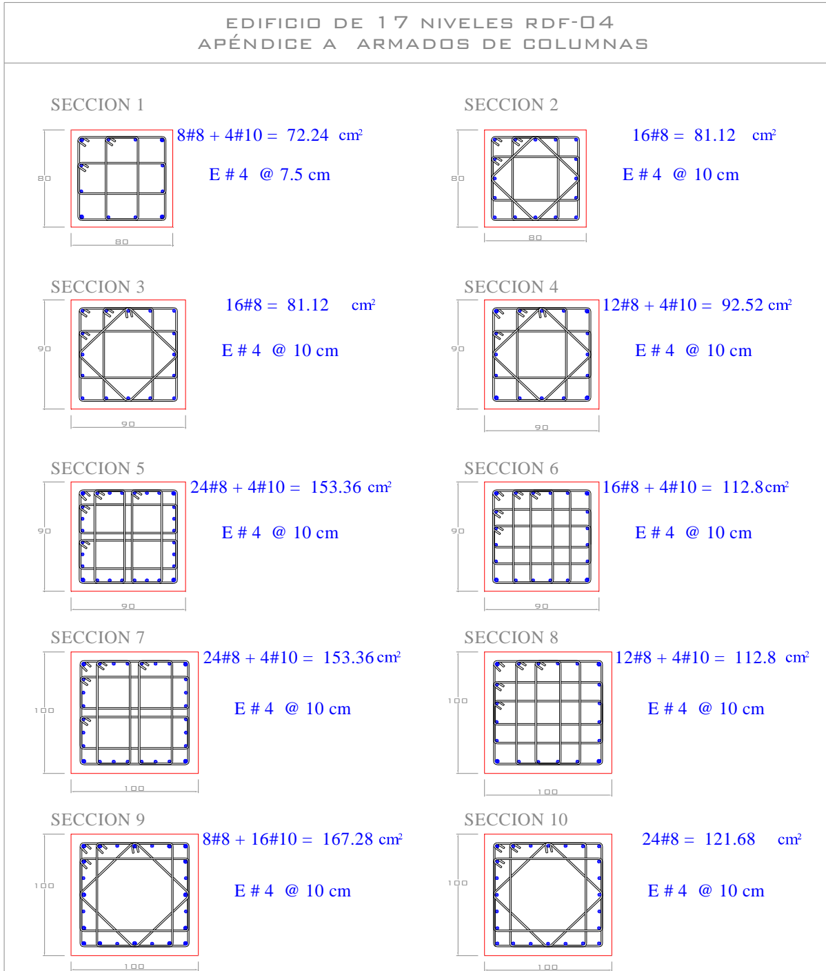
Fig 3.34a.- Armados de acero longitudinal y transversal propuestos en columnas, edificio 17 niveles, Apéndice A (caso B) de las NTC-Sismo, RDF-04
