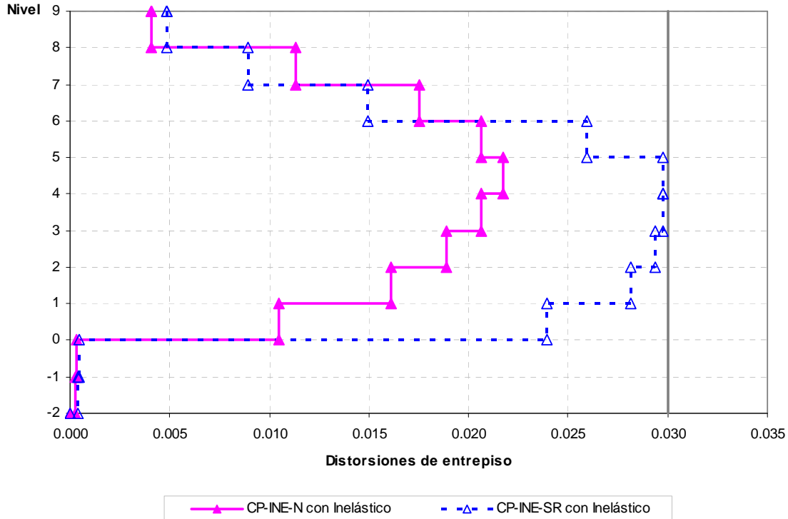
Fig 4.105.- Relaciones desplazamiento lateral relativo entre altura de entropiso, edificio 9 niveles, caso A con resistencias nominales y sobre-resistencias, distribución de cargas del análisis paso a paso inelástico para \Delta_{máx}
