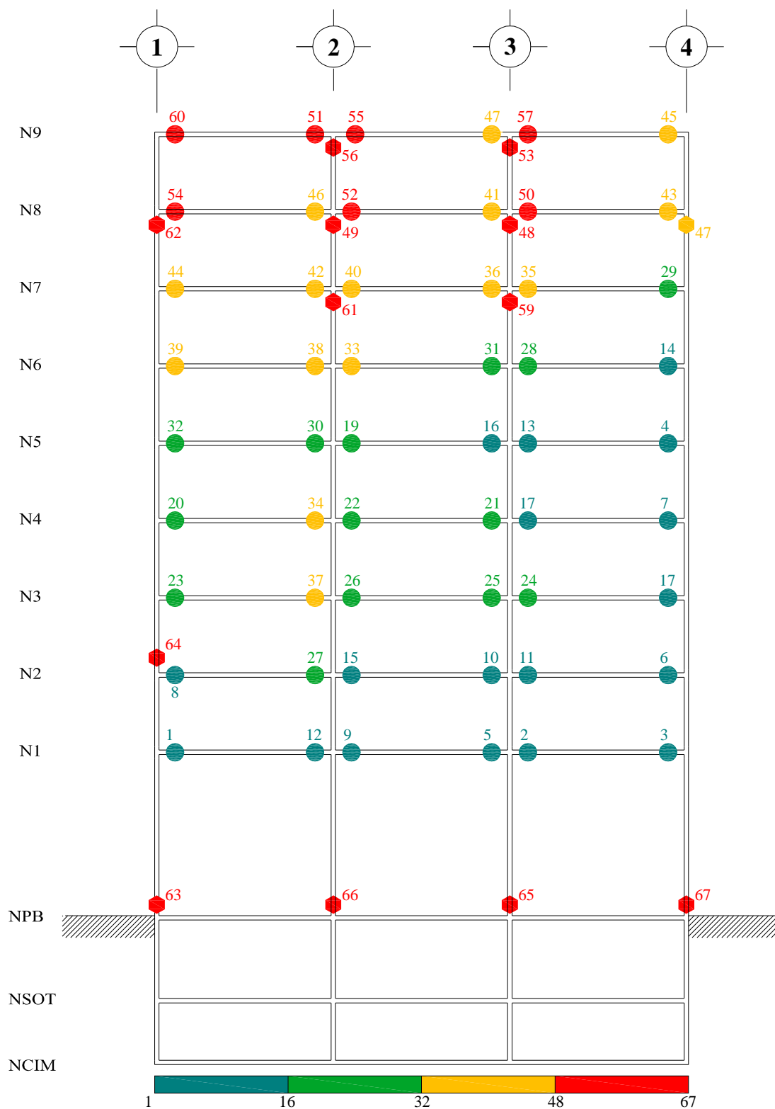
Fig A.9.- Secuencia de formación de articulaciones plásticas, análisis estático no-lineal (Push-over) con distribución de cargas laterales de análisis dinámico modal espectral (DME), resistencias nominales, edificio 9 niveles, caso A (Cuerpo Principal)
