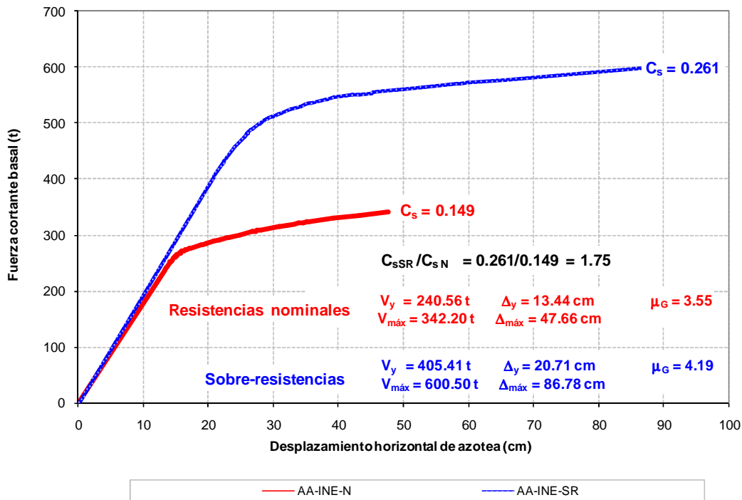
Fig 4.102.- Curvas fuerza cortante basal-desplazamiento lateral de azotea, edificio 9 niveles, caso B (Apéndice A) con resistencias nominales y sobre-resistencias, distribución de fuerzas laterales del análisis paso a paso inelástico para \Delta_{máx}
