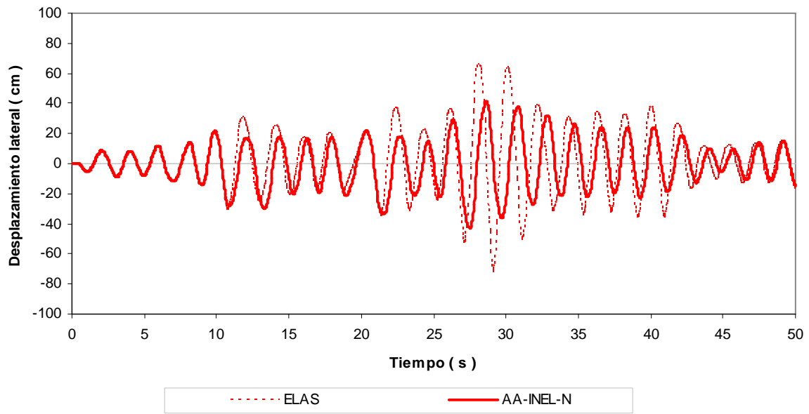
Fig 4.55.- Historia de desplazamientos de azotea, edificio 17 niveles, caso B (Apéndice A) con resistencias nominales
