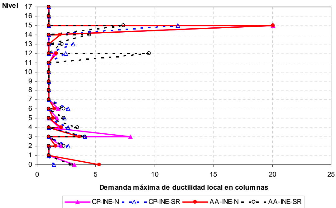
Fig 5.49.- Comparación de demandas máximas de ductilidad local en columnas, análisis estático no-lineal (Push-over), edificio de 17 niveles con resistencias nominales y sobre-resistencias, caso A (Cuerpo Principal) y B (Apéndice A)
