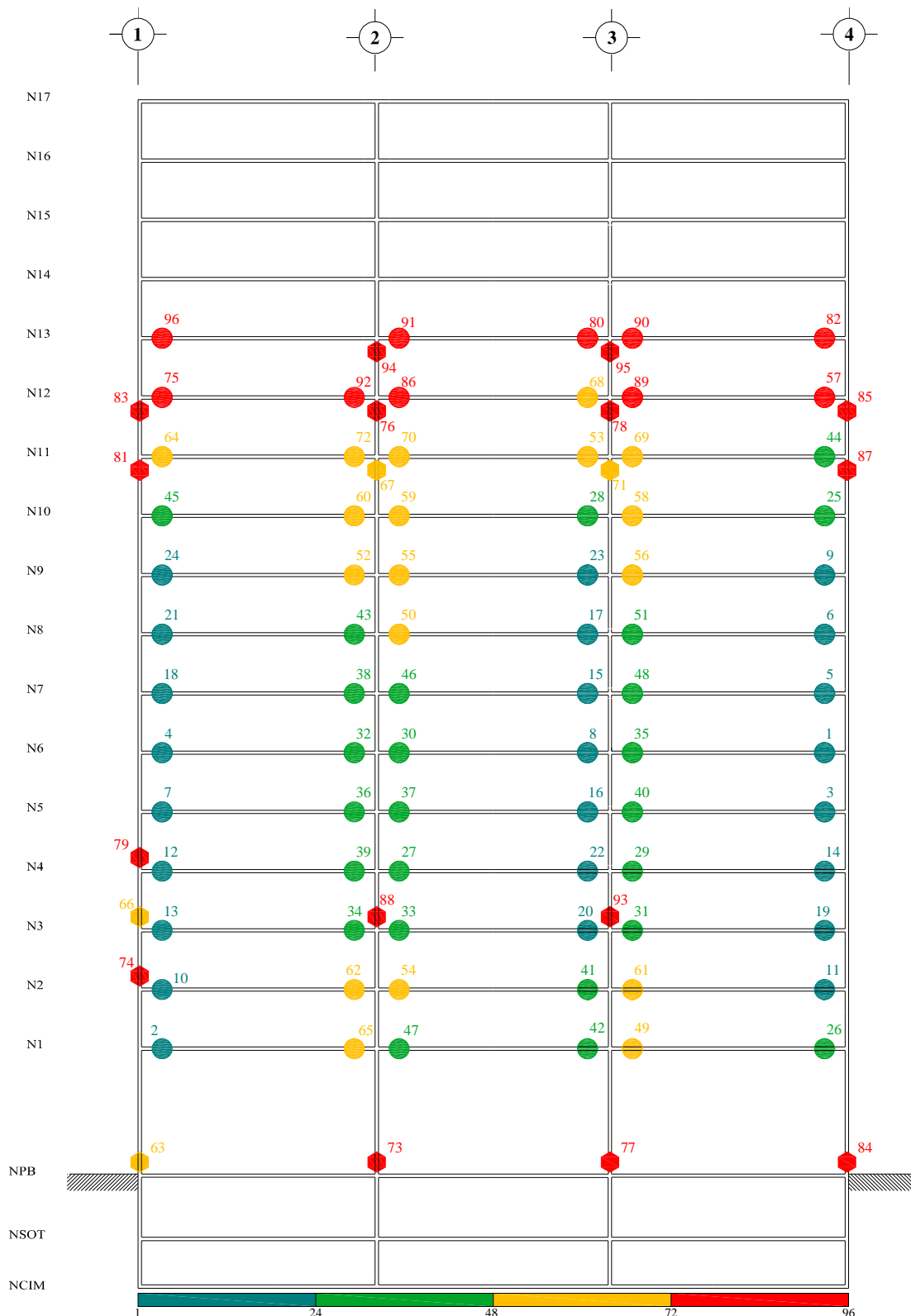
Fig A.30.- Secuencia de formación de articulaciones plásticas, análisis estático no-lineal (Push-over) con distribución de cargas laterales de análisis paso a paso elástico, sobre-resistencia, edificio 17 niveles, caso B (Apéndice A)
