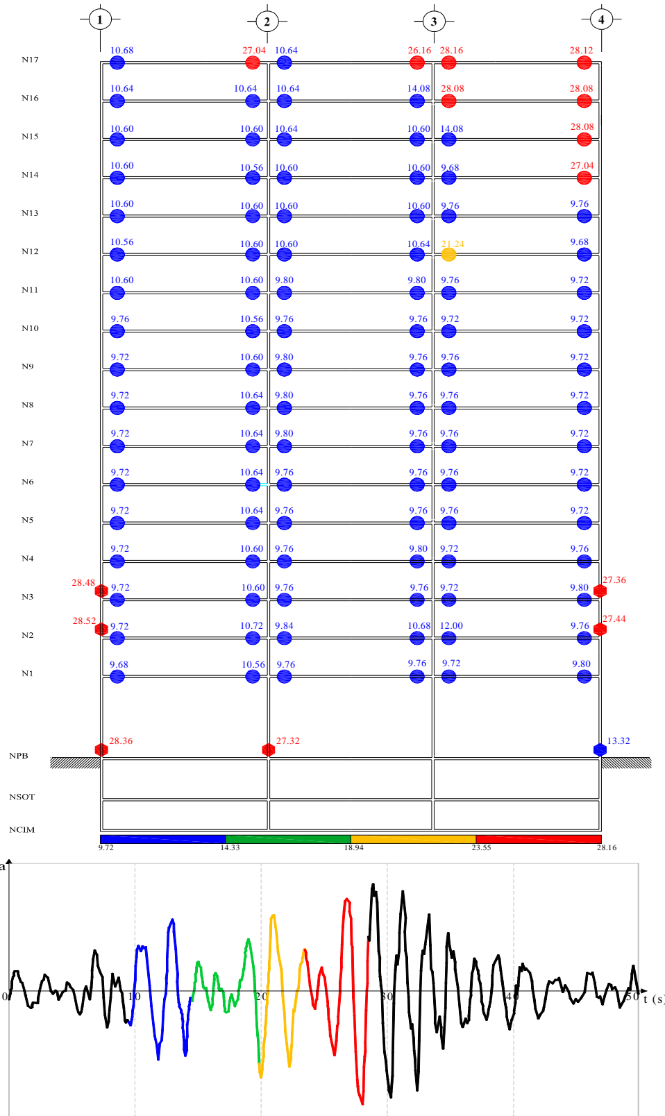
Fig 4.93.- Secuencia de formación y distribución global de articulaciones plásticas, edificio 17 niveles, caso B con resistencias nominales
