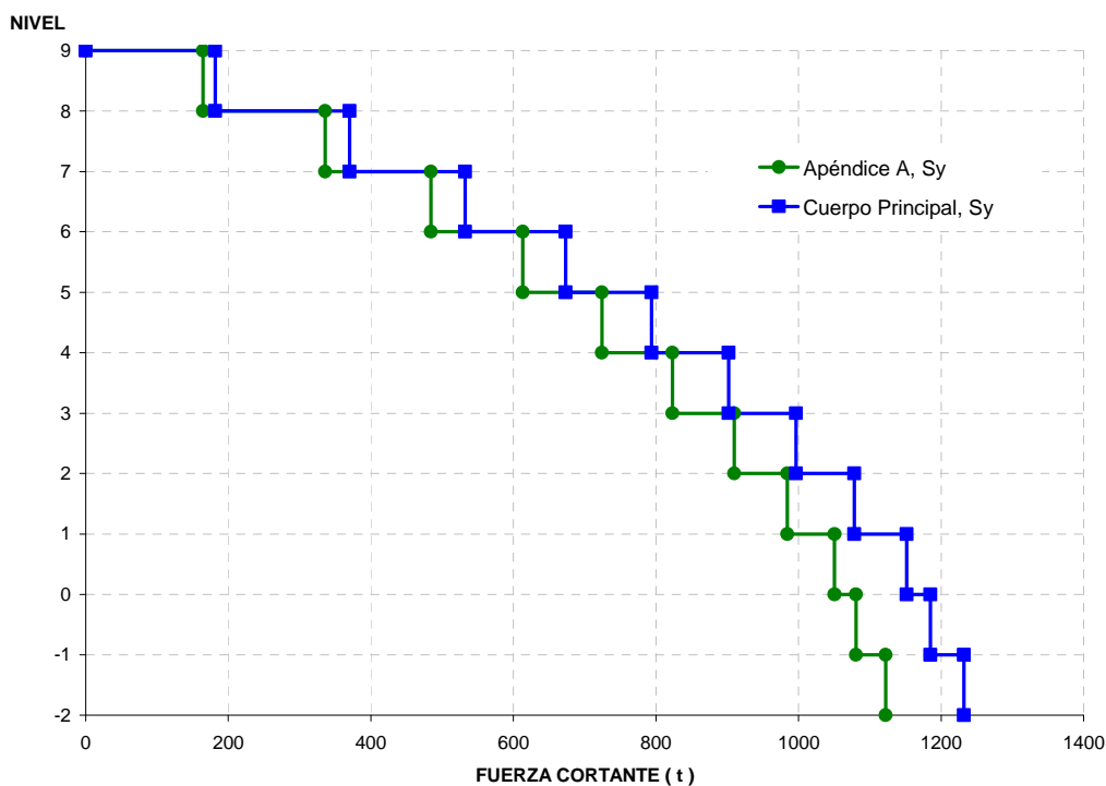
Fig 3.10.- Fuerzas cortantes de entrepiso, sismo en dirección "Y", edificio 9 niveles, Apéndice A y Cuerpo Principal de las NTC-Sismo, RDF-04
