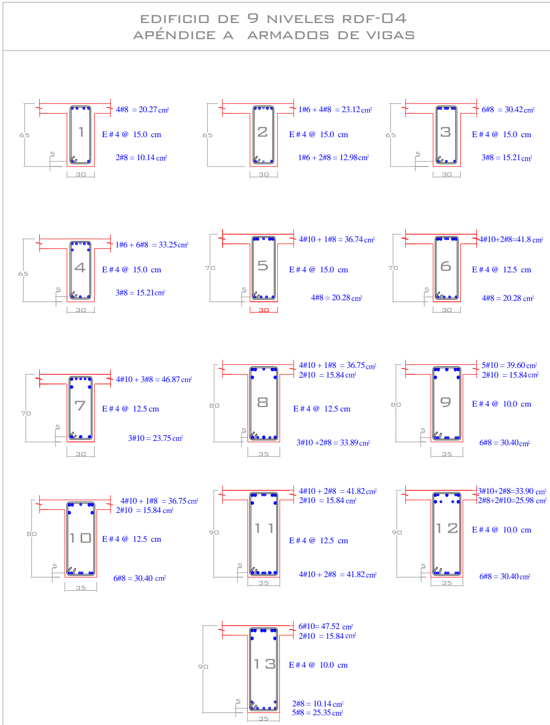
Fig 3.15.- Armados longitudinal y transversal propuestos de las vigas del eje C, edificio 9 niveles, Apéndice A (caso B) de las NTC-Sismo, RDF-04
