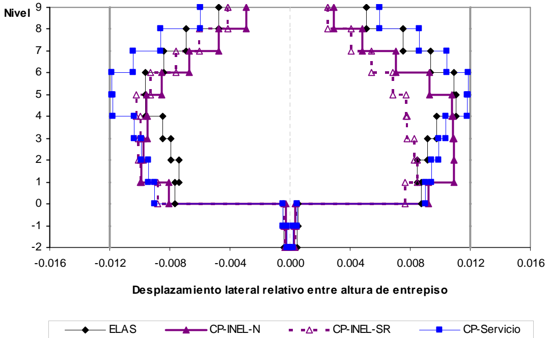
Fig 4.9.- Relaciones desplazamiento lateral relativo entre altura de entrepiso, edificio 9 niveles, caso A (Cuerpo Principal)
