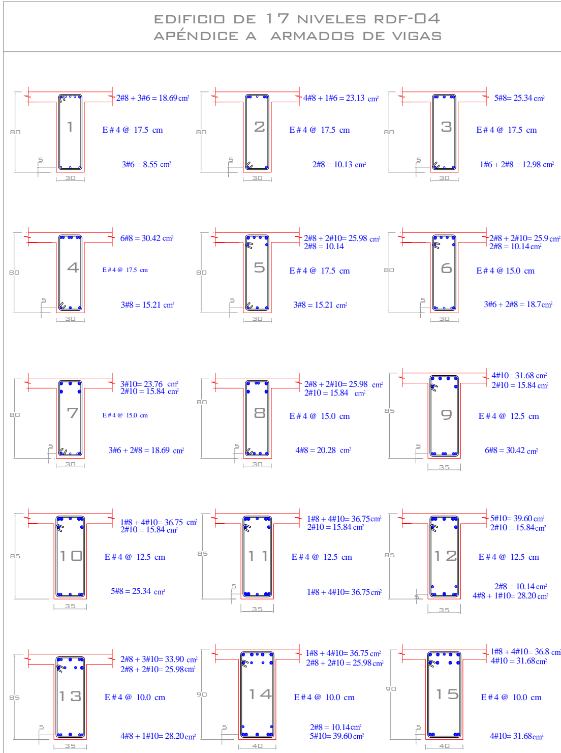
Fig 3.30a.- Armados longitudinal y transversal propuestos de vigas, edificio 17 niveles, Apéndice A (caso B) de las NTC-Sismo, RDF-04
