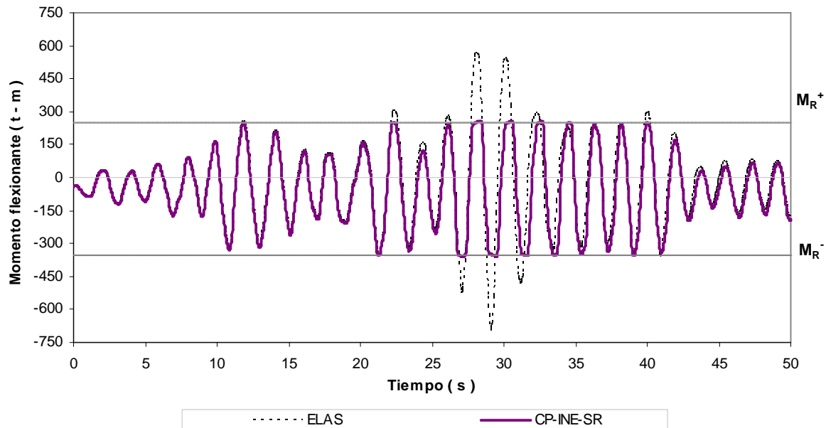
Fig 4.80.- Historias de momentos flexionantes en el extremo izquierdo de la viga 1, edificio 17 niveles, caso A (Cuerpo Principal) con sobre-resistencias
