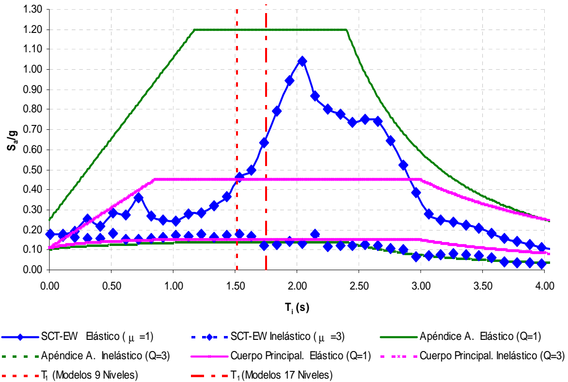
Fig 5.1.- Ubicación de los periodos fundamentales de vibración de los edificios de 9 y 17 niveles con respecto de los espectros de diseño del Cuerpo Principal ( Q=1 y 3 ) y Apéndice A ( Q=1 y 3 ) de las NTC-Sismo del RDF-04, y de los espectros de respuesta del registro SCT-EW-85 ( \mu = 1 y 3 )
