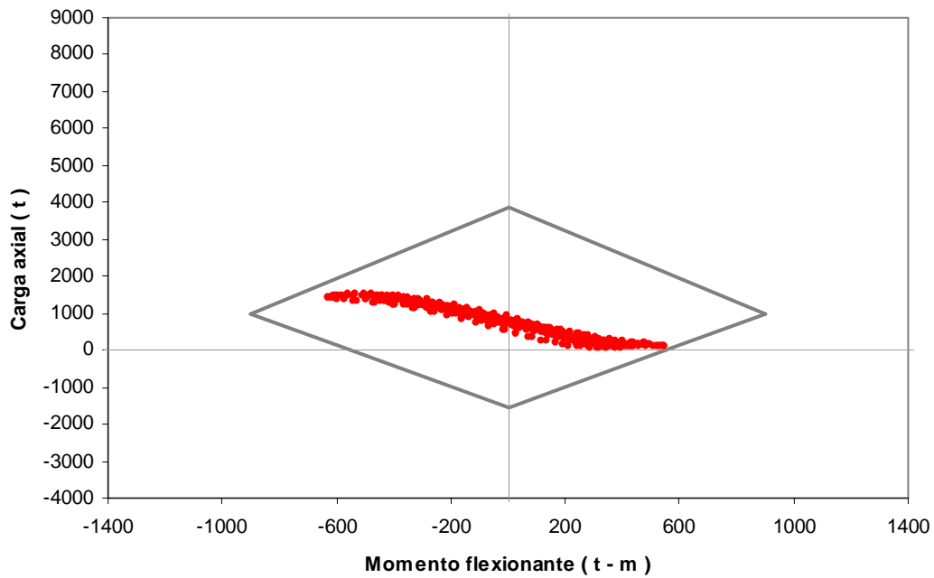
Fig 4.73.- Combinaciones momento flexionante-carga axial del extremo inferior de la columna 1, edificio 17 niveles, caso B (Apéndice A) con resistencias nominales
