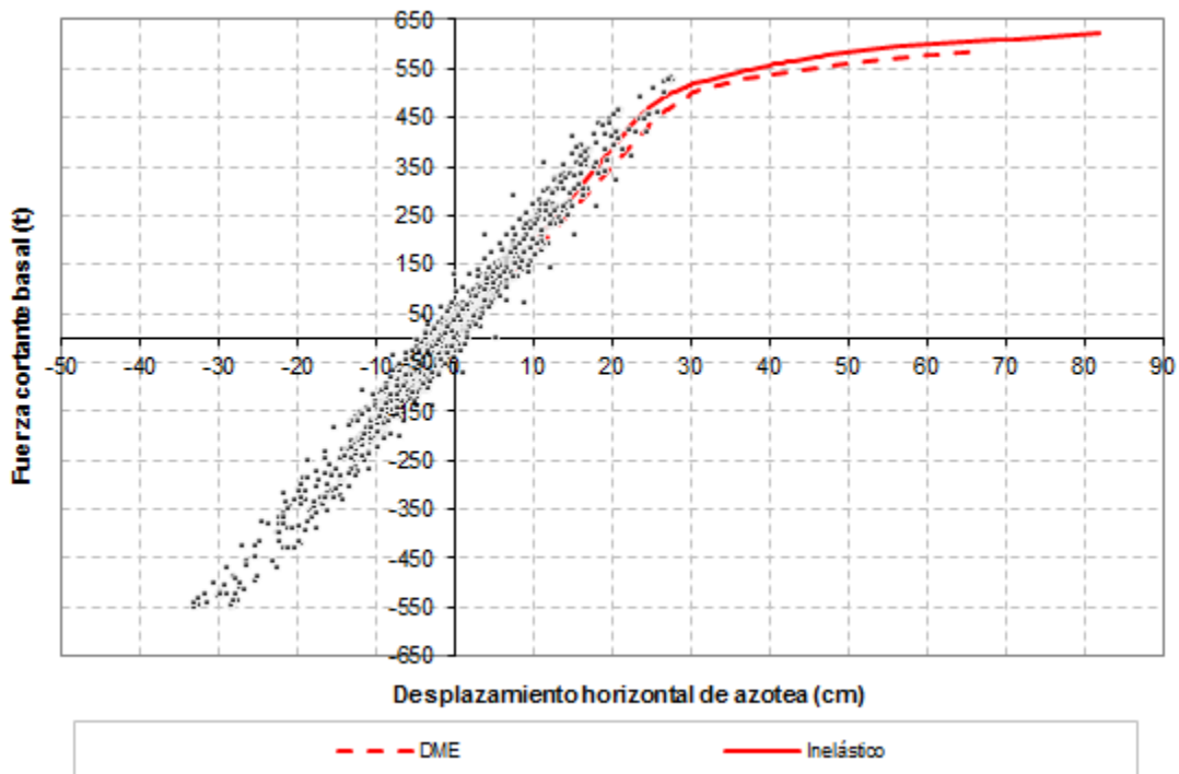
Fig 5.35.- Comparación de relaciones fuerza cortante basal-desplazamiento horizontal de azotea, análisis estático no-lineal (Push-over) y análisis paso a paso inelástico con sobre-resistencias, edificio de 9 niveles, caso A (Cuerpo Principal)
