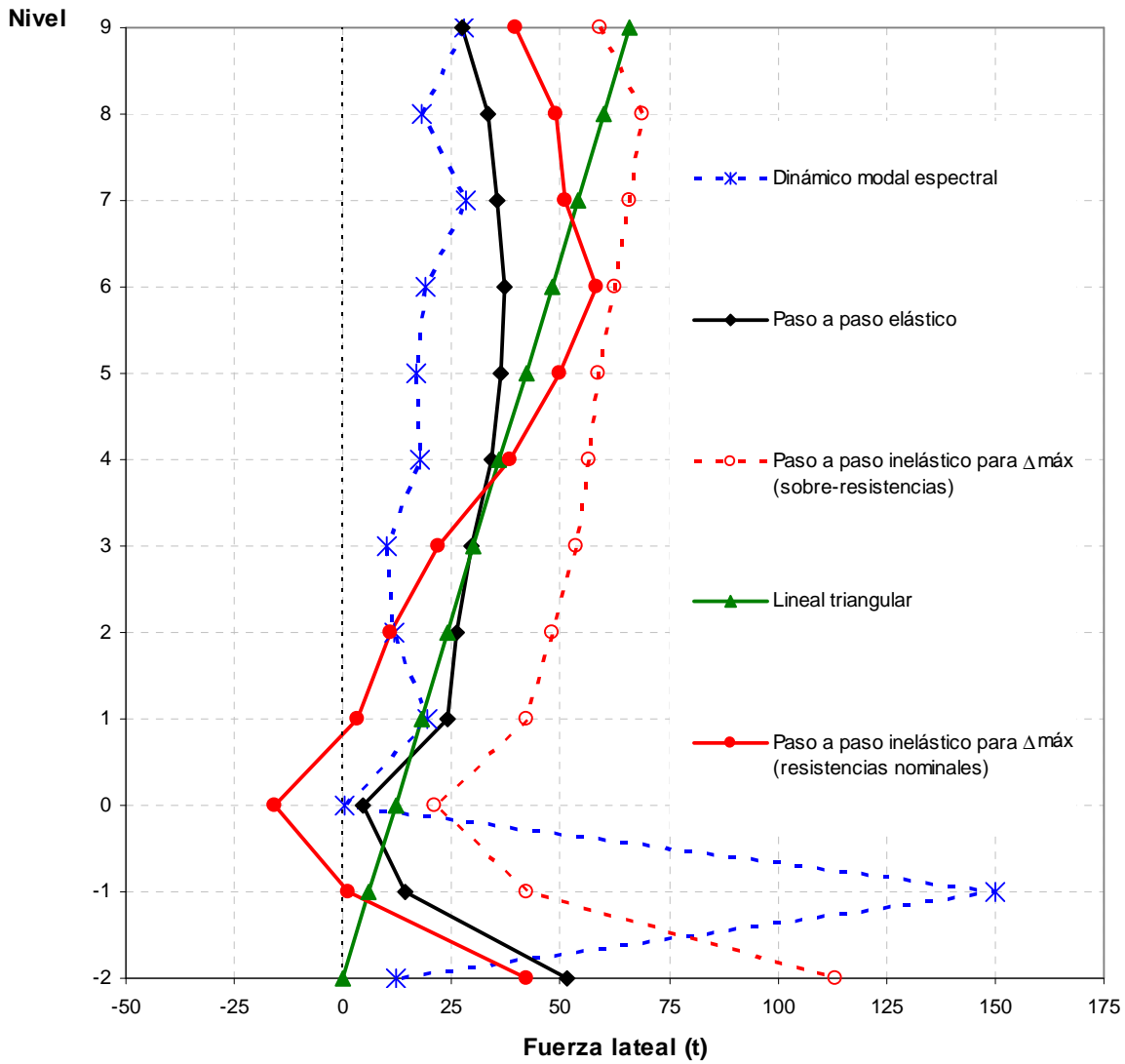
Fig 4.100.- Distribuciones de cargas laterales para el análisis estático no-lineal (Push-over), edificio 9 niveles, caso B (Apéndice A)
