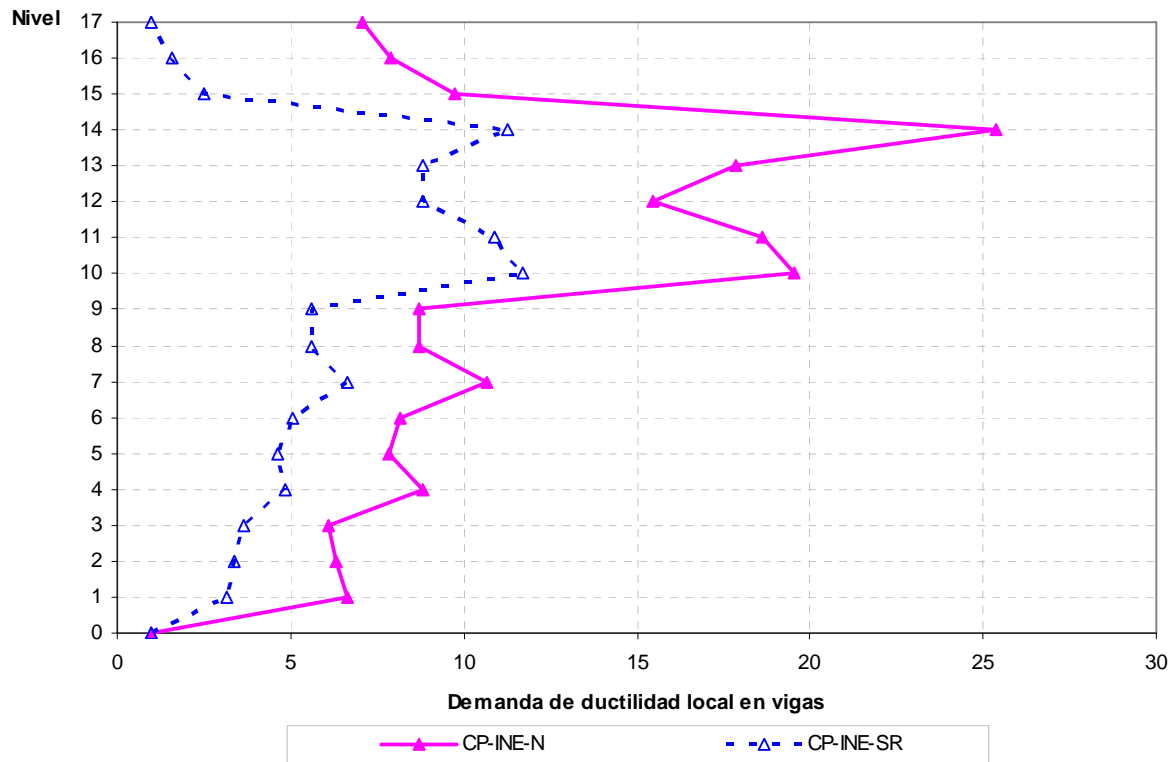
Fig 4.127.- Demandas máximas de ductilidad local en vigas, edificio 17 niveles, caso A (Cuerpo Principal) con resistencias nominales y sobre-resistencias, distribución de fuerzas laterales del análisis dinámico modal espectral
