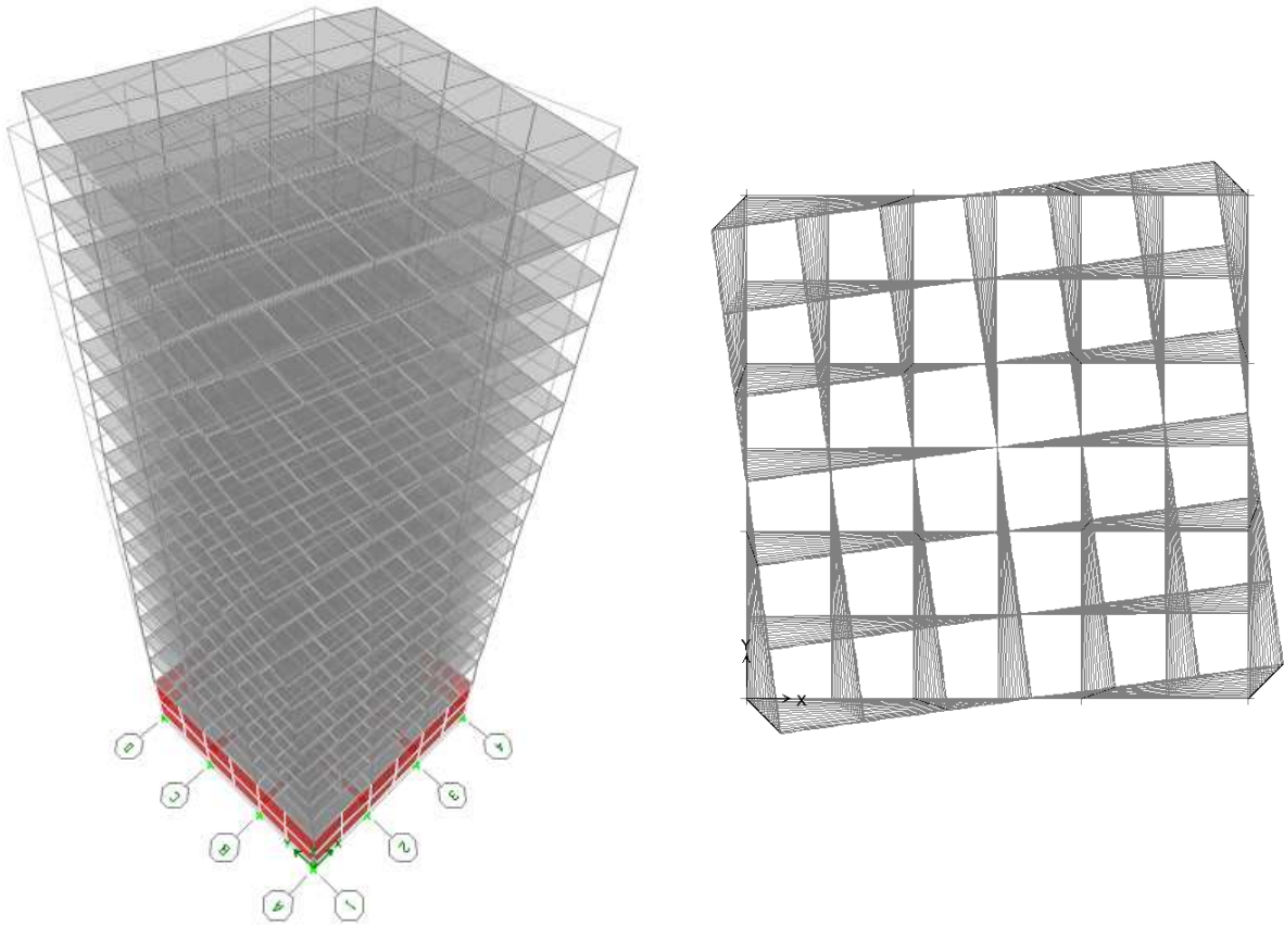
Fig 3.22c.- Vista en elevación y planta de la deformada del tercer modo de vibrar del edificio de 17 niveles
