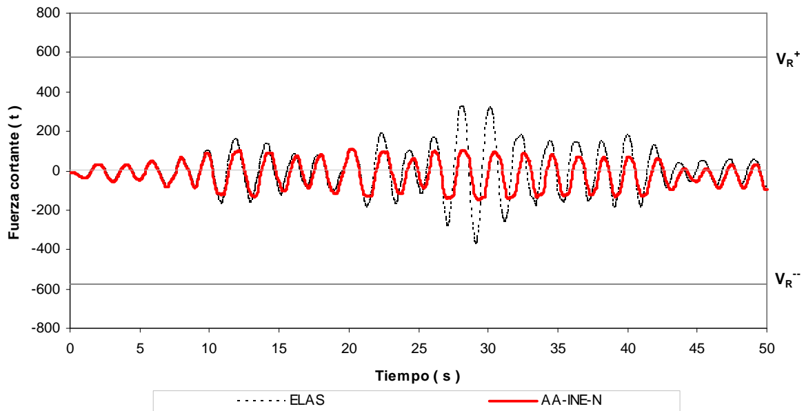
Fig 4.78.- Historias de fuerzas cortantes en el extremo inferior de la columna 1, edificio 17 niveles, caso B (Apéndice A) con sobre-resistencias
