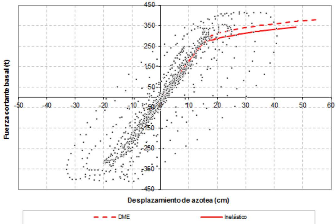
Fig 5.36.- Comparación de relaciones fuerza cortante basal-desplazamiento horizontal de azotea, análisis estático no-lineal (Push-over) y análisis paso a paso inelástico con resistencias nominales, edificio de 9 niveles, caso B (Apéndice A)
