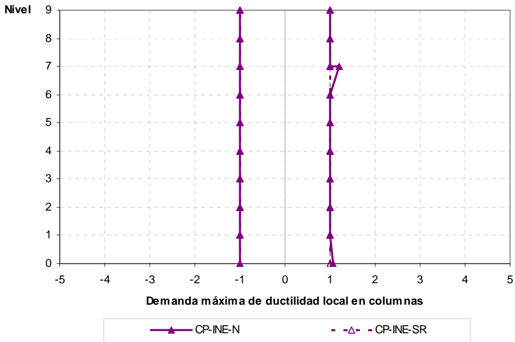
Fig 4.47.- Demandas máximas de ductilidad local en columnas, edificio 9 niveles, caso A (Cuerpo Principal) con resistencias nominales y con sobre-resistencias
