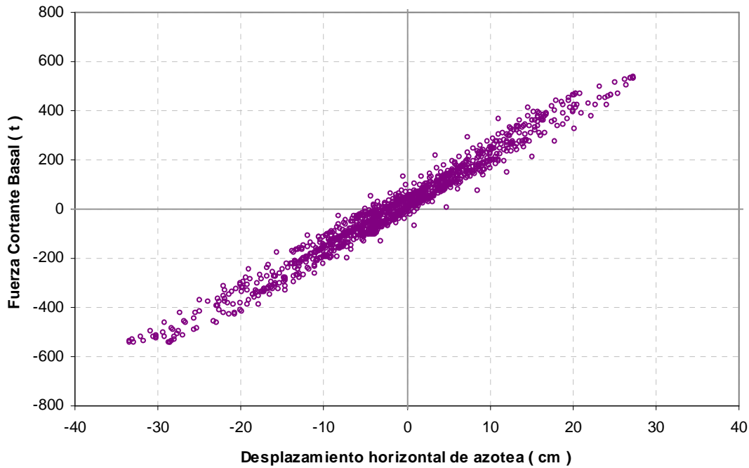
Fig 4.19.- Relaciones fuerza cortante basal – desplazamiento lateral de azotea, edificio 9 niveles, caso A (Cuerpo Principal), comportamiento inelástico con sobre-resistencias
