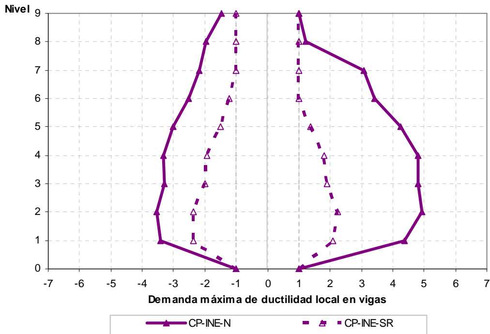
Fig 4.49.- Demandas máximas de ductilidad local en vigas, edificio 9 niveles, caso A (Cuerpo Principal) con resistencias nominales y con sobre-resistencias
