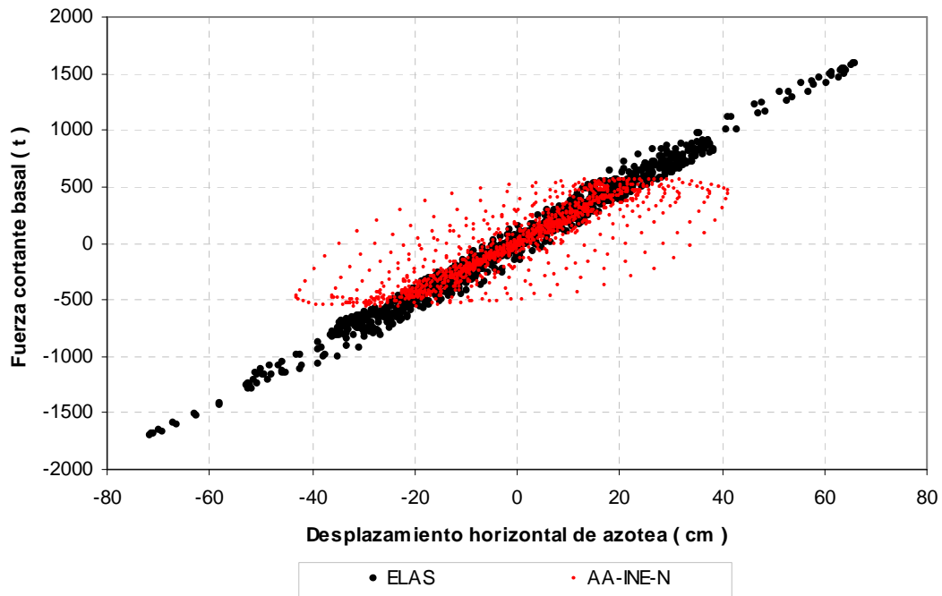
Fig 5.22.- Comparación de relaciones fuerza cortante basal-desplazamiento horizontal de azotea, análisis paso a paso elástico e inelástico (resistencias nominales), edificio de 17 niveles, caso B (Apéndice A)
