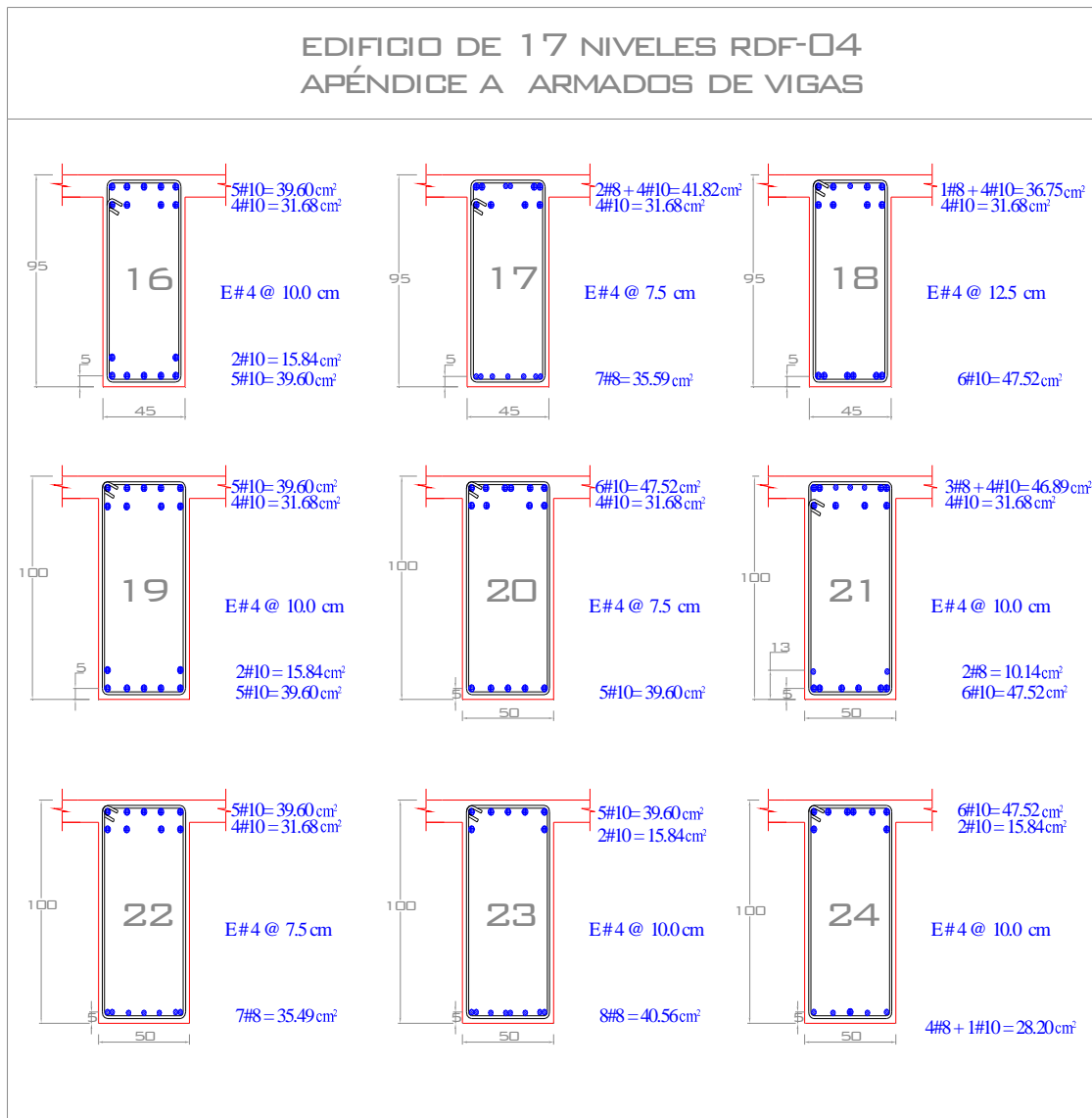
Fig 3.30b.- Armados longitudinal y transversal propuestos de vigas, edificio 17 niveles, Apéndice A (caso B) de las NTC-Sismo, RDF-04
