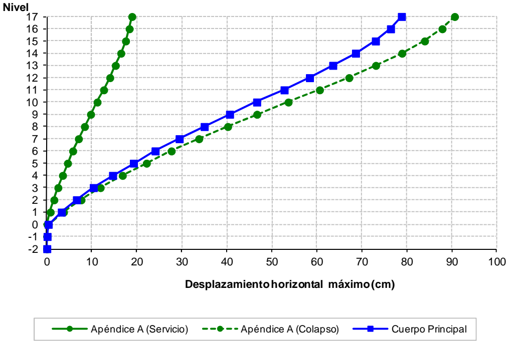
Fig 5.3.- Comparación de desplazamientos horizontales máximos de servicio y de colapso, análisis dinámico modal espectral, edificio de 17 niveles, casos A (Cuerpo Principal) y B (Apéndice A)
