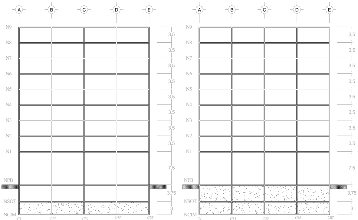
Fig 3.2d.- Cortes transversales interior y exterior en dirección larga "Y", edificio de 9 niveles
