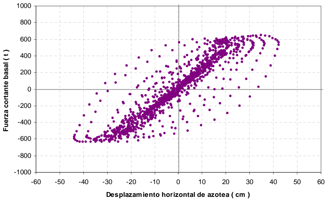
Fig 4.66.- Relaciones fuerza cortante basal – desplazamiento lateral de azotea, edificio 17 niveles, caso A (Cuerpo Principal), comportamiento inelástico con resistencias nominales
