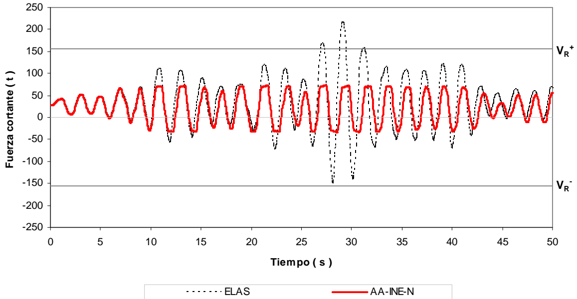
Fig 4.85.- Historias de fuerzas cortantes en el extremo izquierdo de la viga 1, edificio 17 niveles, caso B (Apéndice A) con resistencias nominales
