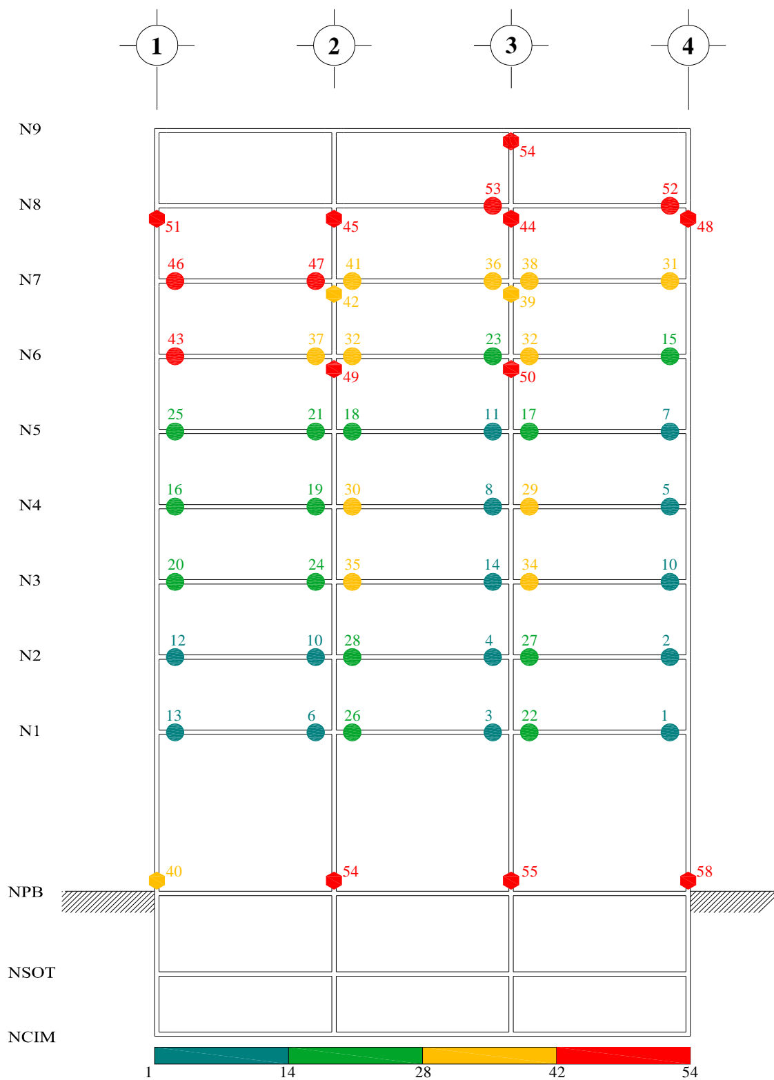
Fig A.14.- Secuencia de formación de articulaciones plásticas, análisis estático no-lineal (Push-over) con distribución de cargas laterales lineal triangular, sobre-resistencias, edificio 9 niveles, caso A (Cuerpo Principal)
