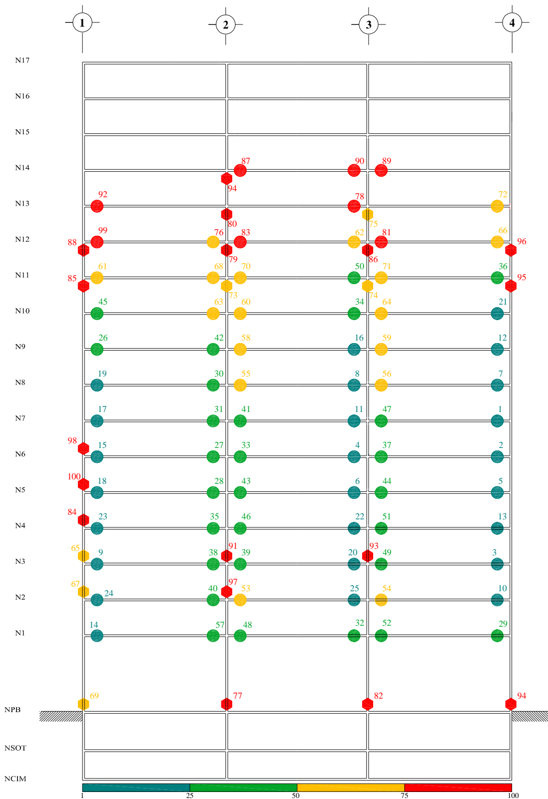
Fig A.24.- Secuencia de formación de articulaciones plásticas, análisis estático no-lineal (Push-over) con distribución de cargas laterales de análisis paso a paso elástico, sobre-resistencia, edificio 17 niveles, caso A (Cuerpo Principal)
