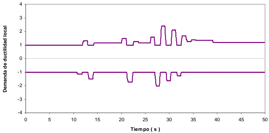
Fig 4.87.- Historias de demandas de ductilidad en el extremo izquierdo de la viga 1, edificio 17 niveles, caso A (Cuerpo Principal) con resistencias nominales
