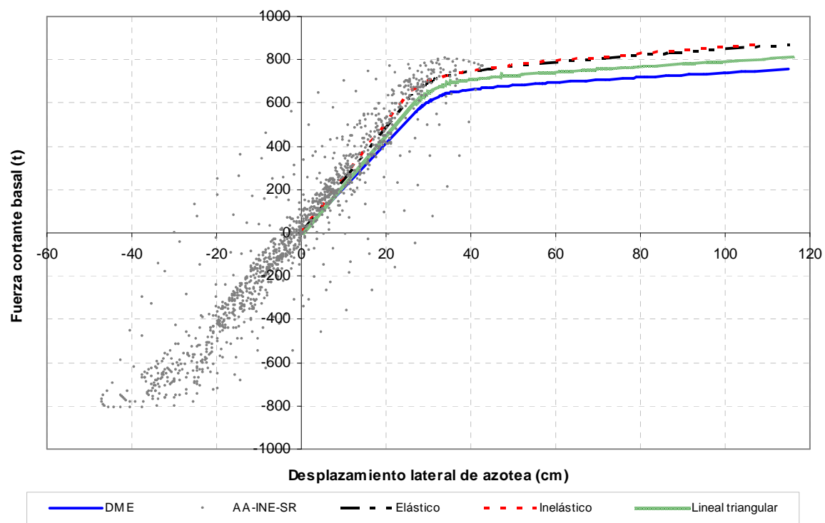
Fig A.8.- Relaciones fuerza cortante basal – desplazamiento lateral de azotea, análisis paso a paso y Push-over con diferentes distribuciones de cargas laterales, sobre-resistencias, edificio 17 niveles, caso B (Apéndice A)
