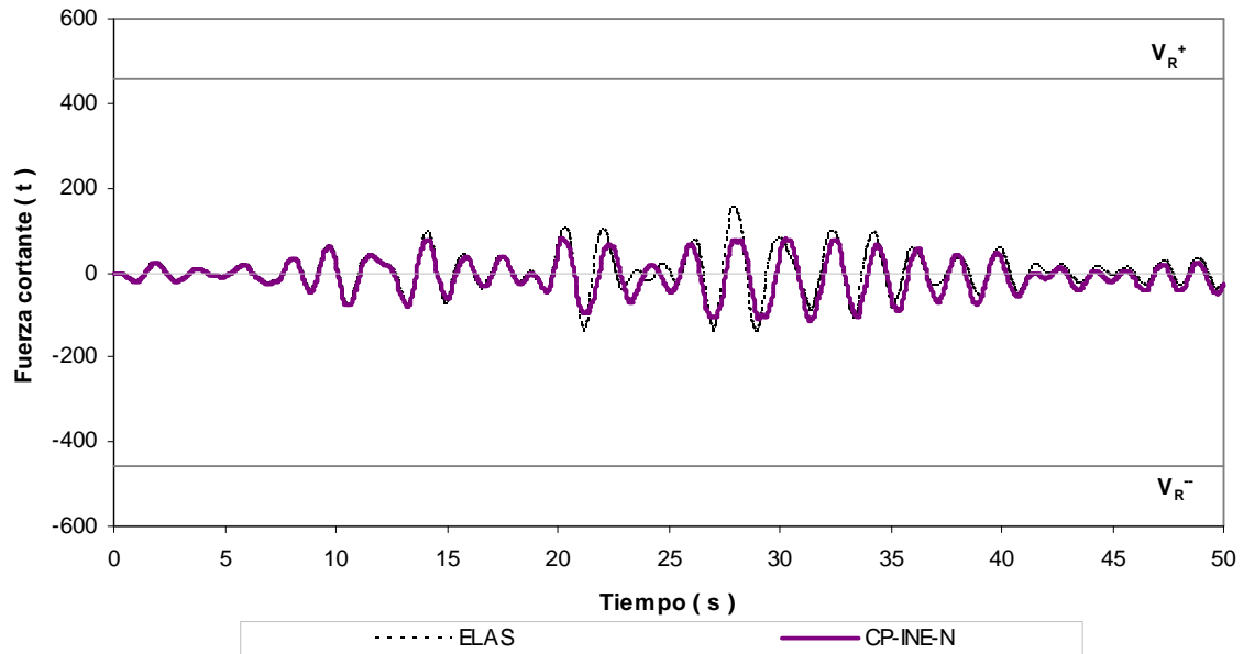
Fig 4.27.- Historias de fuerzas cortantes en el extremo inferior de la columna 1, edificio 9 niveles, caso A (Cuerpo Principal) con resistencias nominales
