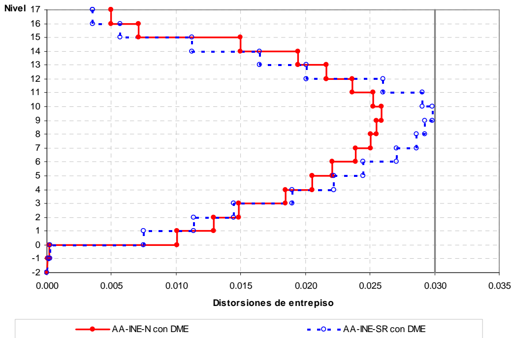
Fig 4.122.- Relaciones desplazamiento relativo entre altura de entrepiso, edificio 17 niveles, caso A con resistencias nominales y sobre-resistencias, distribución de fuerzas laterales del análisis dinámico modal espectral
