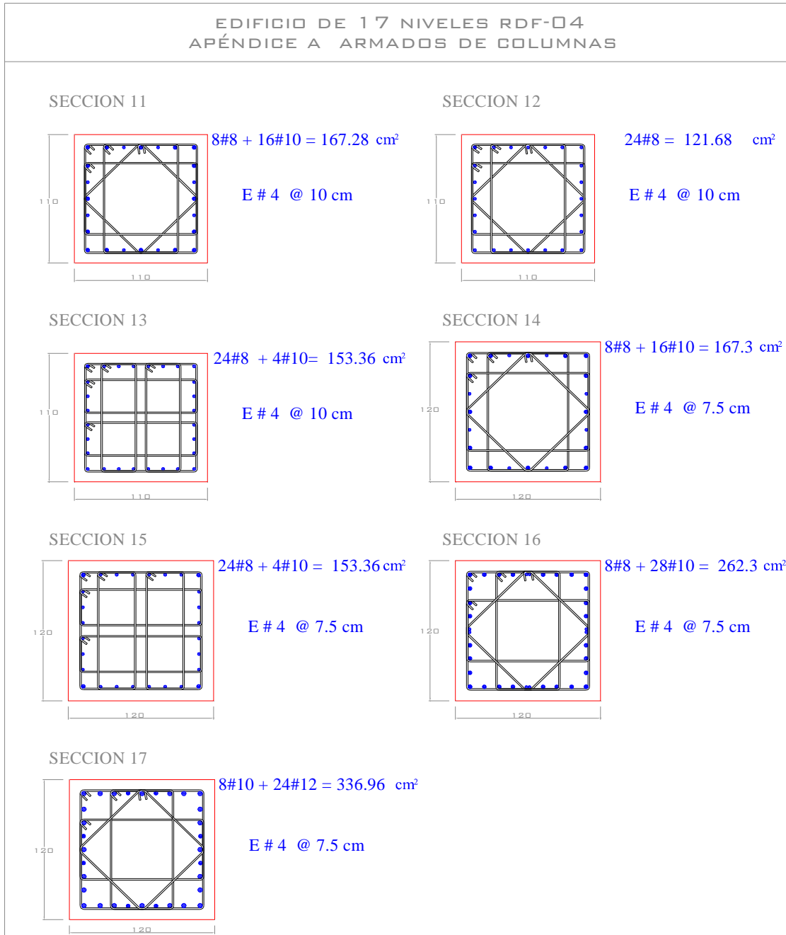
Fig 3.34b.- Armados de acero longitudinal y transversal propuestos en columnas, edificio 17 niveles, Apéndice A (caso B) de las NTC-Sismo, RDF-04
