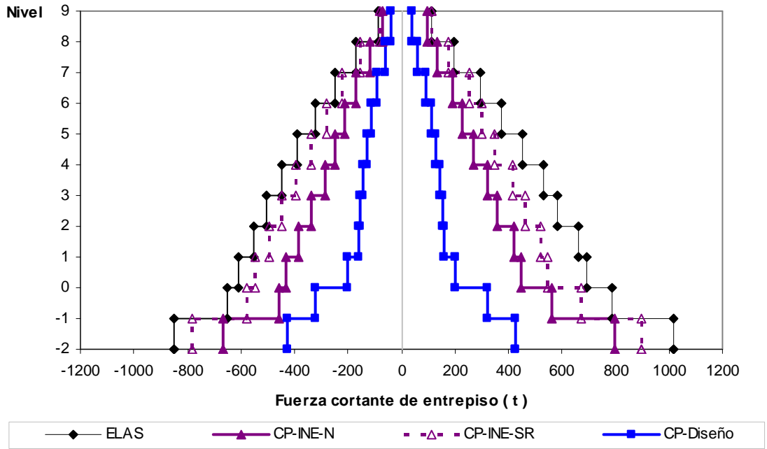
Fig 4.11.- Distribución en elevación de las fuerzas cortantes de entrepiso, edificio 9 niveles, caso A (Cuerpo Principal)
