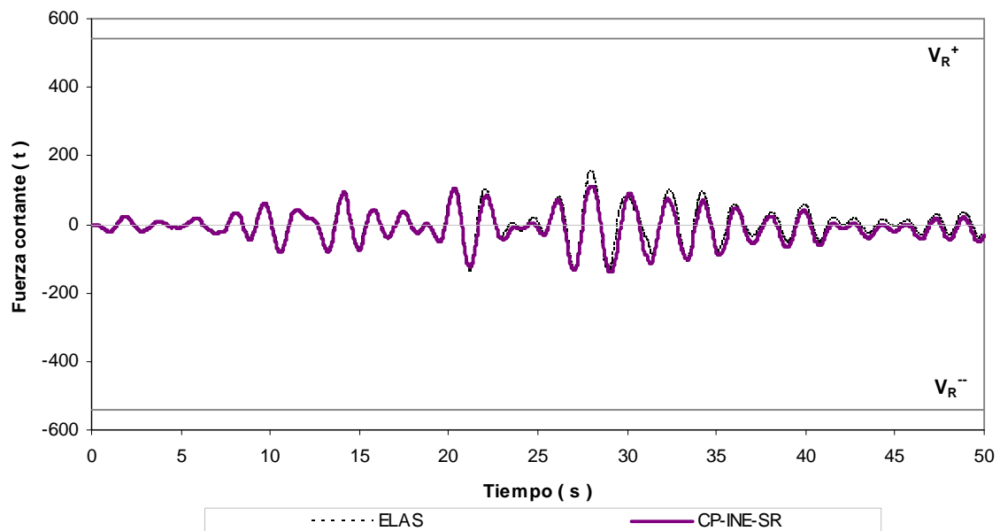
Fig 4.28.- Historias de fuerzas cortantes en el extremo inferior de la columna 1, edificio 9 niveles, caso A (Cuerpo Principal) con sobre-resistencias
