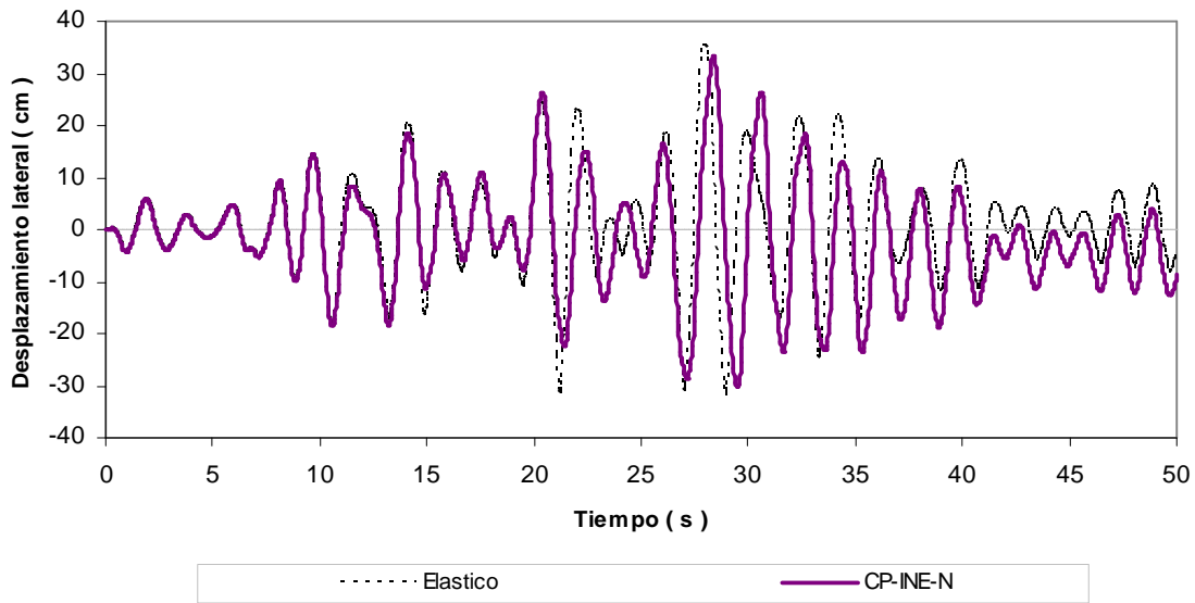
Fig 4.5.- Historia de desplazamientos de azotea, edificio 9 niveles, caso A (Cuerpo Principal) con resistencias nominales
