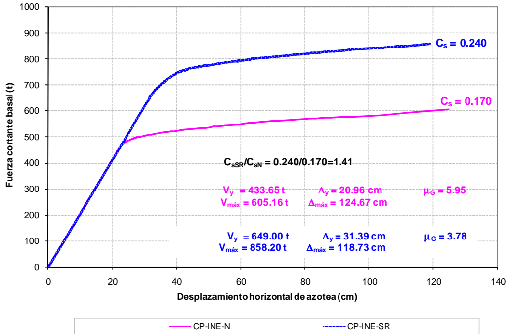
Fig 4.117.- Curvas de fuerza cortante basal-desplazamiento lateral de azotea, edificio 17 niveles, caso A (Cuerpo Principal) con resistencias nominales y sobre-resistencias, distribución de fuerzas laterales del análisis dinámico modal espectral
