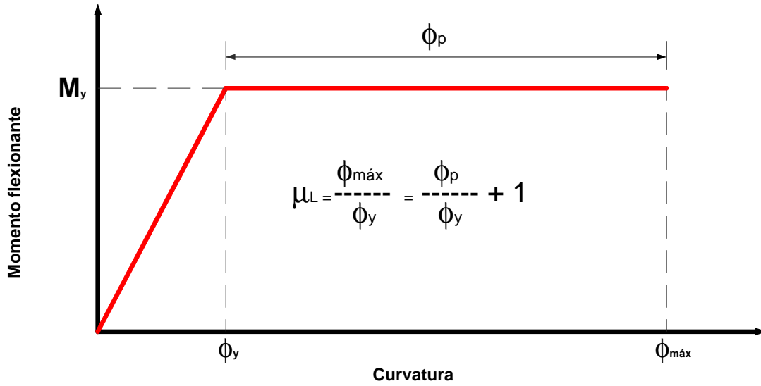
Fig 2.7.- Gráfica momento-curvatura (elasto-plástica perfecta)
