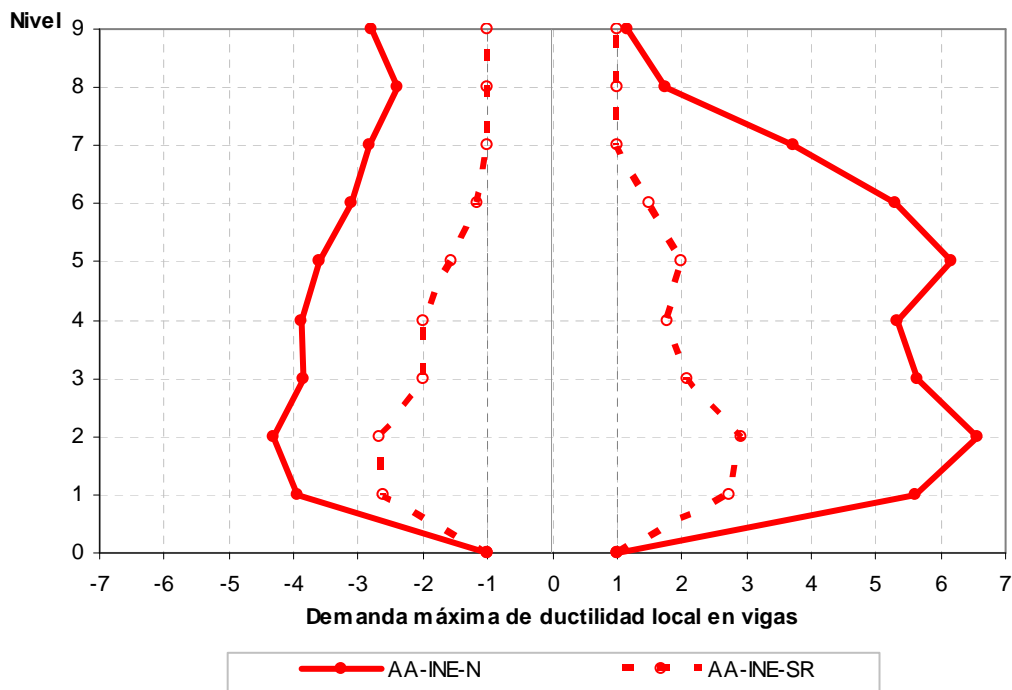
Fig 4.50.- Demandas máximas de ductilidad local en vigas, edificio 9 niveles, caso B (Apéndice A) con resistencias nominales y con sobre-resistencias
