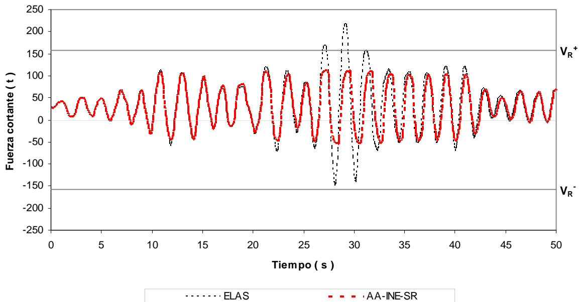
Fig 4.86.- Historias de fuerzas cortantes en el extremo izquierdo de la viga 1, edificio 17 niveles, caso B (Apéndice A) con sobre-resistencias
