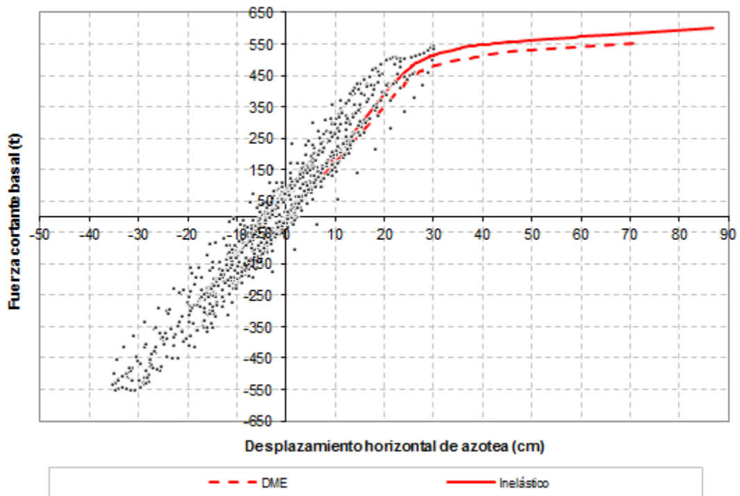
Fig 5.37.- Comparación de relaciones fuerza cortante basal-desplazamiento horizontal de azotea, análisis estático no-lineal (Push-over) y análisis paso a paso inelástico con sobre-resistencias, edificio de 9 niveles, caso B (Apéndice A)
