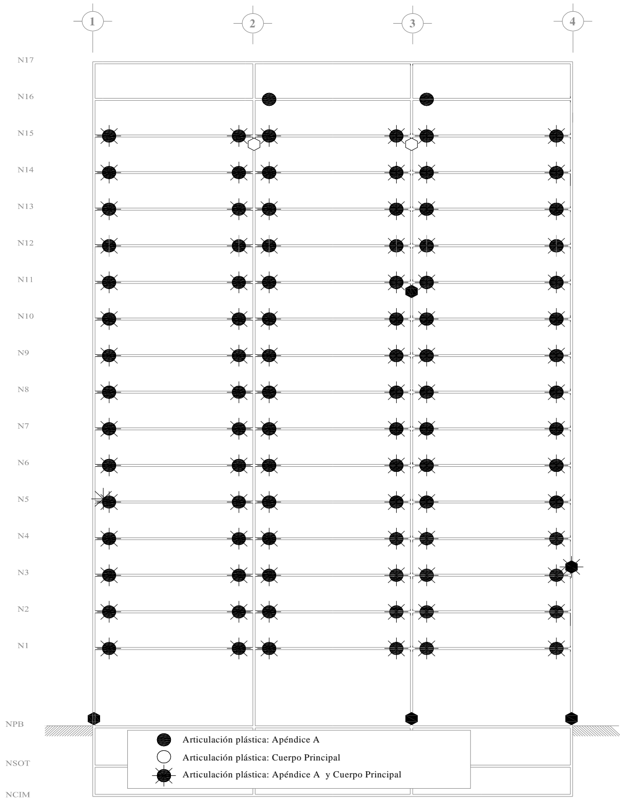
Fig 5.27.- Comparación de distribuciones de articulaciones plásticas, análisis paso a paso inelástico (sobre-resistencias), edificio de 17 niveles, casos A (Cuerpo Principal) y B (Apéndice A)
