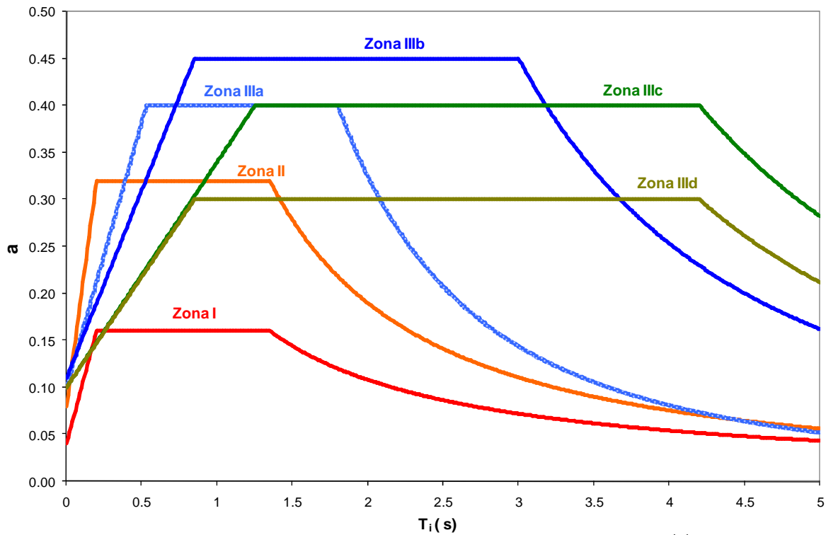
Fig 2.11.- Espectros elásticos de diseño del Cuerpo Principal de las NTC-Sismo del RDF-04
