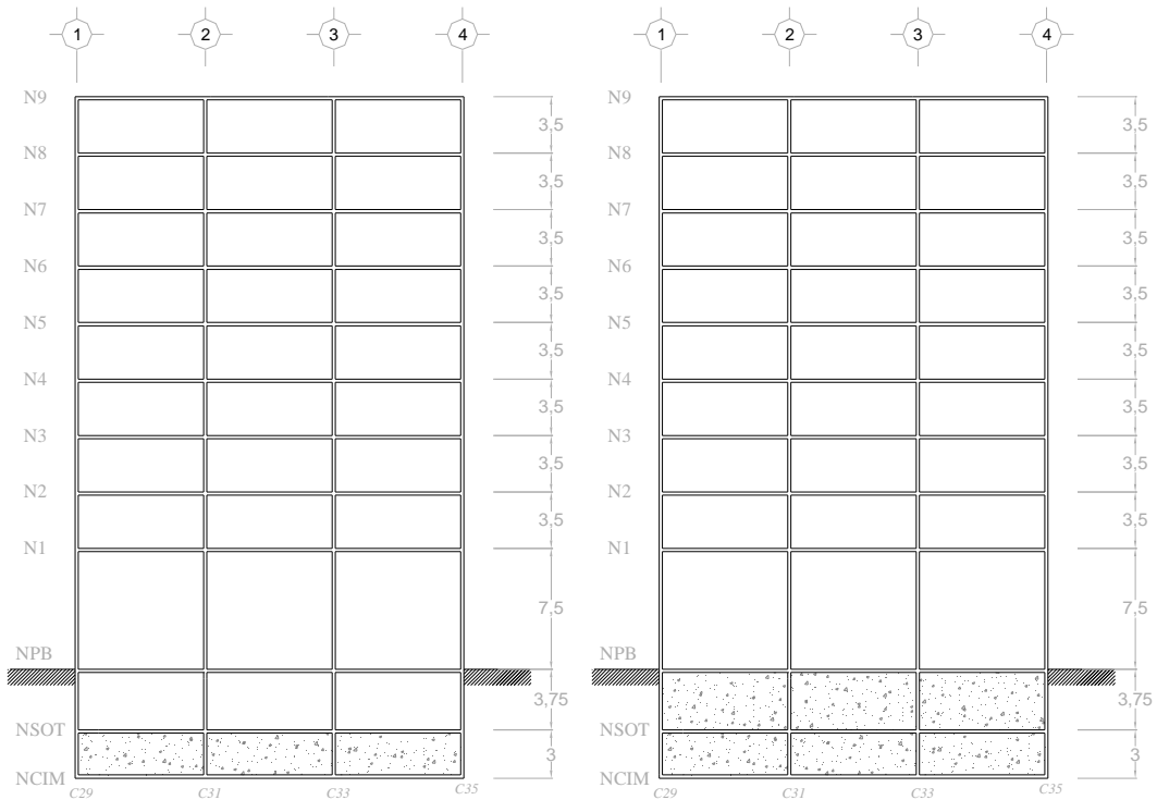
Fig 3.2c.- Cortes transversales interior y exterior en dirección corta "X", edificio de 9 niveles
