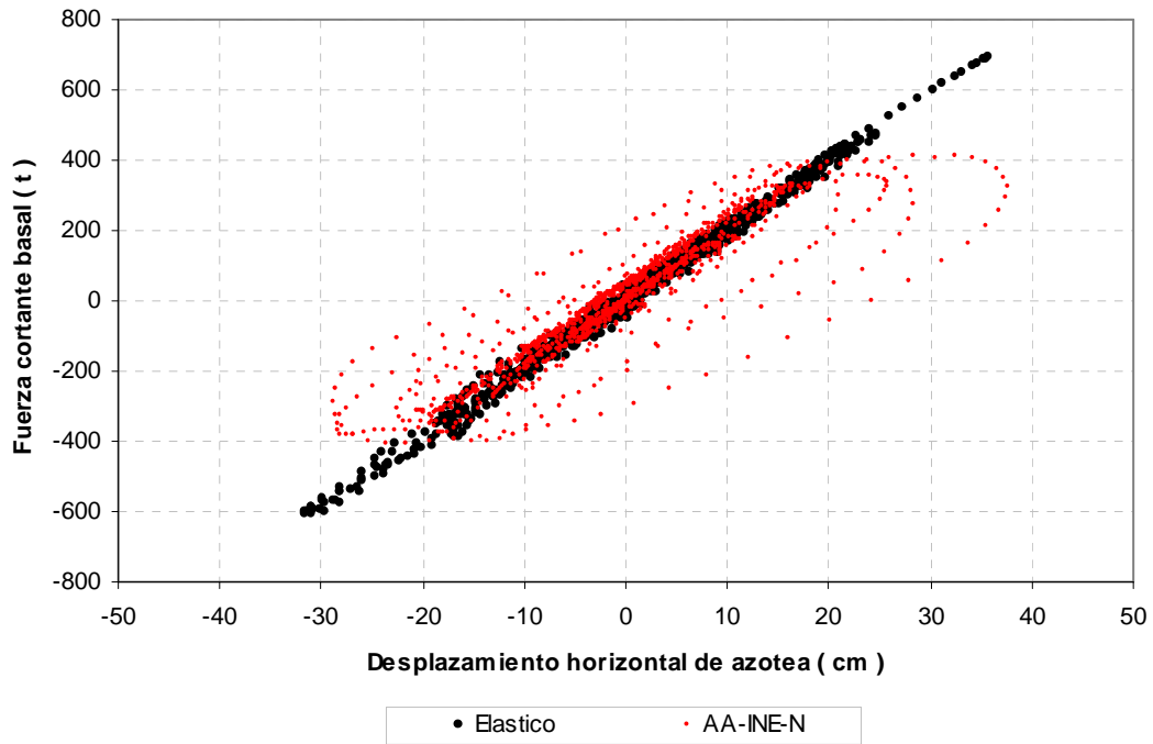
Fig 5.18.- Comparación de relaciones fuerza cortante basal-desplazamiento horizontal de azotea, análisis paso a paso elástico e inelástico (resistencias nominales), edificio de 9 niveles, caso B (Apéndice A)
