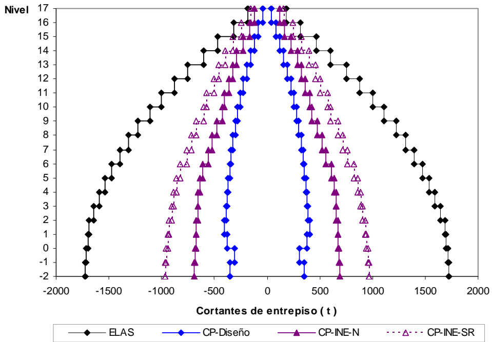
Fig 4.59.- Distribución en elevación de las fuerzas cortantes de entrepiso, edificio 17 niveles, caso A (Cuerpo Principal)
