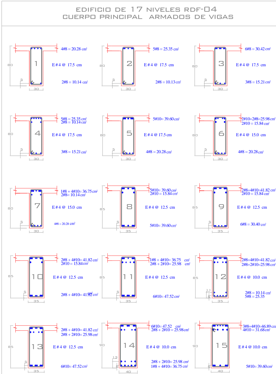
Fig 3.29a.- Armados longitudinal y transversal propuestos de vigas, edificio 17 niveles, Cuerpo Principal (caso A) de las NTC-Sismo, RDF-04
