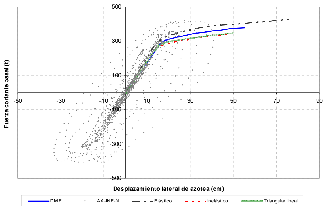
Fig A.3.- Relaciones fuerza cortante basal – desplazamiento lateral de azotea, análisis paso a paso y Push-over con diferentes distribuciones de cargas laterales, resistencias nominales, edificio 9 niveles, caso B (Apéndice A)
