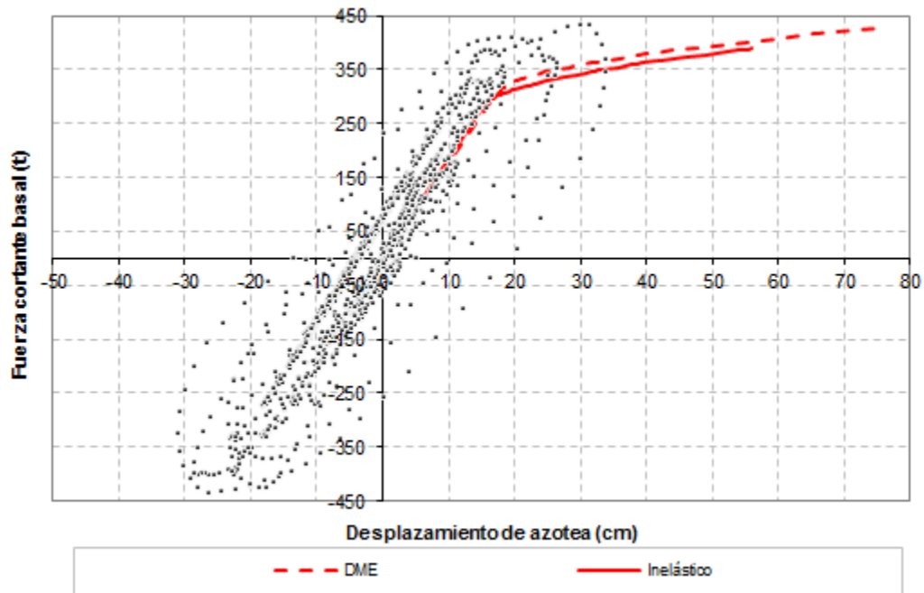
Fig 5.34.- Comparación de relaciones fuerza cortante basal-desplazamiento horizontal de azotea, análisis estático no-lineal (Push-over) y análisis paso a paso inelástico con resistencias nominales, edificio de 9 niveles, caso A (Cuerpo Principal)
