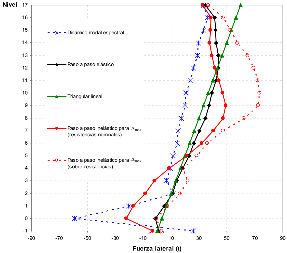
Fig 4.116.- Distribución de cargas laterales para el análisis estático no-lineal (Push-over), edificio 17 niveles, caso B (Apéndice A)
