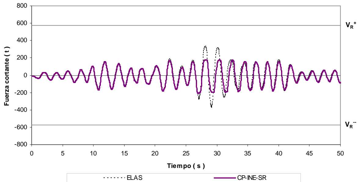
Fig 4.76.- Historias de fuerzas cortantes en el extremo inferior de la columna 1, edificio 17 niveles, caso A (Cuerpo Principal) con sobre-resistencias
