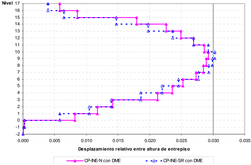
Fig 4.121.- Relaciones desplazamiento relativo entre altura de entrepiso, edificio 17 niveles, caso A con resistencias nominales y sobre-resistencias, distribución de fuerzas laterales del análisis dinámico modal espectral
