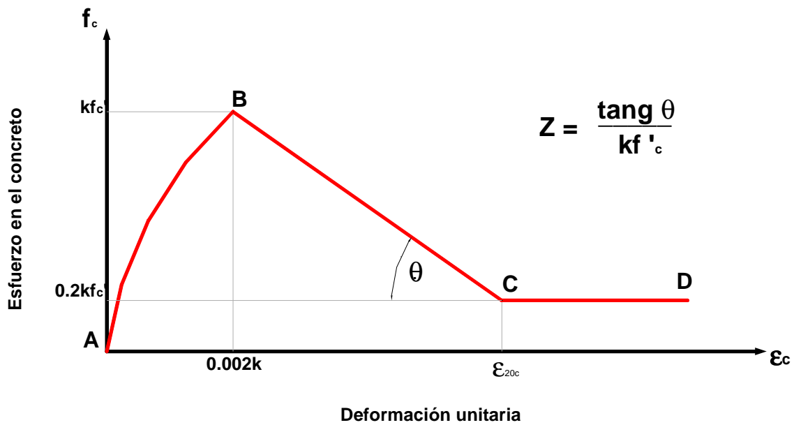
Fig 2.19.- Curva esfuerzo-deformación para concreto confinado, según modelo Kent-Park modificado
