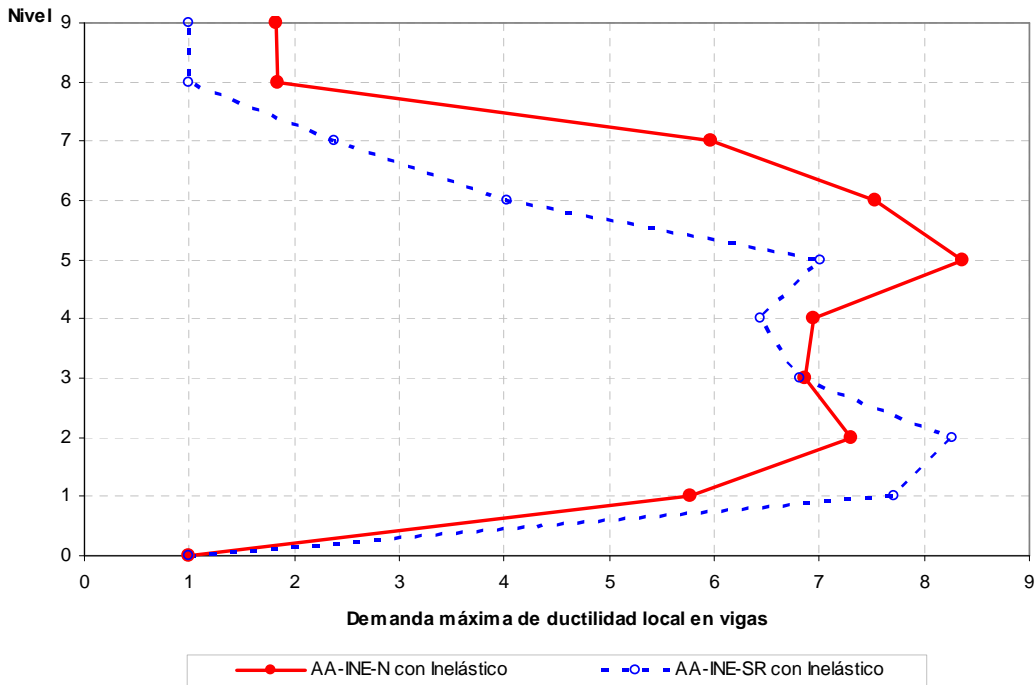
Fig 4.112.- Demandas máximas de ductilidad local en vigas, edificio 9 niveles, caso B (Apéndice A) con resistencias nominales y sobre-resistencias, distribución de fuerzas laterales del análisis paso a paso inelástico para \Delta_{máx}
