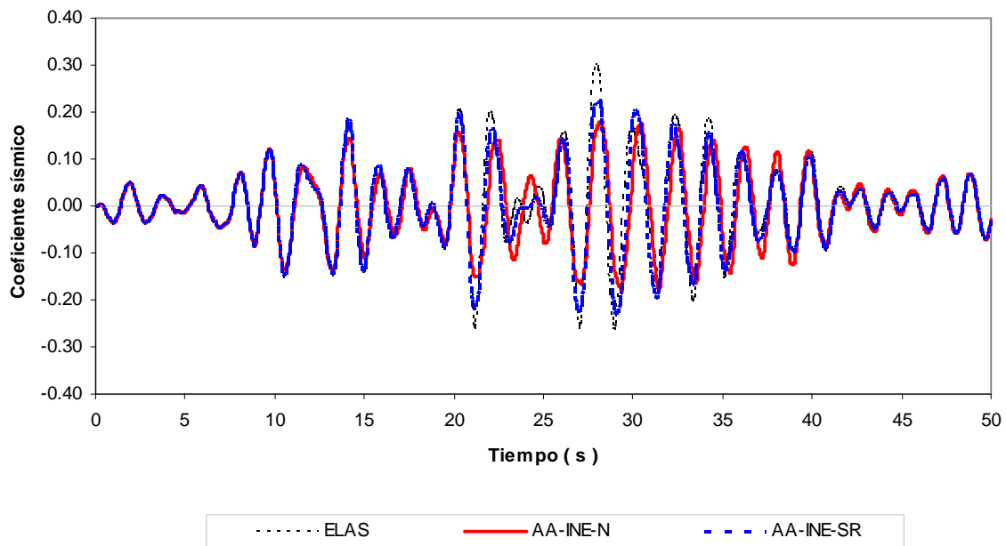
Fig 5.13.- Comparación de coeficientes sísmicos, análisis paso a paso elástico e inelástico (resistencias nominales y sobre-resistencias), edificio de 9 niveles, caso B (Apéndice A)
