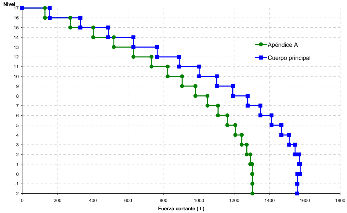
Fig 3.25.- Fuerzas cortantes de entrepiso, sismo en dirección “X” y “Y”, edificio 17 niveles, Apéndice A y Cuerpo Principal de las NTC-Sismo, RDF-04
