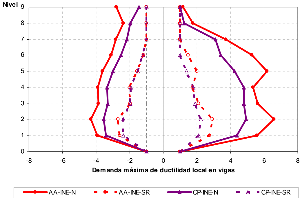
Fig 5.28.- Comparación de demandas máximas de ductilidad local en vigas, análisis paso a paso inelástico (resistencias nominales y sobre-resistencias), edificio de 9 niveles, casos A (Cuerpo Principal) y B (Apéndice A)
