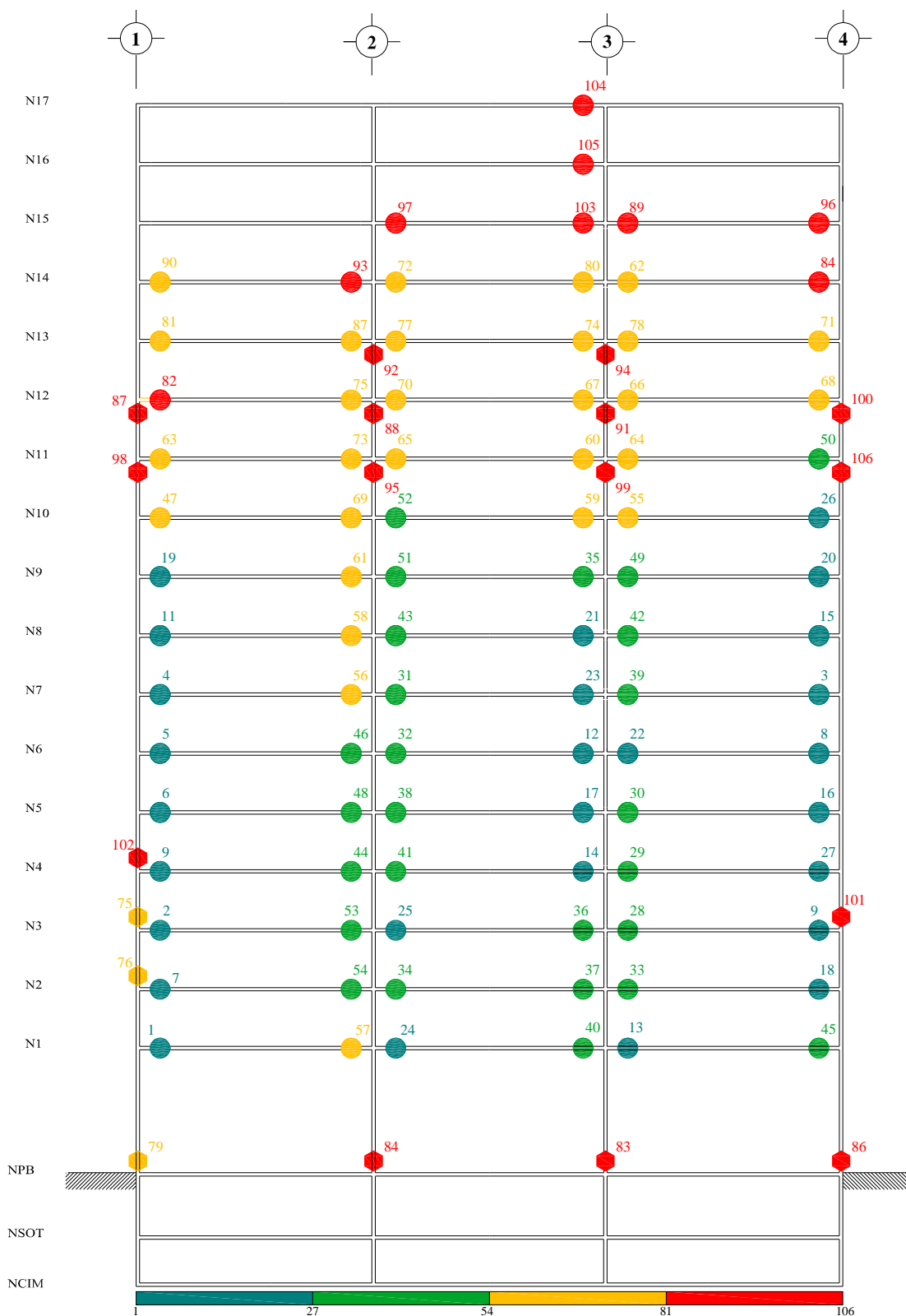
Fig A.21.- Secuencia de formación de articulaciones plásticas, análisis estático no-lineal (Push-over) con distribución de cargas laterales de análisis paso a paso elástico, resistencias nominales, edificio 17 niveles, caso A (Cuerpo Principal)
