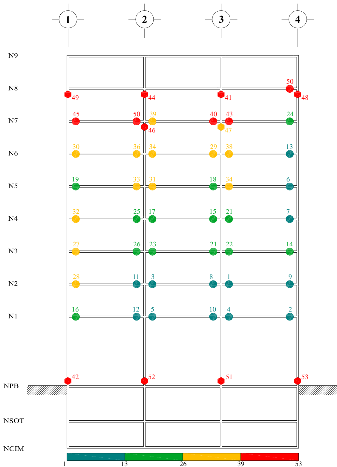
Fig A.20.- Secuencia de formación de articulaciones plásticas, análisis estático no-lineal (Push-over) con distribución de cargas laterales lineal triangular, sobre-resistencias, edificio 9 niveles, caso B (Apéndice A)
