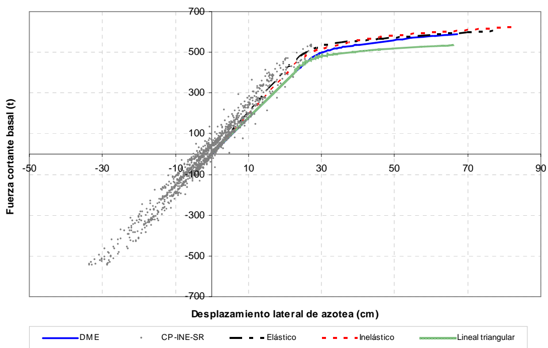
Fig A.2.- Relaciones fuerza cortante basal – desplazamiento lateral de azotea, análisis paso a paso y Push-over con diferentes distribuciones de cargas laterales, sobre-resistencias, edificio 9 niveles, caso A (Cuerpo Principal)
