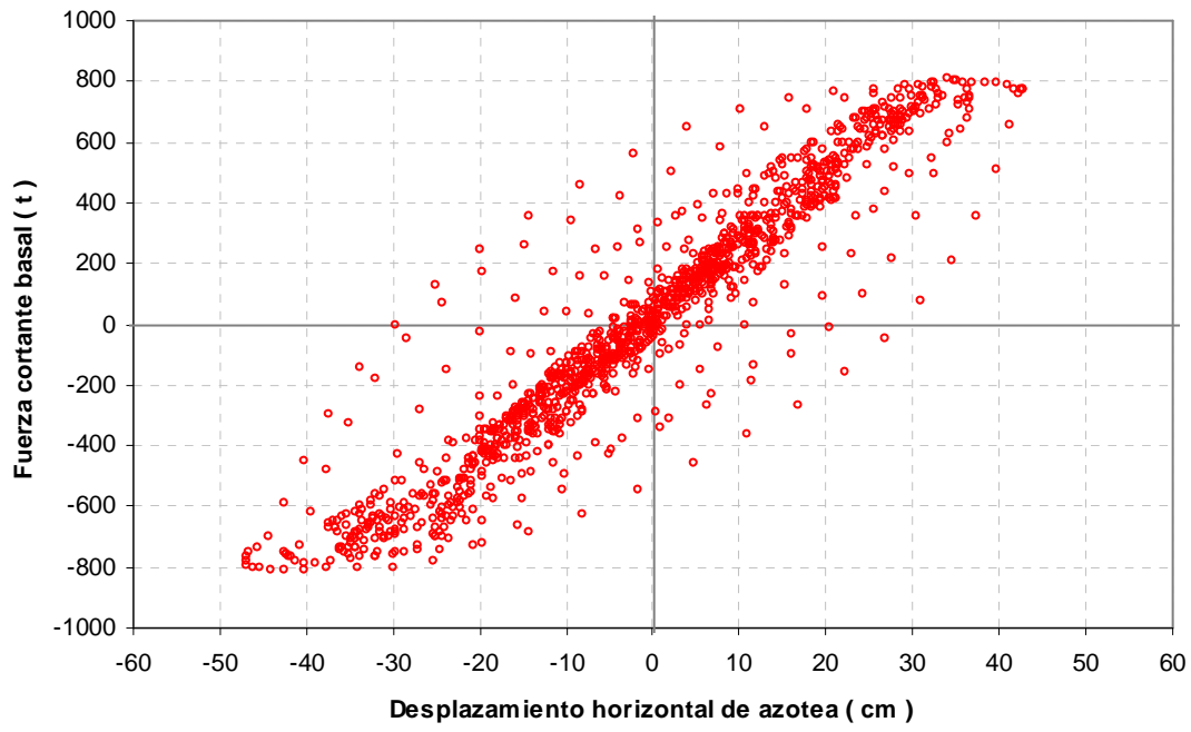
Fig 4.69.- Relaciones fuerza cortante basal – desplazamiento lateral de azotea, edificio 17 niveles, caso B (Apéndice A), comportamiento inelástico con sobre-resistencias
