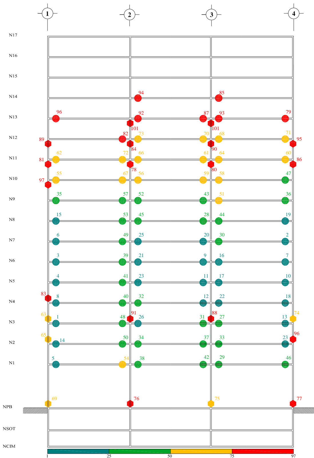
Fig A.22.- Secuencia de formación de articulaciones plásticas, análisis estático no-lineal (Push-over) con distribución de cargas laterales de análisis paso a paso inelástico, resistencias nominales, edificio 17 niveles, caso A (Cuerpo Principal)
