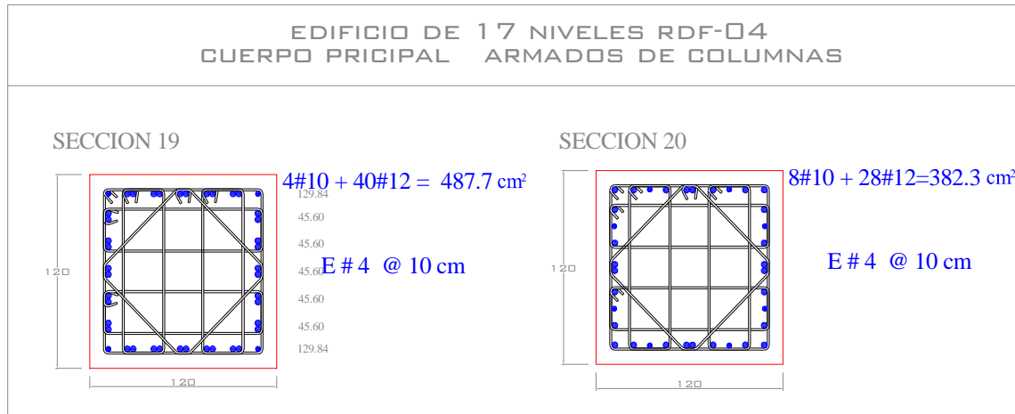
Fig 3.33c.- Armados de acero longitudinal y transversal propuestos en columnas, edificio 17 niveles, Cuerpo Principal (caso A) de las NTC-Sismo, RDF-04
