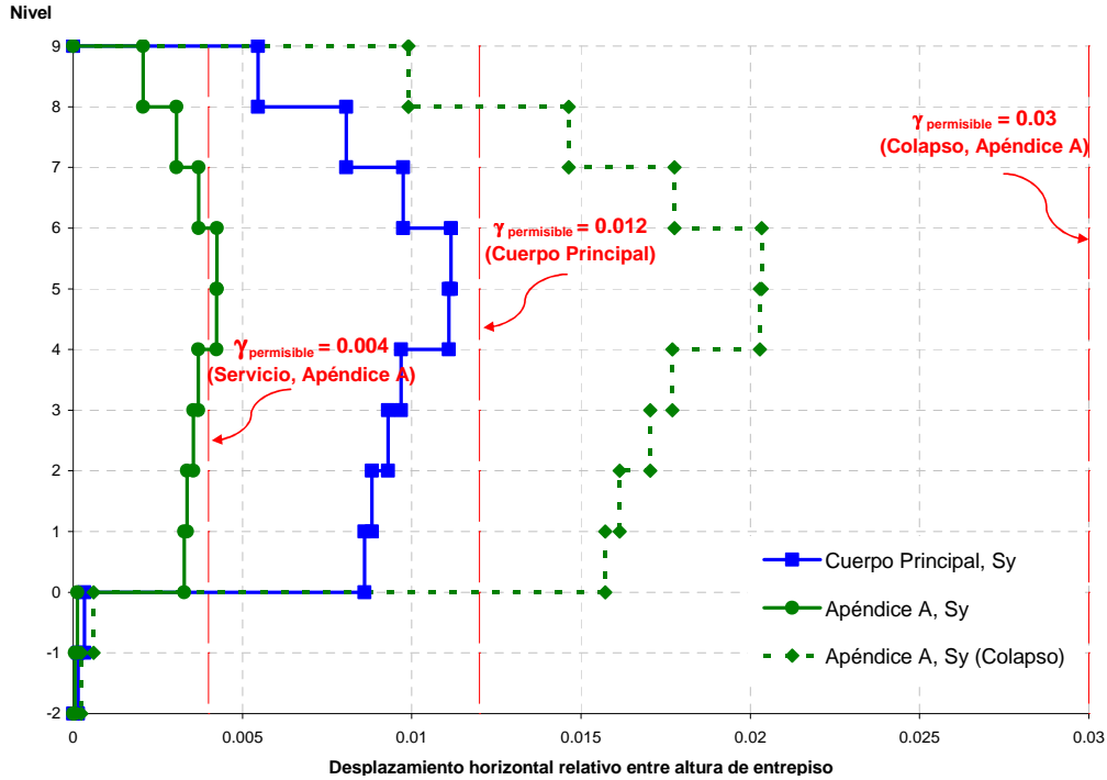
Fig 3.8.- Relaciones máximas de desplazamiento lateral relativo entre altura de entrepiso, sismo en dirección "Y", edificio 9 niveles, Apéndice A y Cuerpo Principal de las NTC-Sismo, RDF-04
