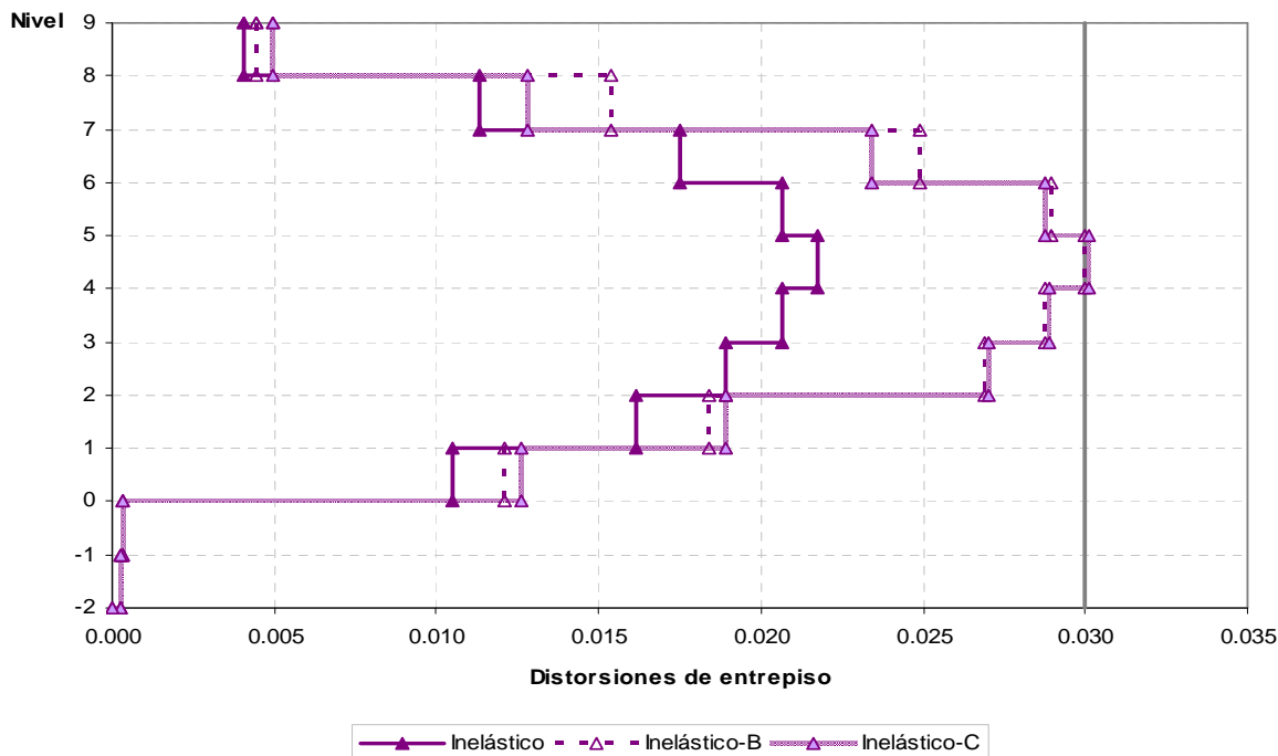
Fig A.34.- Relaciones máximas de desplazamiento horizontal relativo entre altura de entrepiso, análisis estático no-lineal (Push-over) con resistencias nominales, edificio de 9 niveles, caso A (Cuerpo Principal), sin y con cambio en el acero de refuerzo longitudinal de columnas
