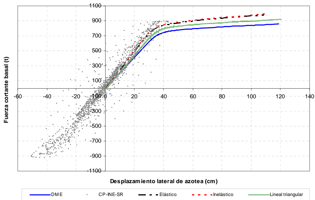
Fig A.6.- Relaciones fuerza cortante basal – desplazamiento lateral de azotea, análisis paso a paso y Push-over con diferentes distribuciones de cargas laterales, sobre-resistencias, edificio 17 niveles, caso A (Cuerpo Principal)
