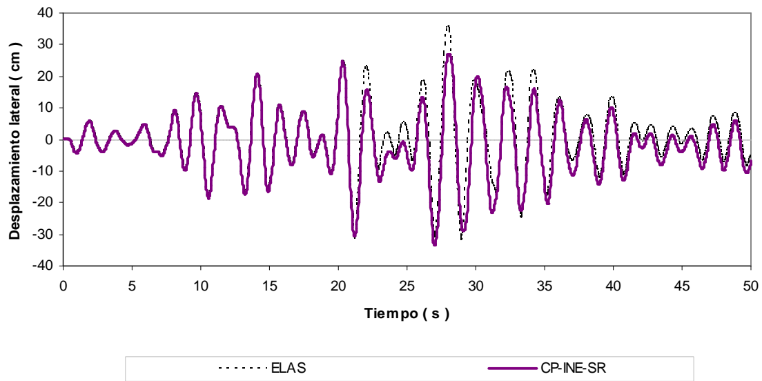
Fig 4.6.- Historias de desplazamientos de azotea, edificio 9 niveles, caso A (Cuerpo Principal) con sobre-resistencia
