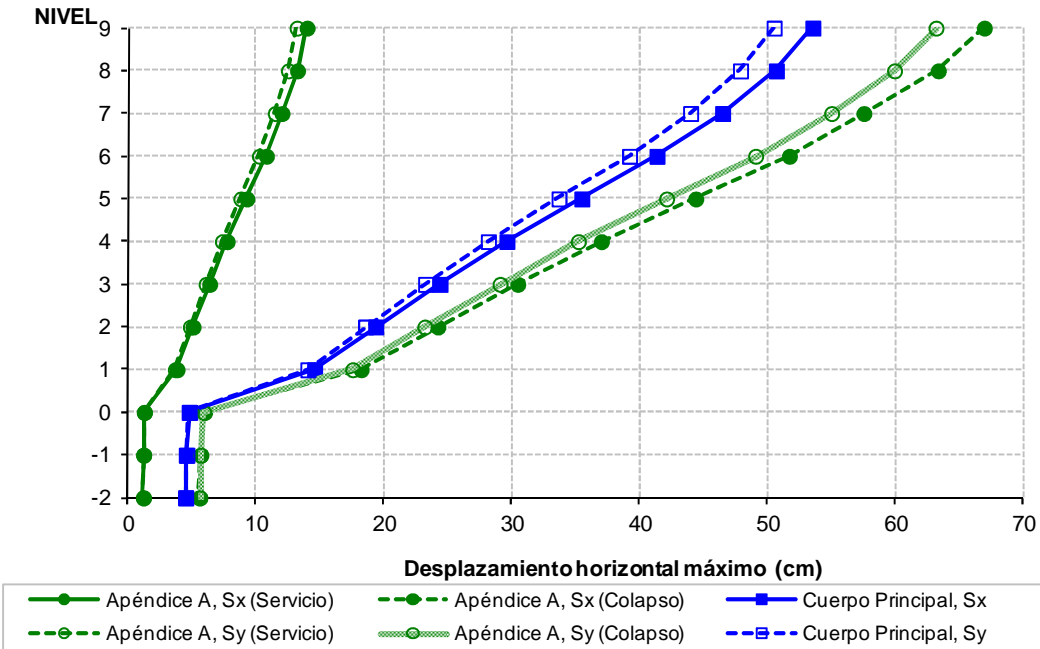
Fig 5.2.- Comparación de desplazamientos horizontales máximos de servicio y de colapso, análisis dinámico modal espectral, sismo en ambas direcciones, edificio de 9 niveles, casos A (Cuerpo Principal) y B (Apéndice A)
