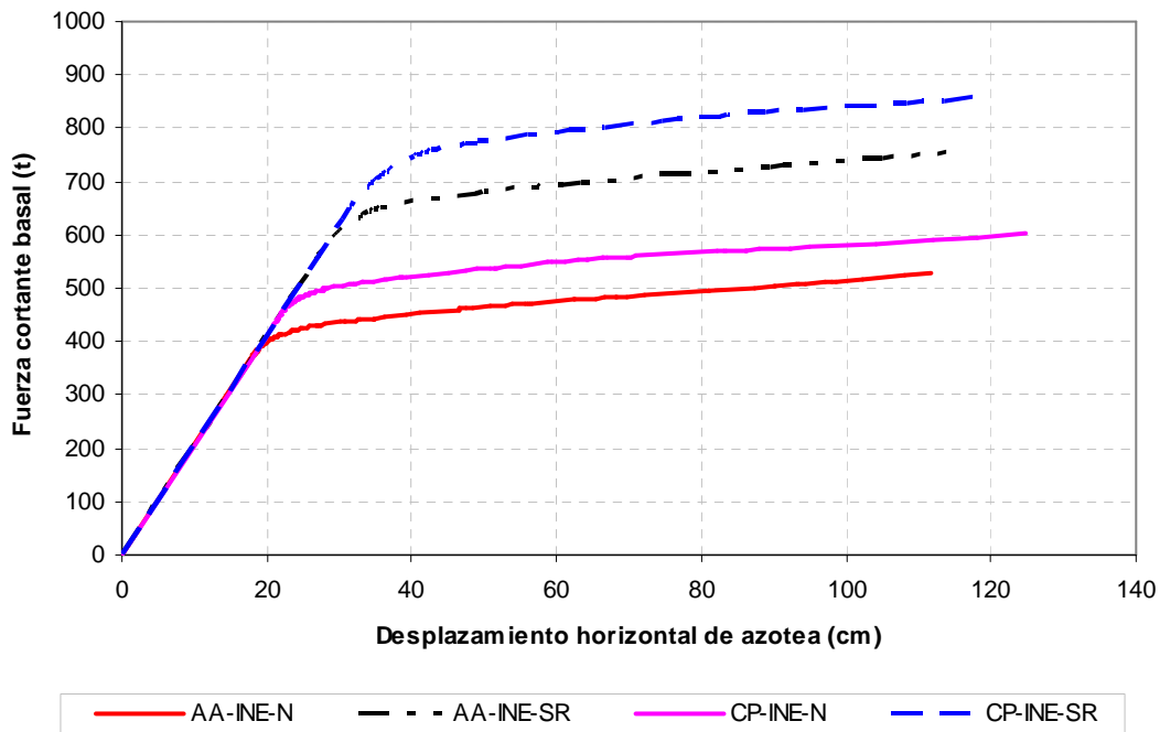
Fig 5.33.- Comparación de relaciones fuerza cortante basal-desplazamiento horizontal de azotea, análisis estático no-lineal (Push-over) con resistencias nominales y sobre-resistencias, edificio de 17 niveles, casos A (Cuerpo Principal) y B (Apéndice A)
