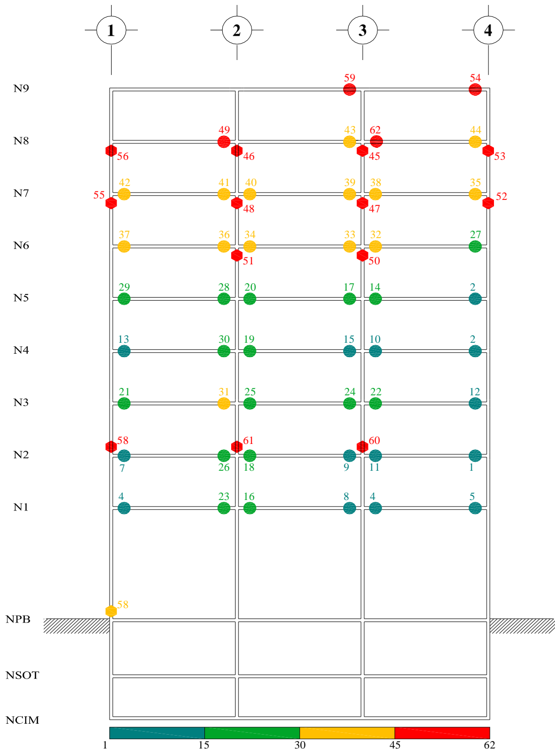
Fig 4.107.- Mecanismo de falla y secuencia de formación de articulaciones plásticas, edificio 9 niveles, caso A (Cuerpo Principal) con resistencias nominales, distribución de fuerzas laterales del análisis paso a paso inelástico para \Delta_{máx}
