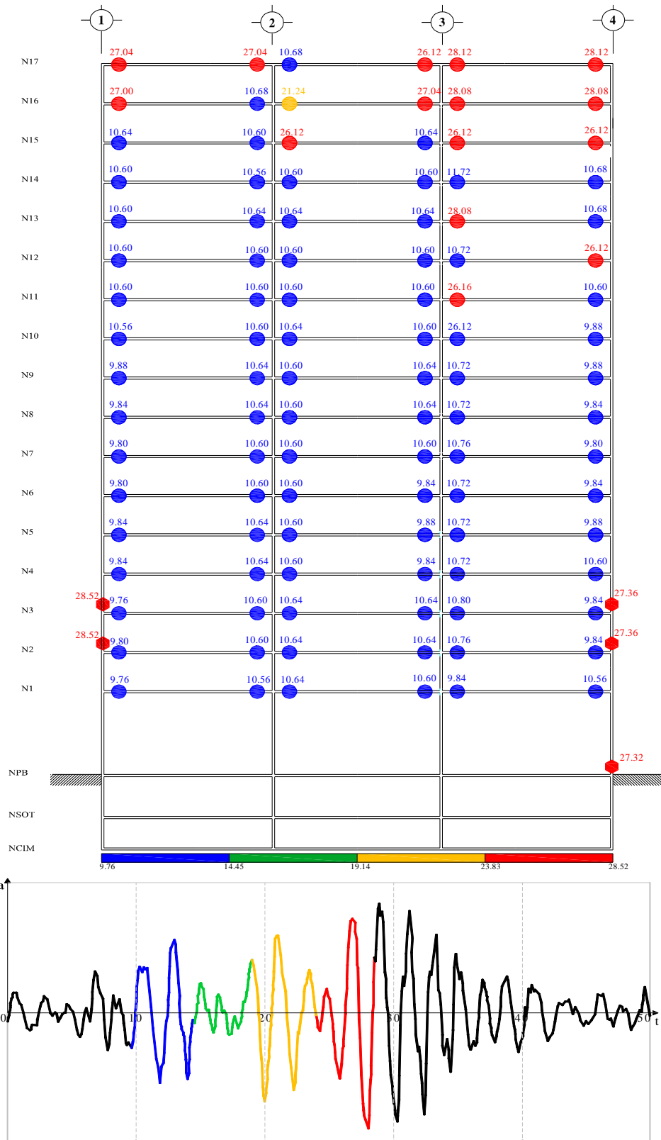
Fig 4.91.- Secuencia de formación y distribución global de articulaciones plásticas, edificio 17 niveles, caso A con resistencias nominales
