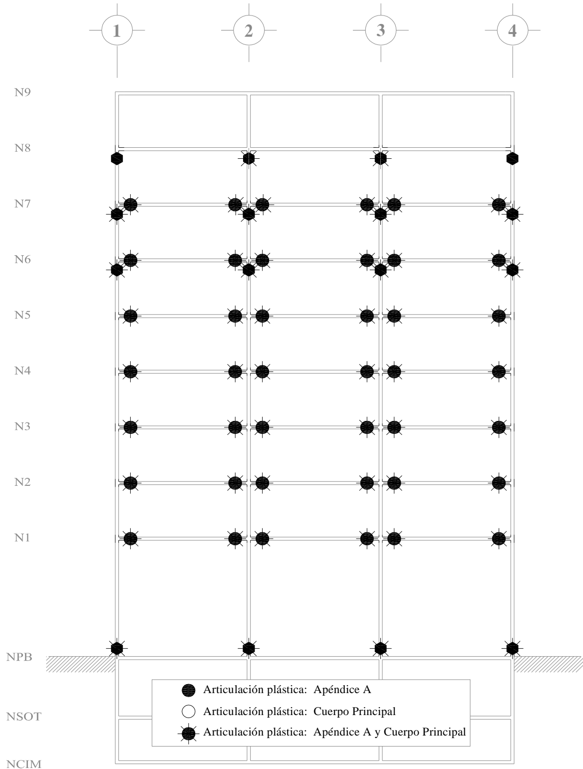
Fig 5.43.- Comparación de distribuciones de articulaciones plásticas, análisis estático no lineal (Push-over) con sobre-resistencia, edificio de 9 niveles, casos A (Cuerpo Principal) y B (Apéndice A)
