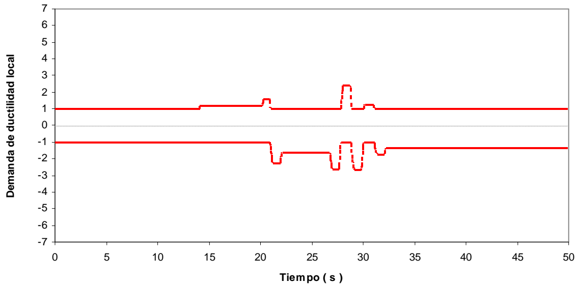
Fig 4.42.- Historias de demandas de ductilidad el extremo izquierdo de la viga 1, edificio 9 niveles, caso B (Apéndice A) con sobre-resistencias
