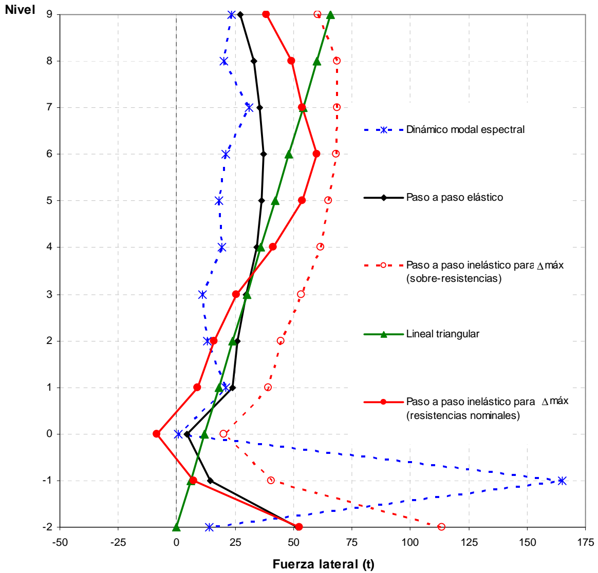
Fig 4.99.- Distribuciones de cargas laterales para el análisis estático no-lineal (Push-over), edificio 9 niveles, caso A (Cuerpo Principal)
