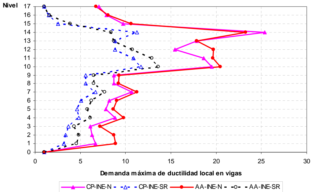
Fig 5.47.- Comparación de demandas máximas de ductilidad local en vigas, análisis estático no-lineal (Push-over), edificio de 17 niveles con resistencias nominales y sobre-resistencias, caso A (Cuerpo Principal) y B (Apéndice A)
