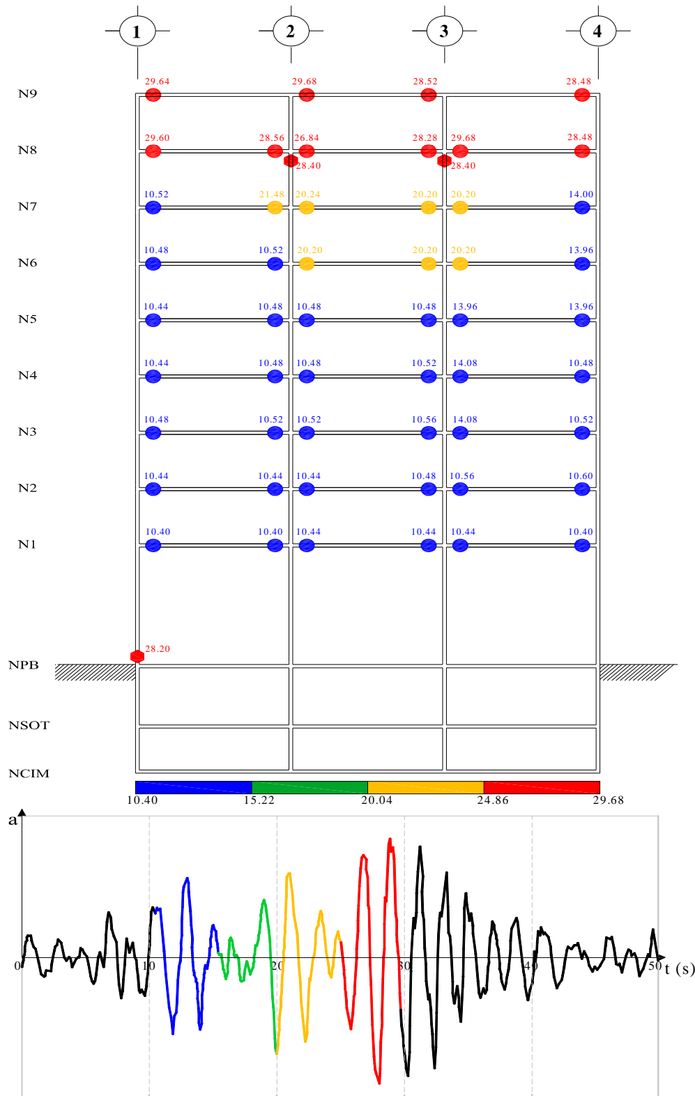
Fig 4.43.- Secuencia de formación y distribución global de articulaciones plásticas, edificio 9 niveles, caso A con resistencias nominales
