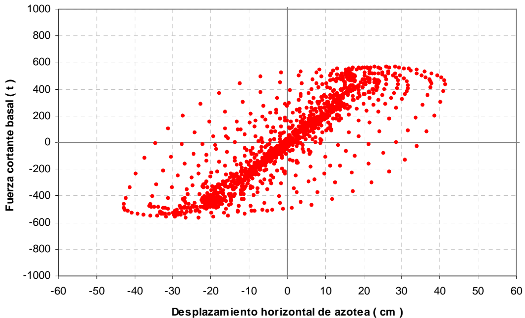
Fig 4.68.- Relaciones fuerza cortante basal – desplazamiento lateral de azotea, edificio 17 niveles, caso B (Apéndice A), comportamiento inelástico con resistencias nominales
