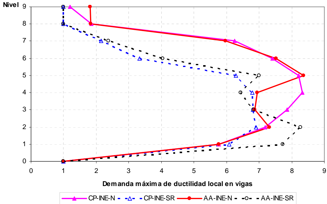
Fig 5.46.- Comparación de demandas máximas de ductilidad local en vigas, análisis estático no-lineal (Push-over), edificio de 9 niveles con resistencias nominales y sobre-resistencias, caso A (Cuerpo Principal) y B (Apéndice A)
