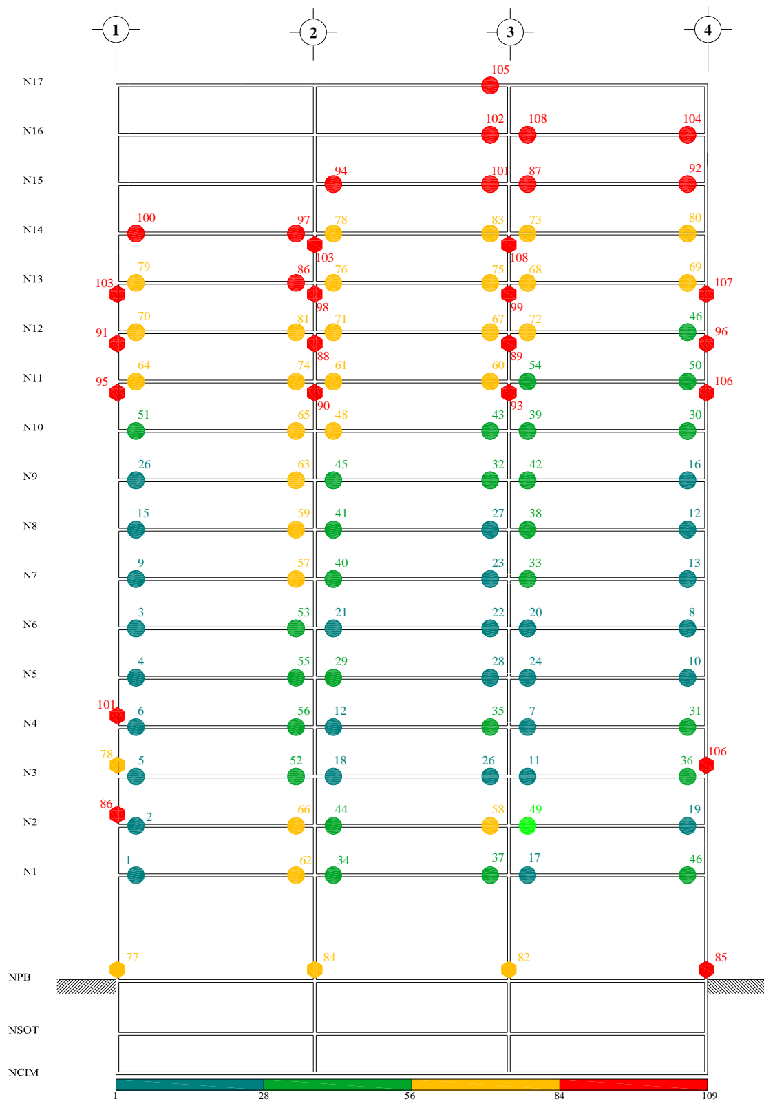
Fig A.27.- Secuencia de formación de articulaciones plásticas, análisis estático no-lineal (Push-over) con distribución de cargas laterales de análisis paso a paso elástico, resistencias nominales, edificio 17 niveles, caso B (Apéndice A)
