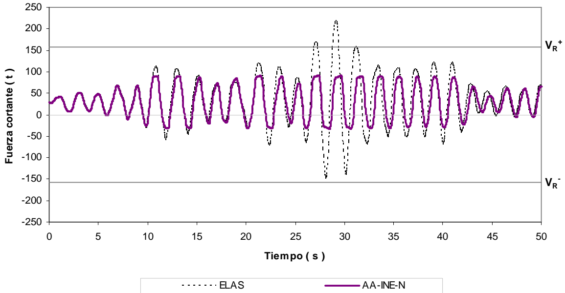
Fig 4.83.- Historias de fuerzas cortantes en el extremo izquierdo de la viga 1, edificio 17 niveles, caso A (Cuerpo Principal) con resistencias nominales
