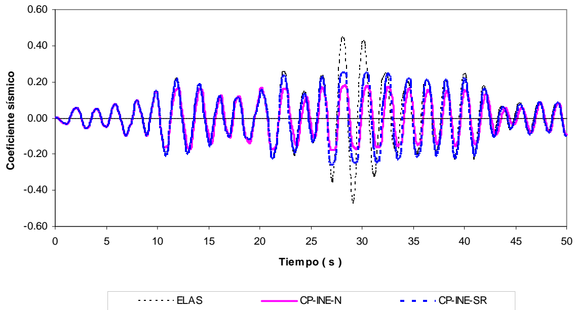
Fig 5.14.- Comparación de coeficientes sísmicos, análisis paso a paso elástico e inelástico (resistencias nominales y sobre-resistencias), edificio de 17 niveles, caso A (Cuerpo Principal)
