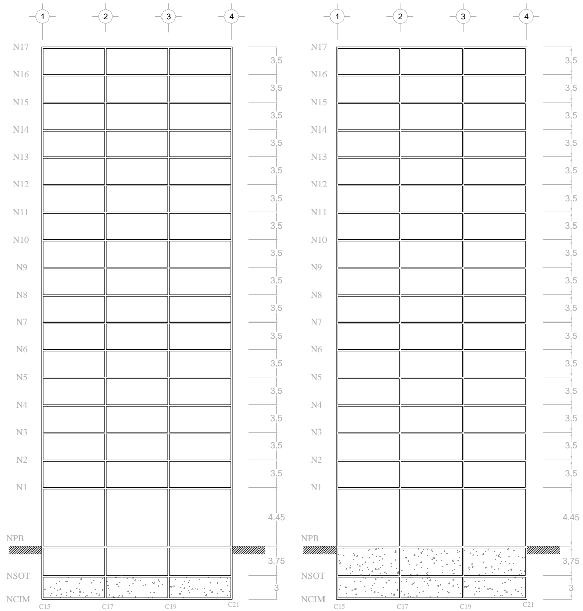
Fig 3.3c.- Cortes transversales interior y exterior, edificio de 17 niveles
