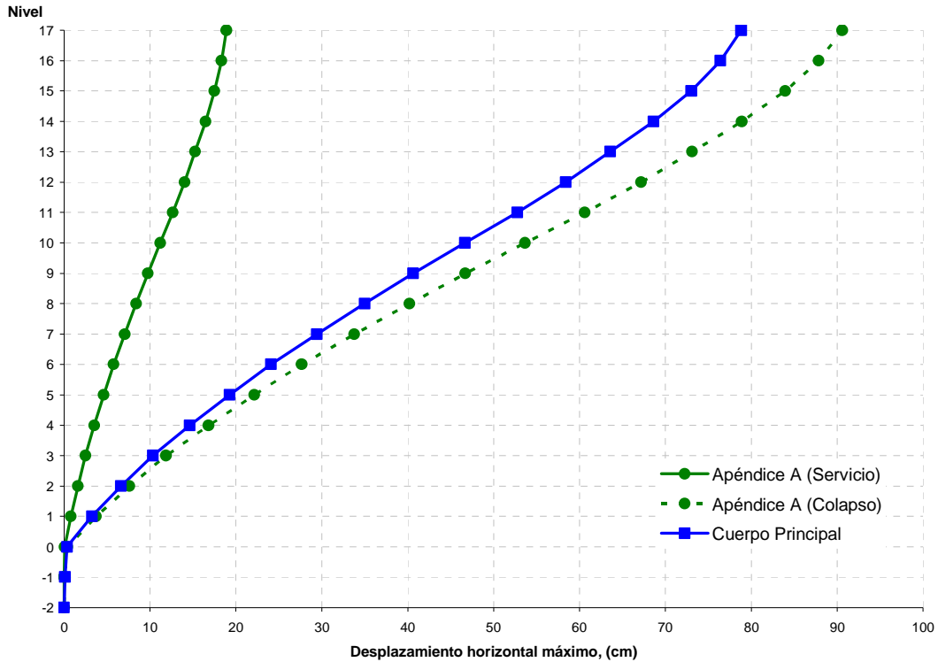
Fig 3.23.- Desplazamientos horizontales máximos, sismo en dirección “X” y “Y”, edificio 17 niveles, Apéndice A y Cuerpo Principal de las NTC-Sismo, RDF-04
