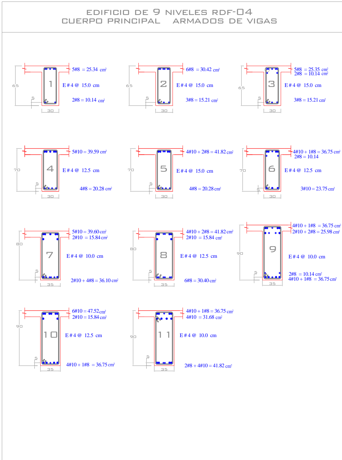
Fig 3.14.- Armados longitudinal y transversal propuestos de las vigas del eje C, edificio 9 niveles, Cuerpo Principal (caso A) de las NTC-Sismo, RDF-04
