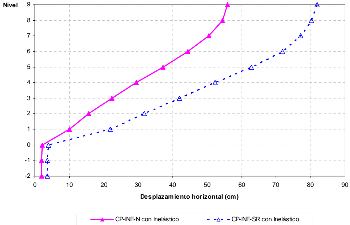
Fig 4.103.- Desplazamientos horizontales máximos, edificio 9 niveles, caso A con resistencias nominales y sobre-resistencias, distribución de cargas del análisis paso a paso inelástico para \Delta_{máx}
