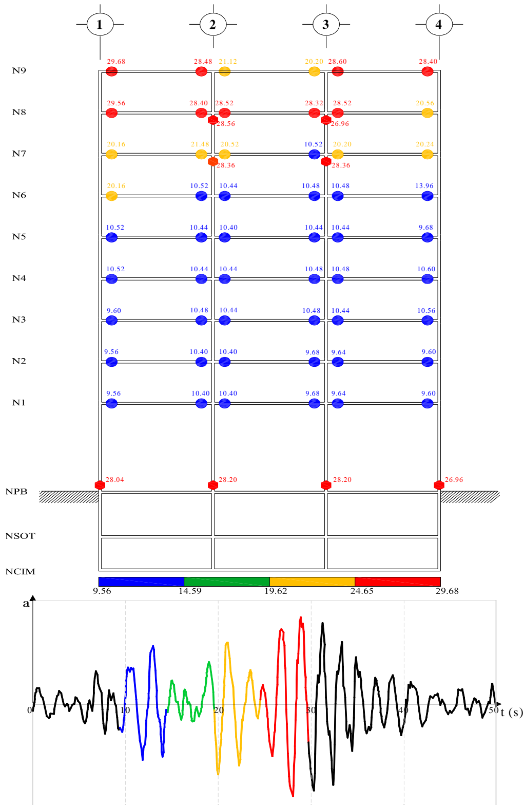
Fig 4.45.- Secuencia de formación y distribución global de articulaciones plásticas, edificio 9 niveles, caso B con resistencias nominales
