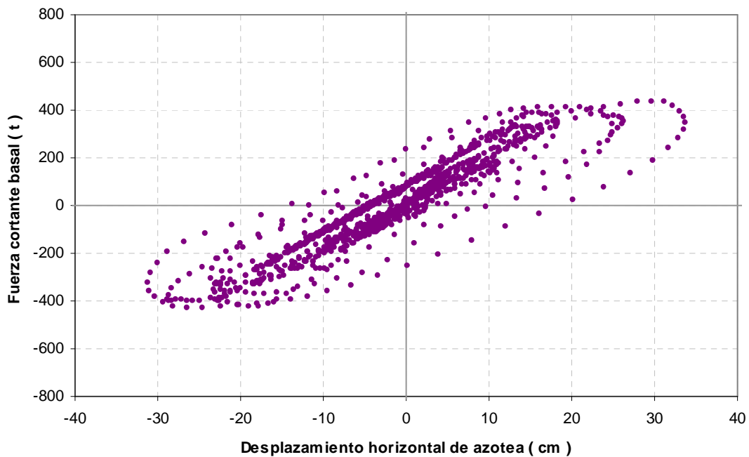
Fig 4.18.- Relaciones fuerza cortante basal – desplazamiento lateral de azotea, 9 niveles, caso A (Cuerpo Principal), comportamiento inelástico con resistencias nominales
