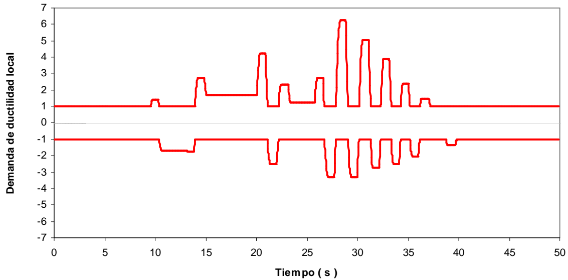
Fig 4.41.- Historias de demandas de ductilidad el extremo izquierdo de la viga 1, edificio 9 niveles, caso B (Apéndice A) con resistencias nominales
