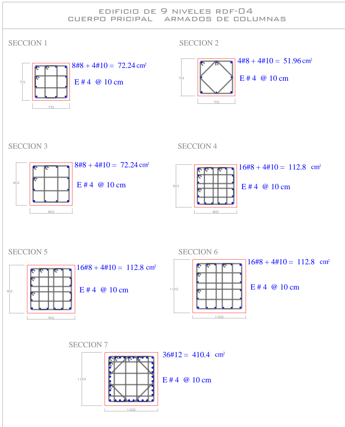
Fig 3.18.- Armados de acero longitudinal y transversal propuestos en columnas del eje C, edificio 9 niveles, Cuerpo Principal (caso A) de las NTC-Sismo, RDF-04
