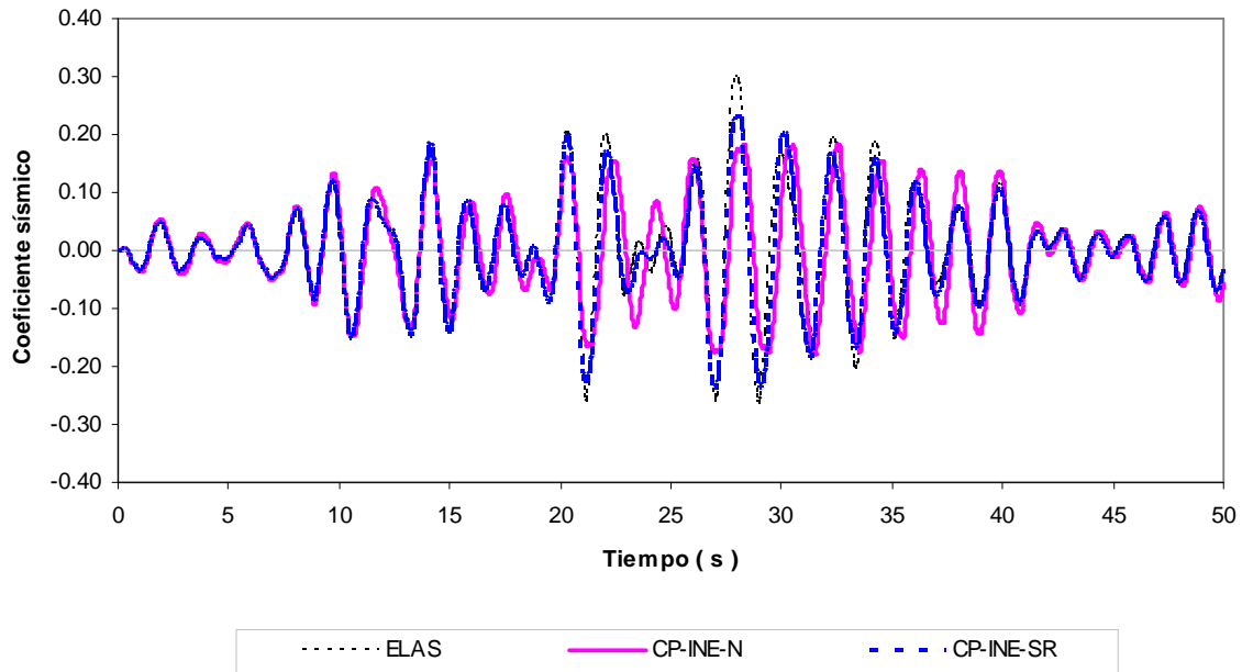
Fig 5.12.- Comparación de coeficientes sísmicos, análisis paso a paso elástico e inelástico (resistencias nominales y sobre-resistencias), edificio de 9 niveles, caso A (Cuerpo Principal)
