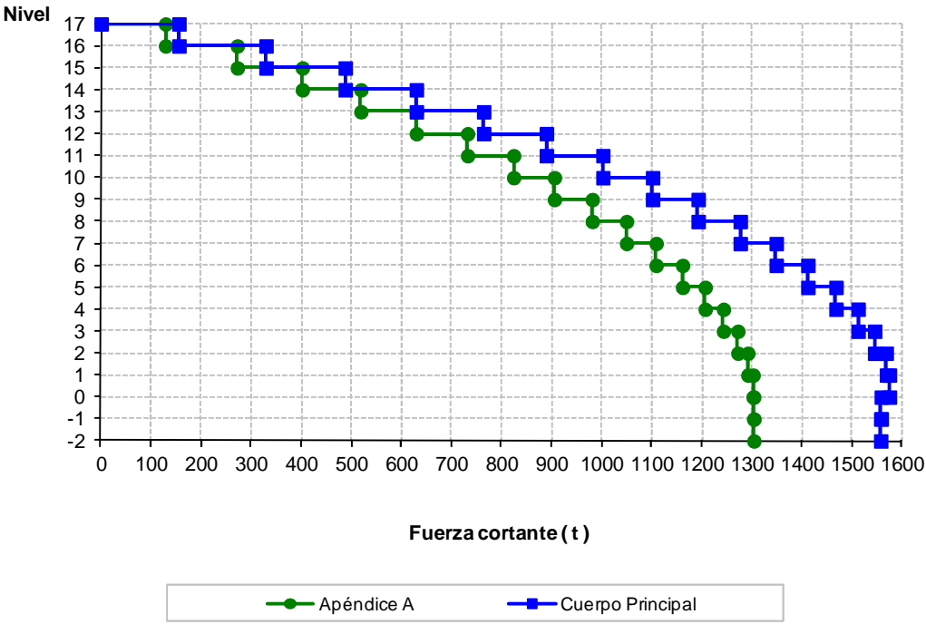
Fig 5.7.- Comparación de fuerzas cortantes de entrepiso, análisis dinámico modal espectral, edificio de 17 niveles, casos A (Cuerpo Principal) y B (Apéndice A)
