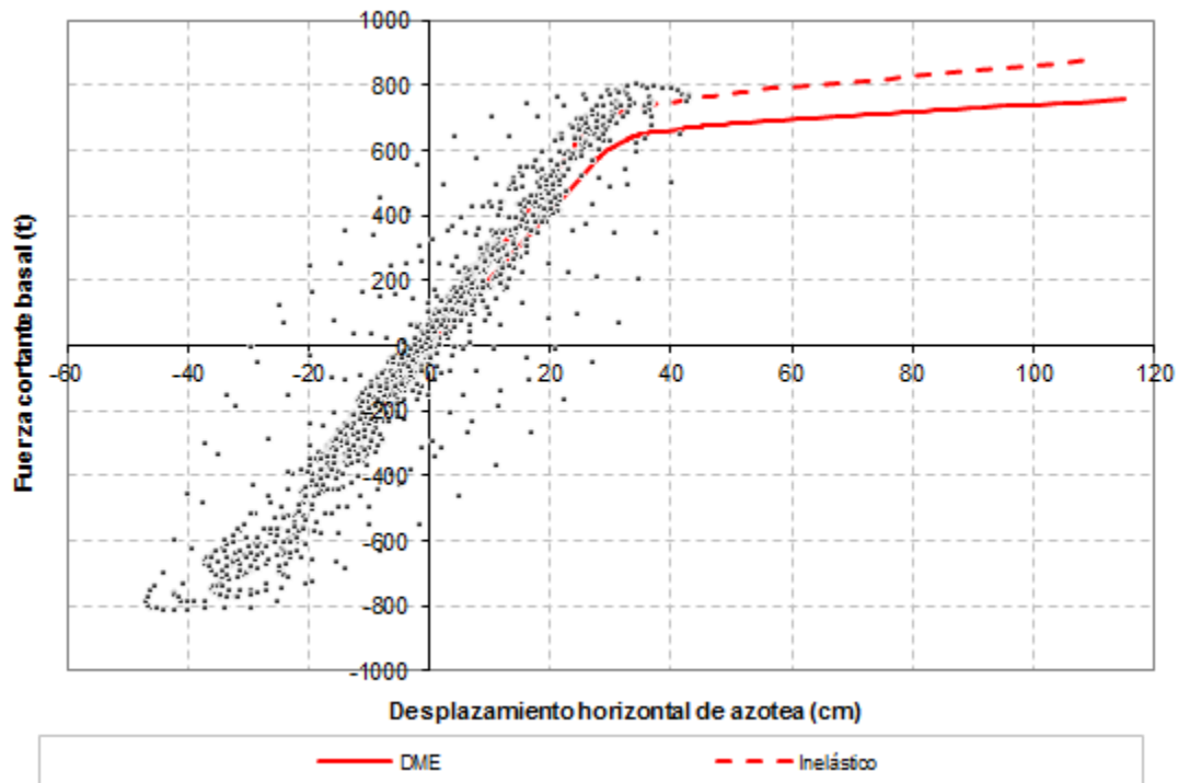
Fig 5.41.- Comparación de relaciones fuerza cortante basal-desplazamiento horizontal de azotea, análisis estático no-lineal ( Push-over ) y análisis paso a paso inelástico con sobre-resistencias, edificio de 17 niveles, caso B (Apéndice A)
