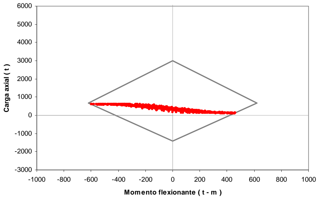
Fig 4.25.- Combinaciones momento flexionante-carga axial del extremo inferior de la columna 1, edificio 9 niveles, caso B (Apéndice A) con resistencias nominales
