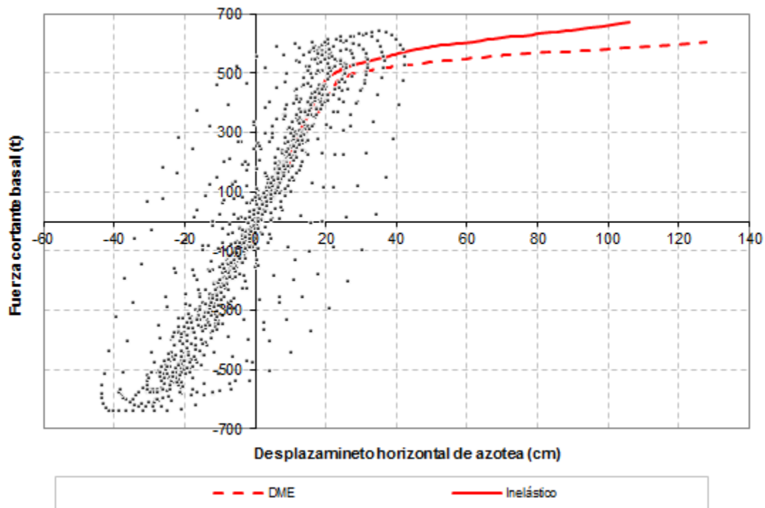
Fig 5.38.- Comparación de relaciones fuerza cortante basal-desplazamiento horizontal de azotea, análisis estático no-lineal (Push-over) y análisis paso a paso inelástico con resistencias nominales, edificio de 17 niveles, caso A (Cuerpo Principal)
