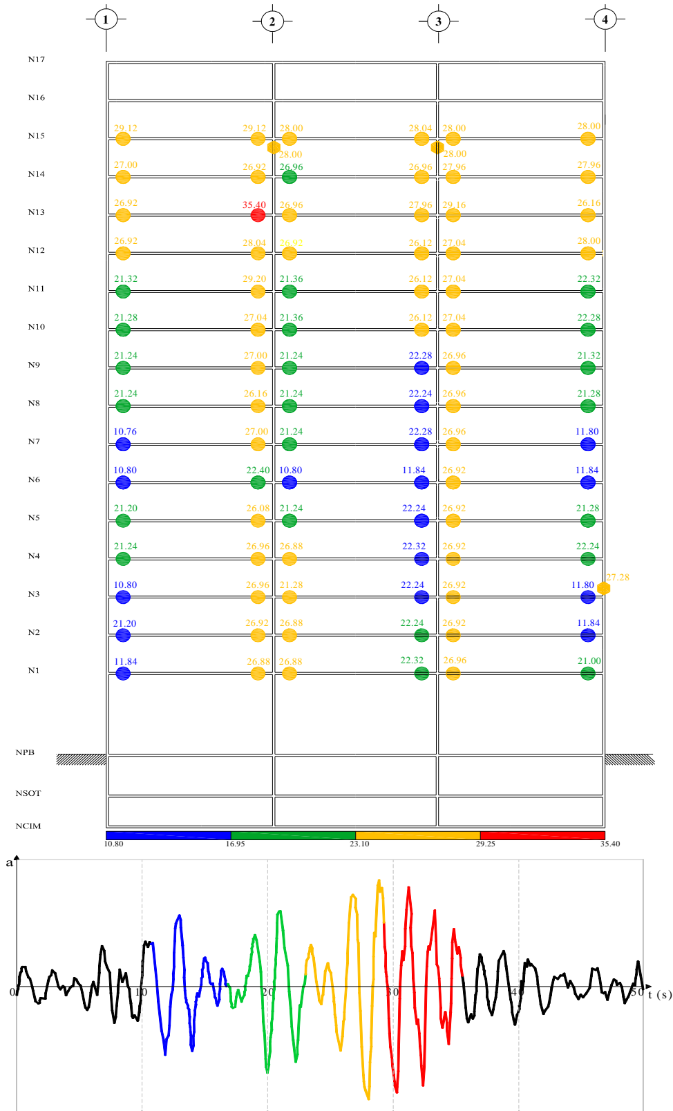
Fig 4.92.- Secuencia de formación y distribución global de articulaciones plásticas, edificio 17 niveles, caso A con sobre-resistencias
