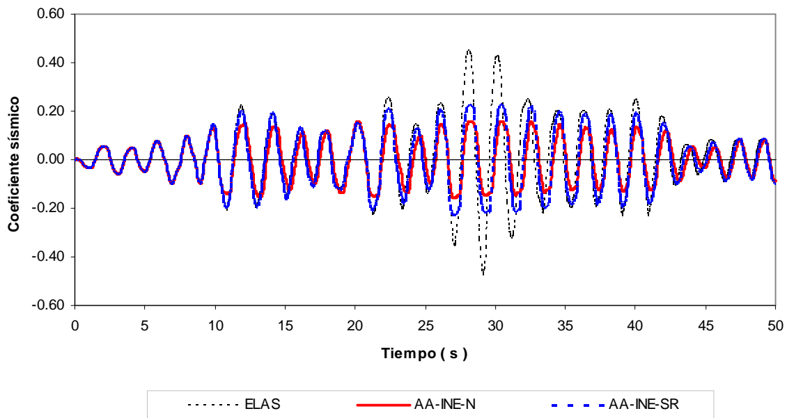
Fig 5.15.- Comparación de coeficientes sísmicos, análisis paso a paso elástico e inelástico (resistencias nominales y sobre-resistencias), edificio de 17 niveles, caso B (Apéndice A)
