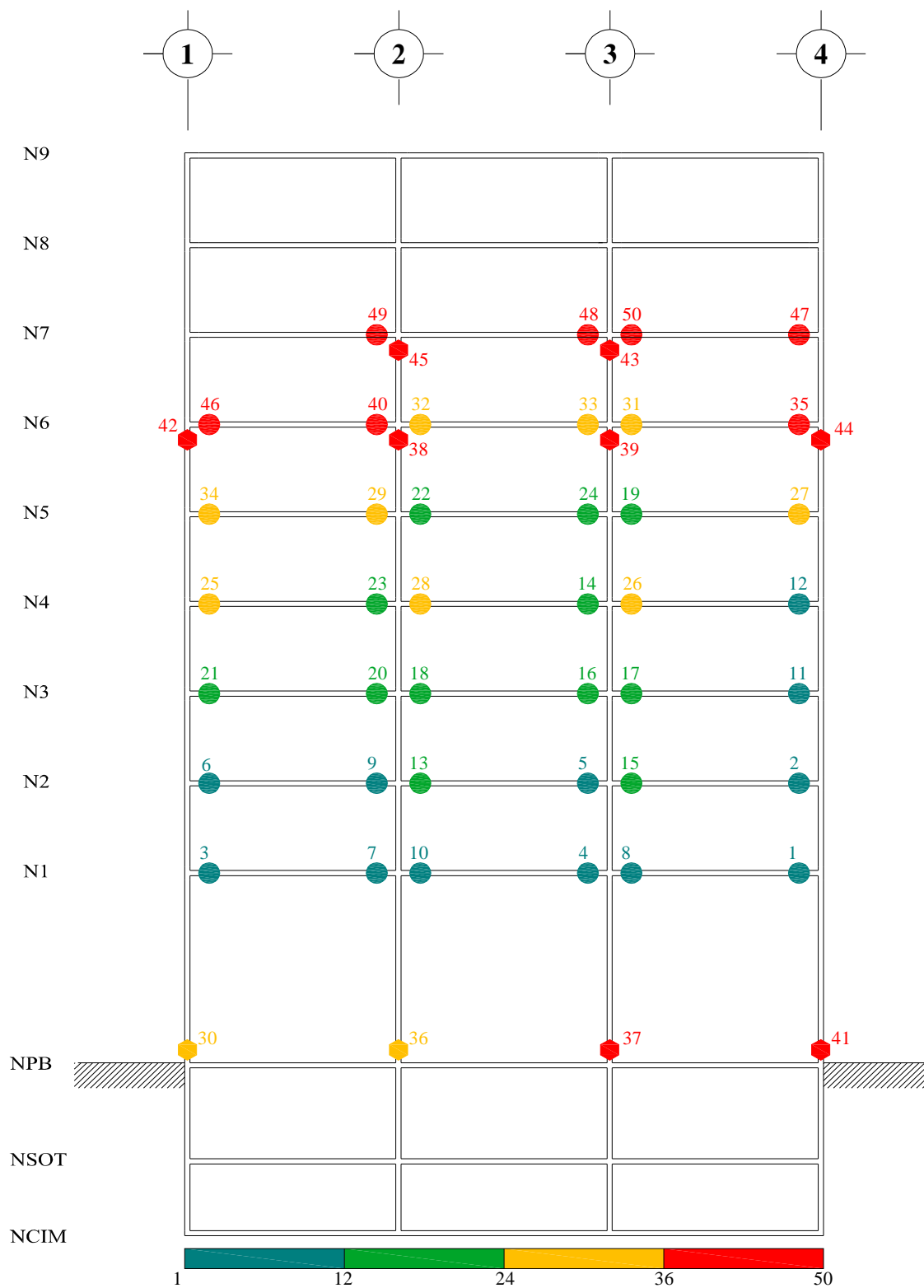
Fig A.19.- Secuencia de formación de articulaciones plásticas, análisis estático no-lineal (Push-over) con distribución de cargas de análisis paso a paso elástico, sobrerresistencias, edificio 9 niveles, caso B (Apéndice A)
