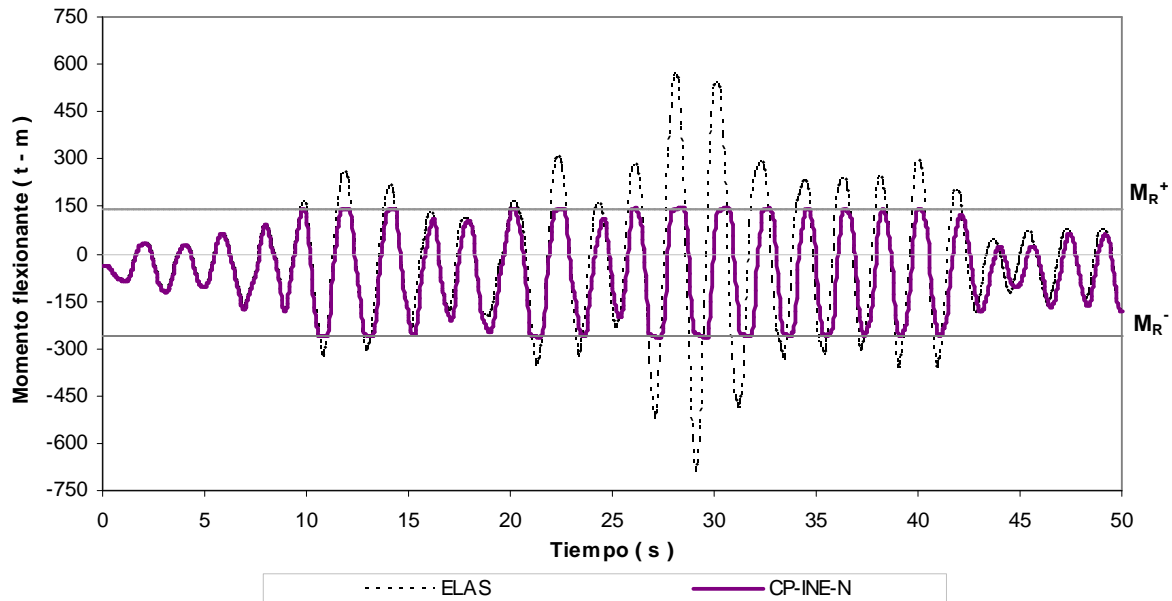
Fig 4.79.- Historias de momentos flexionantes en el extremo izquierdo de la viga 1, edificio 17 niveles, caso A (Cuerpo Principal) con resistencias nominales
