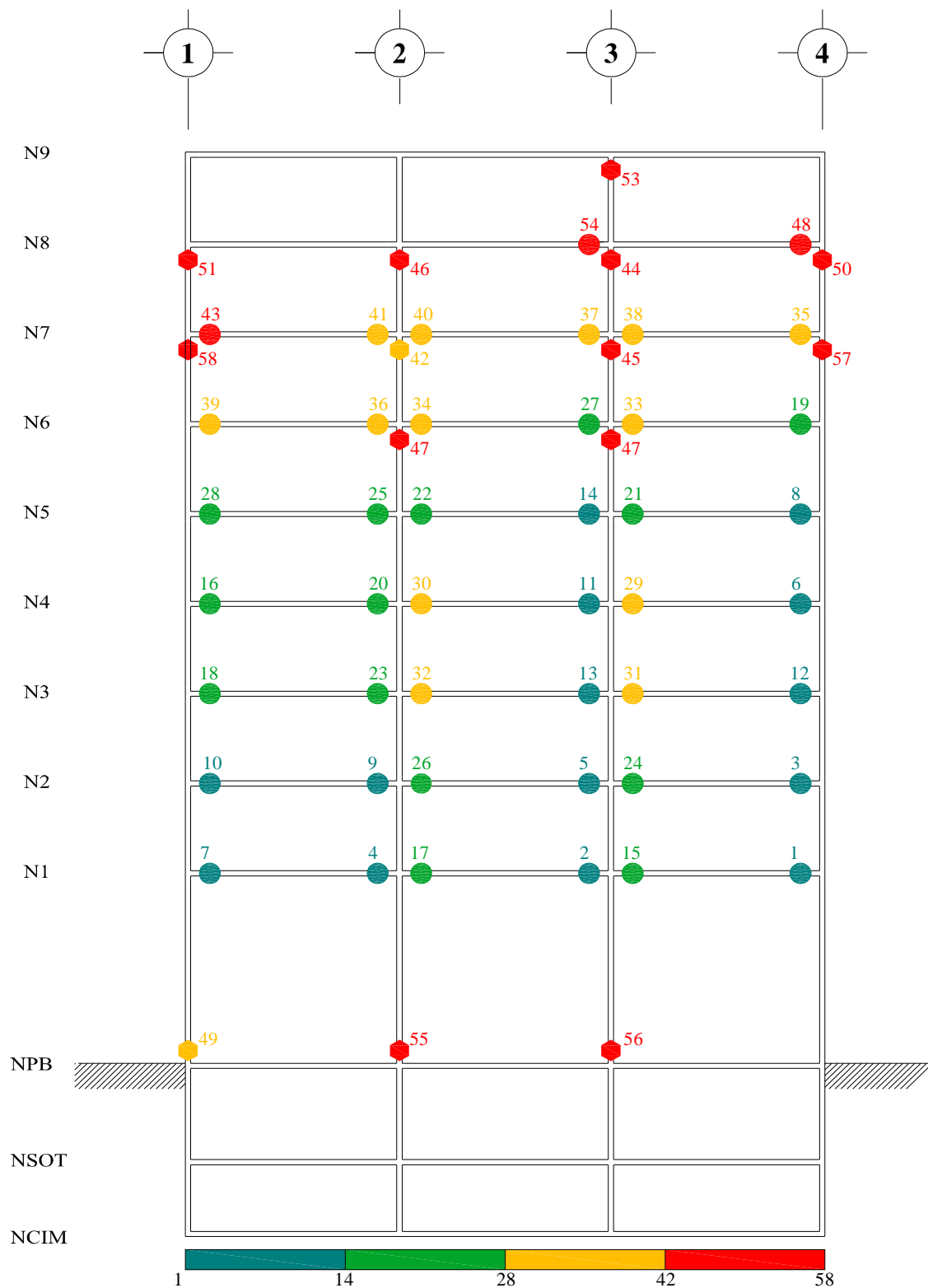
Fig A.12.- Secuencia de formación de articulaciones plásticas, análisis estático no-lineal (Push-over) con distribución de cargas laterales de análisis dinámico modal espectral (DME), sobre-resistencias, edificio 9 niveles, caso A (Cuerpo Principal)
