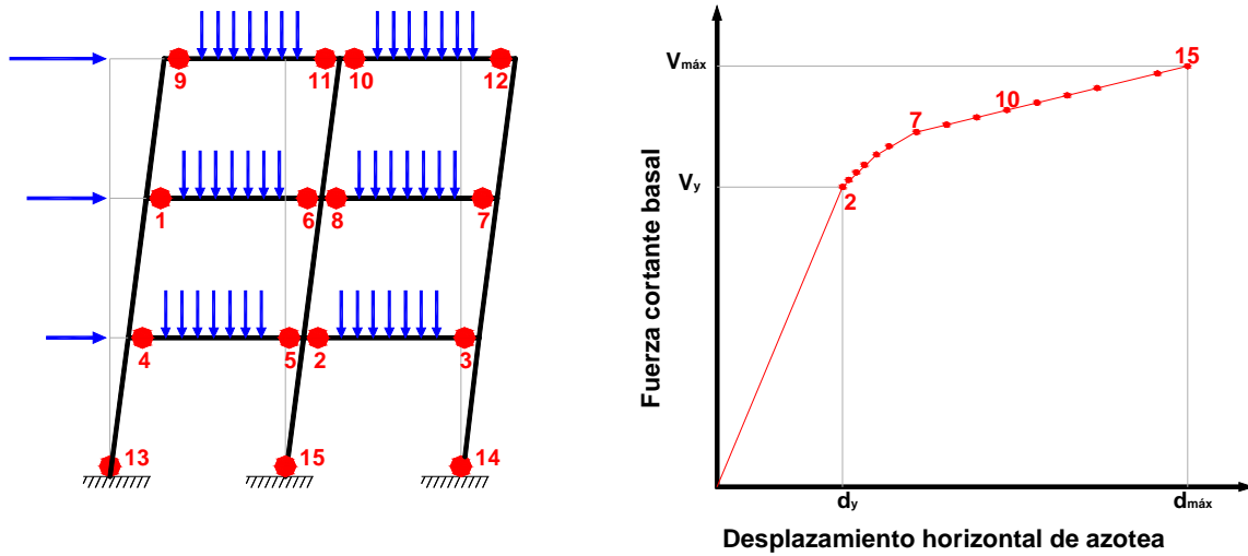
Fig 2.4.- Ilustración del análisis estático no-lineal Push-over
