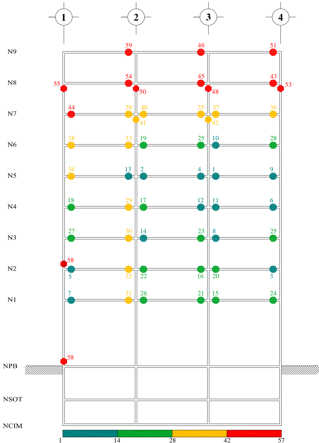
Fig 4.109.- Mecanismo de falla y secuencia de formación de articulaciones plásticas, edificio 9 niveles, caso B (Apéndice A) con resistencias nominales, distribución de fuerzas laterales del análisis paso a paso inelástico para \Delta_{máx}
