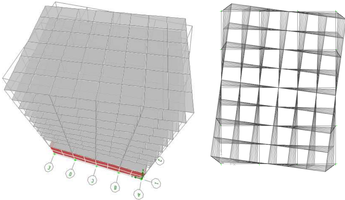
Fig 3.4c.- Vista en elevación y planta de la deformada del tercer modo de vibrar del edificio de 9 niveles
