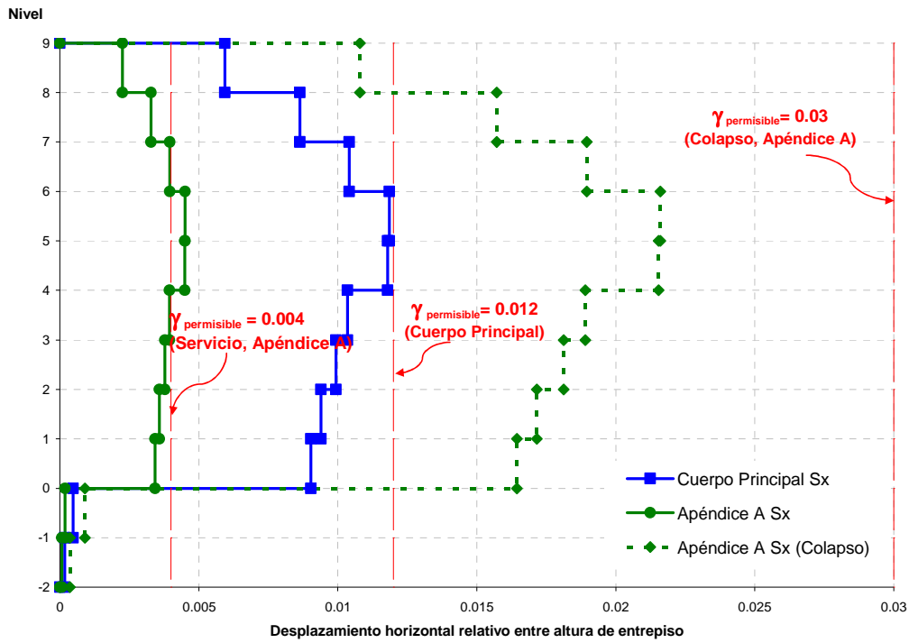
Fig 3.7.- Relaciones máximas de desplazamiento lateral relativo entre altura de entrepiso, sismo en dirección "X", edificio 9 niveles, Apéndice A y Cuerpo principal de las NTC-Sismo, RDF-04
