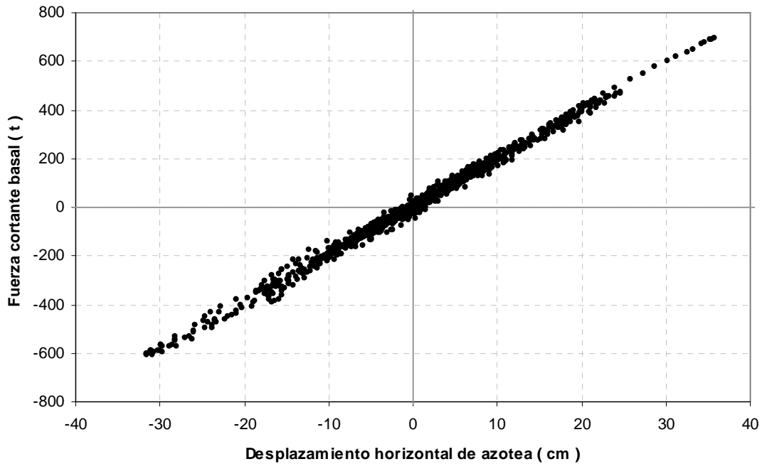
Fig 4.17.- Relaciones fuerza cortante basal – desplazamiento lateral de azotea, edificio 9 niveles, comportamiento elástico
