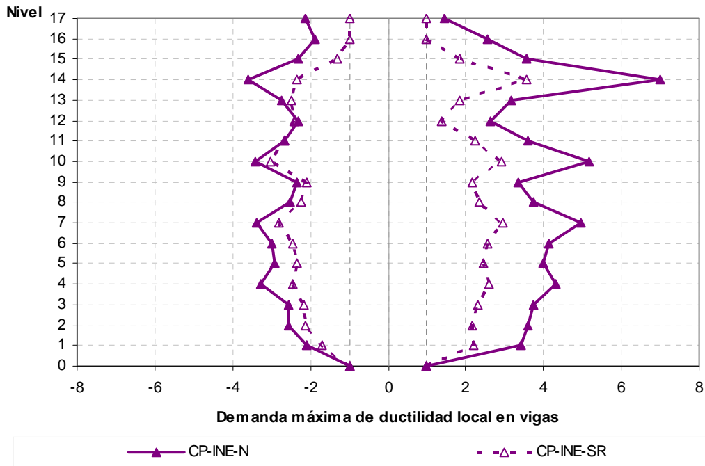
Fig 4.97.- Demandas máximas de ductilidad local en vigas, edificio 17 niveles, caso A (Cuerpo Principal) con resistencias nominales y con sobre-resistencias
