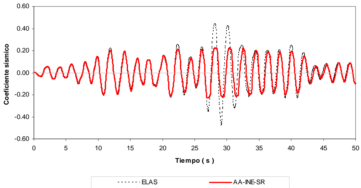
Fig 4.64- Historias de coeficientes sísmicos, edificio 17 niveles, caso B (Apéndice A) con sobre-resistencias
