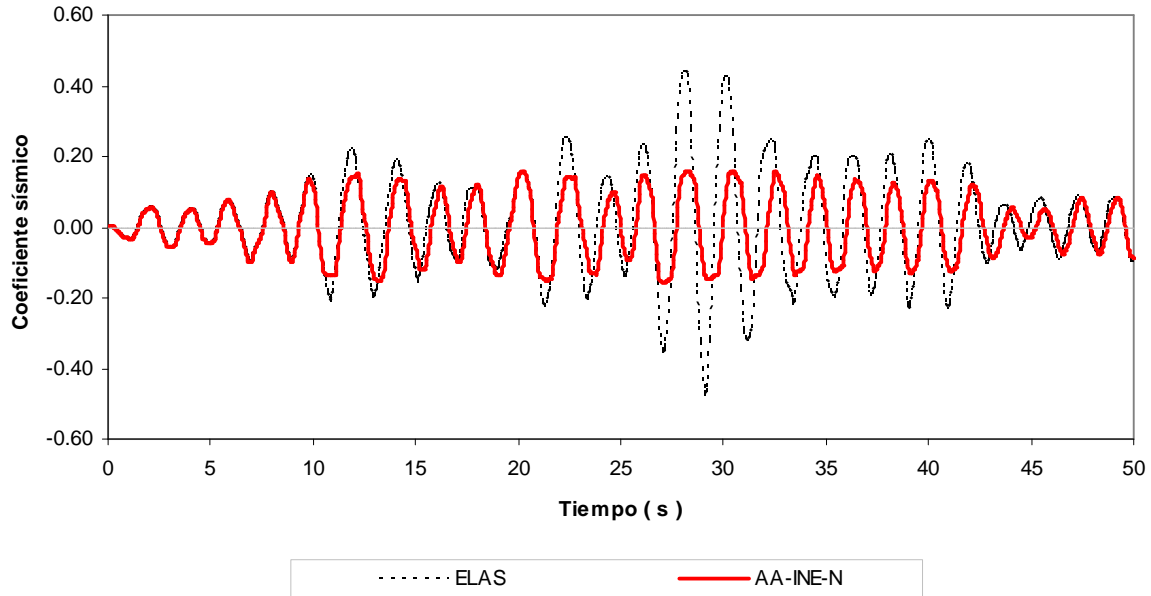
Fig 4.63.- Historias de coeficientes sísmicos, edificio 17 niveles, caso B (Apéndice A) con resistencias nominales
