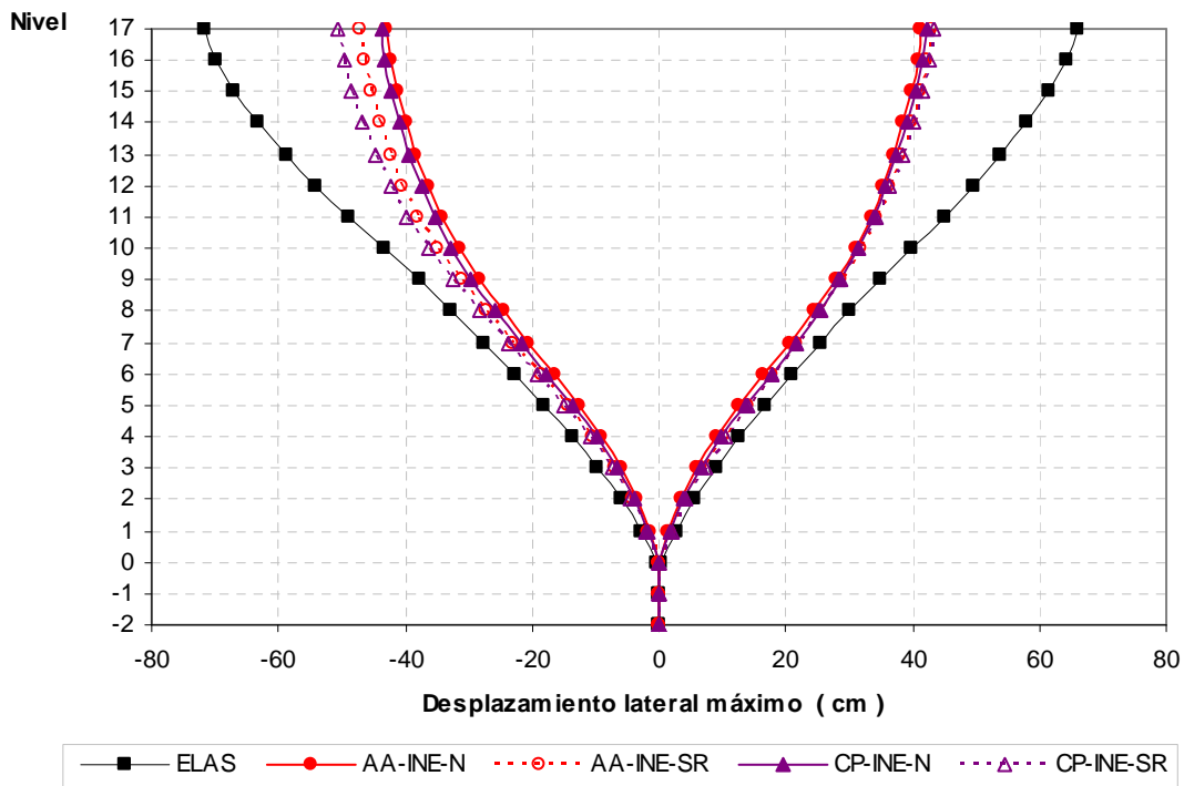
Fig 5.9.- Comparación de desplazamientos horizontales máximos, análisis paso a paso elástico e inelástico (resistencias nominales y sobre-resistencias), edificio de 17 niveles, casos A (Cuerpo Principal) y B (Apéndice A)
