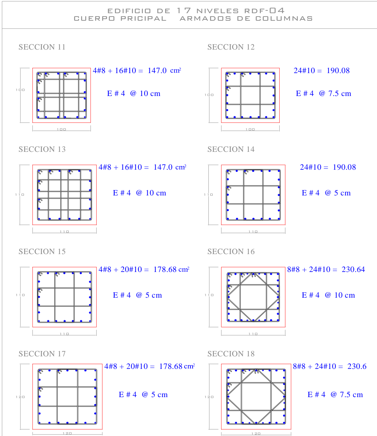
Fig 3.33b.- Armados de acero longitudinal y transversal propuestos en columnas, edificio 17 niveles, Cuerpo Principal (caso A) de las NTC-Sismo, RDF-04
