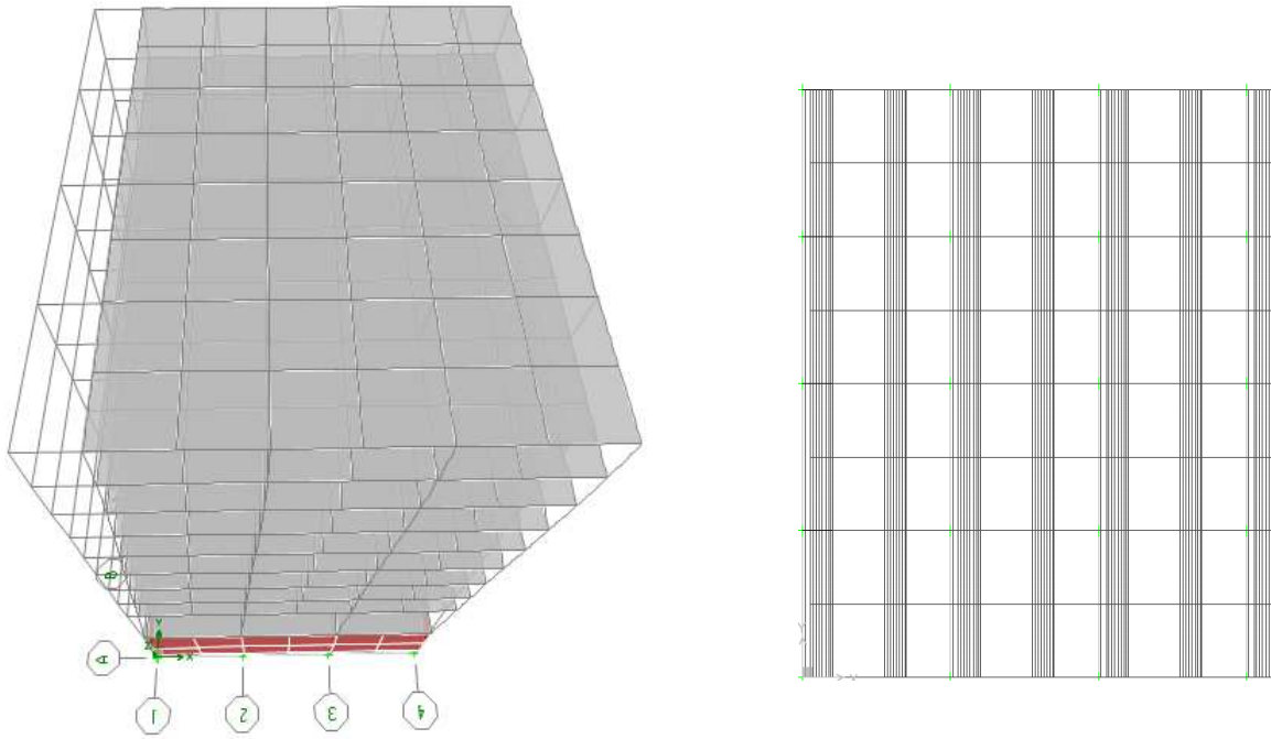
Fig 3.4a.- Vista en elevación y planta de la deformada del primer modo de vibrar del edificio de 9 niveles
