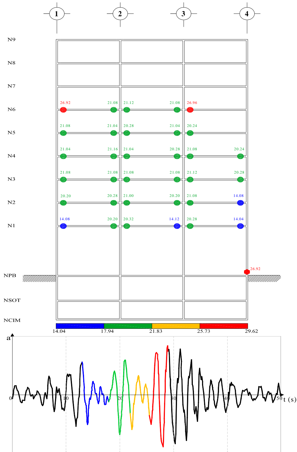
Fig 4.46.- Secuencia de formación y distribución global de articulaciones plásticas, edificio 9 niveles, caso B con sobre-resistencias
