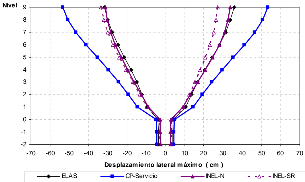
Fig 4.3.- Desplazamientos horizontales máximos, edificio 9 niveles, caso A
