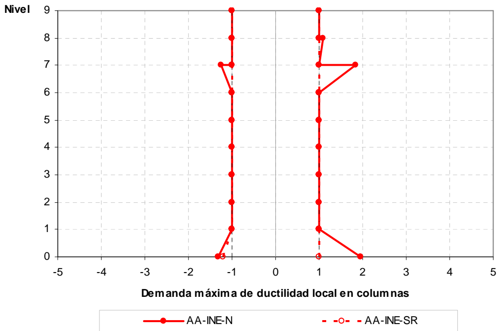
Fig 4.48.- Demandas máximas de ductilidad local en columnas, edificio 9 niveles, caso B (Apéndice A) con resistencias nominales y con sobre-resistencias
