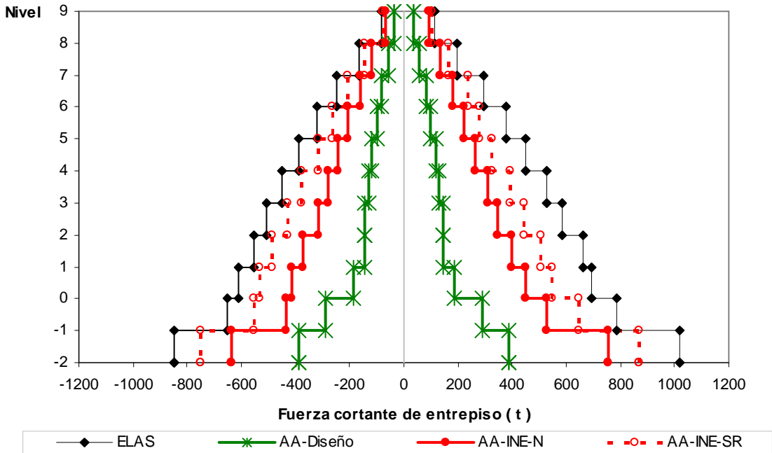
Fig 4.12.- Distribución en elevación de las fuerzas cortantes de entrepiso, edificio 9 niveles, caso B (Apéndice A)
