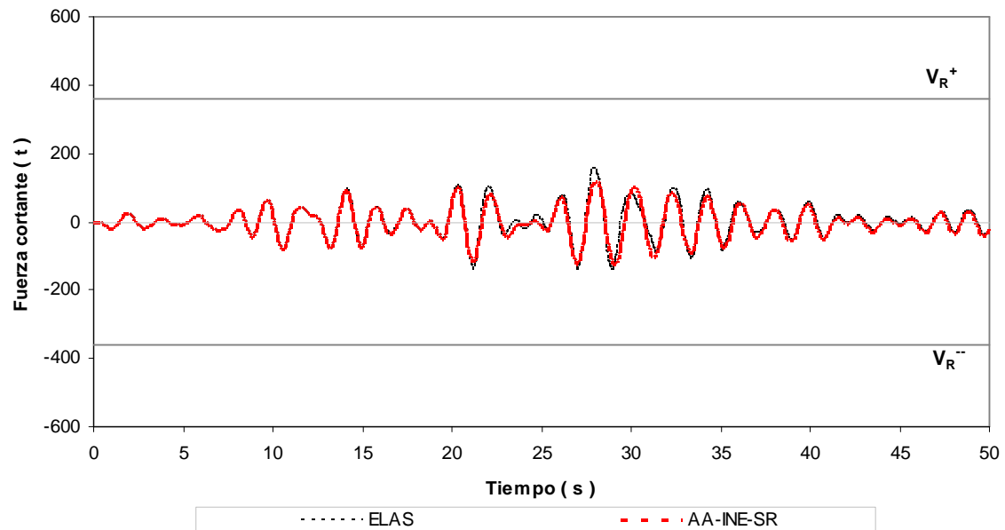
Fig 4.30.- Historias de fuerzas cortantes en el extremo inferior de la columna 1, edificio 9 niveles, caso B (Apéndice A) con sobre-resistencias
