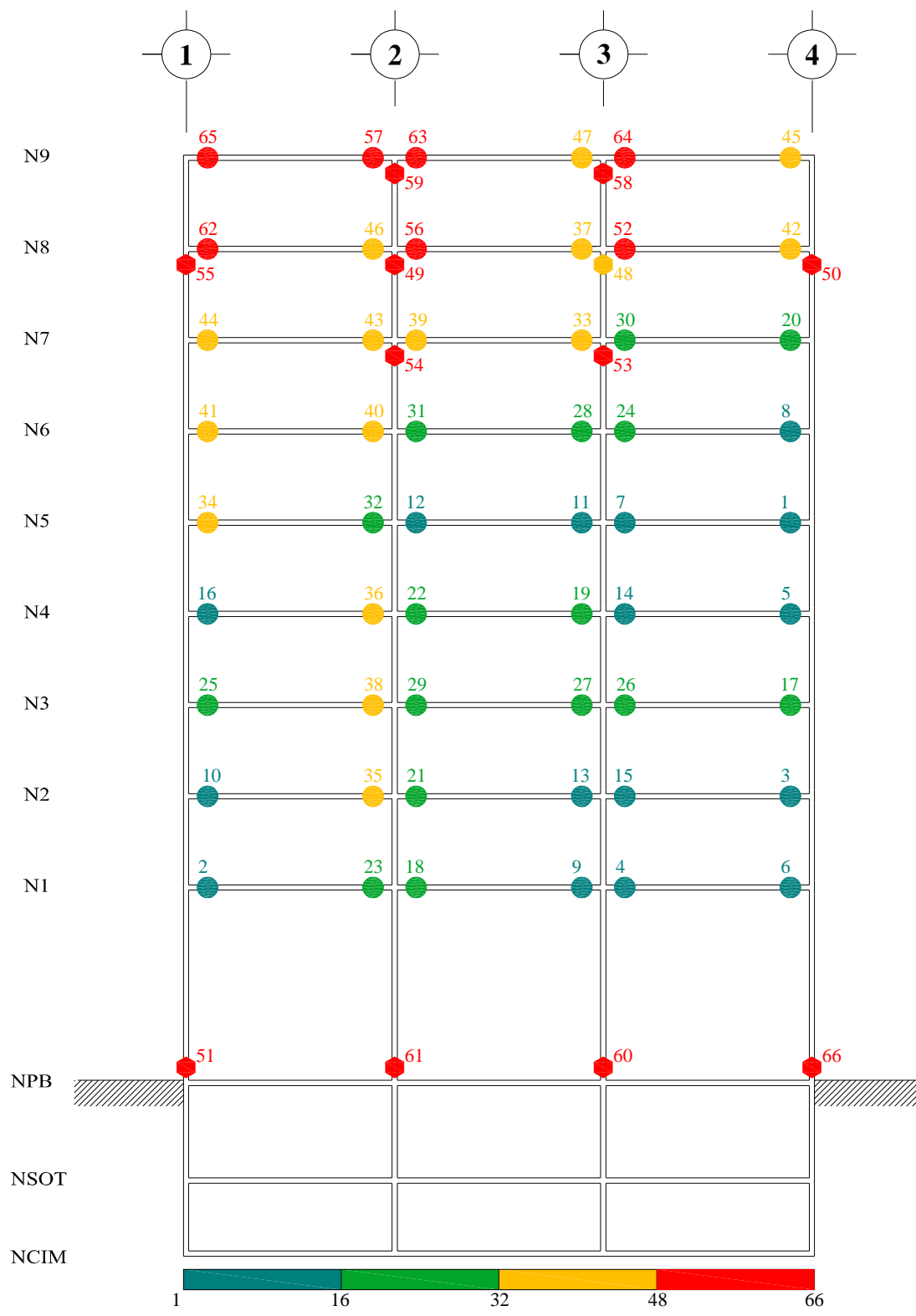
Fig A.11.- Secuencia de formación de articulaciones plásticas, análisis estático no-lineal (Push-over) con distribución de cargas laterales lineal triangular, resistencias nominales, edificio 9 niveles, caso A (Cuerpo Principal)
