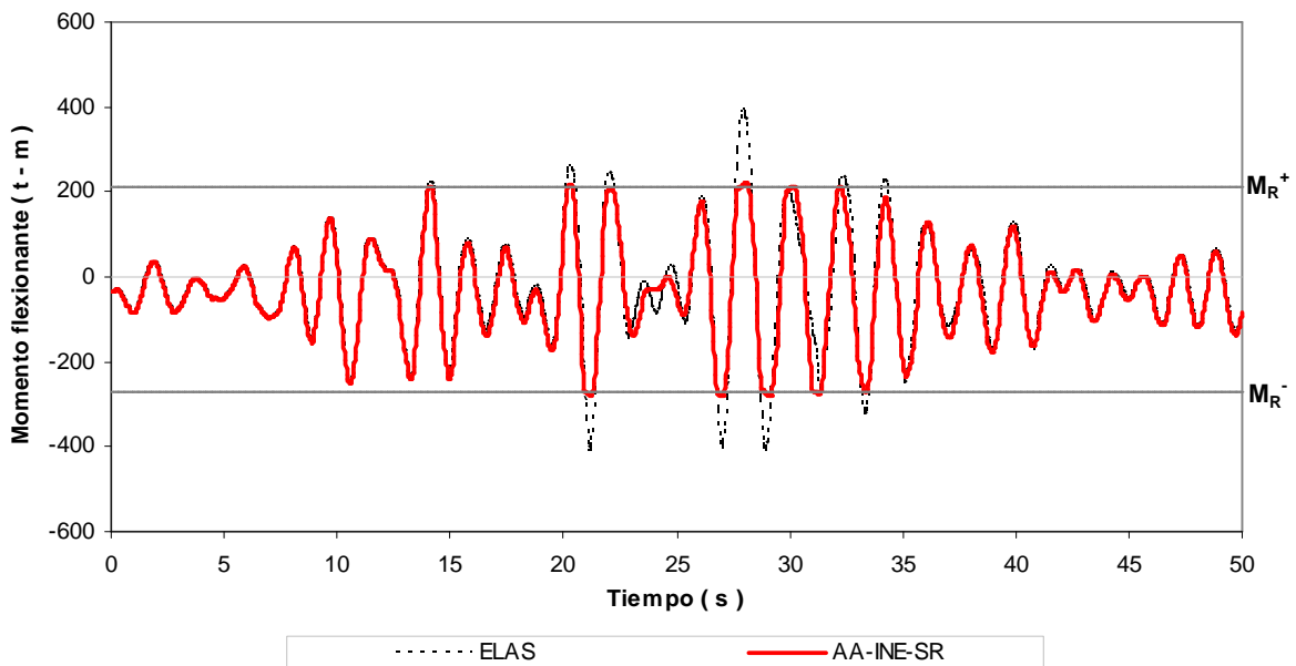
Fig 4.34.- Historias de momentos flexionantes en el extremo izquierdo de la viga 1, edificio 9 niveles, caso B (Apéndice A) con sobre-resistencias
