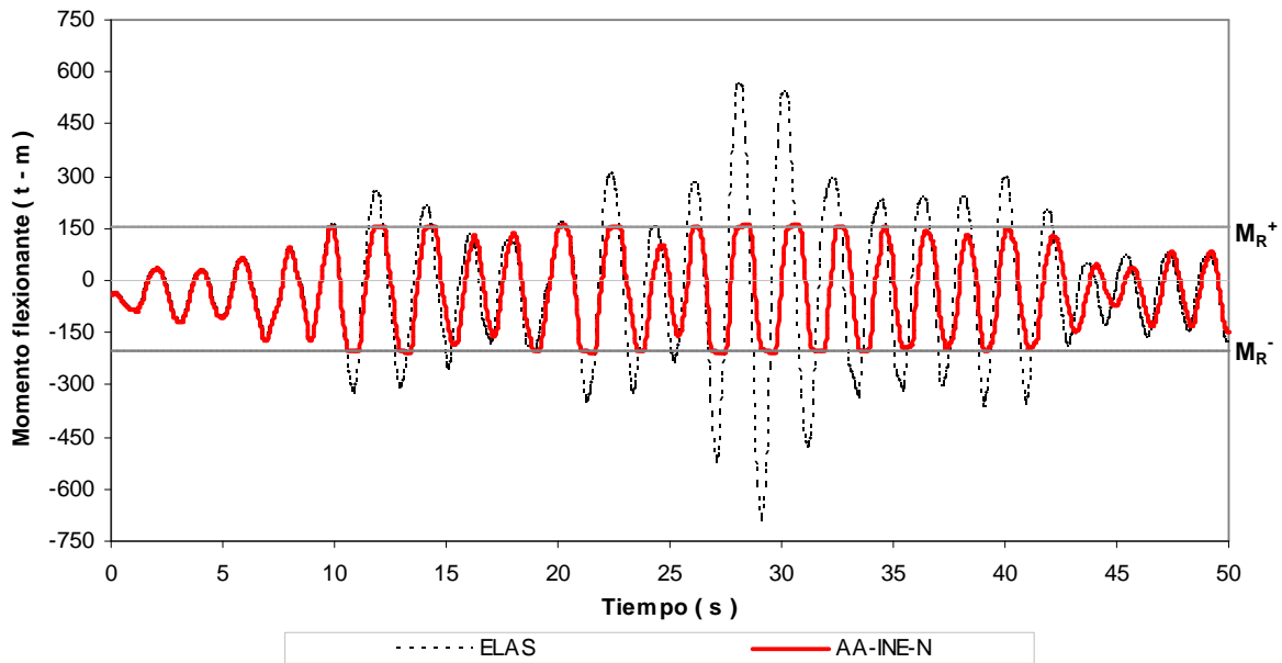
Fig 4.81.- Historias de momentos flexionantes en el extremo izquierdo de la viga 1, edificio 17 niveles, caso B (Apéndice A) con resistencias nominales
