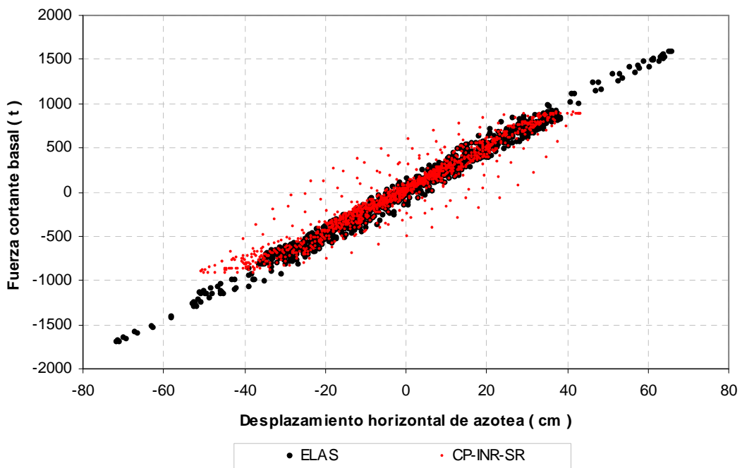
Fig 5.21.- Comparación de relaciones fuerza cortante basal-desplazamiento horizontal de azotea, análisis paso a paso elástico e inelástico (sobre-resistencias), edificio de 17 niveles, caso A (Cuerpo Principal)
