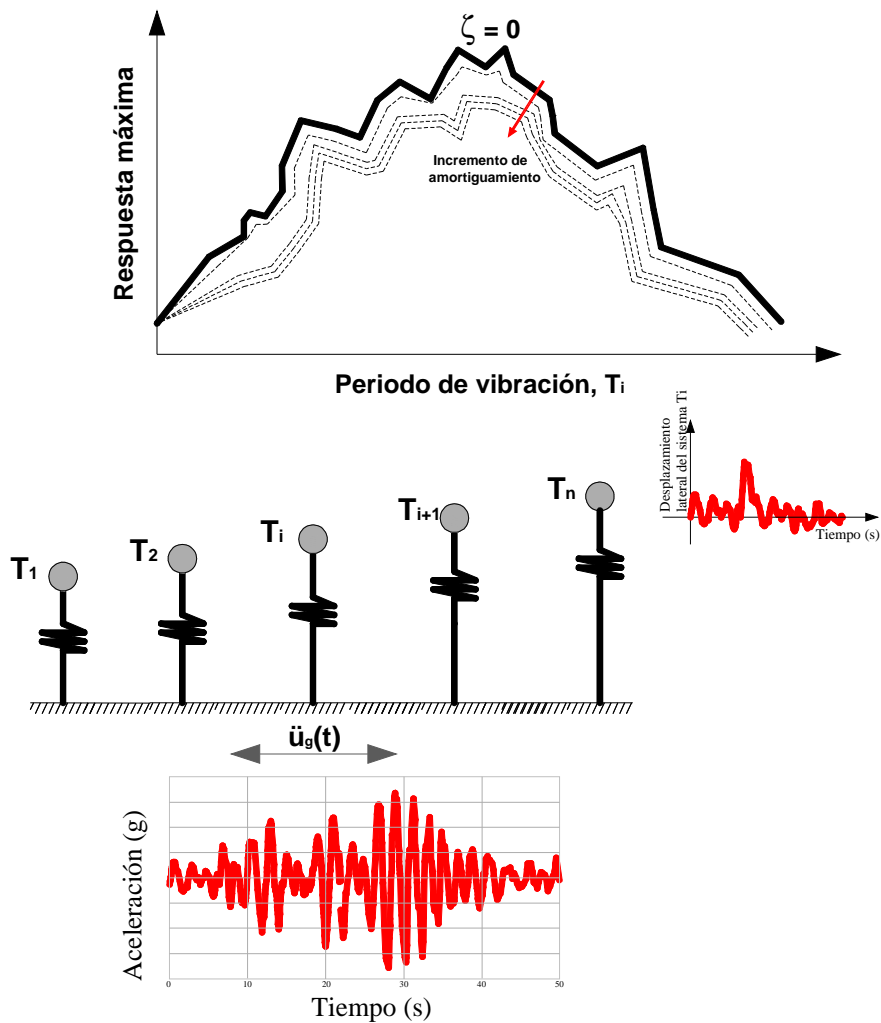
Fig 2.8.- Construcción de un espectro de respuesta
