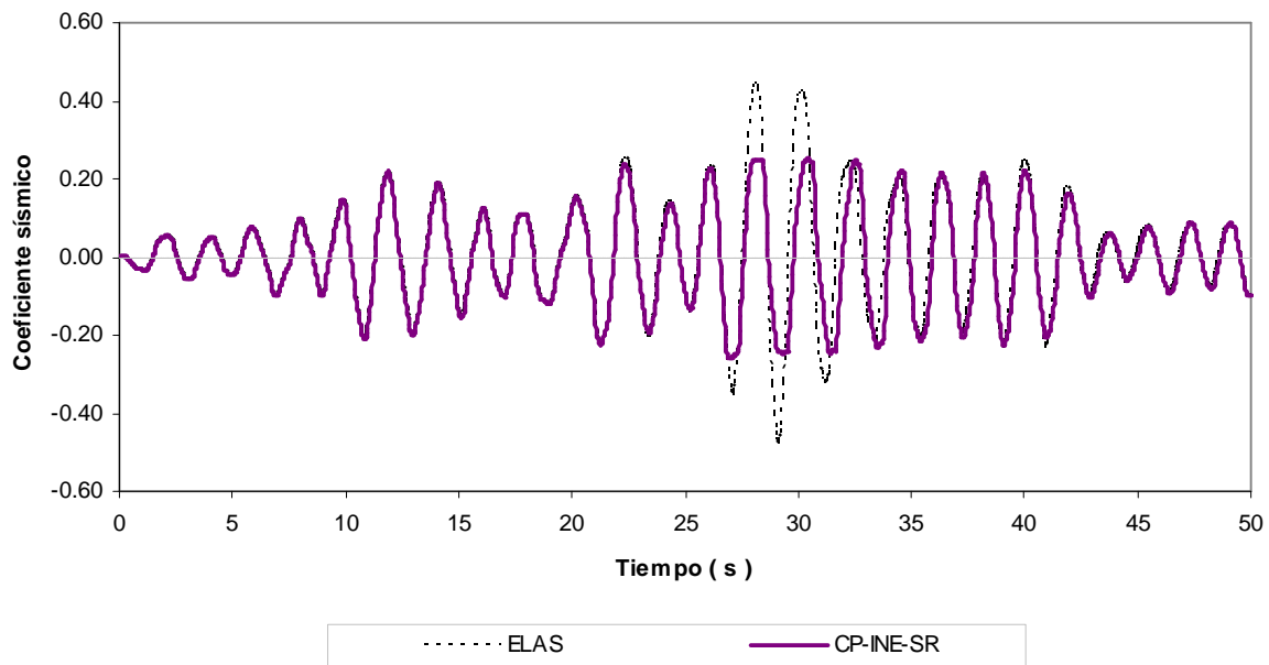
Fig 4.62.- Historias de coeficientes sísmicos, edificio 17 niveles, caso A (Cuerpo Principal) con sobre-resistencias
