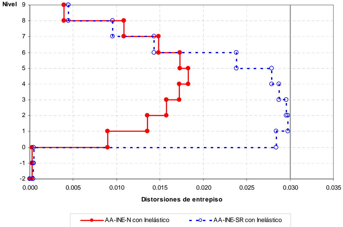
Fig 4.106.- Relaciones desplazamiento lateral relativo entre altura de entropiso, edificio 9 niveles, caso B con resistencias nominales y sobre-resistencias, distribución de cargas del análisis paso a paso inelástico para \Delta_{máx}
