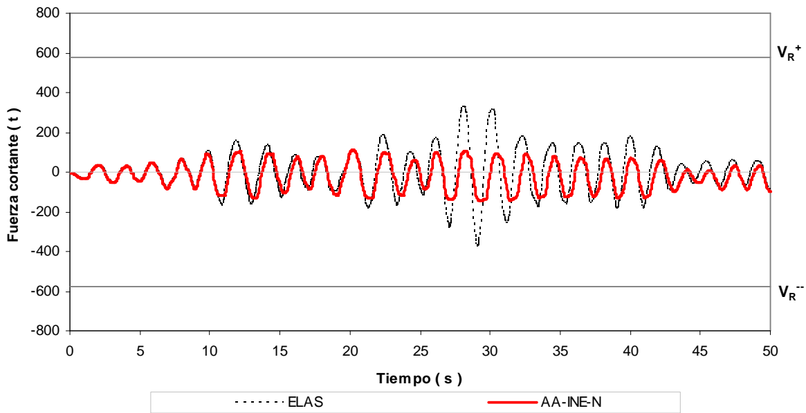
Fig 4.77.- Historias de fuerzas cortantes en el extremo inferior de la columna 1, edificio 17 niveles, caso B (Apéndice A) con resistencias nominales
