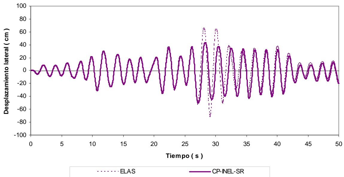
Fig 4.54.- Historias de desplazamientos de azotea, edificio 17 niveles, caso A (Cuerpo Principal) con sobre-resistencias
