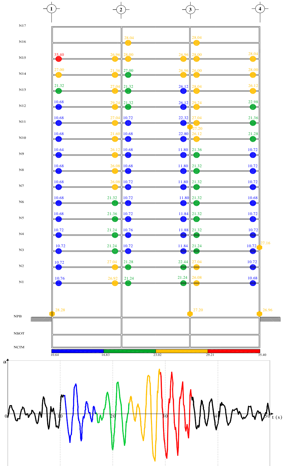
Fig 4.94.- Secuencia de formación y distribución global de articulaciones plásticas, edificio 17 niveles, caso B con sobre-resistencias
