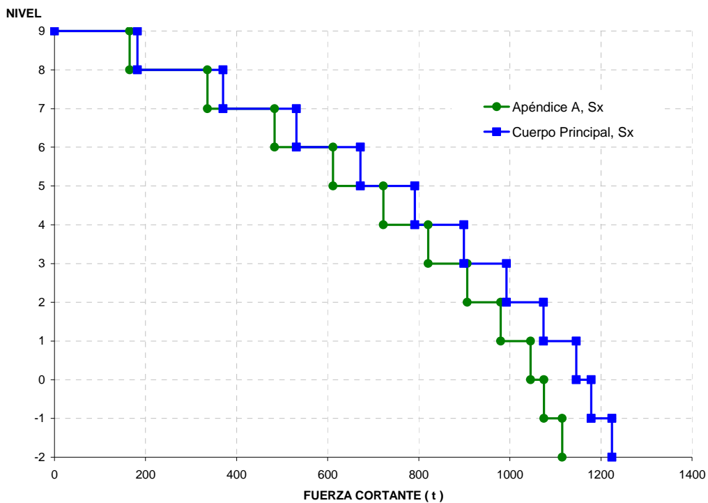
Fig 3.9.- Fuerzas cortantes de entrepiso, sismo en dirección "X", edificio 9 niveles, Apéndice A y Cuerpo Principal de las NTC-Sismo, RDF-04
