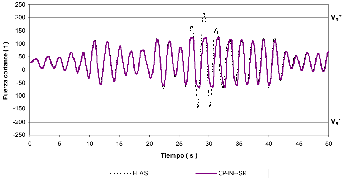
Fig 4.84.- Historias de fuerzas cortantes en el extremo izquierdo de la viga 1, edificio 17 niveles, caso A (Cuerpo Principal) con sobre-resistencias
