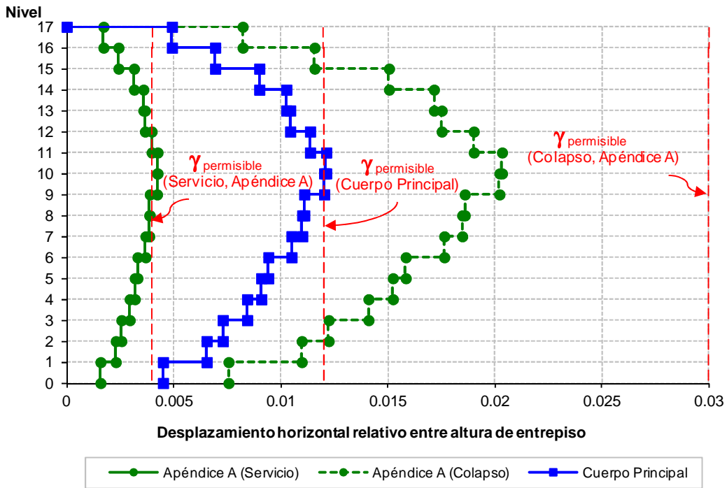
Fig 5.5.- Comparación de relaciones máximas de desplazamiento horizontal relativo entre altura de entrepiso, análisis dinámico modal espectral, edificio de 17 niveles, casos A (Cuerpo Principal) y B (Apéndice A)
