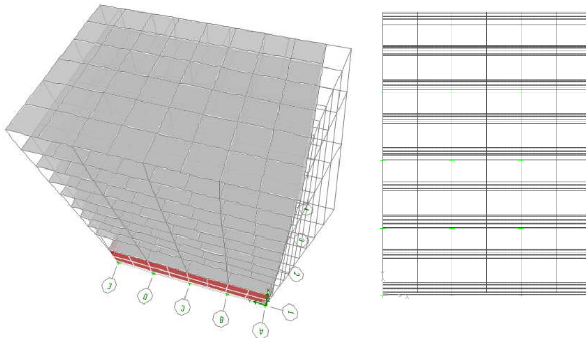
Fig 3.4b.- Vista en elevación y planta de la deformada del segundo modo de vibrar del edificio de 9 niveles
