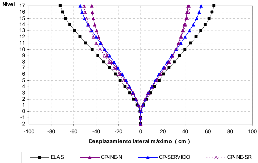
Fig 4.51.- Desplazamientos horizontales máximos, edificio 17 niveles, caso A
