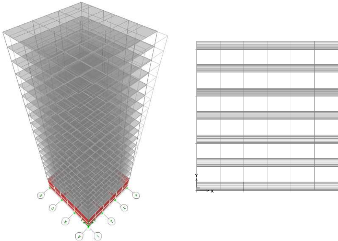
Fig 3.22b.- Vista en elevación y planta de de la deformada del segundo modo de vibrar del edificio 17 niveles
