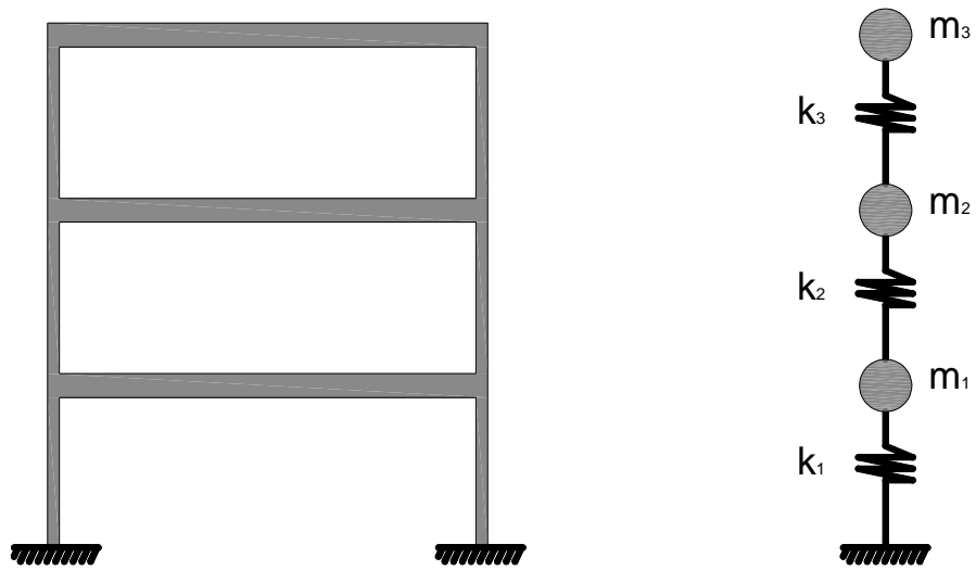
Fig 2.1.- Modelo de edificio de tres niveles
