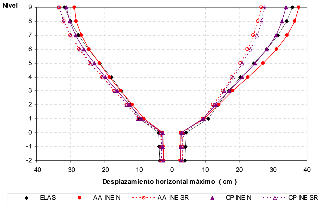
Fig 5.8.- Comparación de desplazamientos horizontales máximos, análisis paso a paso elástico e inelástico (resistencias nominales y sobre-resistencias), edificio de 9 niveles, casos A (Cuerpo Principal) y B (Apéndice A)
