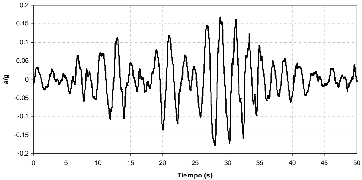
Fig 4.1.- Acelerograma SCT-EW-85
