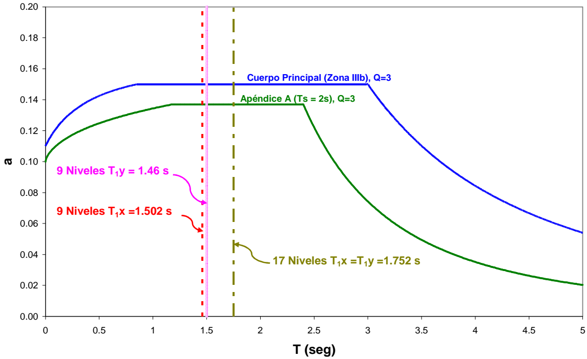
Fig 3.1.- Comparación de espectros de diseño inelásticos para Q=3 del Cuerpo Principal (Zona IIIb) y del Apéndice A ( T_s=2s ) de las NTC-Sismo del RDF-04
