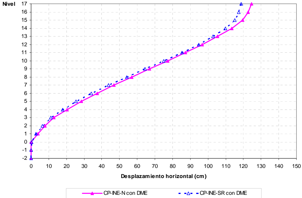
Fig 4.119.- Desplazamientos horizontales máximos, edificio 17 niveles, caso A con resistencias nominales y sobre-resistencias, distribución de fuerzas laterales del análisis dinámico modal espectral
