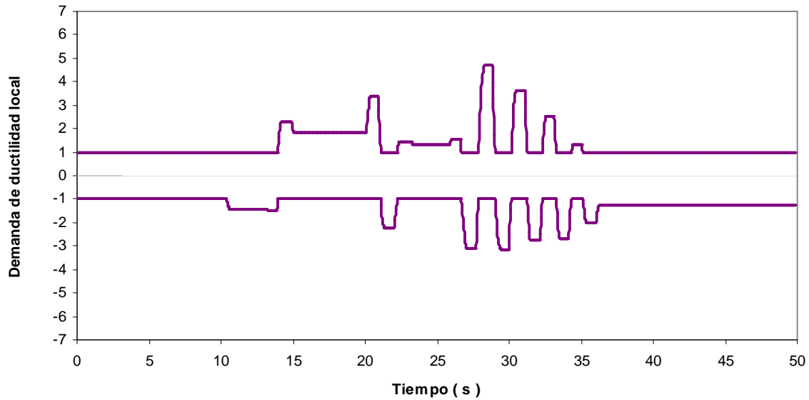
Fig 4.39.- Historias de demandas de ductilidad en el extremo izquierdo de la viga 1, edificio 9 niveles, caso A (Cuerpo Principal) con resistencias nominales
