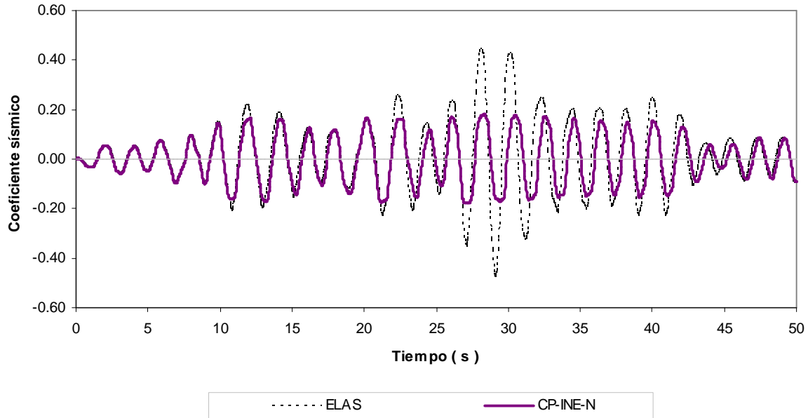
Fig 4.61.- Historias de coeficientes sísmicos, edificio 17 niveles, caso A (Cuerpo Principal) con resistencias nominales
