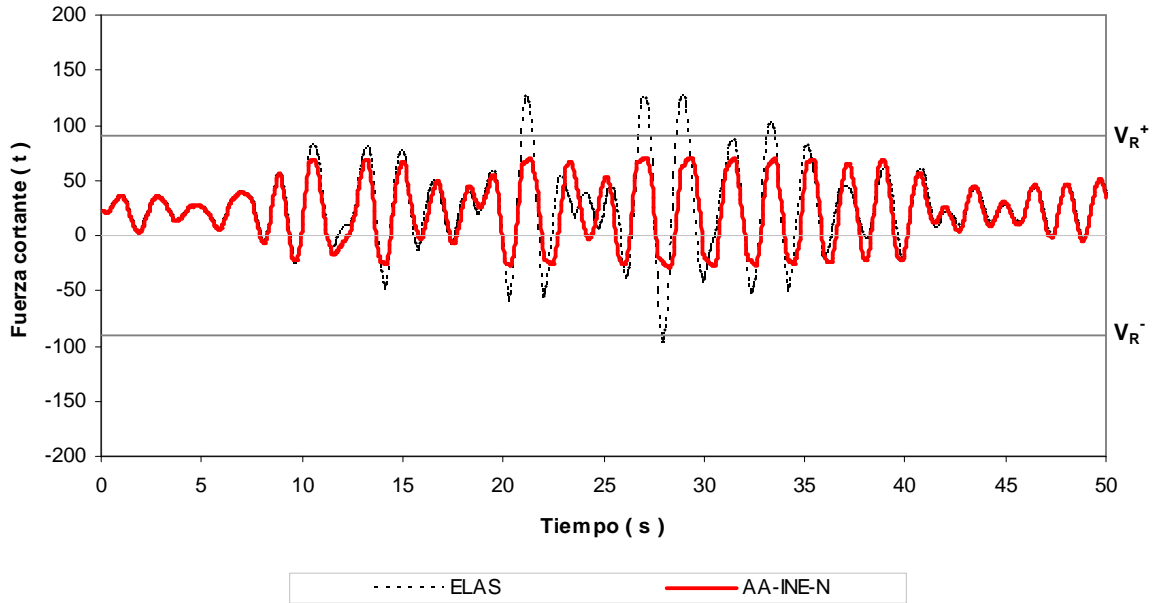
Fig 4.37.- Historias de fuerzas cortantes en el extremo izquierdo de la viga 1, edificio 9 niveles, caso B (Apéndice A) con resistencias nominales
