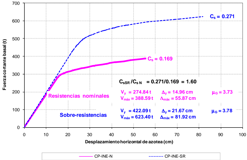
Fig 4.101.- Curvas fuerza cortante basal-desplazamiento lateral de azotea, edificio 9 niveles, caso A (Cuerpo Principal) con resistencias nominales y sobre-resistencias, distribución de fuerzas laterales del análisis paso a paso inelástico para \Delta_{máx}
