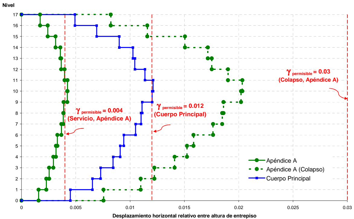
Fig 3.24.- Relaciones máximas de desplazamiento lateral relativo entre altura de entrepiso, sismo en dirección “X” y “Y”, edificio 17 niveles, Apéndice A y Cuerpo Principal de las NTC-Sismo, RDF-04
