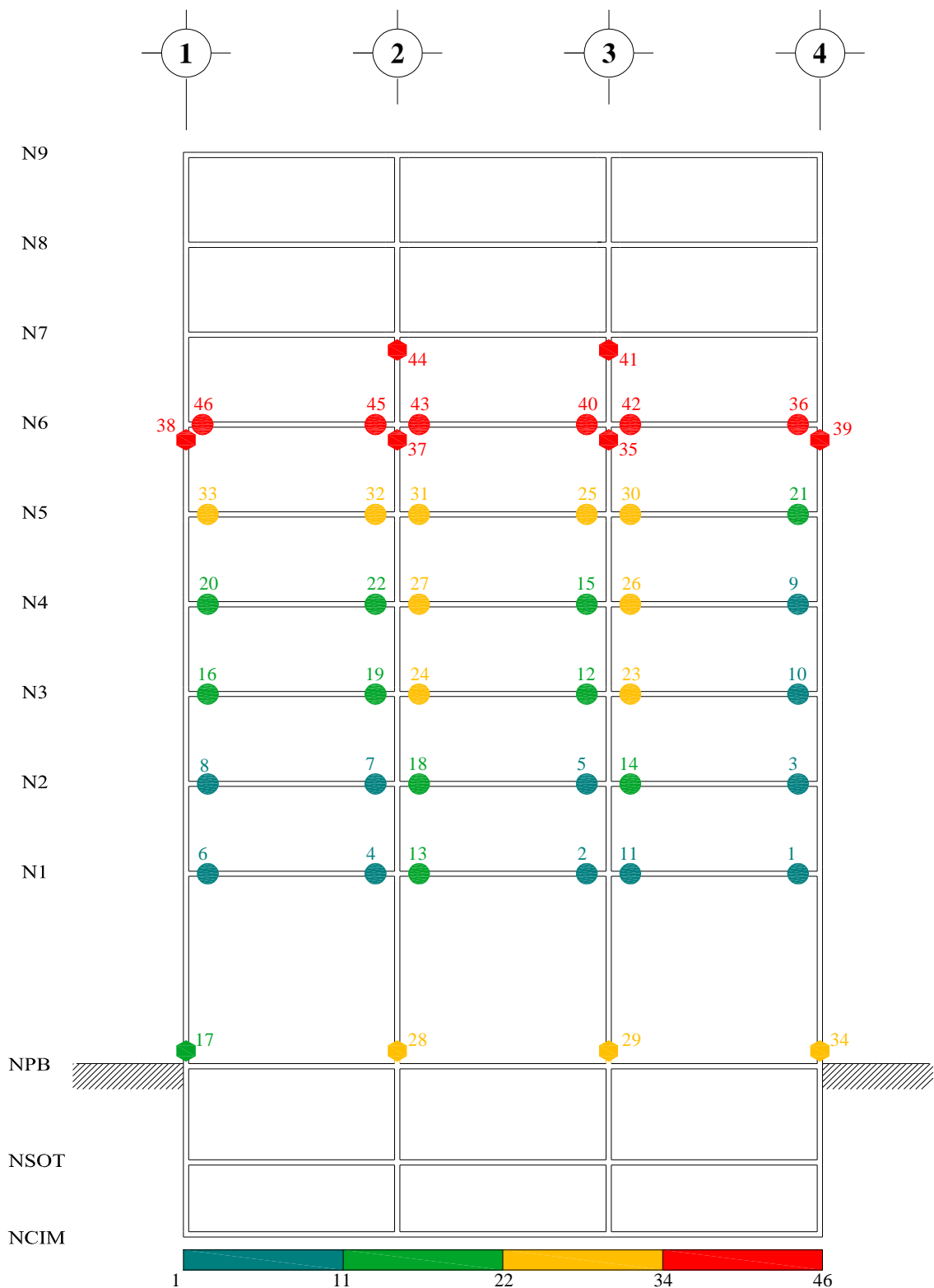
Fig A.13.- Secuencia de formación de articulaciones plásticas, análisis estático no-lineal (Push-over) con distribución de cargas laterales de análisis paso a paso elástico, sobre-resistencia, edificio 9 niveles, caso A (Cuerpo Principal)
