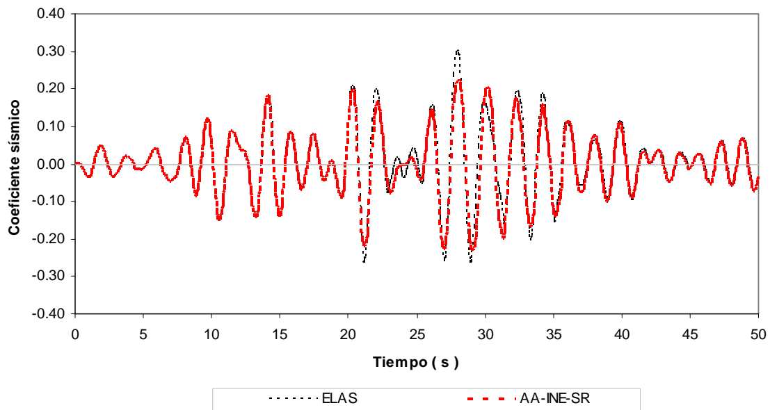
Fig 4.16.- Historias de coeficientes sísmicos, edificio 9 niveles, caso B (Apéndice A) con sobre-resistencias
