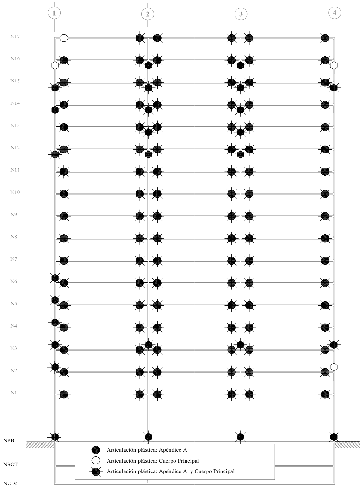
Fig 5.44.- Comparación de distribuciones de articulaciones plásticas, análisis estático no-lineal (Push-over) con resistencias nominales, edificio de 17 niveles, casos A (Cuerpo Principal) y B (Apéndice A)
