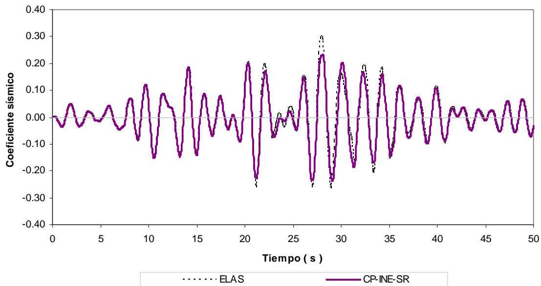
Fig 4.14.- Historias de coeficientes sísmicos, edificio 9 niveles, caso A (Cuerpo Principal) con sobre-resistencias
