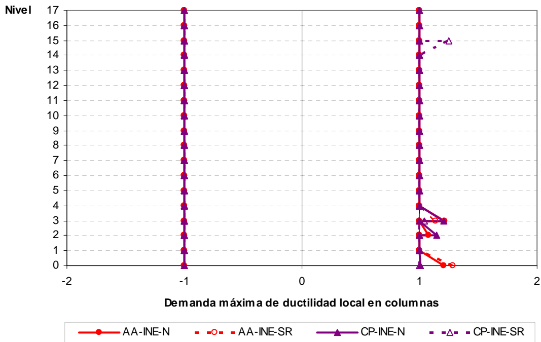
Fig 5.31.- Comparación de demandas máximas de ductilidad local en columnas, análisis paso a paso inelástico (resistencias nominales y sobre-resistencias), edificio de 17 niveles, casos A (Cuerpo Principal) y B (Apéndice A)
