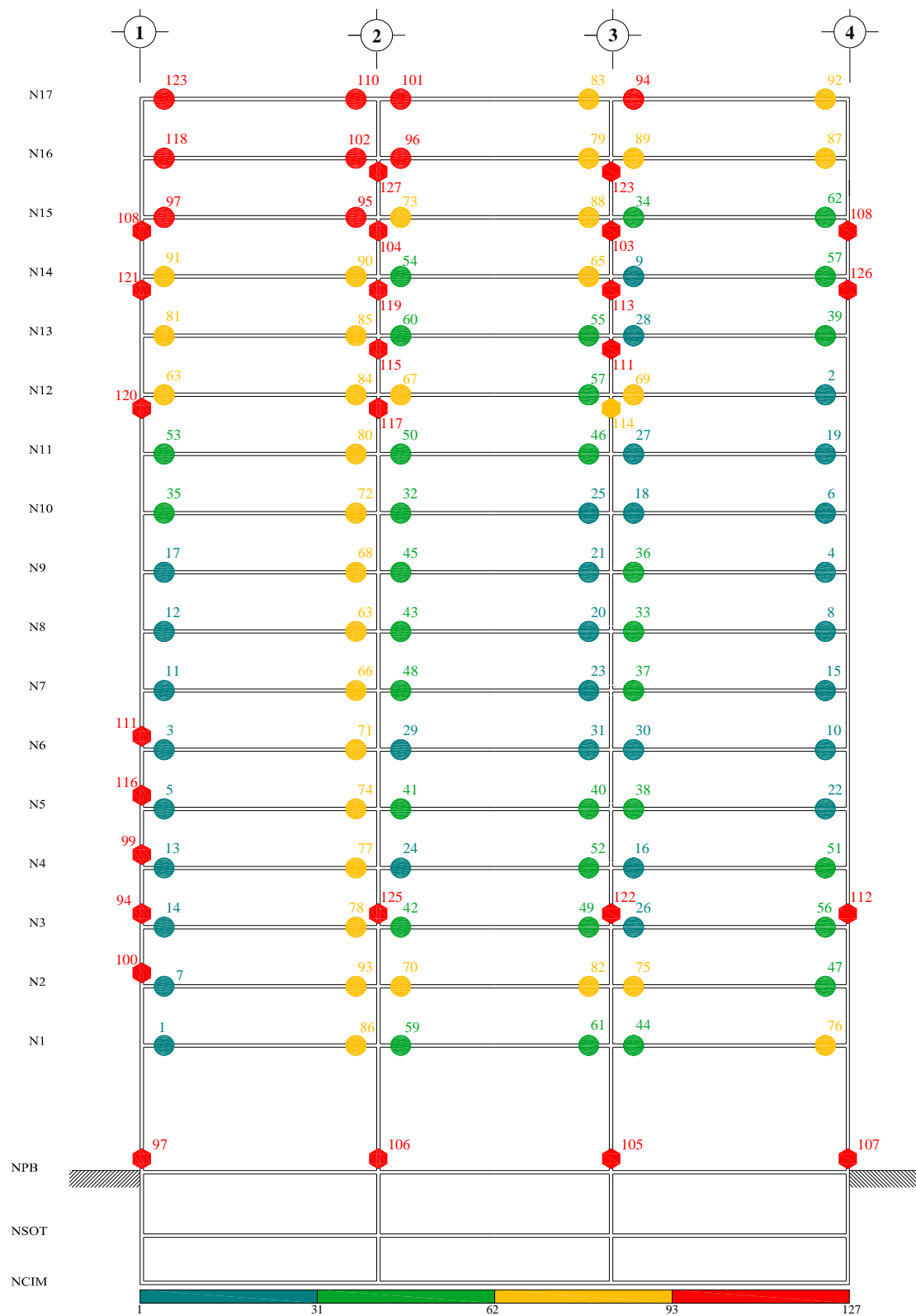
Fig A.29.- Secuencia de formación de articulaciones plásticas, análisis estático no-lineal (Push-over) con distribución de cargas laterales lineal triangular, resistencias nominales, edificio 17 niveles, caso B (Apéndice A)
