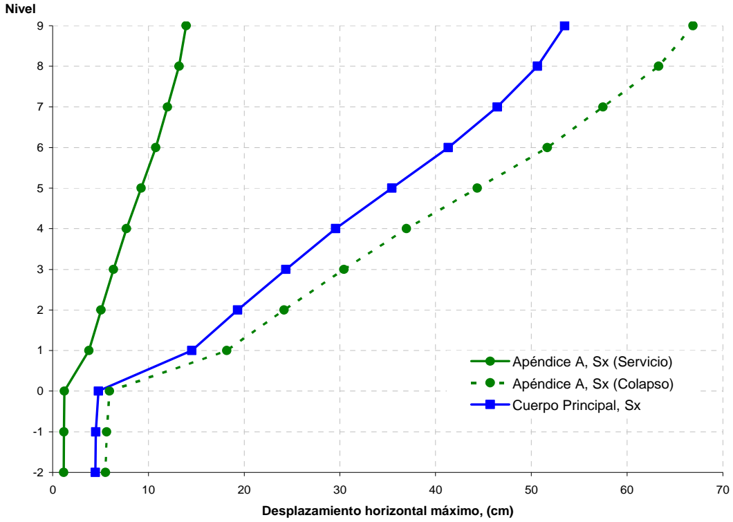
Fig 3.5.- Desplazamientos horizontales máximos, sismo en dirección "X", edificio 9 niveles, Apéndice A y Cuerpo Principal de las NTC-Sismo, RDF-04
