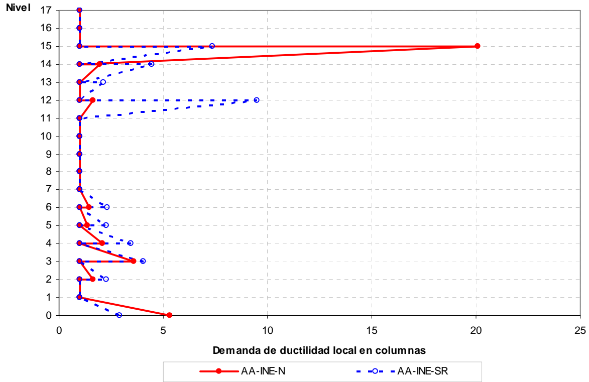
Fig 4.130.- Demandas máximas de ductilidade local en columnas, edificio 17 niveles, caso B (Apéndice A) con resistencias nominales y sobre-resistencias, distribución de fuerzas laterales del análisis dinámico modal espectral
