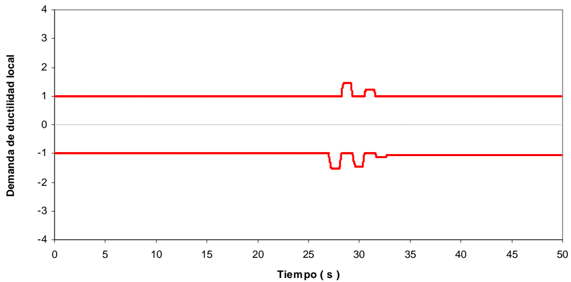
Fig 4.90.- Historias de demandas de ductilidad en el extremo izquierdo de la viga 1, edificio 17 niveles, caso B (Apéndice A) con sobre-resistencia
