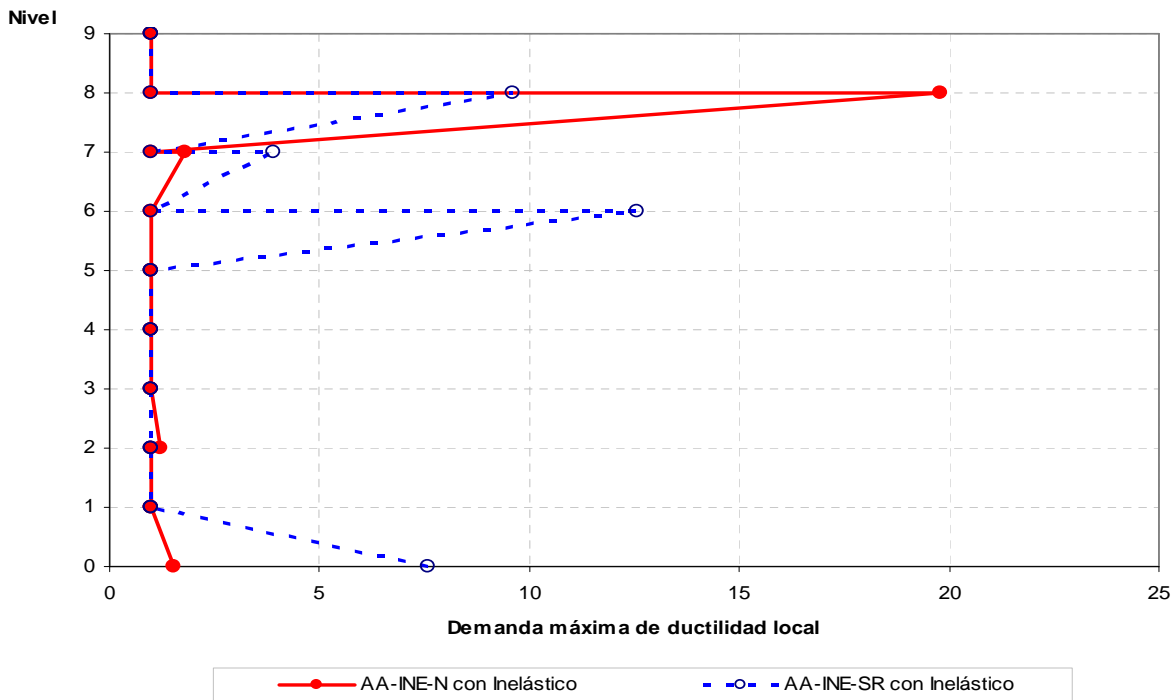
Fig 4.114.- Demandas máximas de ductilidad local en columnas, edificio 9 niveles, caso B (Apéndice A) con resistencias nominales y sobre-resistencias, distribución de fuerzas laterales del análisis paso a paso inelástico para \Delta_{m\acute{a}x}
