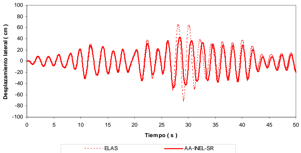
Fig 4.56.- Historia de desplazamientos de azotea, edificio 17 niveles, caso B (Apéndice A) con sobre-resistencia
