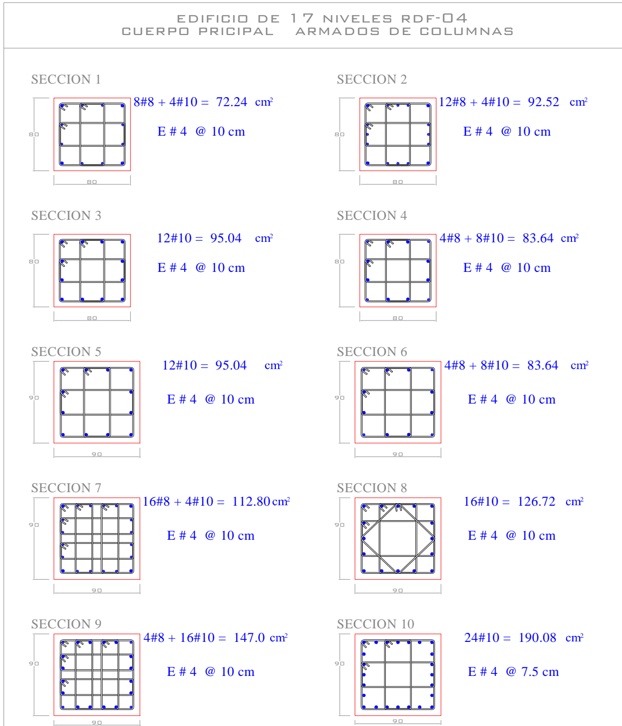
Fig 3.33a.- Armados de acero longitudinal y transversal propuestos en columnas, edificio 17 niveles, Cuerpo Principal (caso A) de las NTC-Sismo, RDF-04
