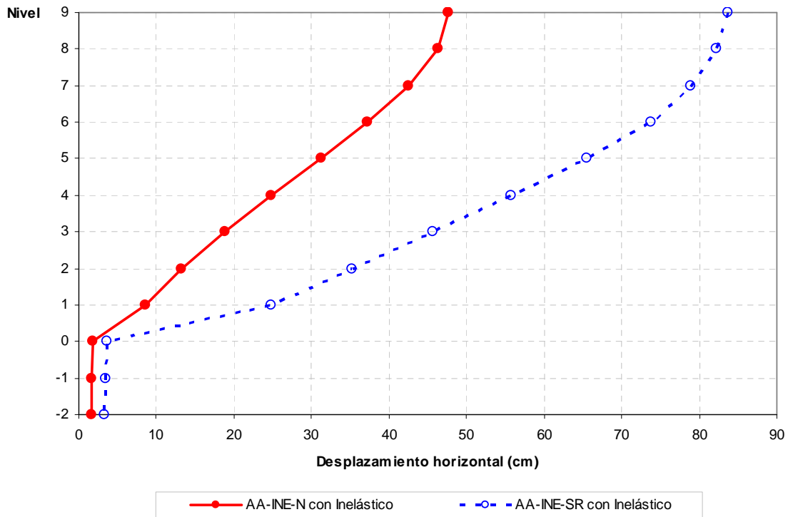
Fig 4.104.- Desplazamientos horizontales máximos, edificio 9 niveles, caso B con resistencias nominales y sobre-resistencias, distribución de cargas del análisis paso a paso inelástico para \Delta_{máx}
