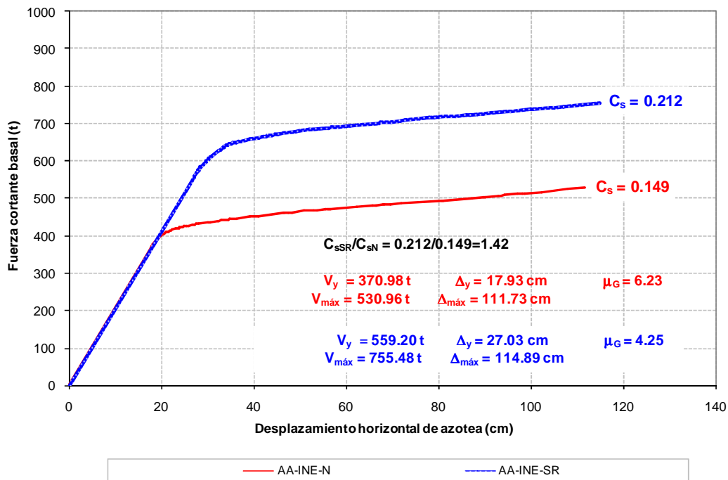
Fig 4.118.- Curvas de fuerza cortante basal-desplazamiento lateral de azotea, edificio 17 niveles, caso B (Apéndice A) con resistencias nominales y sobre-resistencias, distribución de fuerzas laterales del análisis dinámico modal espectral
