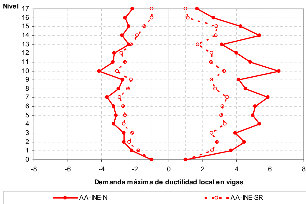
Fig 4.98.- Demandas máximas de ductilidad local en vigas, edificio 17 niveles, caso B (Apéndice A) con resistencias nominales y con sobre-resistencias
