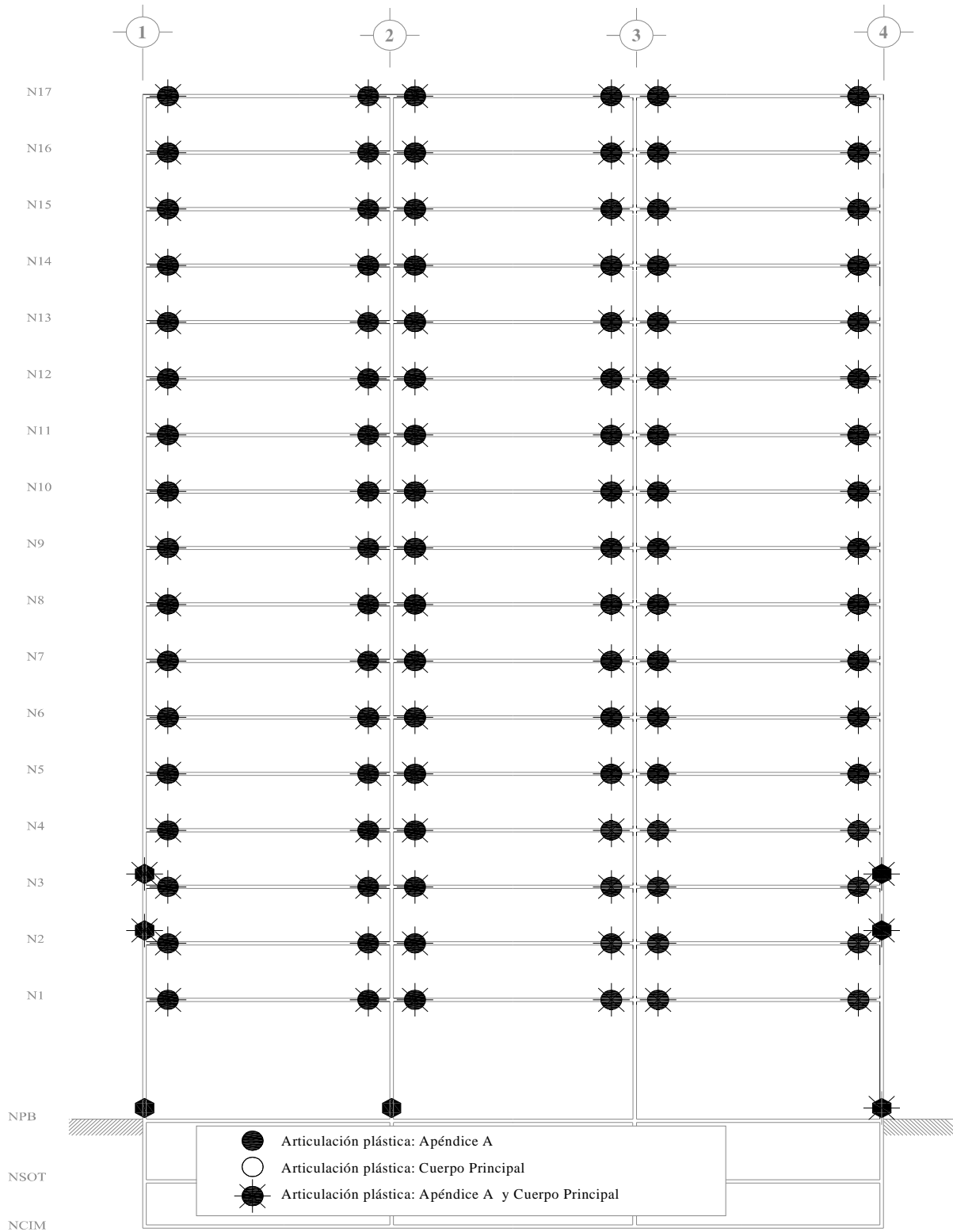
Fig 5.26.- Comparación de distribuciones de articulaciones plásticas, análisis paso a paso inelástico (resistencias nominales), edificio de 17 niveles, casos A (Cuerpo Principal) y B (Apéndice A)
