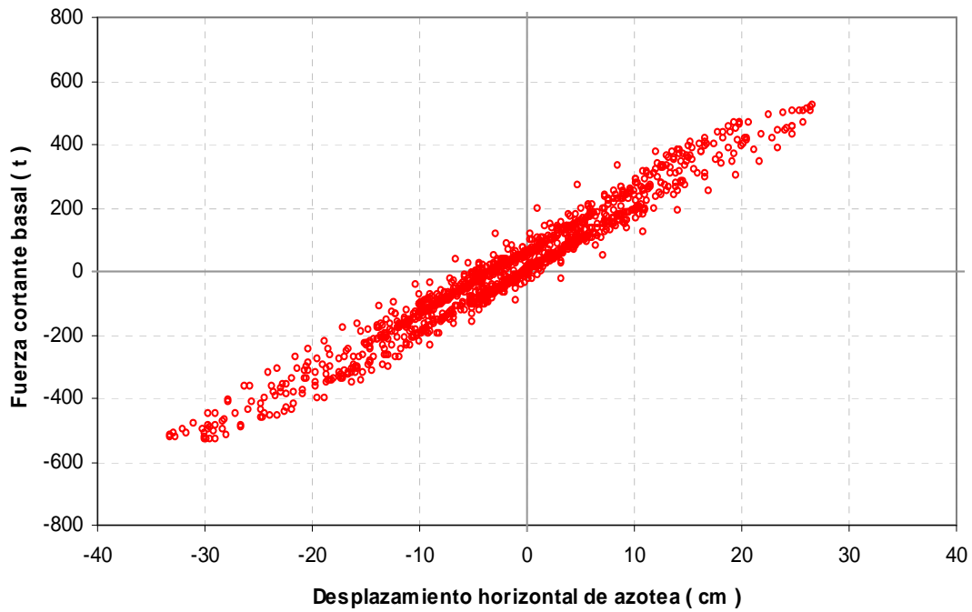
Fig 4.21.- Relaciones fuerza cortante basal – desplazamiento lateral de azotea, edificio 9 niveles, caso B (Apéndice A), comportamiento inelástico con sobre-resistencias
