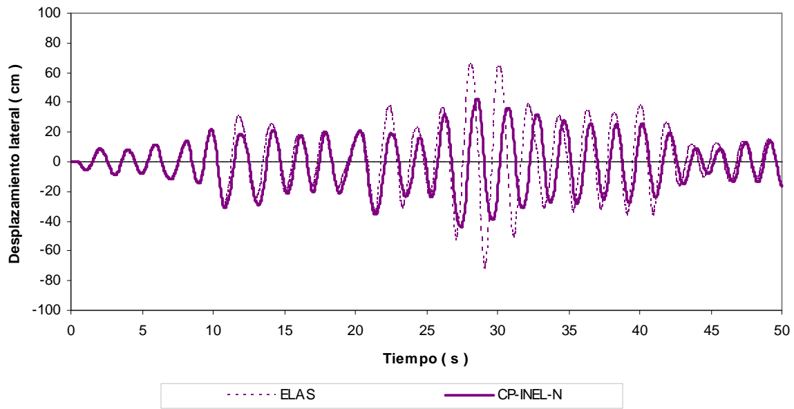
Fig 4.53.- Historia de desplazamientos de azotea, edificio 17 niveles, caso A (Cuerpo Principal) con resistencias nominales
