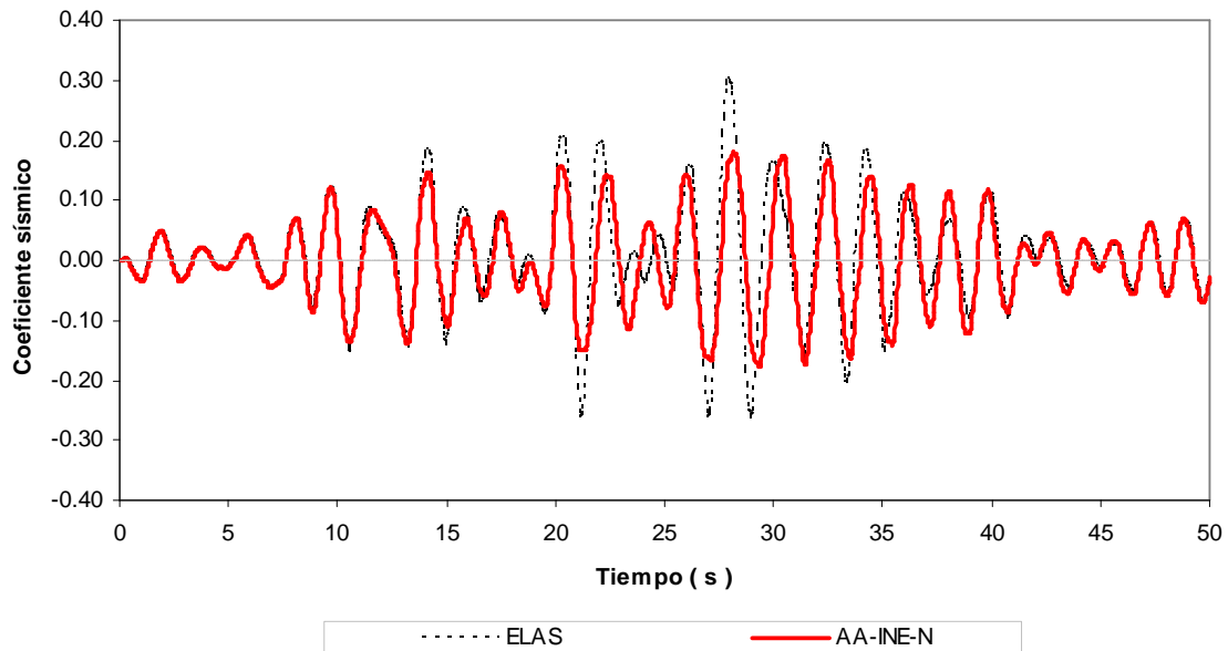
Fig 4.15.- Historias de coeficientes sísmicos, edificio 9 niveles, caso B (Apéndice A) con resistencias nominales
