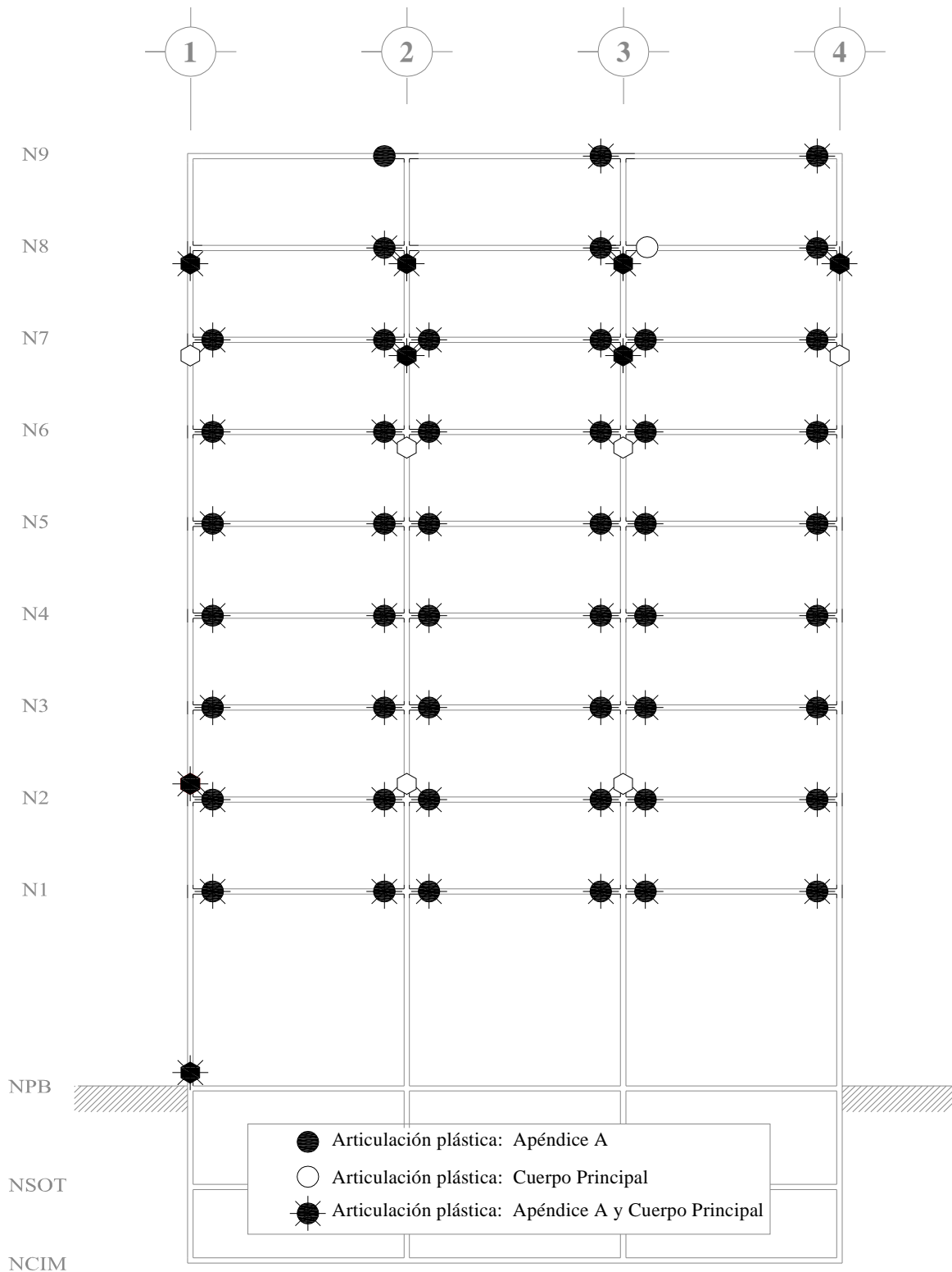
Fig 5.42.- Comparación de distribuciones de articulaciones plásticas, análisis estático no-lineal (Push-over) con resistencias nominales, edificio de 9 niveles, casos A (Cuerpo Principal) y B (Apéndice A)
