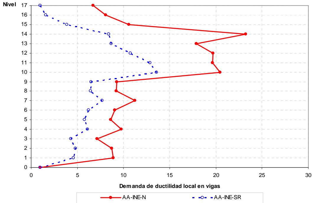
Fig 4.128.- Demandas máximas de ductilidad local en vigas, edificio 17 niveles, caso B (Apéndice A) con resistencias nominales y sobre-resistencias, distribución de fuerzas laterales del análisis dinámico modal espectral
