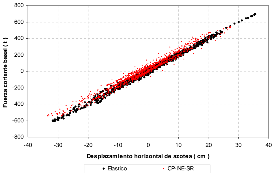
Fig 5.17.- Comparación de relaciones fuerza cortante basal-desplazamiento horizontal de azotea, análisis paso a paso elástico e inelástico (sobre-resistencias), edificio de 9 niveles, caso A (Cuerpo Principal)
