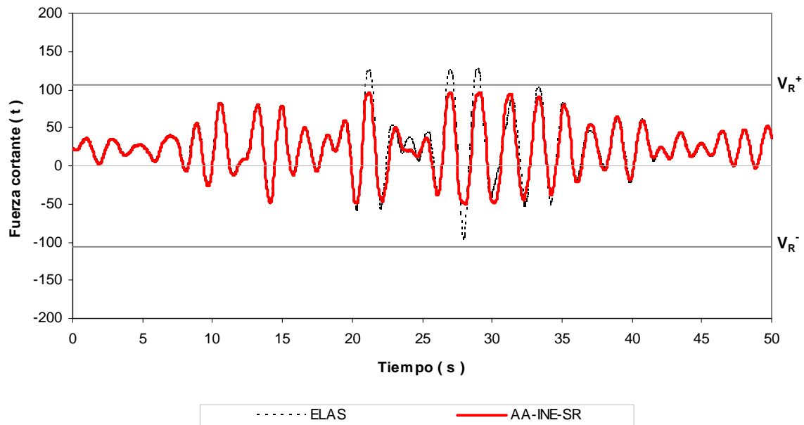
Fig 4.38.- Historias de fuerzas cortantes en el extremo izquierdo de la viga 1, edificio 9 niveles, caso B (Apéndice A) con sobre-resistencias
