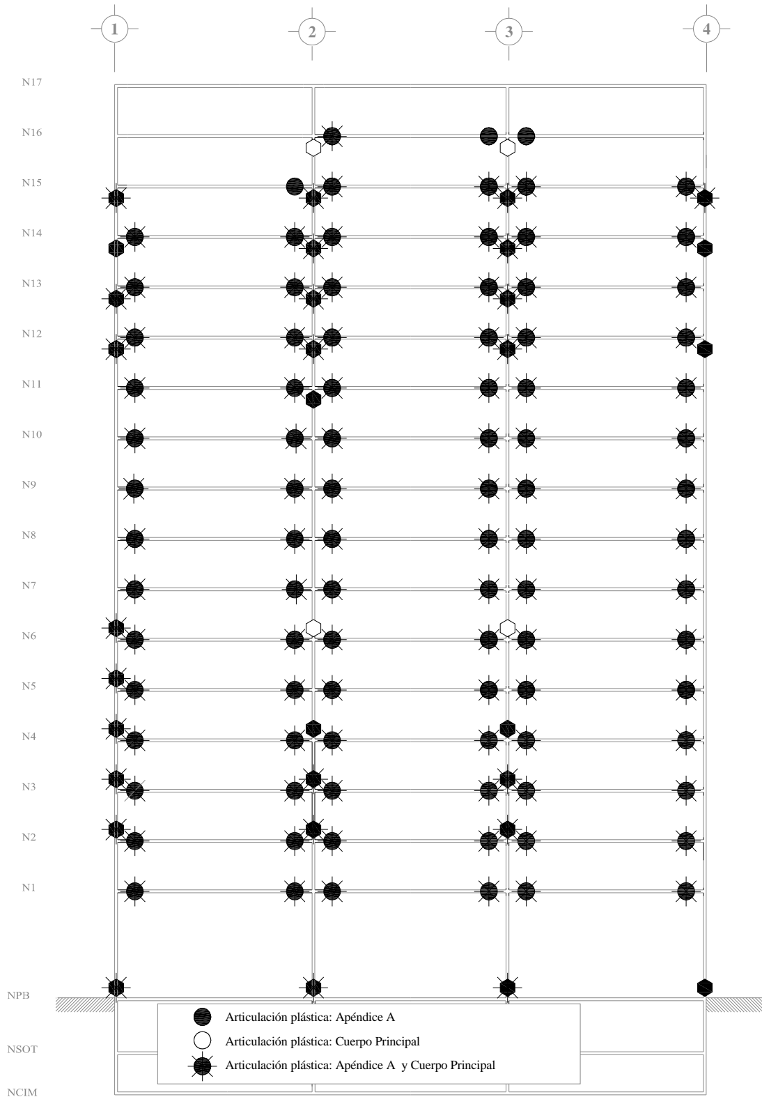
Fig 5.45.- Comparación de distribuciones de articulaciones plásticas, análisis estático no-lineal (Push-over) con sobre-resistencias, edificio de 17 niveles, casos A (Cuerpo Principal) y B (Apéndice A)
