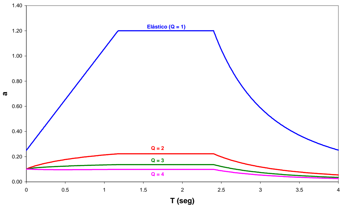
Fig 2.13.- Espectros inelásticos de diseño del Apéndice A ( T_s = 2 s) de las NTC-Sismo del RDF-04
