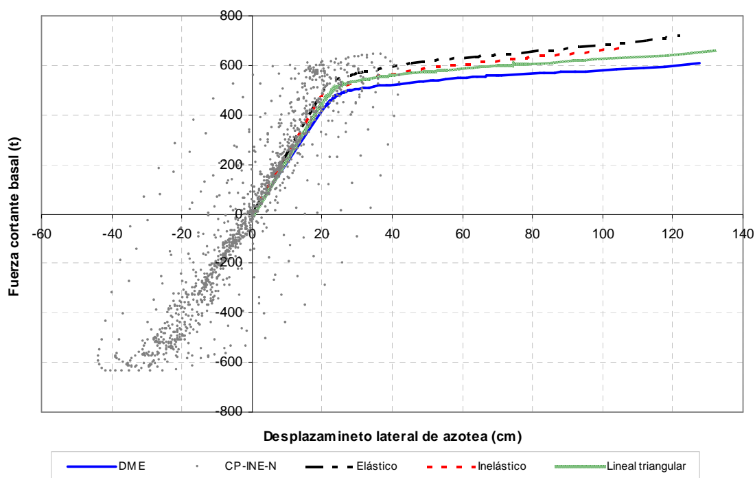
Fig A.5.- Relaciones fuerza cortante basal – desplazamiento lateral de azotea, análisis paso a paso y Push-over con diferentes distribuciones de cargas laterales, resistencias nominales, edificio 17 niveles, caso A (Cuerpo Principal)
