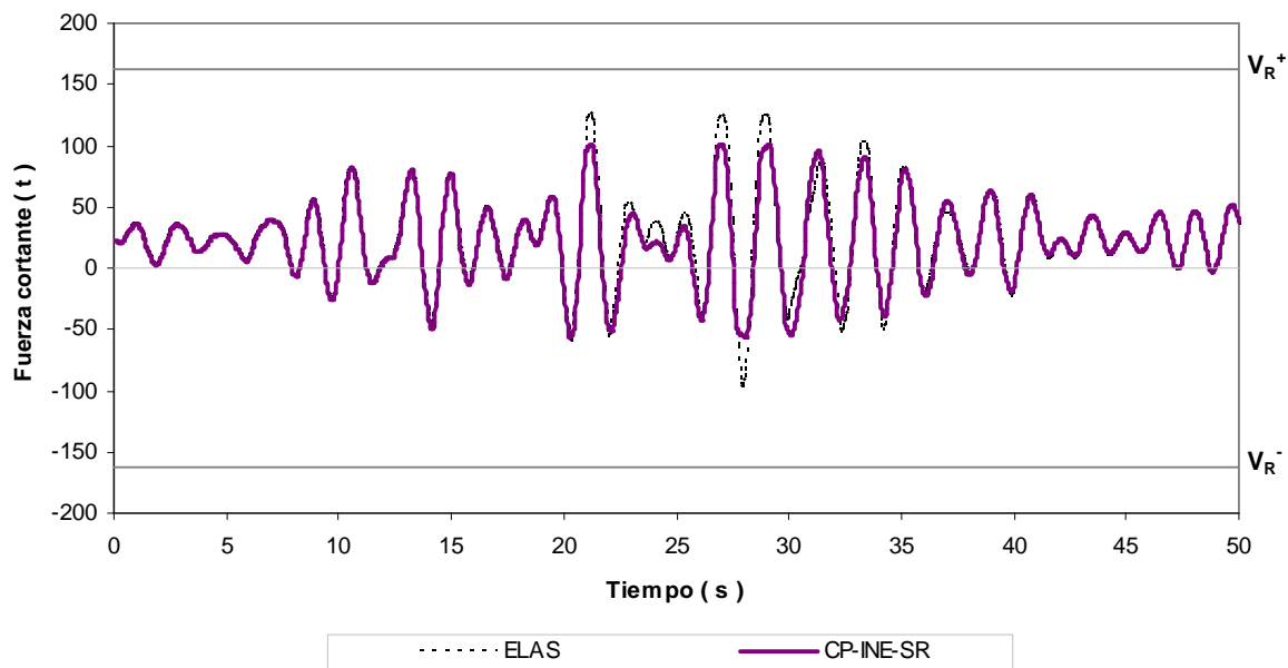
Fig 4.36.- Historias de fuerzas cortantes en el extremo izquierdo de la viga 1, edificio 9 niveles, caso A (Cuerpo Principal) con sobre-resistencias
