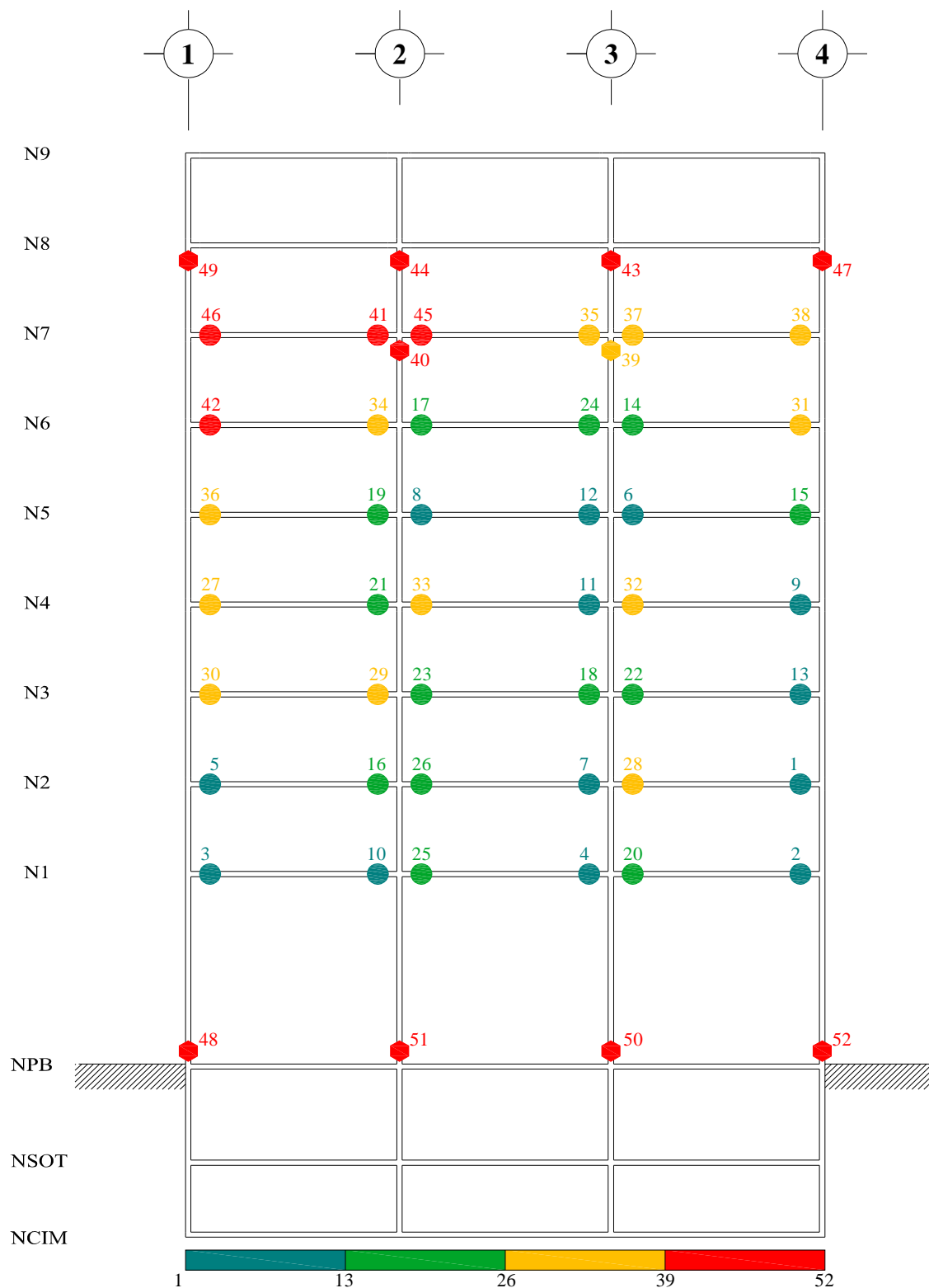
Fig A.18.- Secuencia de formación de articulaciones plásticas, análisis estático no-lineal (Push-over) con distribución de cargas de análisis dinámico modal espectral (DME), sobre-resistencias, edificio 9 niveles, caso B (Apéndice A)
