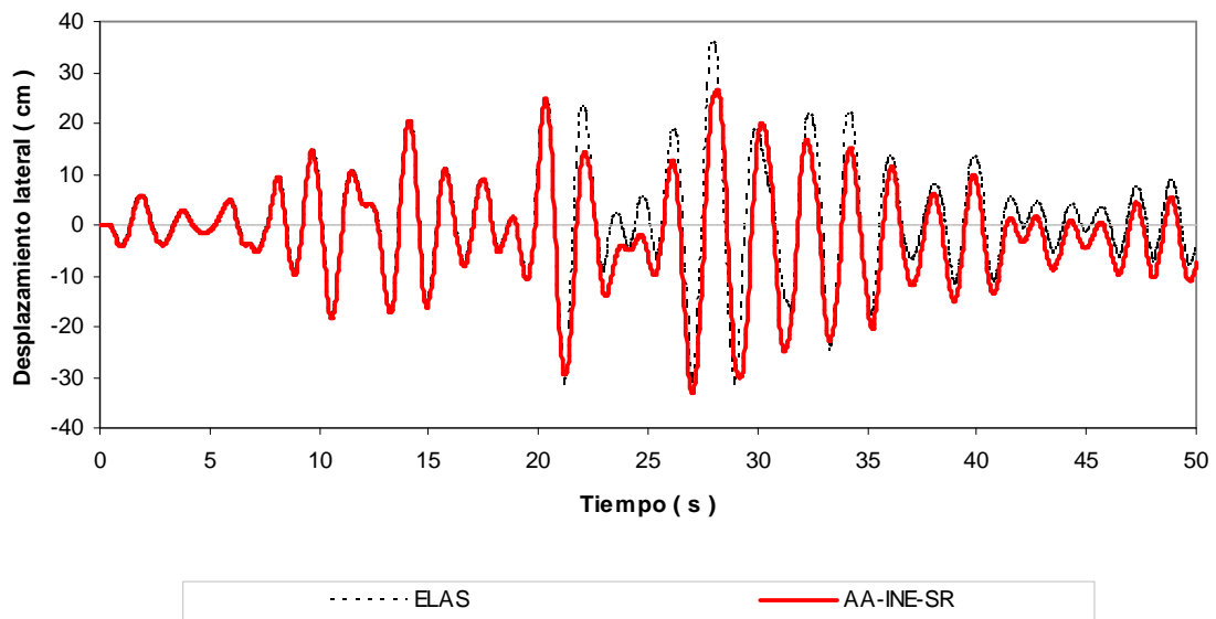
Fig 4.8.- Historia de desplazamientos de azotea, edificio 9 niveles, caso B (Apéndice A) con sobre-resistencias
