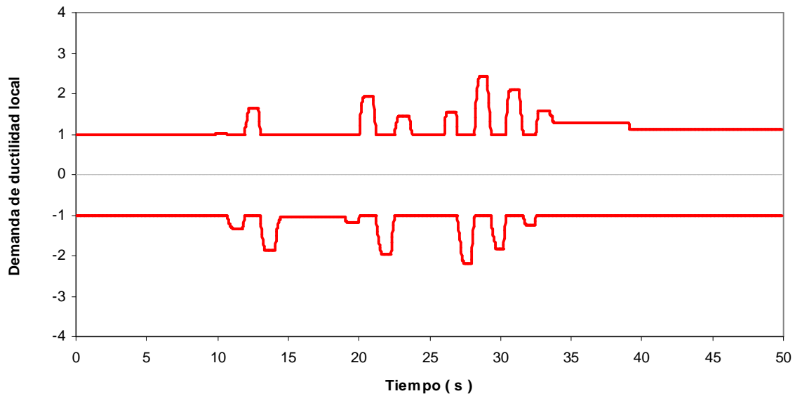
Fig 4.89.- Historias de demandas de ductilidad en el extremo izquierdo de la viga 1, edificio 17 niveles, caso B (Apéndice A) con resistencias nominales
