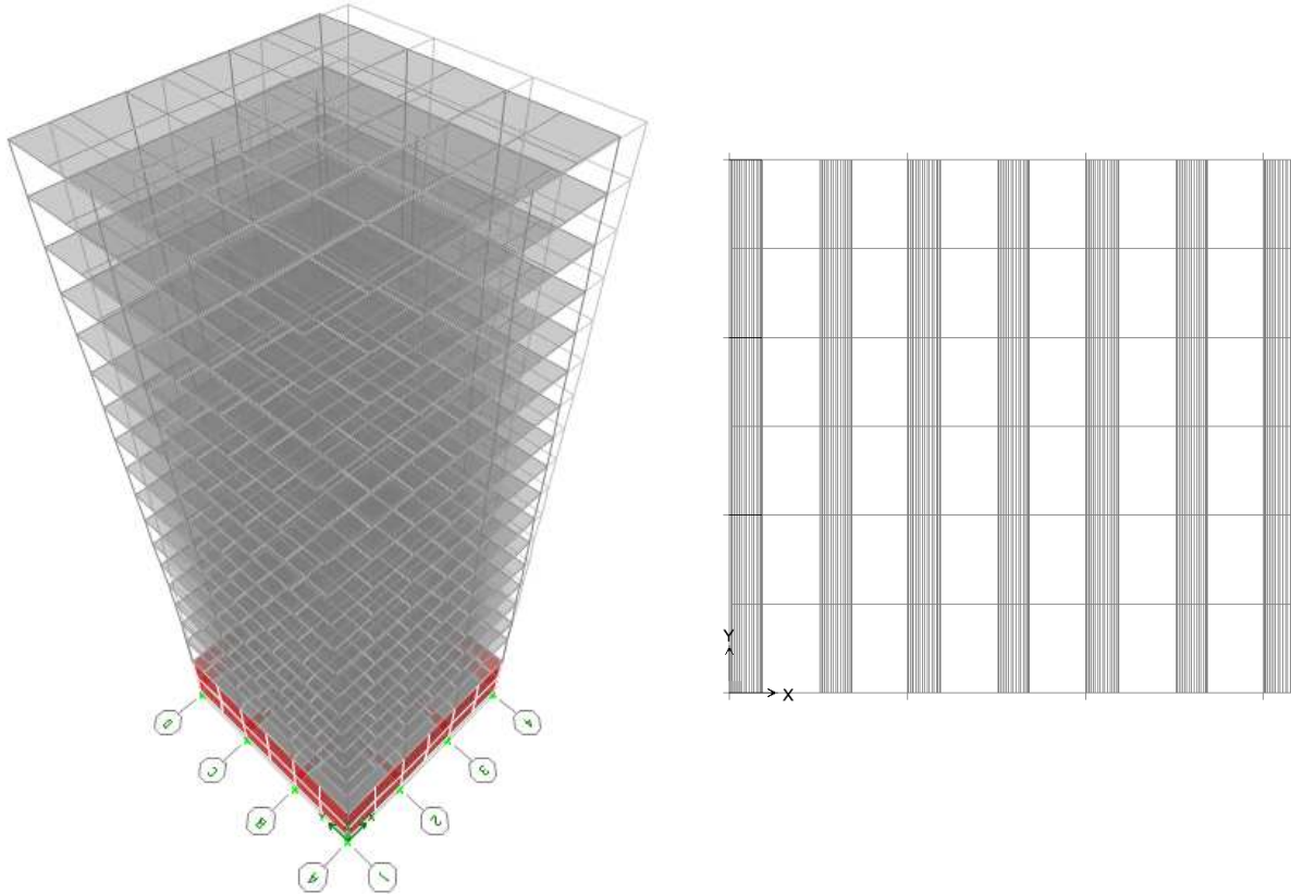
Fig 3.22a.- Vista en elevación y planta de la deformada del primer modo de vibrar del edificio de 17 niveles
