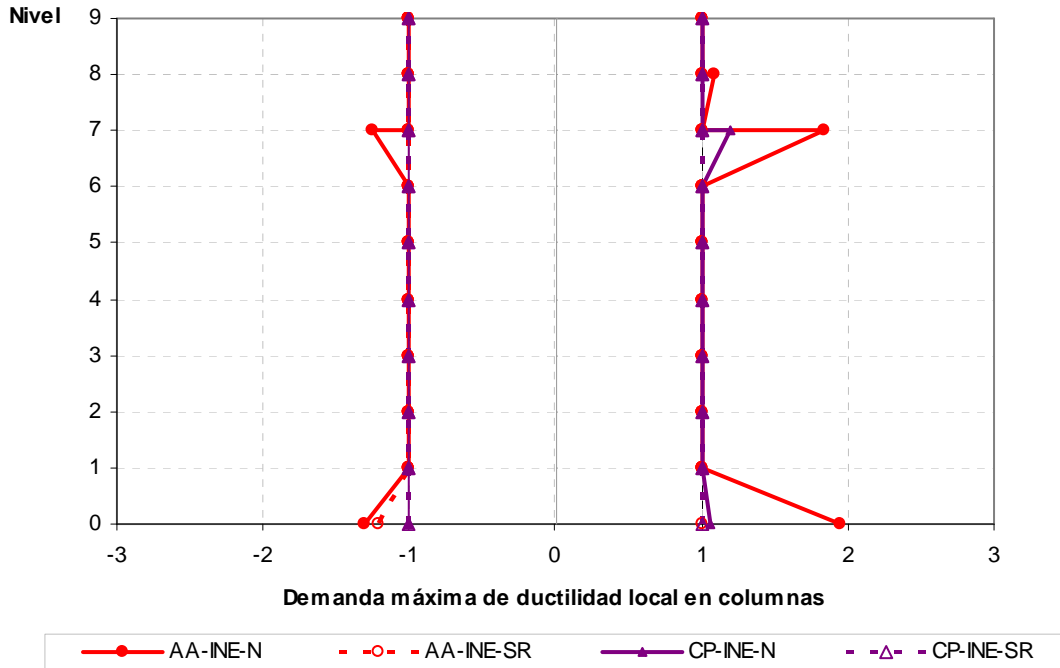
Fig 5.30.- Comparación de demandas máximas de ductilidad local en columnas, análisis paso a paso inelástico (resistencias nominales y sobre-resistencias), edificio de 9 niveles, casos A (Cuerpo Principal) y B (Apéndice A)
