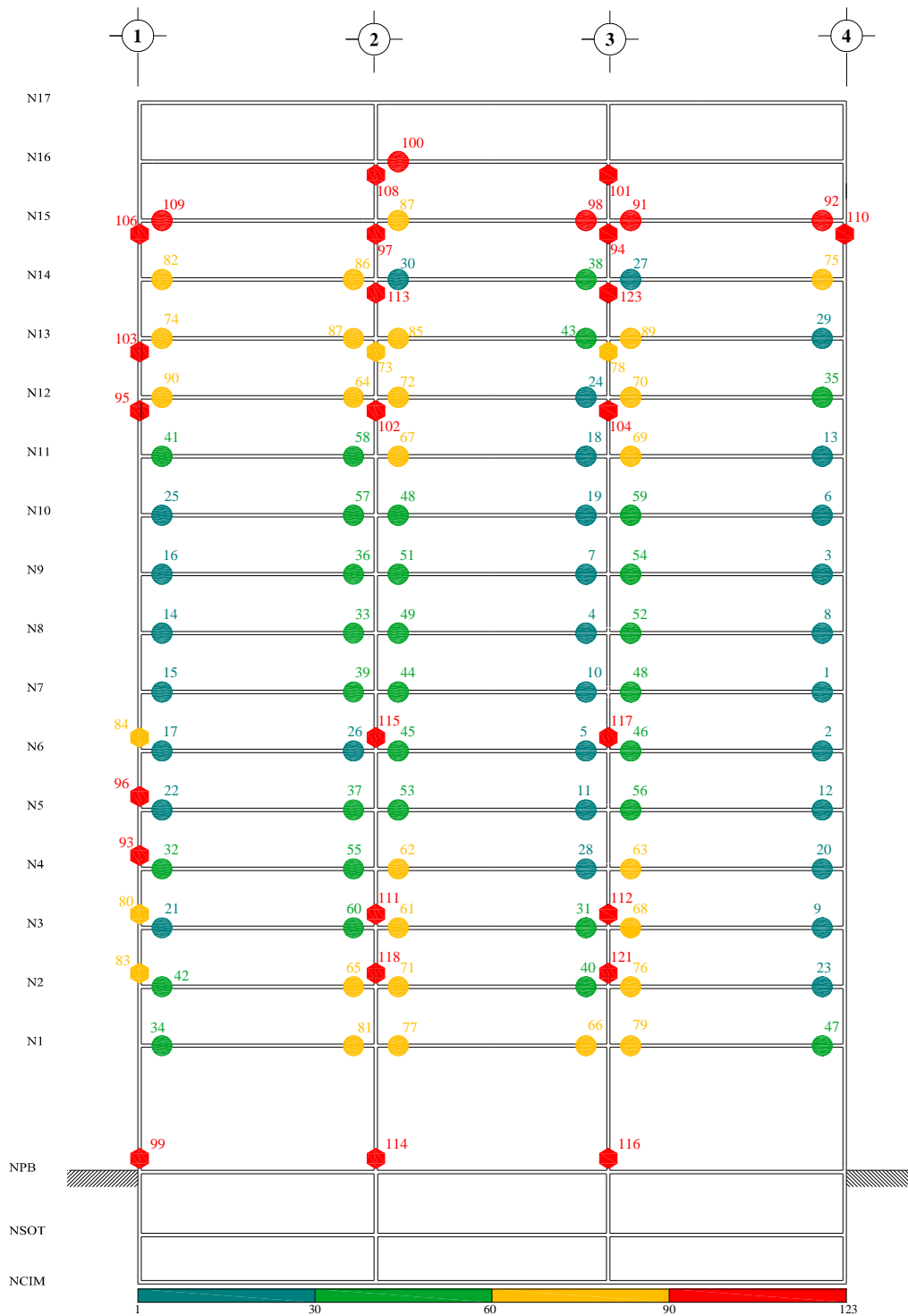
Fig 4.124.- Mecanismo de falla y secuencia de formación de articulaciones plásticas, edificio 17 niveles, caso A (Cuerpo Principal) con sobre-resistencias, distribución de fuerzas laterales del análisis dinámico modal espectral
