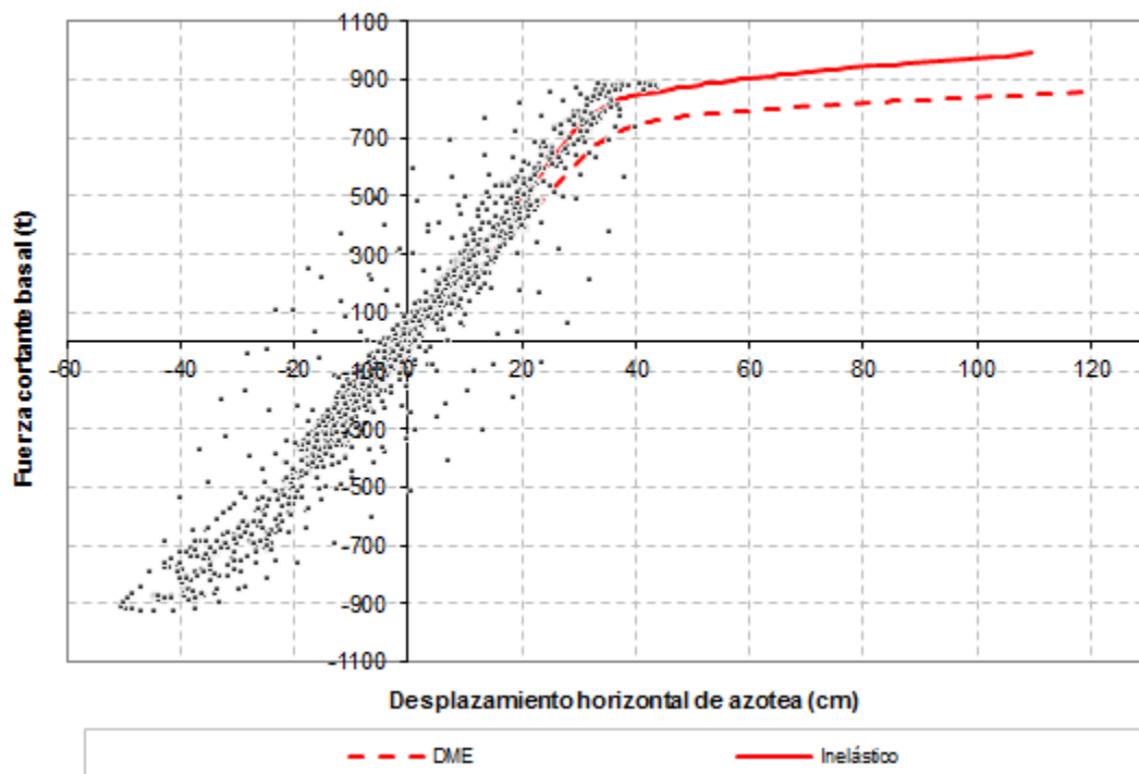
Fig 5.39.- Comparación de relaciones fuerza cortante basal-desplazamiento horizontal de azotea, análisis estático no-lineal (Push-over) y análisis paso a paso inelástico con sobre-resistencias, edificio de 17 niveles, caso A (Cuerpo Principal)
