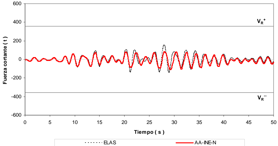
Fig 4.29.- Historias de fuerzas cortantes en el extremo inferior de la columna 1, edificio 9 niveles, caso B (Apéndice A) con resistencias nominales
