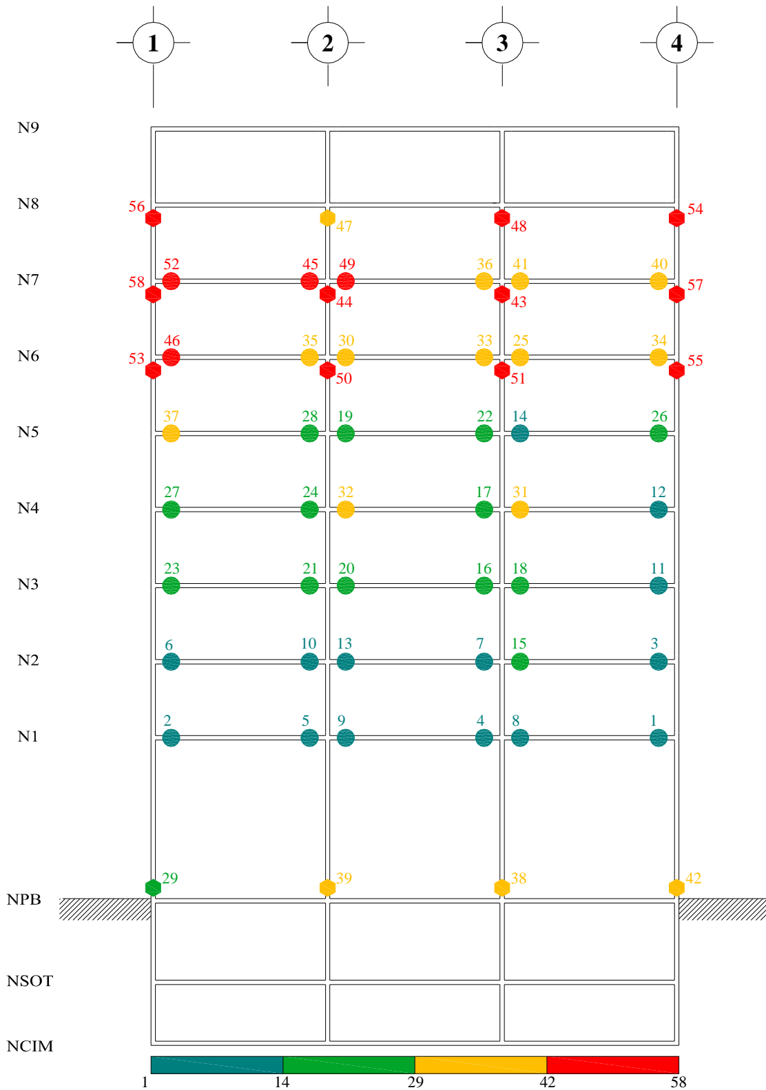
Fig 4.110.- Mecanismo de falla y secuencia de formación de articulaciones plásticas, edificio 9 niveles, caso B (Apéndice A) con sobre-resistencias, distribución de fuerzas laterales del análisis paso a paso inelástico para \Delta_{máx}
