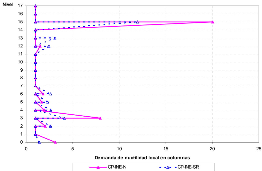
Fig 4.129.- Demandas máximas de ductilidad local en columnas, edificio 17 niveles, caso A (Cuerpo Principal) con resistencias nominales y sobre-resistencias, distribución de fuerzas laterales del análisis dinámico modal espectral
