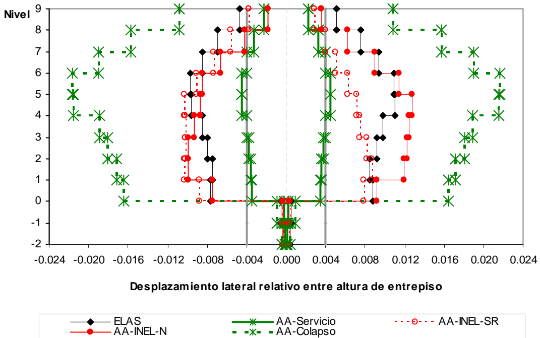
Fig 4.10.- Relaciones desplazamiento lateral relativo entre altura de entrepiso, edificio 9 niveles, caso B (Apéndice A)
