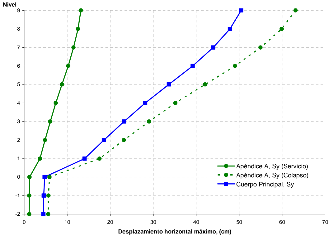
Fig 3.6.- Desplazamientos horizontales máximos, sismo en dirección "Y", edificio 9 niveles, Apéndice A y Cuerpo Principal de las NTC-Sismo, RDF-04
