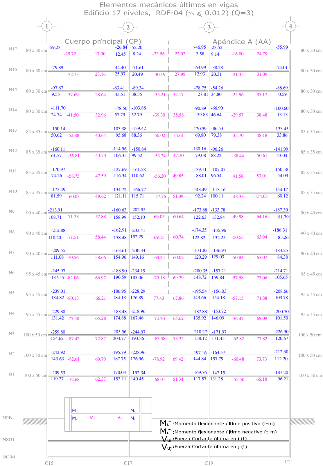
Fig 3.26.- Elementos mecánicos últimos de las vigas del eje B, edificio 17 niveles, Apéndice A y Cuerpo Principal de las NTC-Sismo, RDF-04
