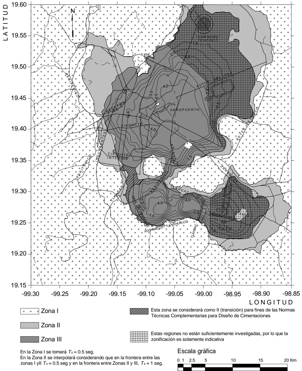
Fig 2.10.- Curvas de iguales periodos predominantes del movimiento del suelo, T_s , según las NTC-Sismo del RDF-04
