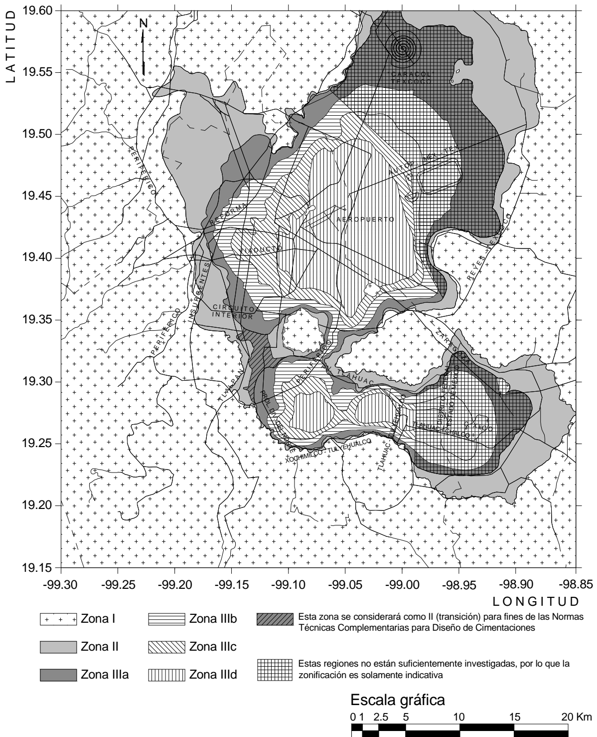
Fig 2.9.- Zonificación de la ciudad de México según las NTC-Sismo del RDF-04
