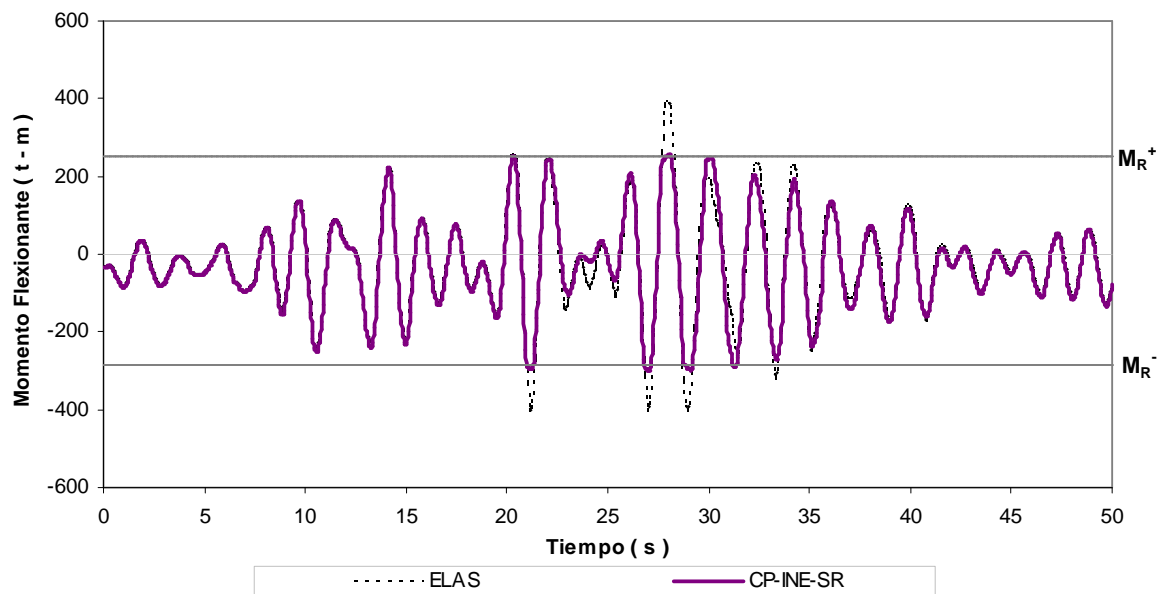
Fig 4.32.- Historias de momentos flexionantes en el extremo izquierdo de la viga 1, edificio 9 niveles, caso A (Cuerpo Principal) con sobre-resistencias
