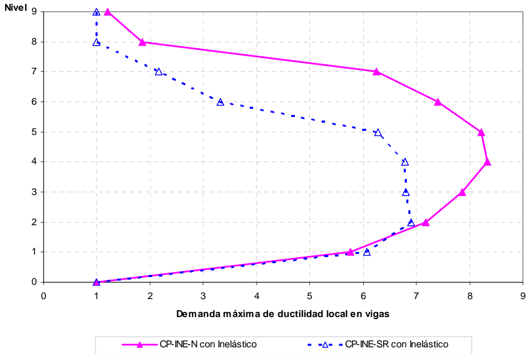
Fig 4.111.- Demandas máximas de ductilidad local en vigas, edificio 9 niveles, caso A (Cuerpo Principal) con resistencias nominales y sobre-resistencias, distribución de fuerzas laterales del análisis paso a paso inelástico para \Delta_{máx}
