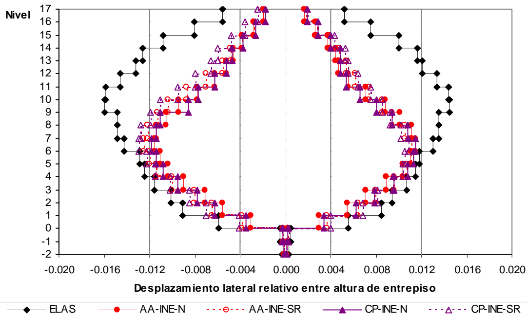
Fig 5.11.- Comparación de relaciones máximas de desplazamiento horizontal relativo entre altura de entrepiso, análisis paso a paso elástico e inelástico (resistencias nominales y sobre-resistencias), edificio de 17 niveles, casos A (Cuerpo Principal) y B (Apéndice A)
