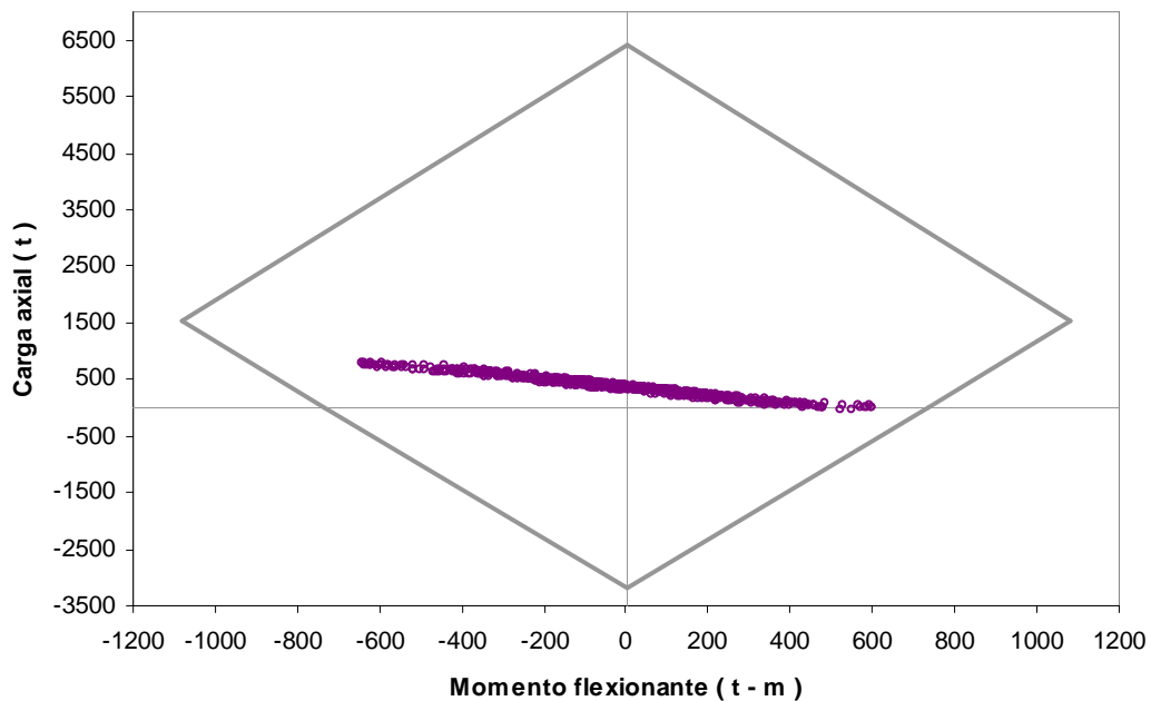
Fig 4.24.- Combinaciones momento flexionante-carga axial del extremo inferior de la columna 1, edificio 9 niveles, caso A (Cuerpo principal) con sobre-resistencias
