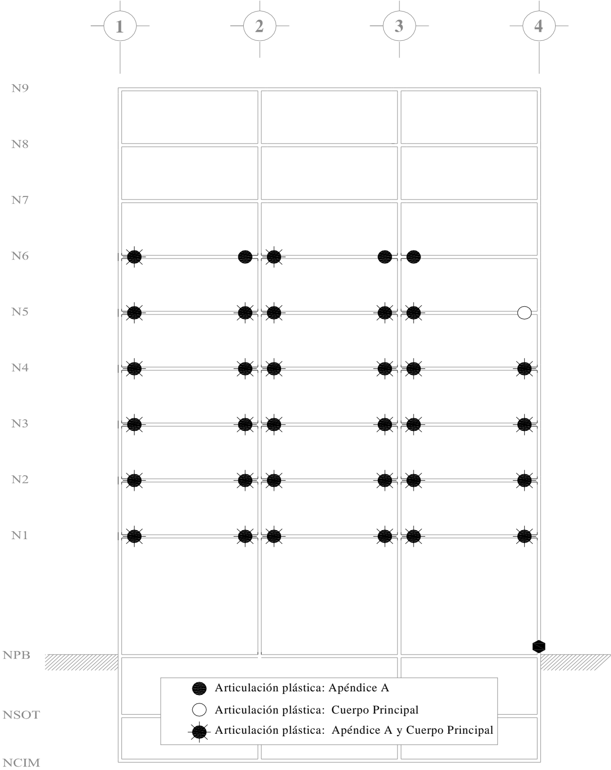
Fig 5.25.- Comparación de distribuciones de articulaciones plásticas, análisis paso a paso inelástico (sobre-resistencias), edificio de 9 niveles, casos A (Cuerpo Principal) y B (Apéndice A)
