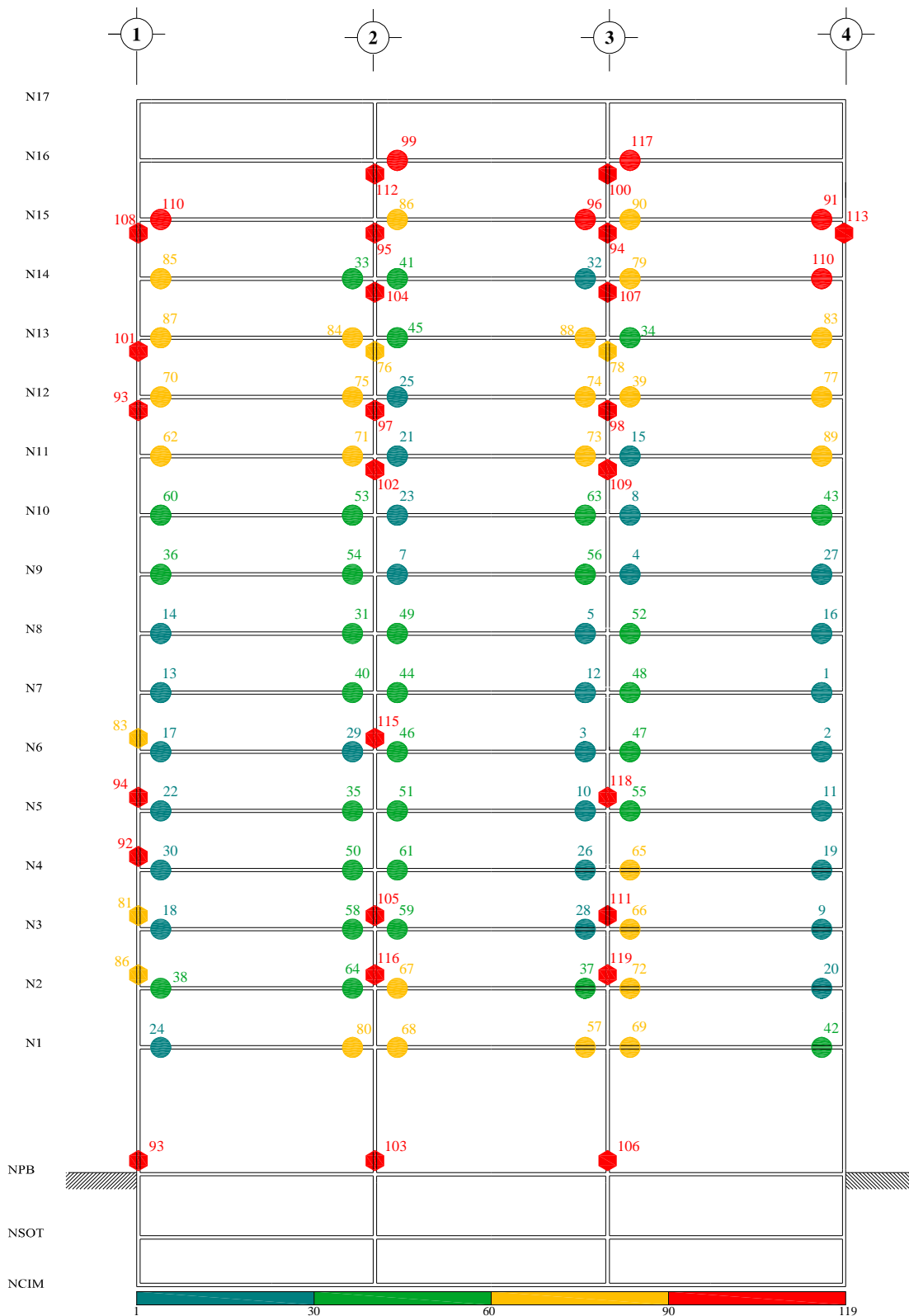
Fig A.26.- Secuencia de formación de articulaciones plásticas, análisis estático no-lineal (Push-over) con distribución de cargas laterales lineal triangular, sobre-resistencias, edificio 17 niveles, caso A (Cuerpo Principal)
