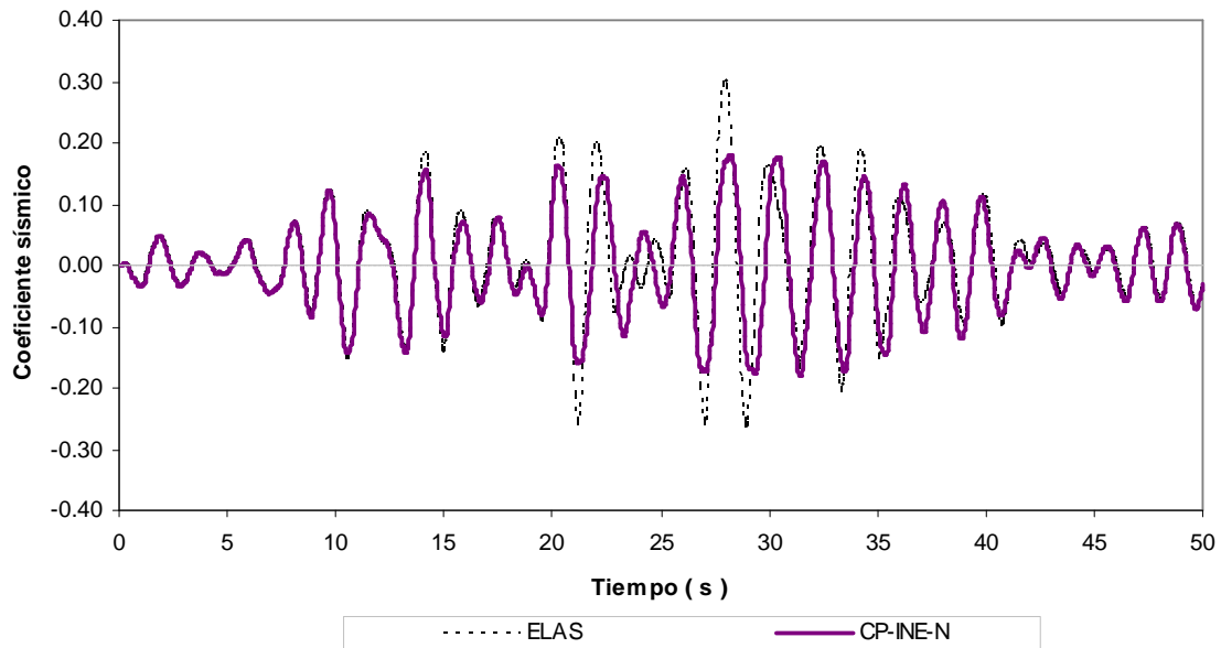
Fig 4.13.- Historias de coeficientes sísmicos, edificio 9 niveles, caso A (Cuerpo Principal) con resistencias nominales
