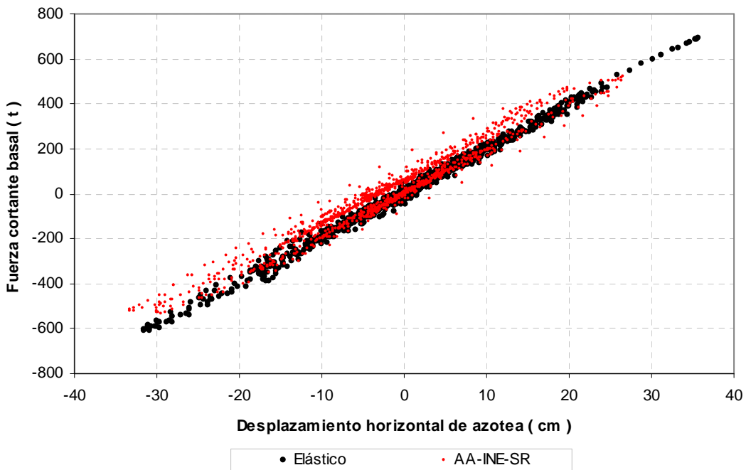
Fig 5.19.- Comparación de relaciones fuerza cortante basal-desplazamiento horizontal de azotea, análisis paso a paso elástico e inelástico (sobre-resistencias), edificio de 9 niveles, caso B (Apéndice A)
