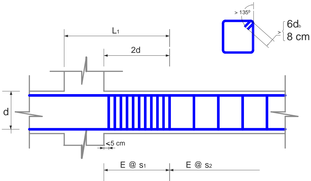
Fig 2.15.- Requisitos necesarios de acero transversal en vigas, capítulo de marcos dúctiles (Q = 3 ó 4) de las NTC-Concreto del RDF-04
