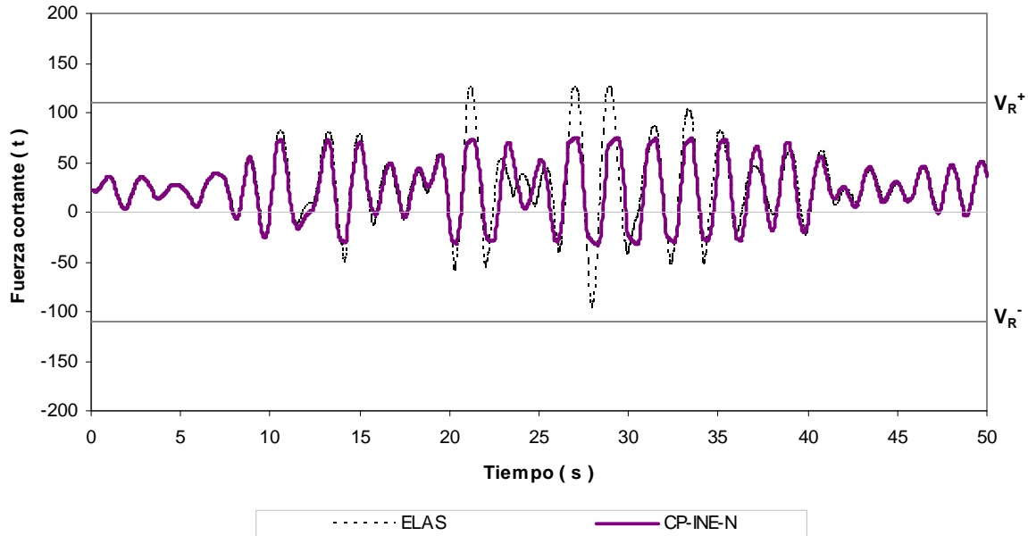
Fig 4.35.- Historias de fuerzas cortantes en el extremo izquierdo de la viga 1, edificio 9 niveles, caso A (Cuerpo Principal) con resistencias nominales
