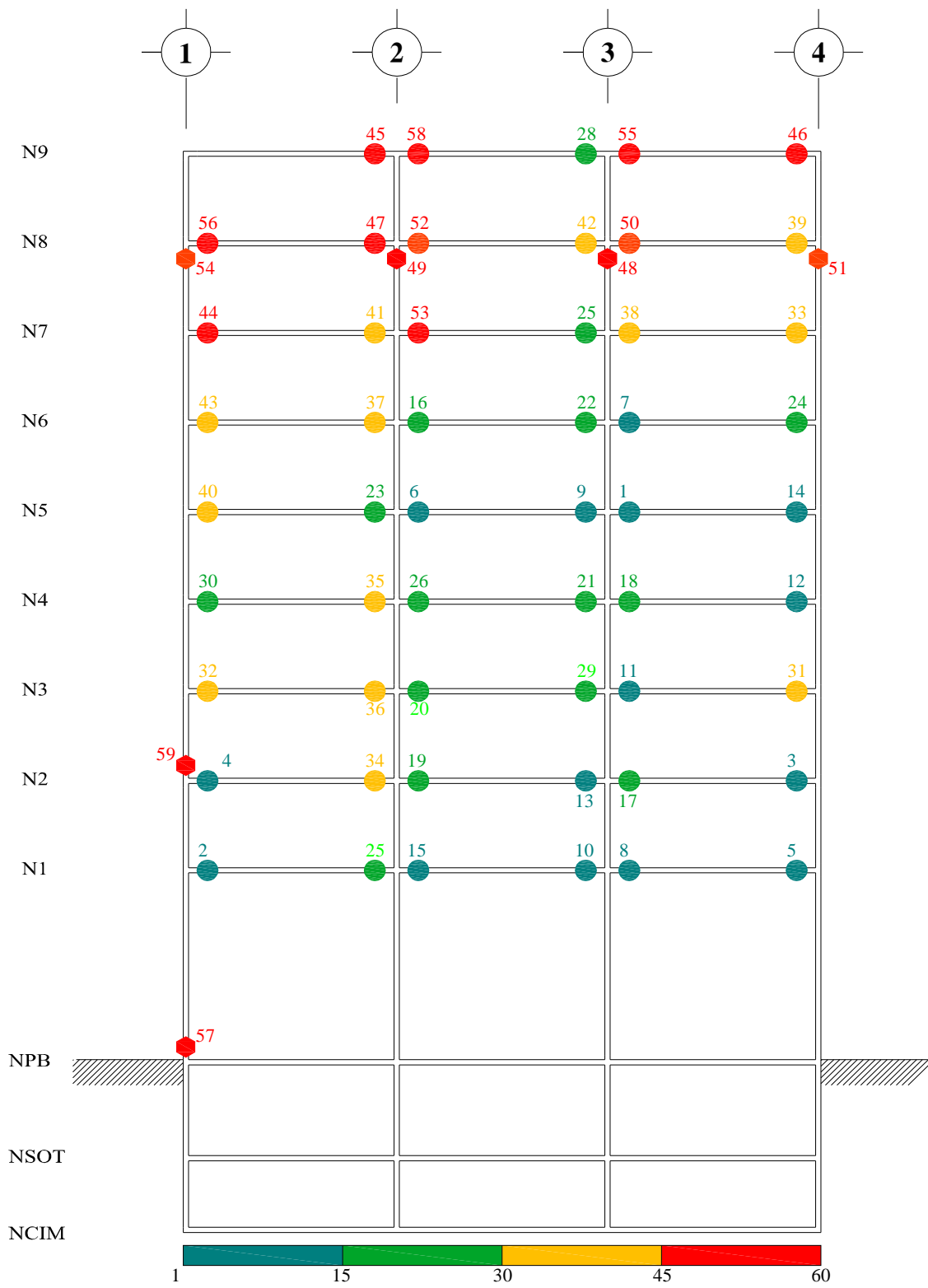
Fig A.17- Secuencia de formación de articulaciones plásticas, análisis estático no-lineal (Push-over) con distribución de cargas laterales lineal triangular, resistencias nominales, edificio 9 niveles, caso B (Apéndice A)
