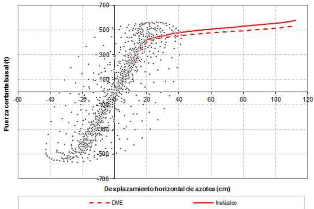
Fig 5.40.- Comparación de relaciones fuerza cortante basal-desplazamiento horizontal de azotea, análisis estático no-lineal ( Push-over ) y análisis paso a paso inelástico con resistencias nominales, edificio de 17 niveles, caso B (Apéndice A)
