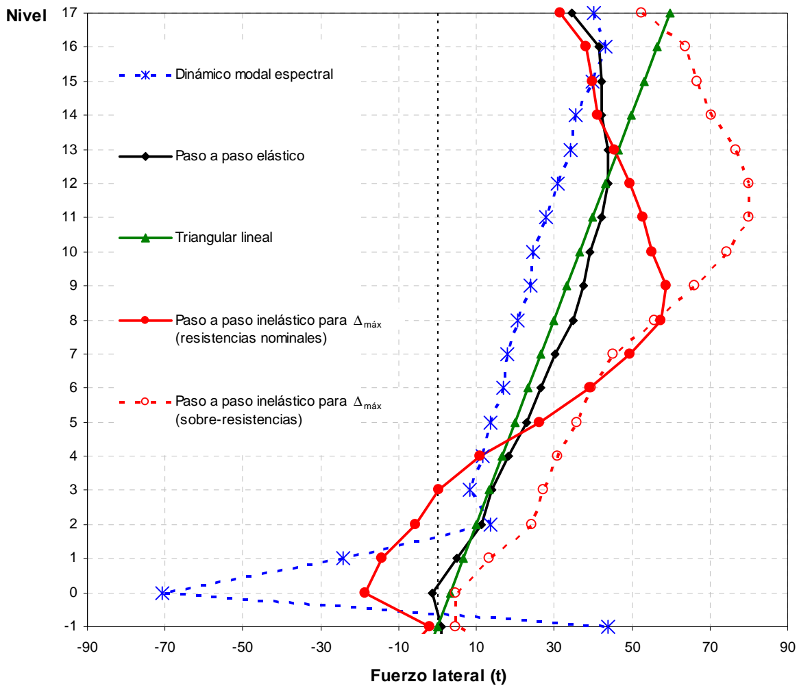
Fig 4.115.- Distribuciones de cargas laterales para el análisis estático no-lineal (Push-over), edificio 17 niveles, caso A (Cuerpo Principal)
