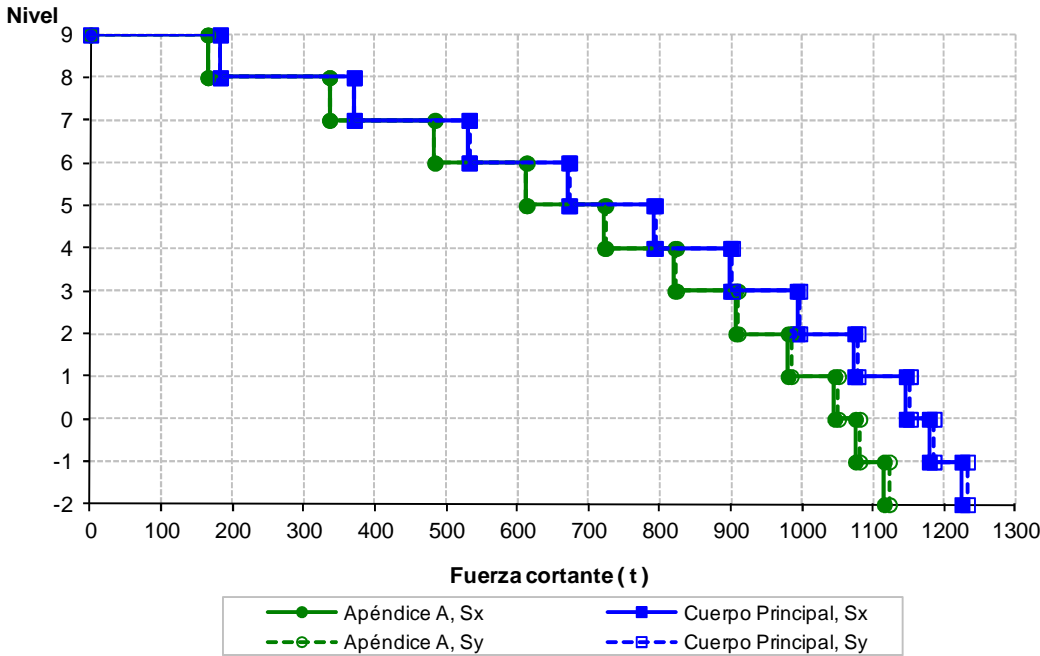
Fig 5.6.- Comparación de fuerzas cortantes de entrepiso, análisis dinámico modal espectral, sismo en ambas direcciones, edificio de 9 niveles, casos A (Cuerpo Principal) y B (Apéndice A)
