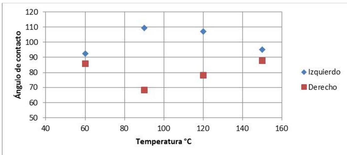
Figura 4.8 Grafica del comportamiento de los ángulos de contacto para la gota de aceite del campo Aguacate
