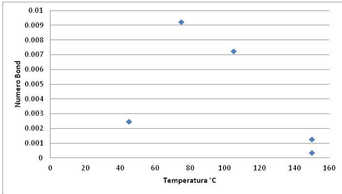
Figura 5.3 Número de bond en función de la temperatura
