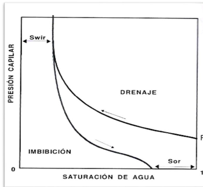
Figura 1.4 comportamiento de la Presión capilar sobre la saturación de agua
