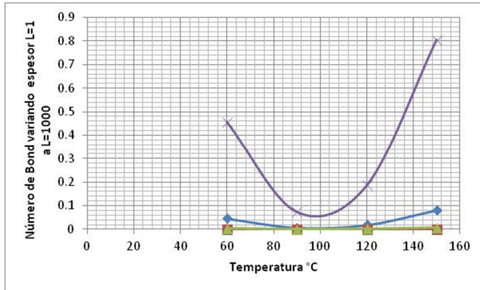
Figura 5.10 Graficando Número de Bond para diferentes espesores
