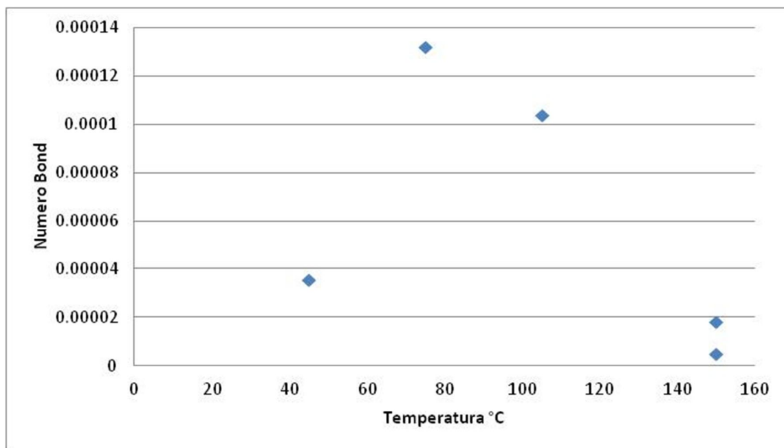
Figura 5.2 Número de Bond para r_p=1000 micras y L=.1 m
