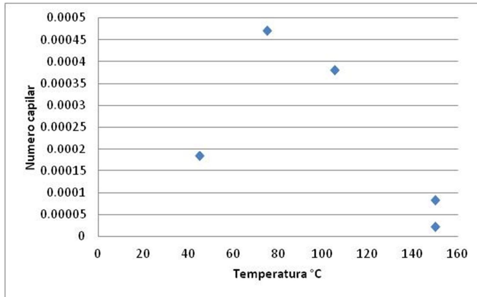
Figura 5.1 Comportamiento del Número Capilar campo Cacalilao en función de la temperatura.
