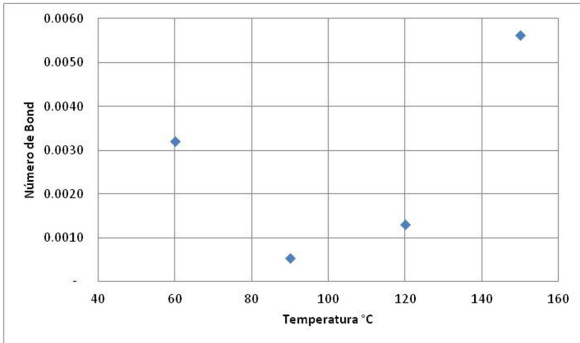
Figura 5.8 Número de Bond variando radio de poro
