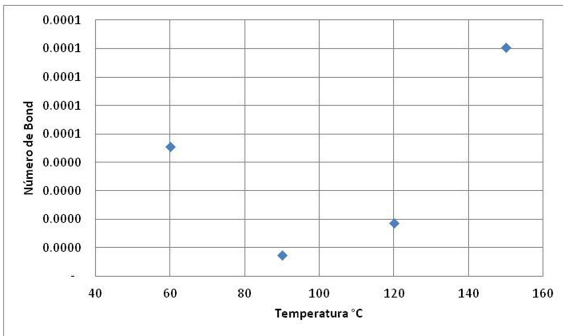
Figura 5.7 Comportamiento número de Bond campo Aguacate
