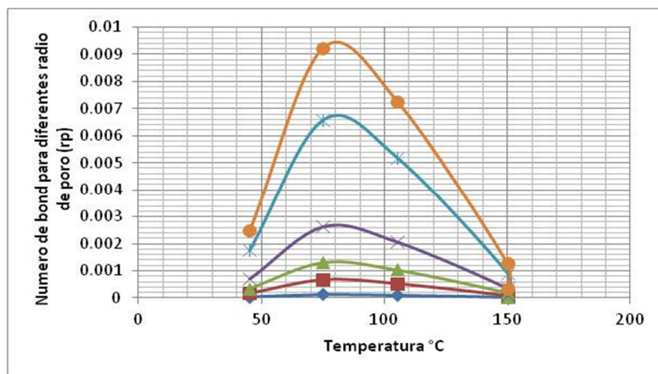
Figura 5.4 Número de Bond Para diferentes valores de radio de poro
