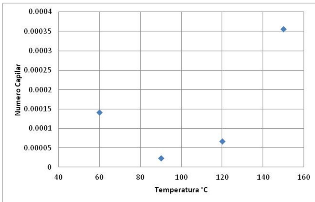
Figura 5.6 Número Capilar campo Aguacate 1
