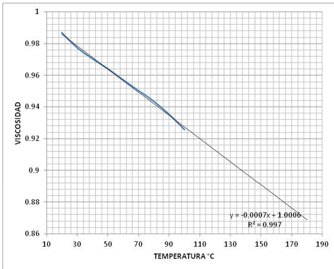
Figura 4.1 Comportamiento de la curva para obtener la ecuación de la viscosidad de Cacalilao
