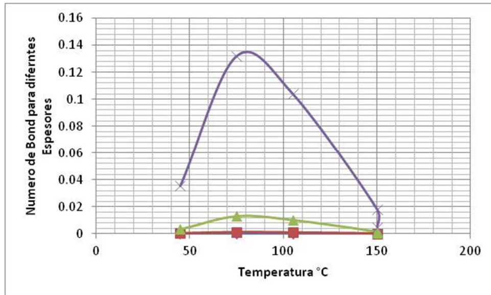
Figura 5.5 Numero de Bond Variando el espesor de la formación
