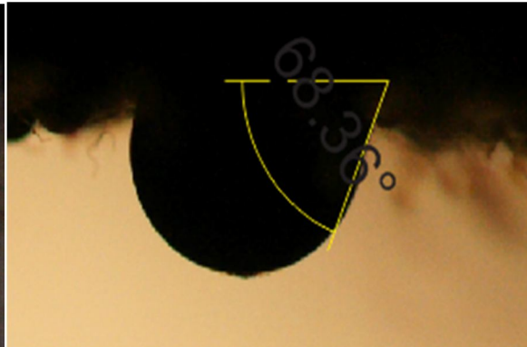
Figura 4.6 Medición ángulo contacto
