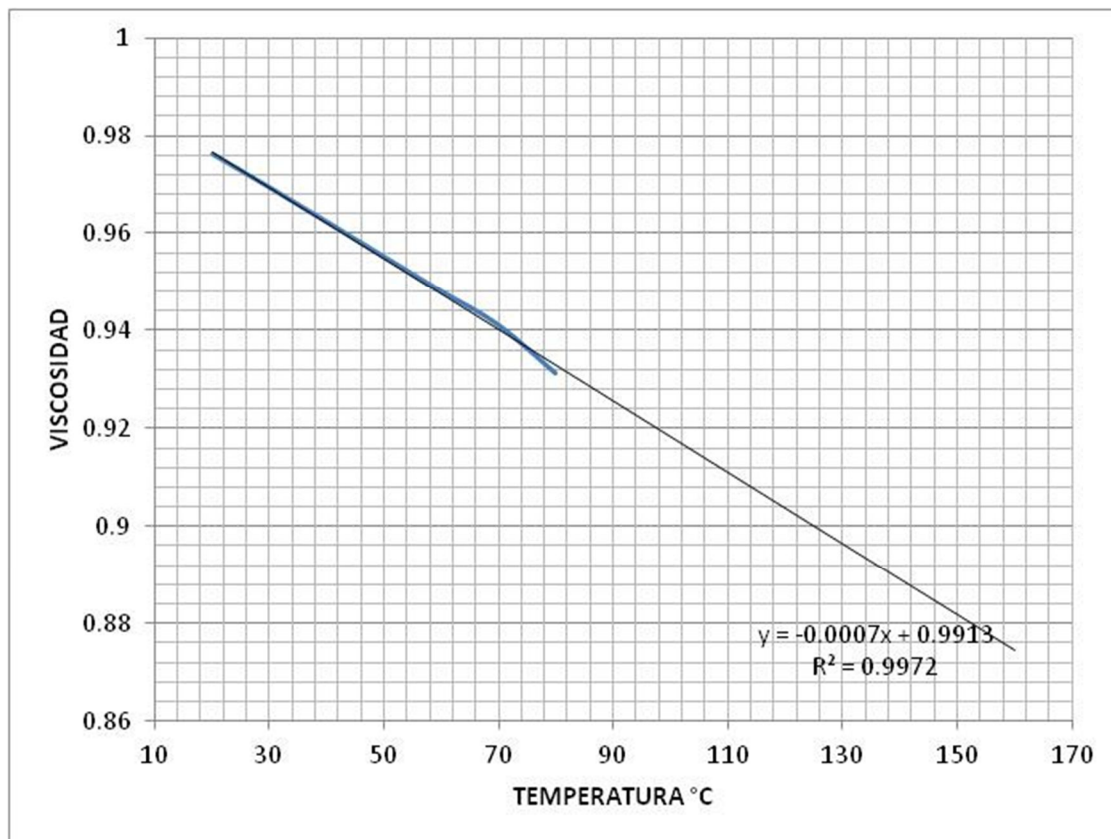
Figura 4.2 Viscosidad del campo Aguacate en función de la temperatura.
