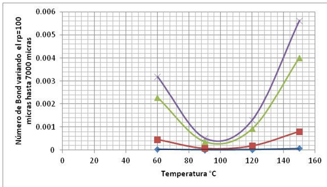
Figura 5.9 Número de Bond con diferentes valores de radio de poro
