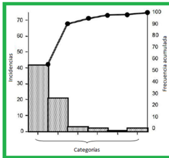
Figura 2.9 Ejemplos de gráfico de Pareto.
