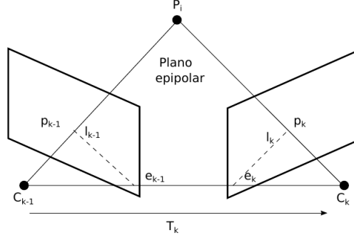
Figura 2.4.1: Geometría epipolar: se muestran las relaciones que existen entre un punto del mundo P_i , su proyección en los planos p_{k-1} , p_k , y la posición del centro de las cámaras C_{k-1} , C_k .
