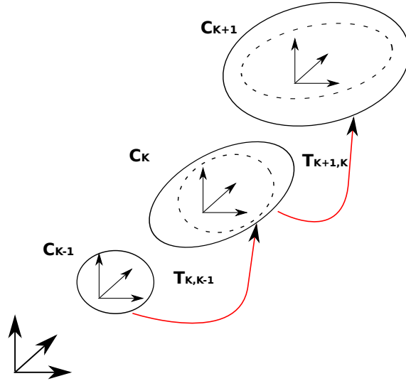
Figura 2.5.1: La incertidumbre de la posición de la cámara es una combinación entre la incertidumbre de la pose anterior y la incertidumbre en la transformación. Es un error incremental que se debe minimizar.
