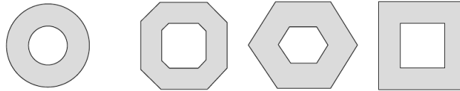
Figura 2.2.6: Filtros bi-nivel usados en CenSurE para aproximar el laplaciano. El círculo es la figura ideal que mejor aproxima al laplaciano, pero su cálculo es muy costoso; es más eficiente el cálculo de las imágenes a la derecha, pero se sacrifica un poco de precisión.
