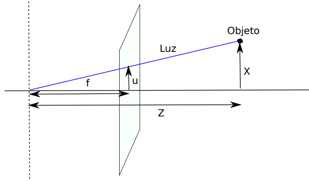
Figura 2.1.2: Modelo equivalente a la Figura 2.1.1. Este es usado para simplificar las operaciones de proyección.
