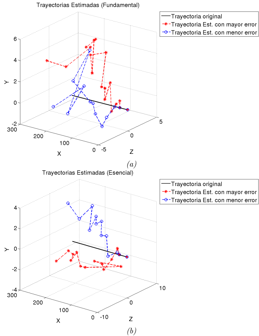
Figura 4.1.6: Se muestran las trayectorias con mejor y peor desempeño con respecto a la trayectoria original usando (a) la matriz Fundamental y (b) la matriz Esencial. Aunque la trayectoria roja es la que tiene mayor error acumulado se puede ver que no es una mala estimación y que le da seguimiento a la trayectoria original.
