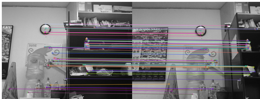
Figura 2.3.2: Emparejamiento con Fuerza Bruta + RANSAC. En esta imagen se muestra como solo se conservan los emparejamientos que cumplen con la restricción epipolar. Sin embargo, aún quedan emparejamientos falsos (emparejamiento entre un punto de la botella y un punto del cono en la parte inferior) pero estos errores ya son mínimos.
