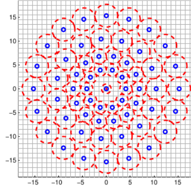
Figura 2.2.9: Patrón usado en el descriptor BRISK. Se escogen parejas de círculos a partir de un patrón definido. Estas combinaciones dan información sobre la escala y la orientación del punto. Adaptada de [24].
