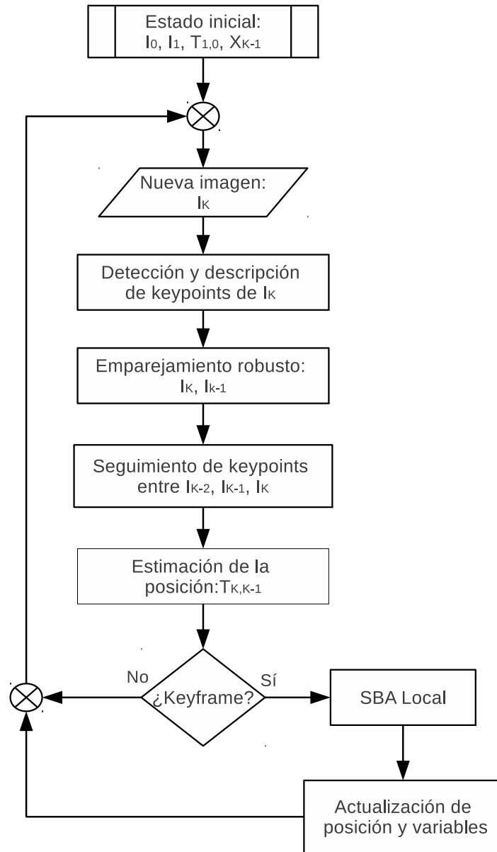
Figura 3.0.1: Diagrama de flujo del algoritmo propuesto.
