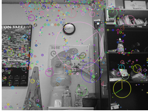
Figura 2.2.1: Ejemplo de la detección de puntos característicos usando el algoritmo SIFT. Este detector encuentra características sobresalientes en la imagen a partir de cambio de intensidad; los círculos muestran la posición, orientación y tamaño del punto detectado.
