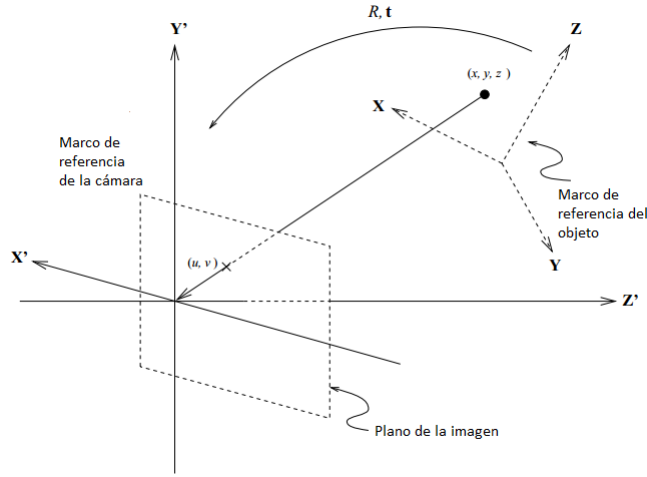
Figura 2.1.3: En esta figura se ilustra la transformación de cuerpo rígido que es necesaria para proyectar un objeto que se encuentra en un marco de referencia diferente.
