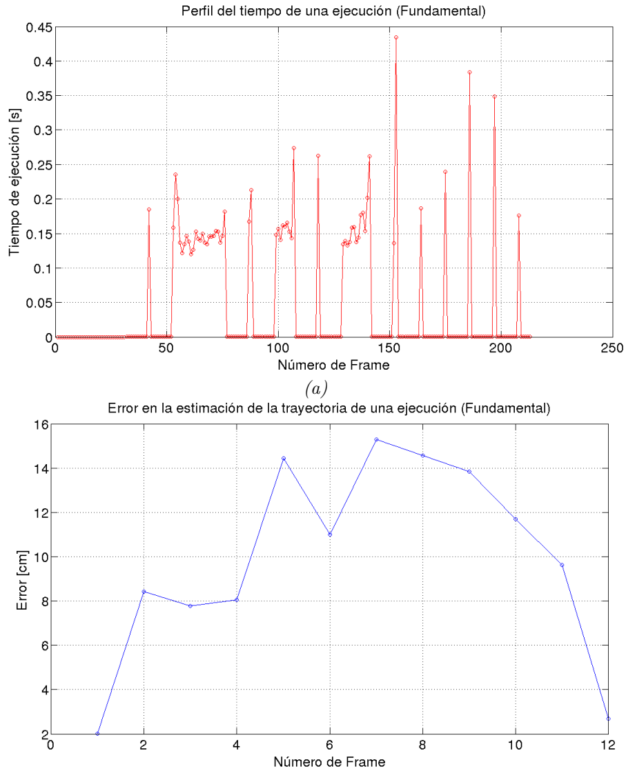
Figura 4.1.3: Perfil de tiempo y error de estimación en una sola ejecución. En (a) se puede observar el tiempo que tarda el sistema en procesar un frame, se muestra a los Keyframes como los picos más sobresalientes seguidos por tiempos cercanos a cero. Y en (b) se observa el error de estimación por Keyframe, se puede observar que el error no es del todo incremental como sucede en la odometría por ruedas, esto se sucede porque el SBA minimiza este error a partir de los puntos 3D y sus reproyecciones.
