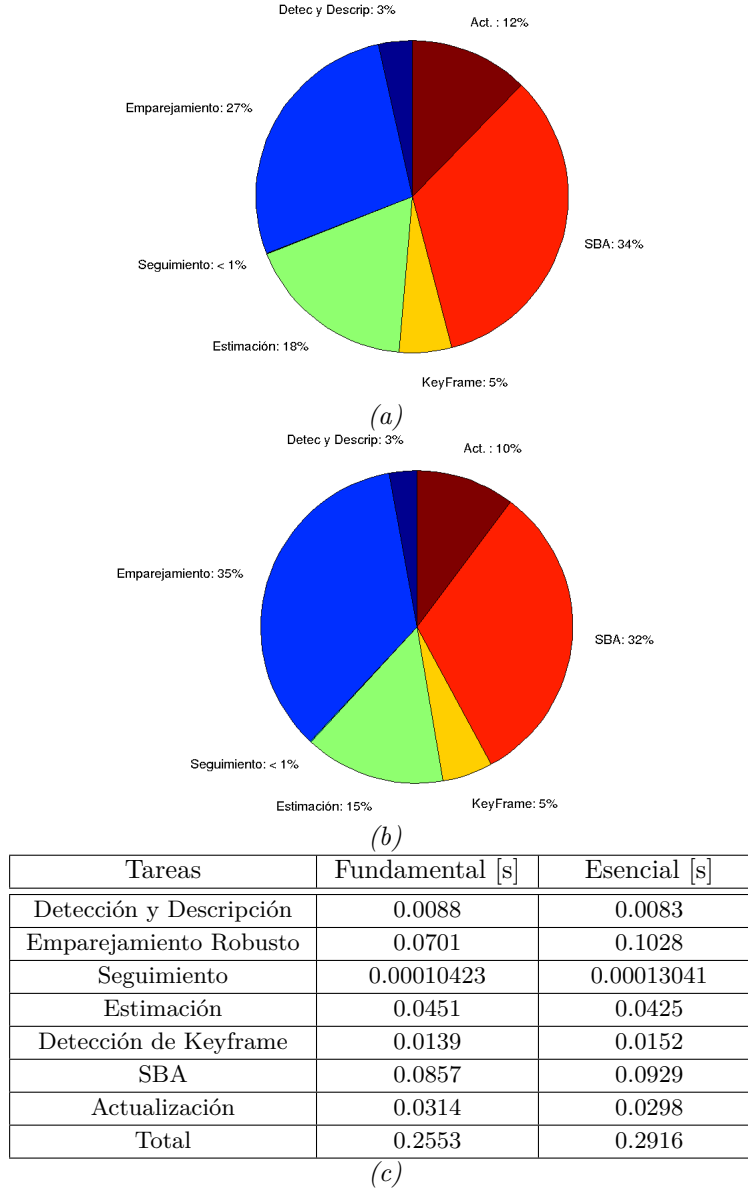
Figura 4.1.8: Se muestra el porcentaje de tiempo de cada tarea usando la matriz (a) Fundamental y (b) Esencial. De la tabla (c) observamos la cantidad de tiempo promedio por tarea. Las etapas que son más costosas computacionalmente son el emparejamiento robusto y el Sparse Bundle Adjustment.
