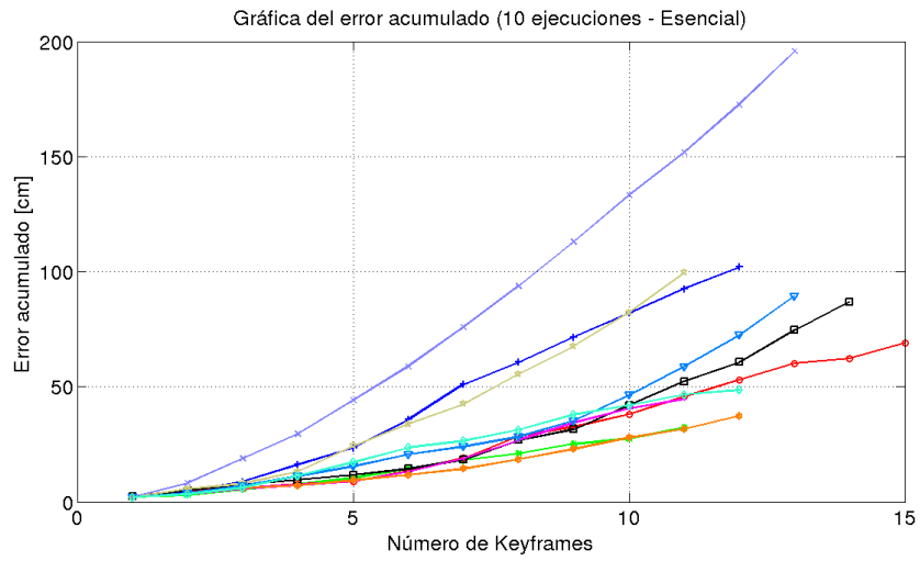
Figura 4.1.5: Con estas gráficas del error acumulado se puede determinar el desempeño individual de cada una de las ejecuciones. Las diferentes pendientes entre puntos indican las fluctuaciones en el error en cada estimación, es decir, en ocasiones el error puede ser mayor o menor a la estimación anterior.
