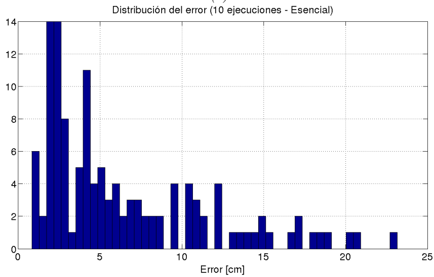
Figura 4.1.4: La distribución de los errores de las trayectorias estimadas; (a) matriz Fundamental, promedio = 9.3042 y desviación estándar = 6.4830; (b) matriz Esencial, promedio = 6.4956 y desviación estándar = 5.1094.
