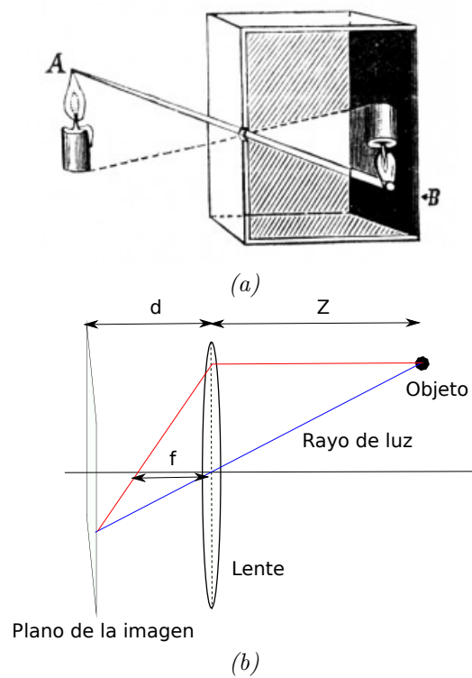
Figura 2.1.1: En (a) se muestra el concepto de pinhole , como un objeto en el espacio 3D es mapeado a un plano. Y en (b) se ilustra como este modelo es usado para describir la proyección en una cámara moderna.
