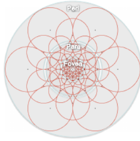
Figura 2.2.10: Patrón basado en de BRISK y en la retina humana usado en FREAK.
