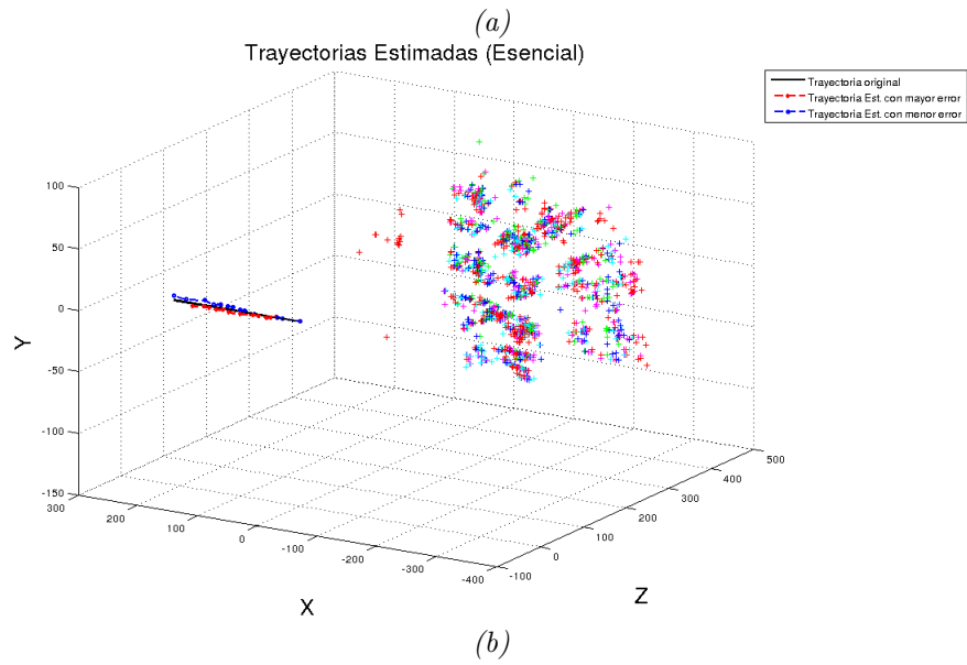
Figura 4.1.7: Vista de las trayectorias con respecto a la trayectoria original y con respecto a los puntos tridimensionales calculados para (a) Fundamental y (b) Esencial. A partir de los puntos tridimensionales podemos observar que existe una buena distribución de puntos de interés en la escena.
