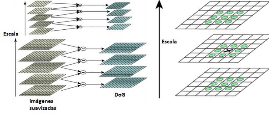
Figura 2.2.4: Representación gráfica de la extracción de características usando SIFT. Se observa como se obtienen las diferencias de Gaussianas y como se escoge el punto con mayor respuesta entre sus vecinos.
