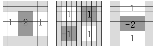
Figura 2.2.5: Filtros usados para aproximar la convolución en SURF.
