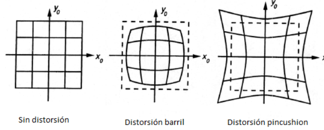
Figura 2.1.4: En esta figura se muestra como el lente de la cámara puede distorsionar el plano de la imagen. Adaptada de [35].
