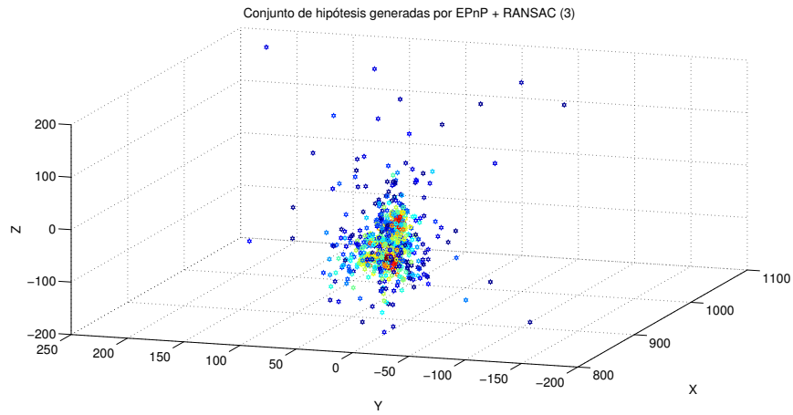
Figura 4.1.12: Las gráficas (a) y (b) muestran la disposición de las estimaciones en diferentes perspectivas de manera que se pueda apreciar con mayor detalle como varía la distribución en este Keyframe que falló. La notación usada es la misma que en la Figura 4.1.11. Aquí se puede observar que la distribución es multimodal, se tienen dos regiones con máximos. Tener más de un máximo en regiones distintas del espacio es la causa por la que el sistema falla, una de esas estimaciones considerada como máximo debe ser falsa.
