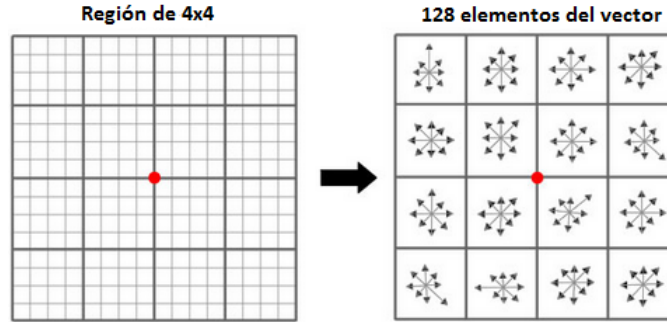
Figura 2.2.8: Forma en la que SIFT obtiene los valores de su vector de descripción. Se crean histogramas de orientaciones ponderadas sobre la vecindad del punto de interés. La orientación del punto y los valores de estos histogramas conforman al vector de descripción.
