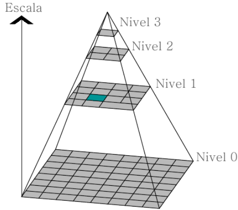
Figura 3.2.1: El detector FAST se aplica a cada celda de la cuadrícula en todos los niveles de la pirámide Gaussiana y sólo se conservan los puntos con la mayor respuesta en su respectiva celda.
