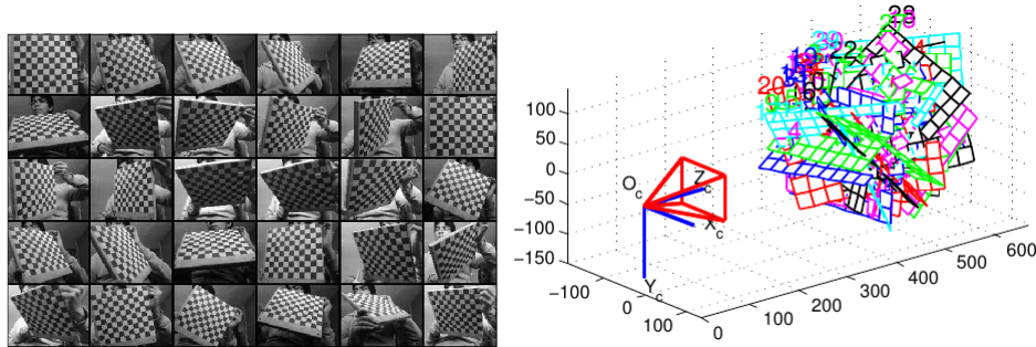
Figura 2.1.5: Calibración de la cámara usando el toolbox de MATLAB: conjunto de imágenes con el patrón de ajedrez (izquierda); posiciones del tablero estimadas por el software de calibración (derecha).
