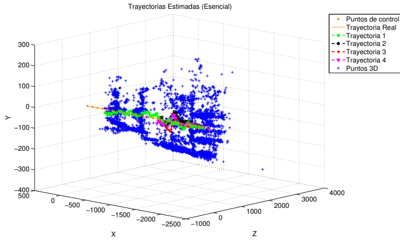
Figura 4.1.10: En la gráfica (a) se puede ver la estimación incompleta de las trayectorias. Y en (b) se ponen en perspectiva estas trayectorias con respecto a los puntos 3D calculados. La odometría visual además de estimar la posición también genera un mapa de puntos de la escena, en la imagen se pueden apreciar las paredes localizadas entre las casas, las banquetas y el adoquín.
