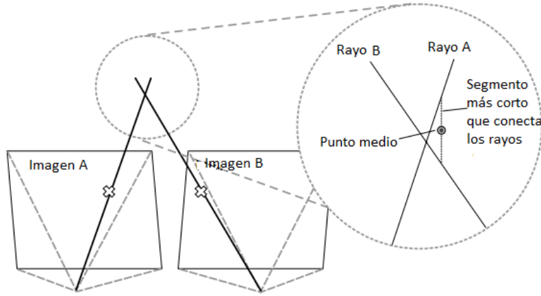
Figura 2.4.2: Triangulación: Método del punto medio para estimar un punto 3D del mundo.
