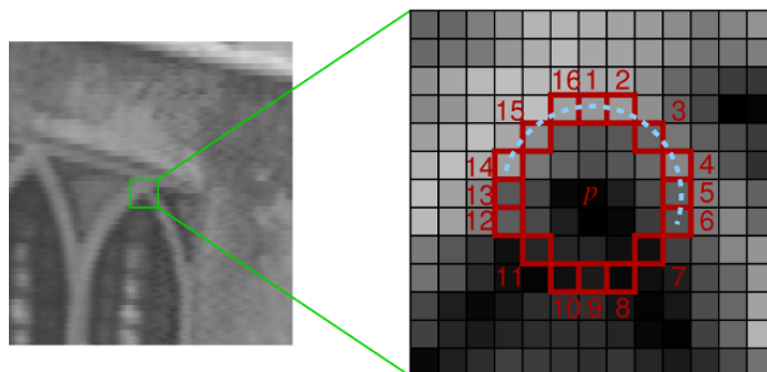
Figura 2.2.3: Representación gráfica de la evaluación que realiza FAST para determinar si el pixel p es una esquina. Adaptada de [36].
