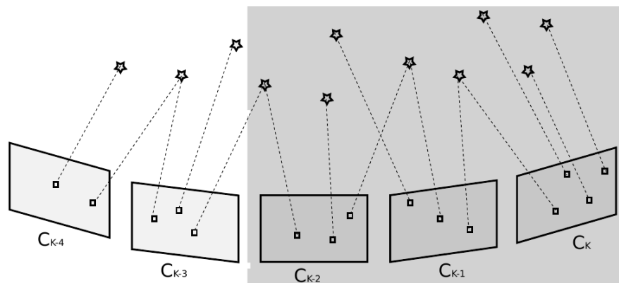
Figura 2.5.2: El Bundle Adjustment Local sólo optimiza los parámetros de las vistas más recientes, en esta figura se observa que sólo se usarán 3 vistas para refinar la estimación.
