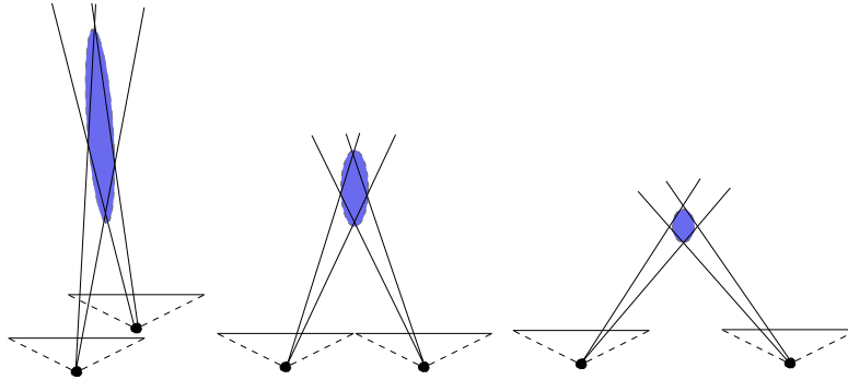
Figura 3.6.1: La región azul indica la incertidumbre en la localización del punto 3D. Esta incertidumbre depende del ángulo entre los rayos proyectados.
