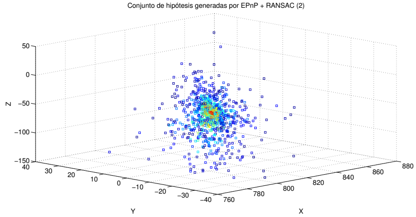
Figura 4.1.11: Distribución de las posiciones estimadas por EPnP con RANSAC antes de que fallara el sistema en el \text{Keyframe}_k . Las posiciones en (a) son las que se estimaron en el \text{Keyframe}_{k-2} y las posiciones en (b) se estimaron en el \text{Keyframe}_{k-1} . Los colores indican el número de puntos que se encuentran dentro del modelo estimado, el color azul es para aquellos con pocos puntos, y el rojo cuanta con la mayoría. Se puede apreciar que las estimaciones siguen una distribución monomodal.
