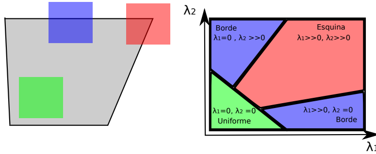
Figura 2.2.2: En esta figura se muestra la relación que existe entre los valores de \lambda_1 y \lambda_2 , y la región de la imagen analizada. Cómo se puede observar, los valores de \lambda_1 y \lambda_2 son altos cuando el área analizada es una esquina.
