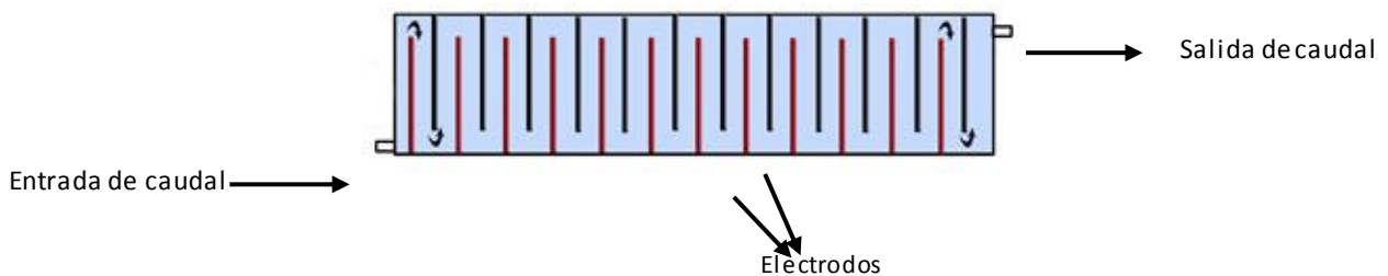
Figura 2.17 Reactor de electrocoagulación a flujo pistón
