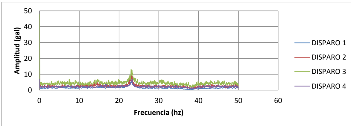
Figura 6.49 Gráfica de promedio H/V, campaña 4, cuarta cerrada la marquesa, equipo 1.
