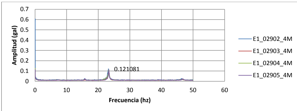
Figura 6.58 Espectro de Fourier Dirección Longitudinal (2).
