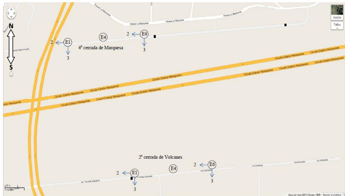
Fig. 5.6 Croquis de localización de equipos correspondiente a la cuarta campaña de mediciones: 4ª cerrada de la marquessa y 2ª cerrada de volcanes (17/12/2012).
