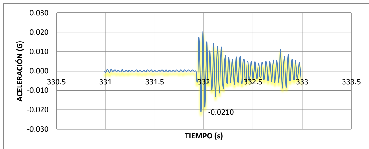
Figura 6.5 Registro acelerográfico de equipo 3, campaña 1, disparo 5, dirección 2.
