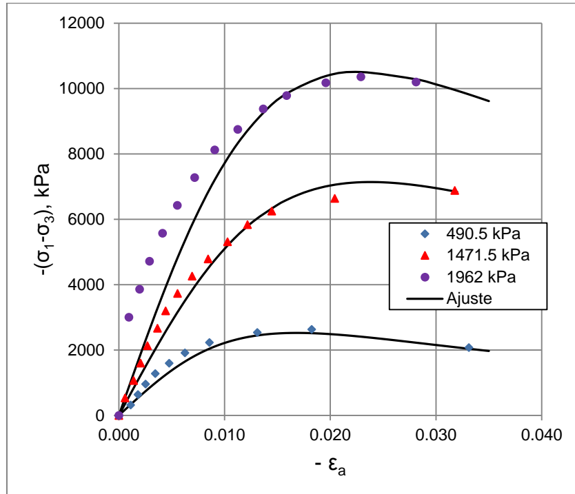
Figura 6.1 Ajuste de curvas esfuerzo – deformación nat. axial con Modelo de Ductilidad tipo Hiperb3lico para el material aluvi3n.
