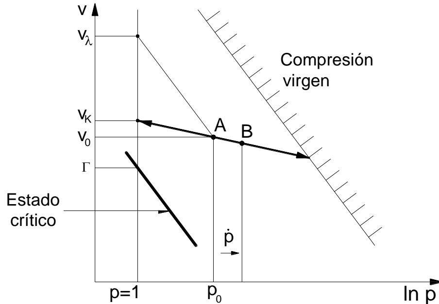
Figura 4.9 Obtención de los parámetros v_\lambda , v_k y \Gamma del modelo del estado crítico (modificado de Romo y Rojas, 1993).
