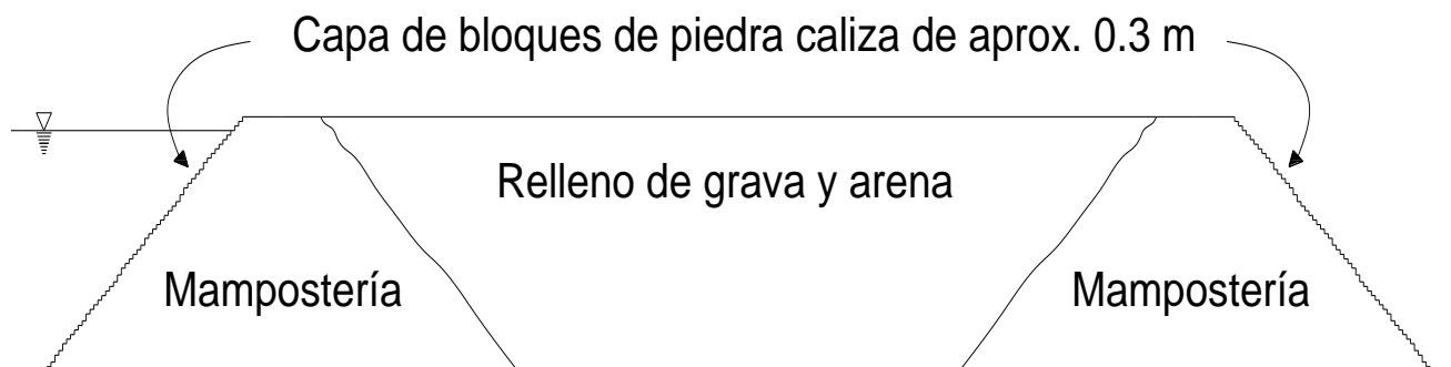
Figura 2.1 Esquema de la presa Sadd el-Kafara: Presa de los Paganos
