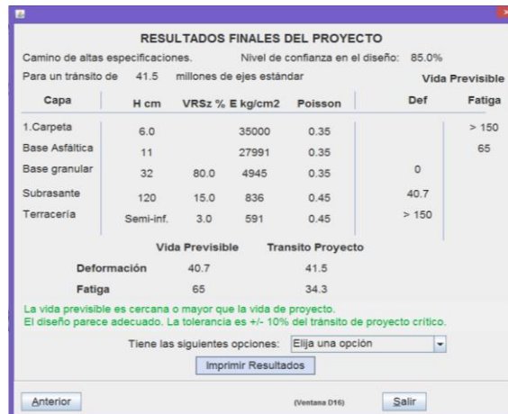
Figura 4.12. Alternativa I del cuerpo B obtenido con el DISPAV 5(V3)
