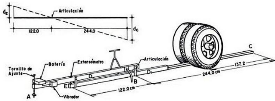
Figura. 3.13 Esquema operacional de la Viga Belkelman (Fuente: La ingeniería de suelos en las vías terrestres, Alfonso Rico Rodríguez, Hermilo del Castillo, 1974).
