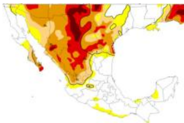
Figura33 Consenso y obtención de mapas del NADM. Fuente: SMN, 2013.
