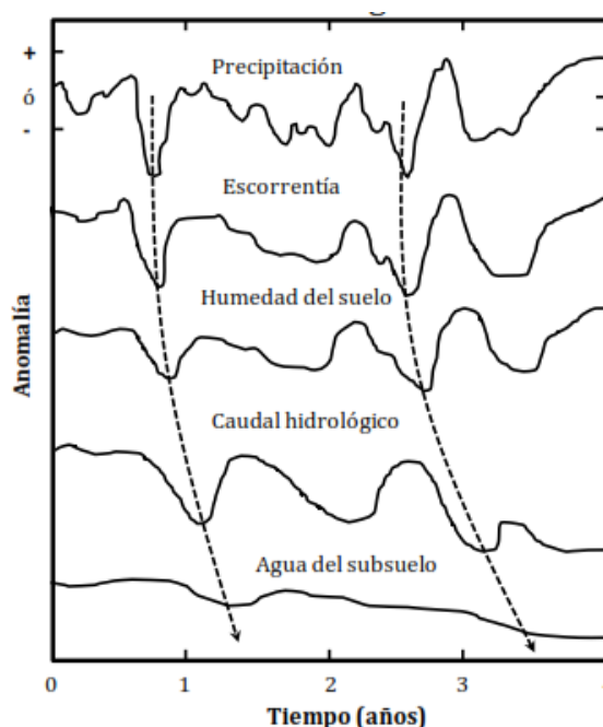
Figura 3 Desfase temporal en la propagación de anomalías pluviométricas hacia los diversos niveles del ciclo hidrológico.
