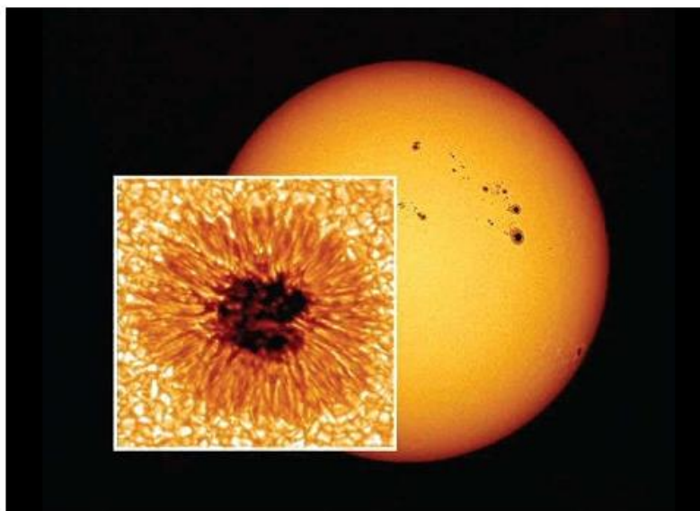
Figura8 La superficie solar y sus manchas, algunas llegan a ser tan grandes como el planeta Júpiter. Fuente: (Universidad de Utrecht, Holanda).
