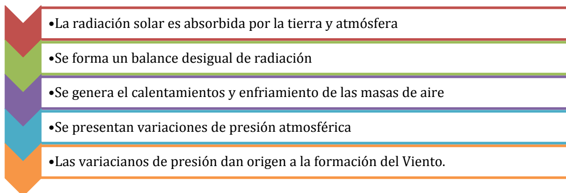
Figura 7. Proceso de formación de las masas de aire. Fuente: (Ortega - Gaucín, 2012).
