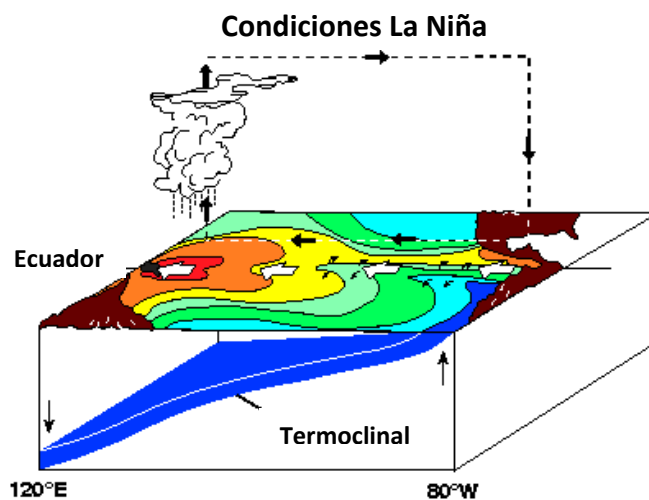
Figura12. Condiciones del clima con Niña. Fuente: (CienciayBiología, 2012)
