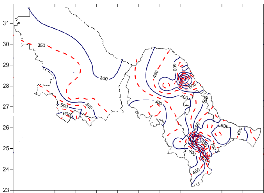
Figura47 Isoyetas medias históricas para la RHA VI.
