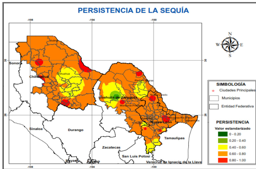
Figura115 Zonas estandarizadas con mayor persistencia de sequía de acuerdo al SPI 6 . Fuente: Elaboración propia.
