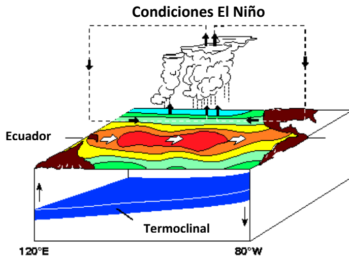
Figura11. Condiciones del clima con Niño. Fuente: (CienciayBiología, 2012)
