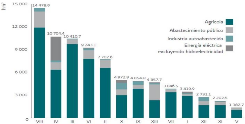
Figura56 Usos consuntivos del agua en México. Fuente: CONAGUA, 2010.
