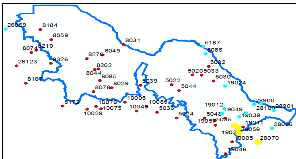
Figura83 Recurrencia de meses con sequía según SPI de 1 mes para el periodo (1980-2012). Fuente: Elaboración propia.
