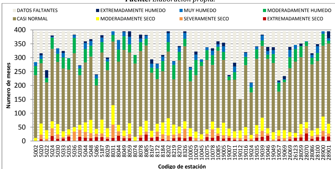
Figura81 Número de eventos de sequías según SPI para una duración de 12 meses (1980-2012).
