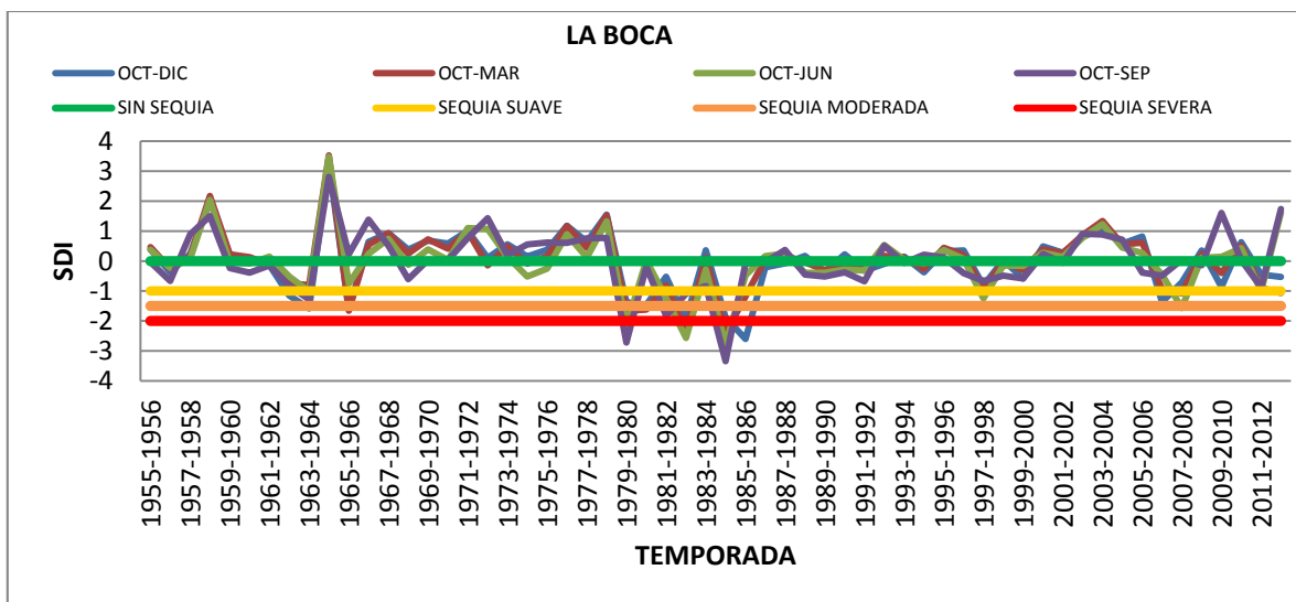
Figura95 Gráfico de comportamiento del SDI histórico para la presa La Boca periodo 1980-2012.
