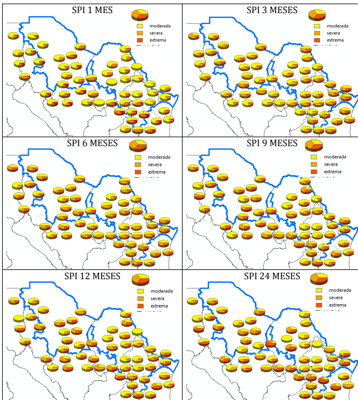
Figura87 Mapas de número de eventos y tipo de sequía según SPI para el periodo (1980-2012).
