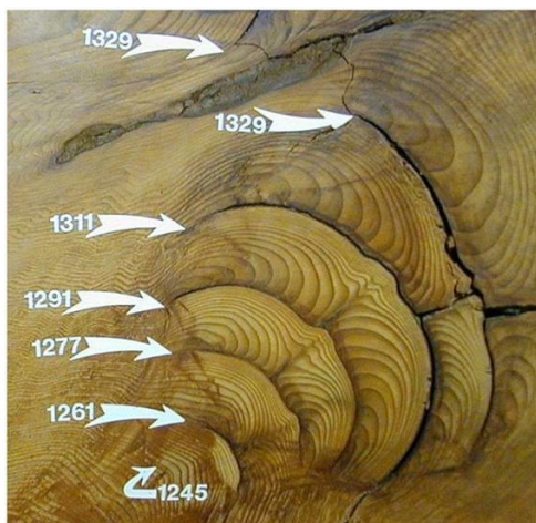
Figura37 Lecturas de datos del clima en anillos de árboles.
