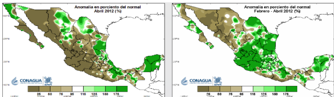
Figura30 Anomalía de lluvias a 1 y 3 meses. Fuente: SMN, 2013.
