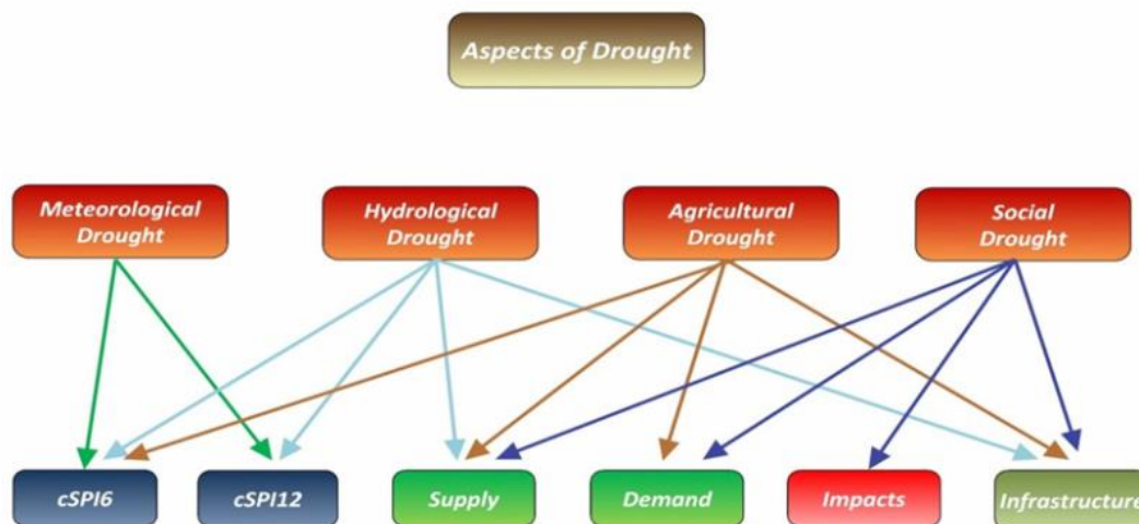
Figura100 Relación entre componentes del índice de vulnerabilidad a la sequía y aspectos de sequía. Fuente: (Karavitis, 2013)
