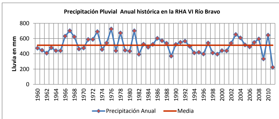
Figura48 Precipitación pluvial anual histórica y media en la RHA VI.
