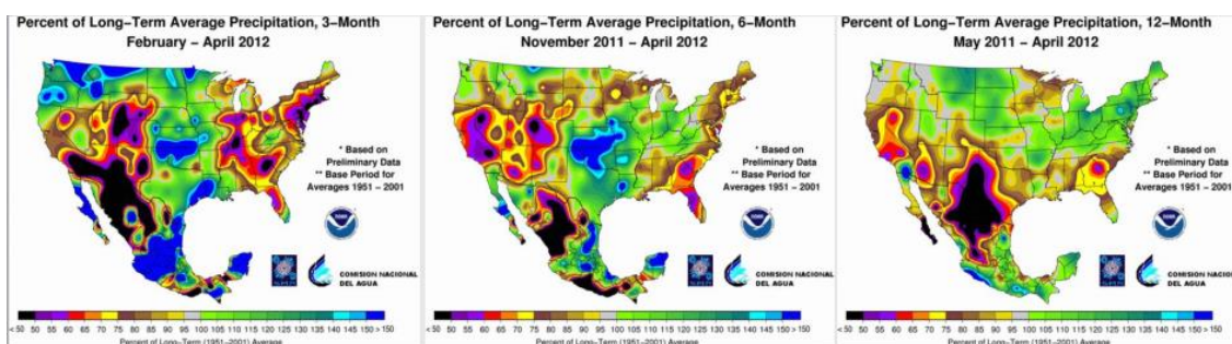
Figura 27 Porciento de precipitación normal calculado para el NADM. Fuente: SMN, 2013.
