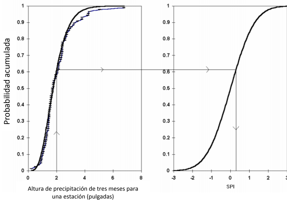
Figura 72 Ejemplo de la transformación de equiprobabilidad de la distribución Gamma ajustada a la distribución normal estandar.
