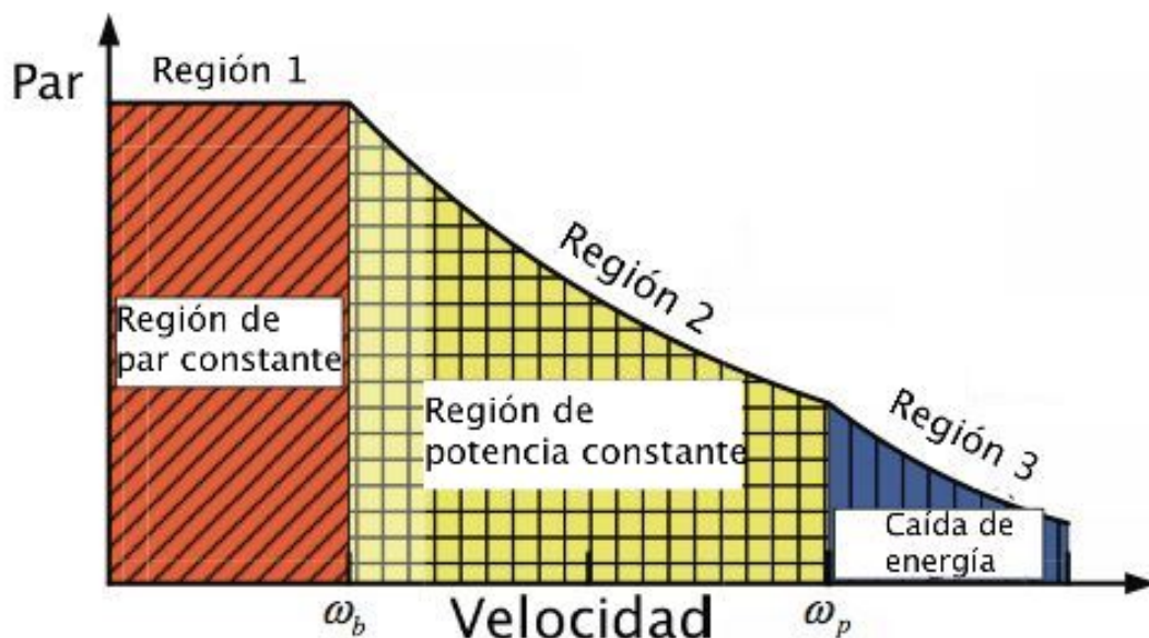
Figura 2.6: Curva Par-Velocidad
