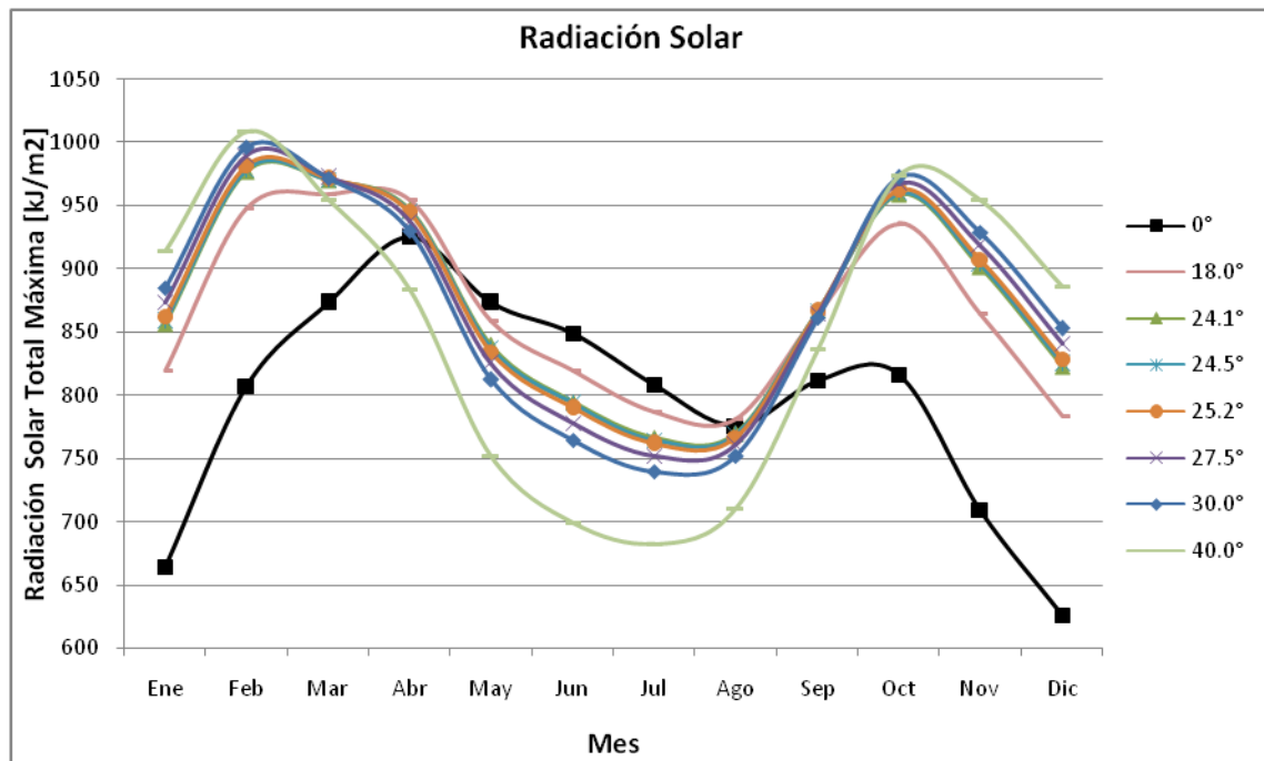
Figura 46. Radiación Solar máxima incidente sobre un plano a diferentes valores de \beta .
