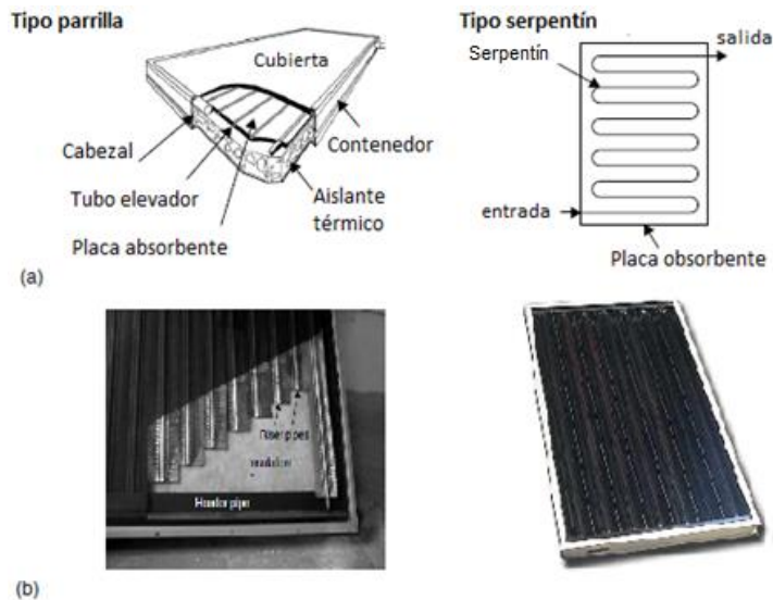
Figura 9. Colector típico de placa plana. a) representación gráfica de los componentes del colector. b) imagen de un colector solar.
