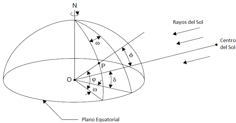
Figura 26. Definición de los ángulos de declinación, latitud y horario.
