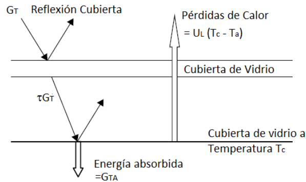
Figura 34. Ganancia y pérdida de calor en el colector solar.
