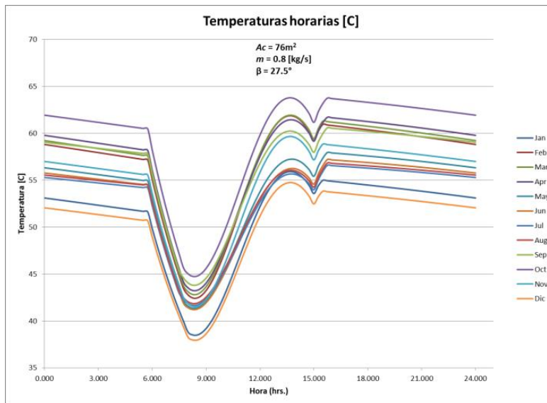
Figura 45. Perfil de temperaturas del caso optimizado (A_c, \beta, m) = (76, 27.5, 0.8)
