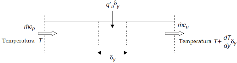
Figura 36. Flujo de energía a través de un elemento infinitesimal a lo largo del tubo.
