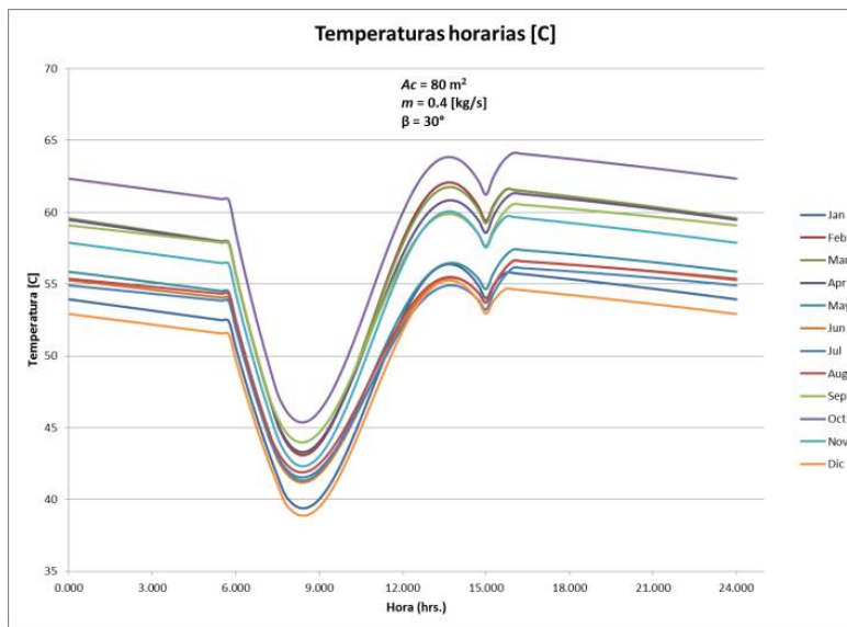
Figura 44. Perfil de temperaturas del caso base (A_c, \beta, m) = (80, 30, 0.4) .
