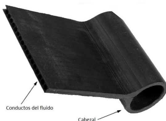
Figura 11. Colector de placa plana de baja temperatura fabricado en plástico.
