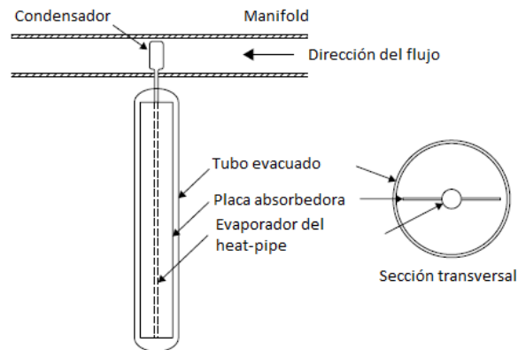
Figura 13. Esquema de funcionamiento de los tubos evacuados con Heat Pipe.
