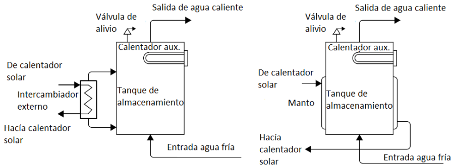
Figura 20. Ejemplificación de posicionamiento de intercambiadores de calor: izquierda, intercambiador externo; derecha, intercambiador de manto.
