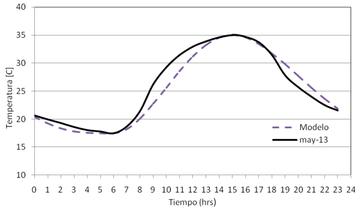
Figura 39. Comprobación del modelo matemático para la T_{amb} .
