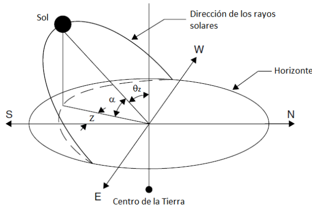
Figura 28. Esquema ángulos de acimut y de altitud del sol.
