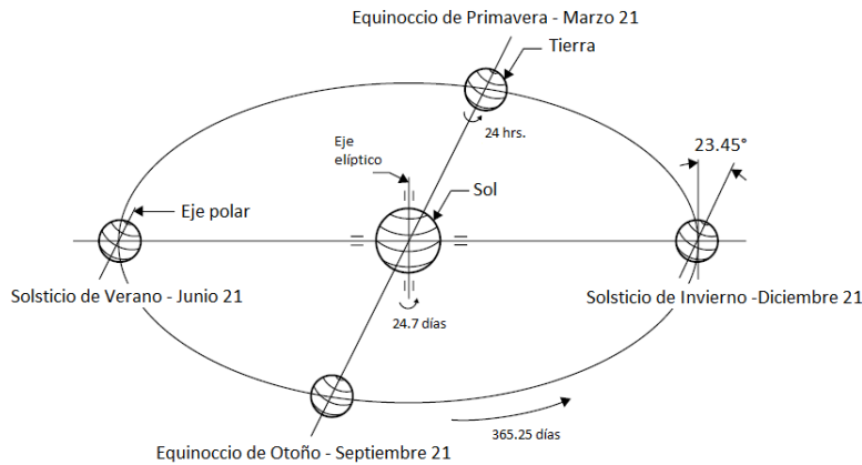
Figura 24. Movimiento de la Tierra alrededor del Sol.
