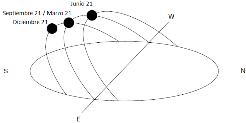
Figura 25. Posiciones del Sol a lo largo del año.
