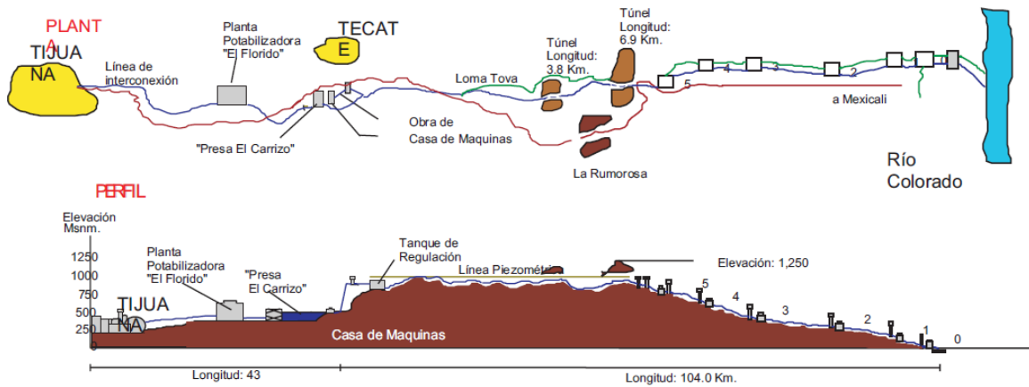
Figura 3.12 Recorrido de la línea de conducción del agua proveniente del río Colorado desde la presa Morelos (límite binacional) hasta la presa El Carrizo (Tijuana) por ARCT
