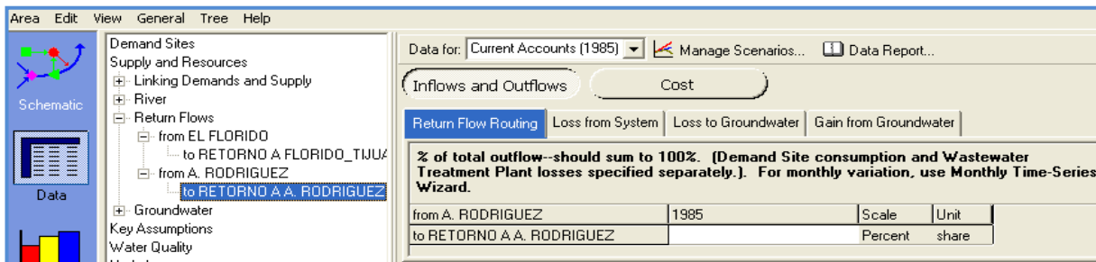
Figura 4. 51 Retorno que va de la A.L. Rodríguez a la derivación Florido_Tijuana en WEAP
