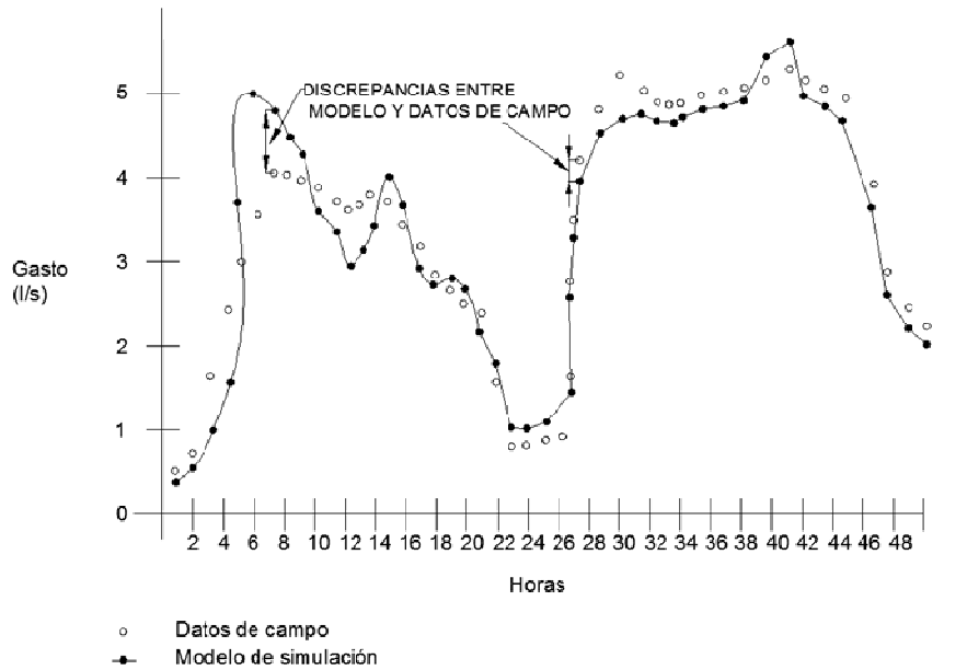
Figura 3.2.- Discrepancias entre el modelo de simulación hidráulico y los datos de campo medidos en el punto X, tomados en la fecha Y. Fuente: Elaboración propia.
