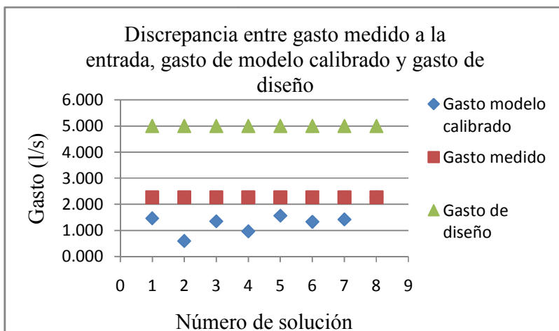
Figura 7.3.9b.-Prueba 2: Discrepancia entre gastos, en red de dos circuitos.
