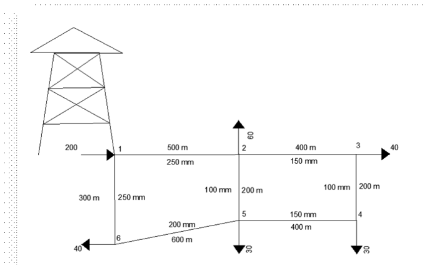
Figura 7.3.2 Red hidráulica ejemplo para calibración de coeficientes de rugosidad y demanda.
