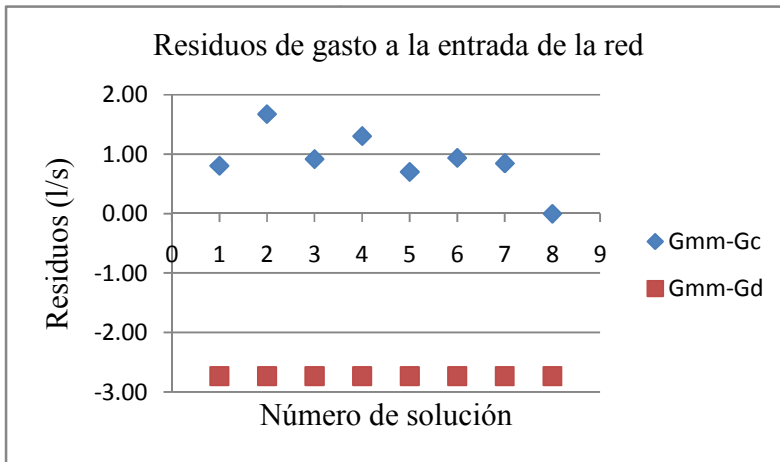
Figura 7.3.9e.-Prueba 2: Residuos de gasto a la entrada de la red de dos circuitos.
