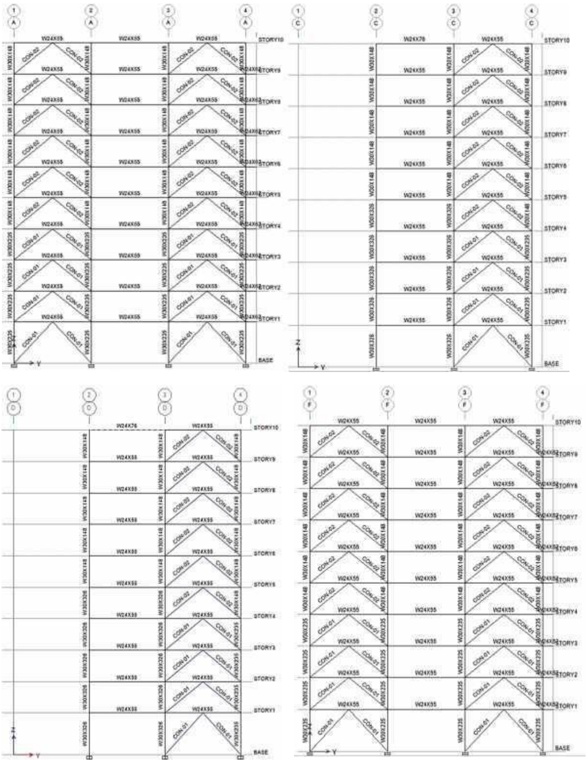
Figura 8.9 Ubicación de los contraventeos, (vista en elevación).
