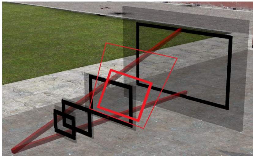
Ilustración 24. En la imagen se muestra un área de visión errónea (en color rojo). Se debe garantizar un área rectangular de visión rectangular paralela al piso para evitar deformaciones indeseadas.
