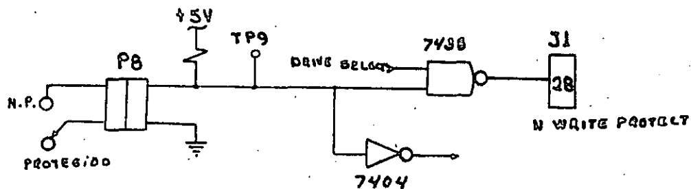
Figura 4.6. Circuito de protección de escritura.
