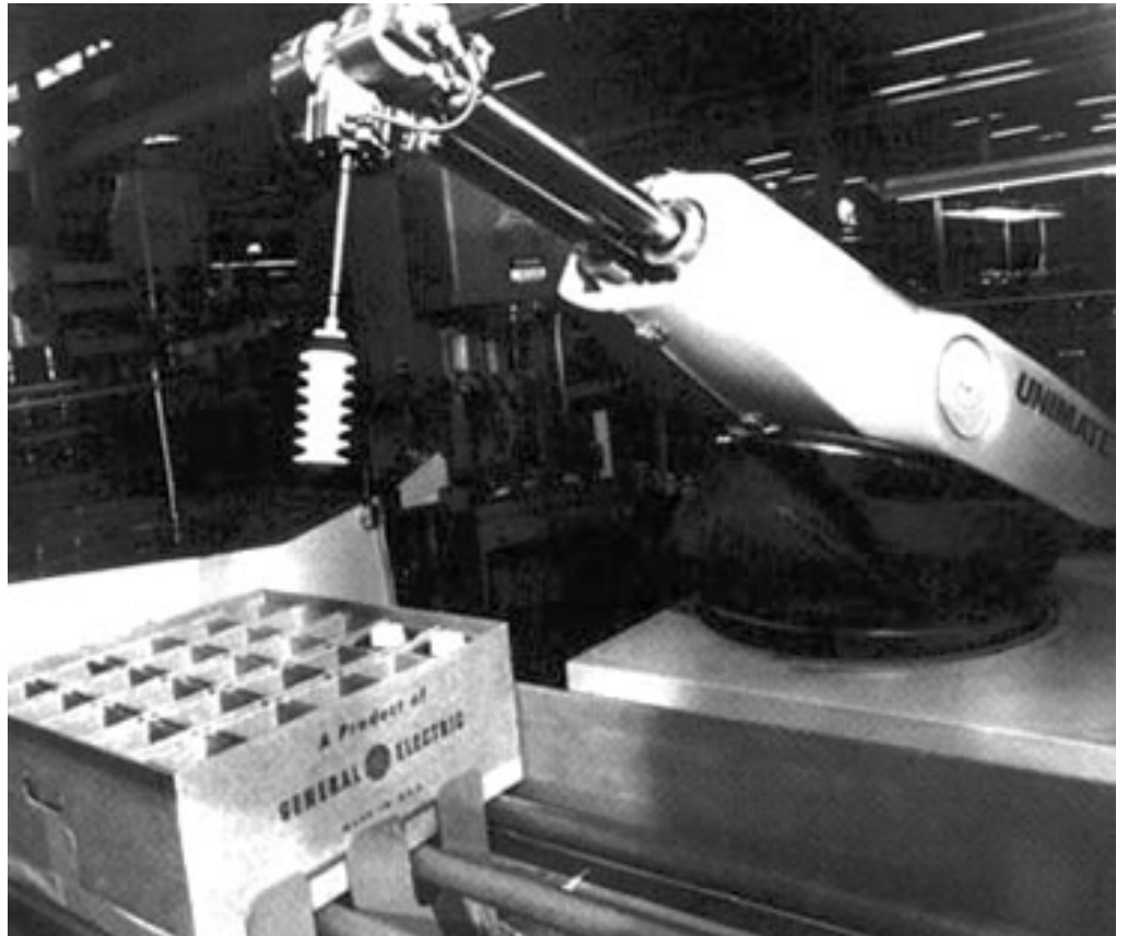
Imagen 2. UNIMATE trabajando.
