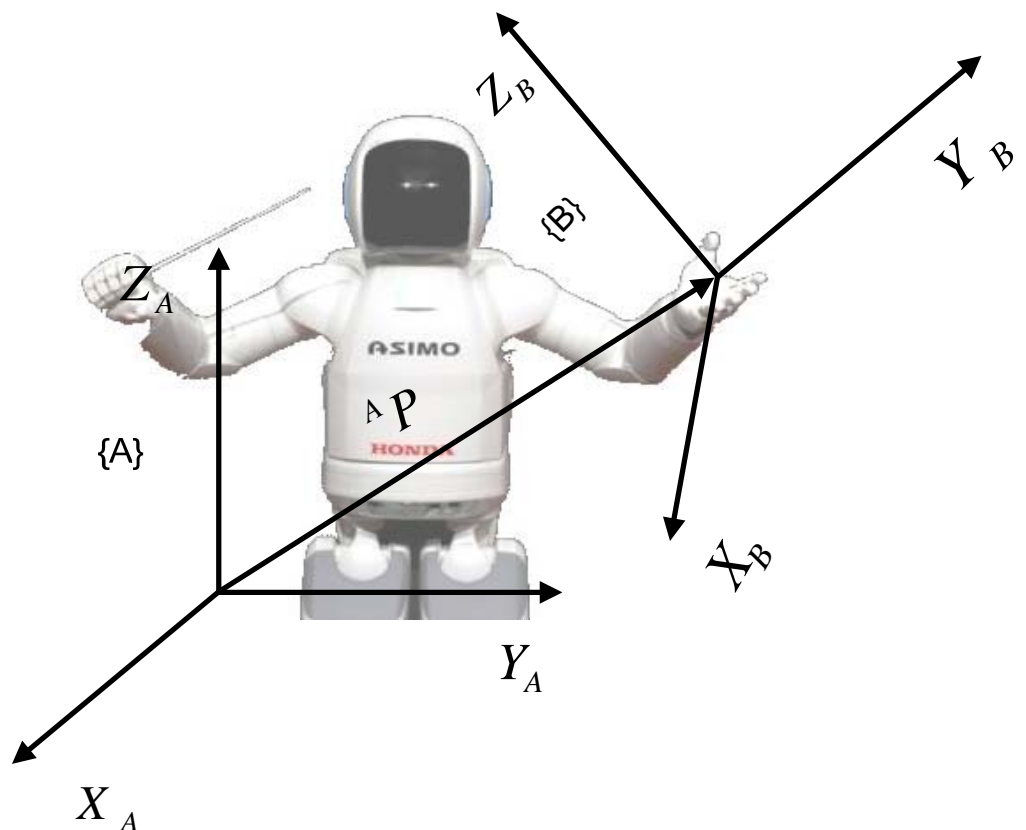
Imagen 19. Ubicación de un objeto en posición y orientación.
