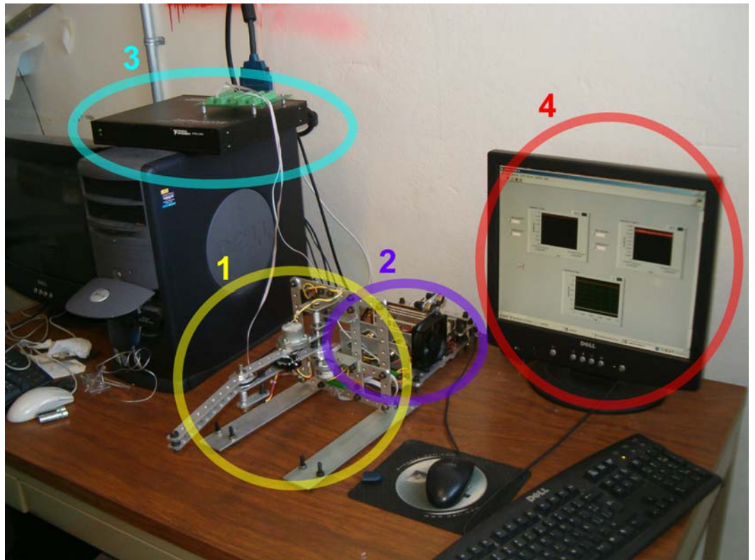
Imagen 6. El SR y cada uno de sus subsistemas, 1. Manipulador de dos grados de libertad, 2. Amplificador de potencia, 3. Dispositivo de adquisición de datos, 4. Interfaz gráfica de usuario.
