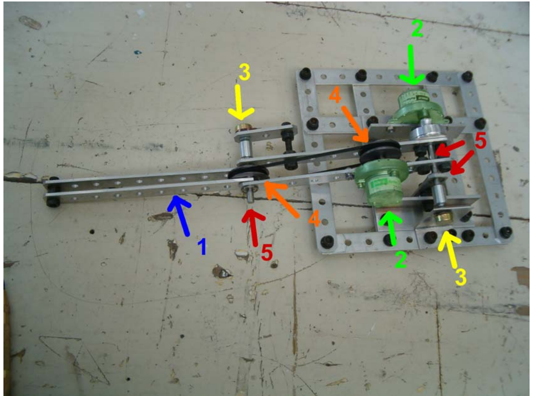
Imagen 7. Manipulador 2 GDL, 1. Perfiles de aluminio, 2. Motores de DC de 12[V], 3. Potenciómetros de 10 [k \Omega ], 4. Poleas dentadas y banda dentada 5. Rodamientos y ejes.
