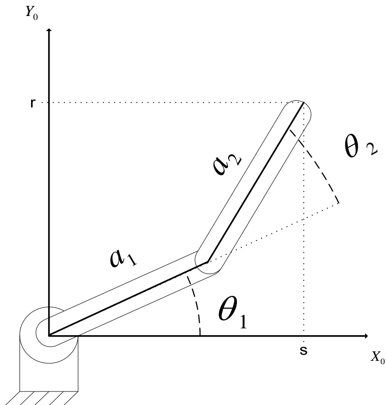
Imagen 10. Angulos y longitudes en el manipulador.
