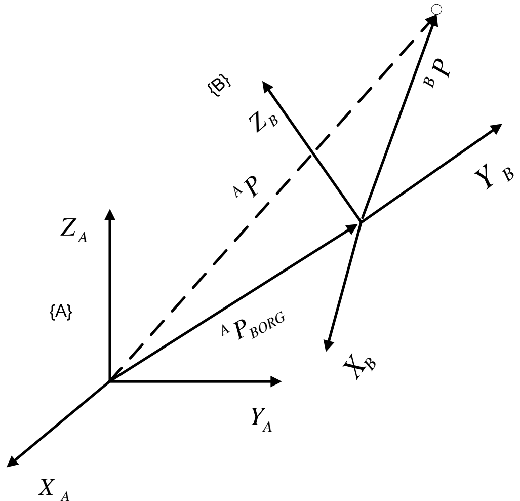
Imagen 20. Transformada general de un vector del sistema {B} al sistema {A}.
