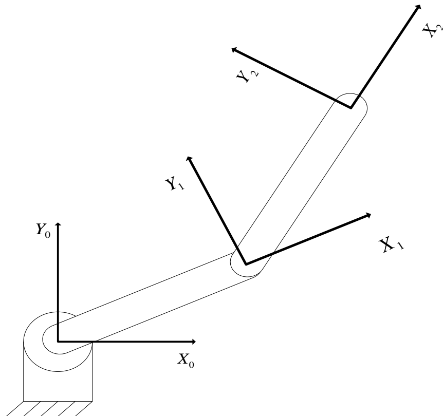
Imagen 9. Sistemas de referencia en el manipulador.
