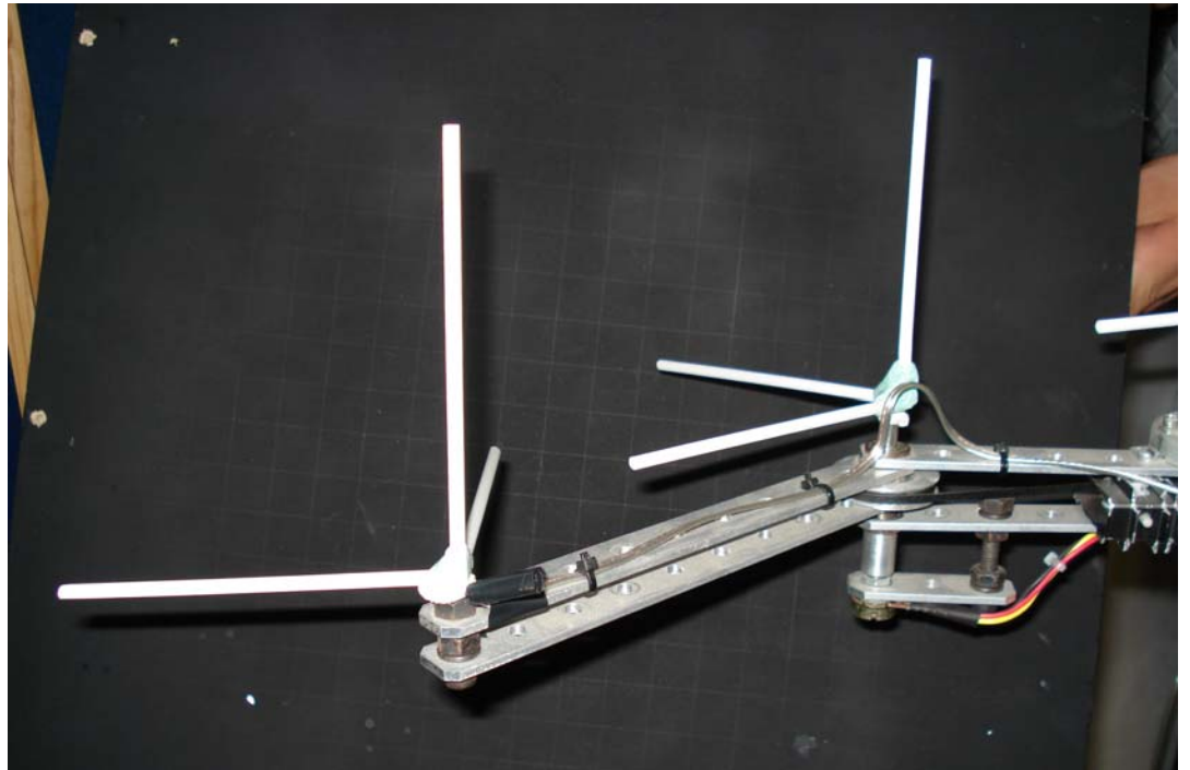
Imagen 22. Orientaciones en el SR, en los sistemas de referencia formados por popotes blancos el eje z es el que apunta hacia arriba.
