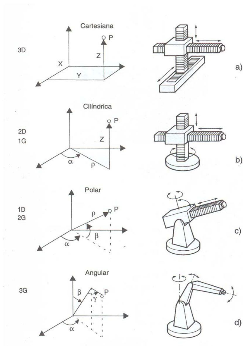
Imagen 16. Configuraciones de manipuladores 21 .
