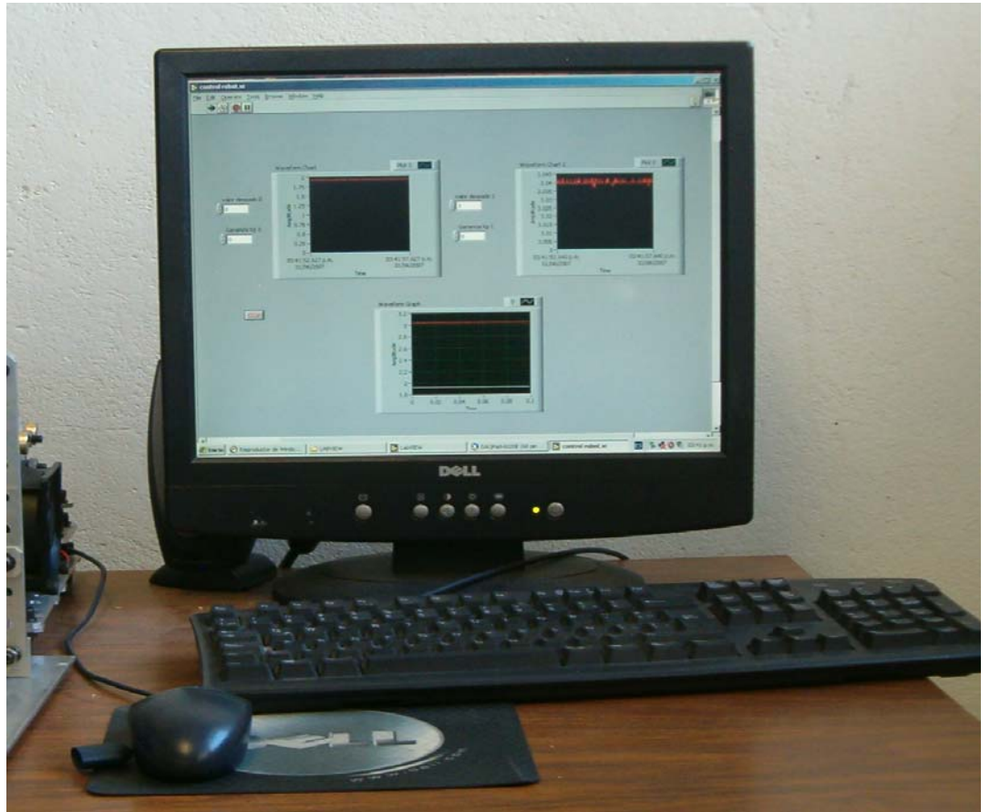
Imagen 14. GUI.
