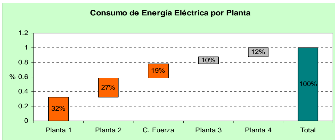
Gráfico 3 Consumo de energía eléctrica por etapa del proceso
