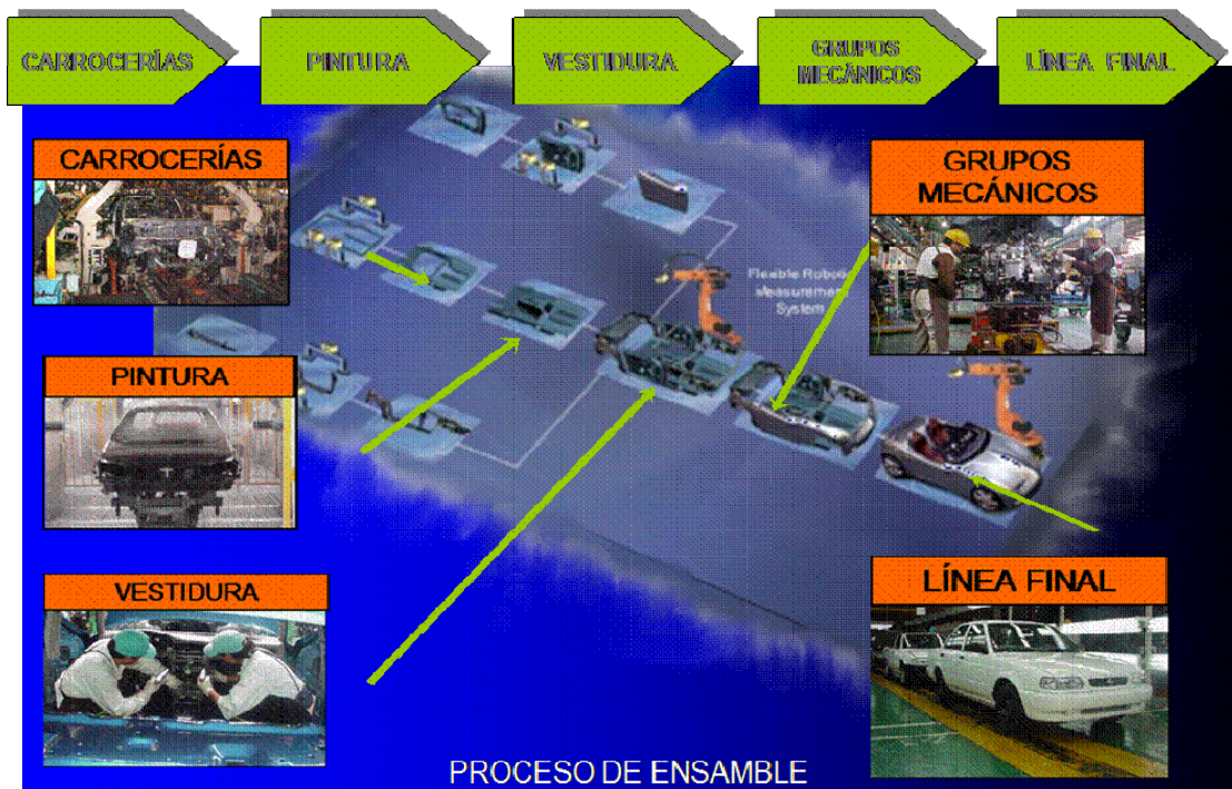
Fig. 2 Etapas del proceso de ensamble del vehículo
