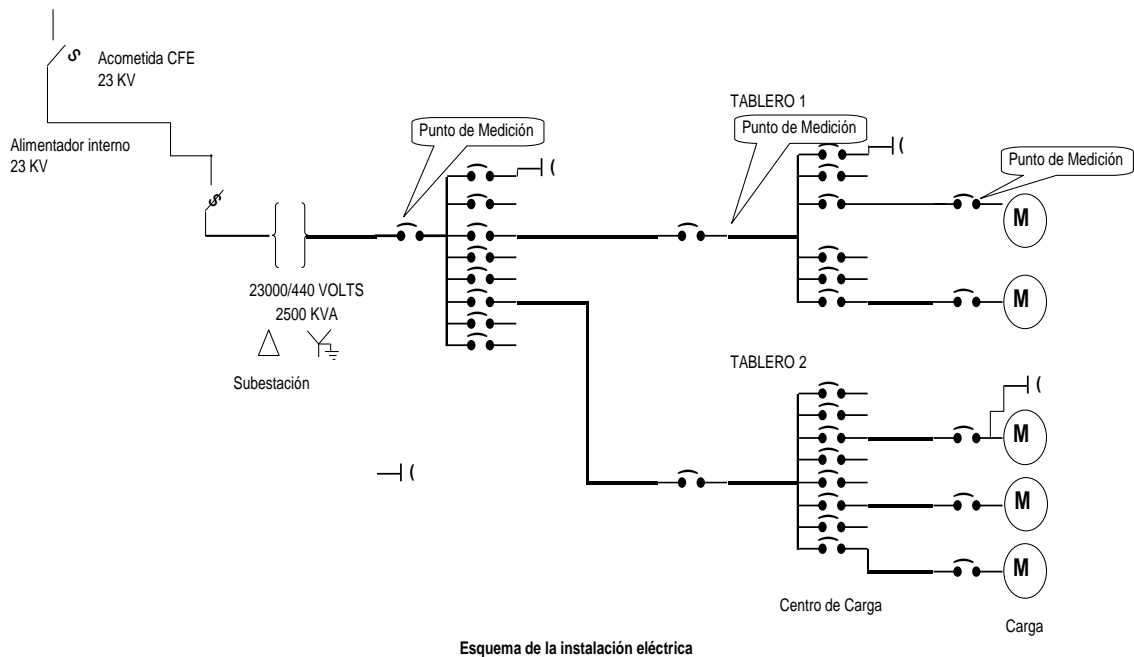
Fig. 5 Esquema de la instalación eléctrica y zonas de medición para el diagnóstico energético
