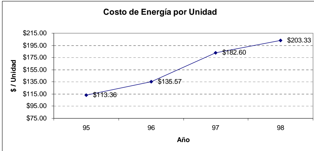
Gráfico 8 Costo de la energía eléctrica por unidad producida Planta Civac (95~98)
