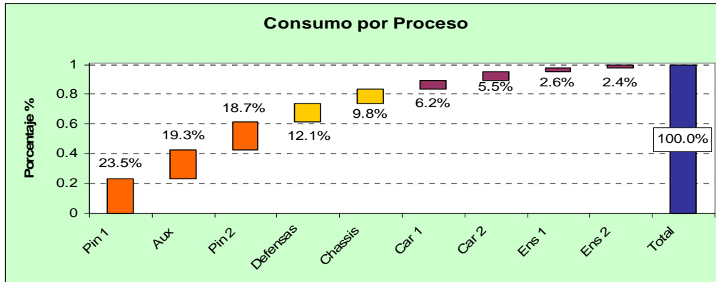
Gráfico 11 Aportación por proceso al consumo total de energía
