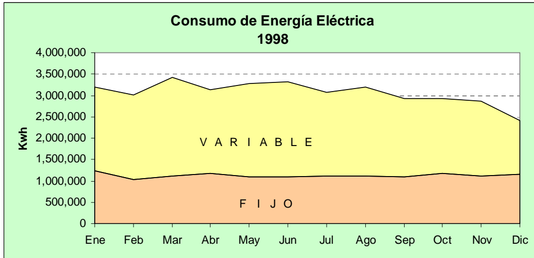
Gráfico 1 Comportamiento del consumo variable y fijo
