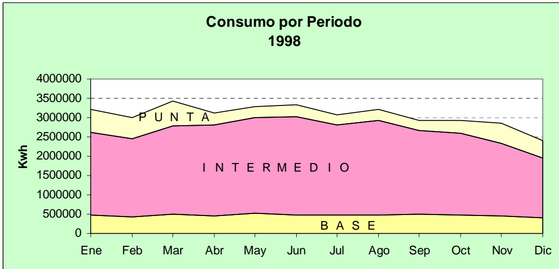
Gráfico 2 Comportamiento del consumo según periodos de facturación
