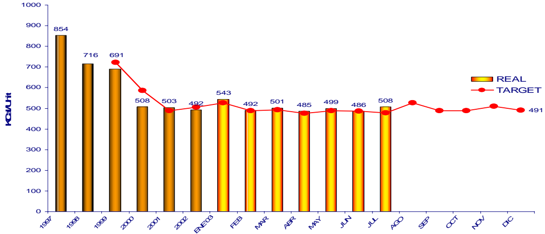
Gráfico 14 Comportamiento del Índice Energético Kcal/Unidad (97~03) del Complejo Industrial Cuernavaca
