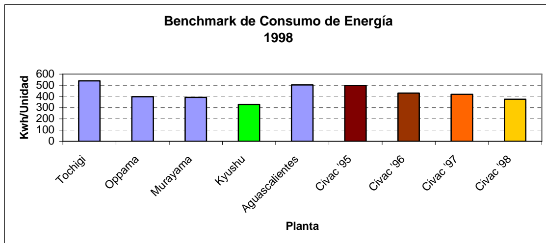
Gráfico 9 Índice energético de plantas industriales de Nissan (Benchmark)
