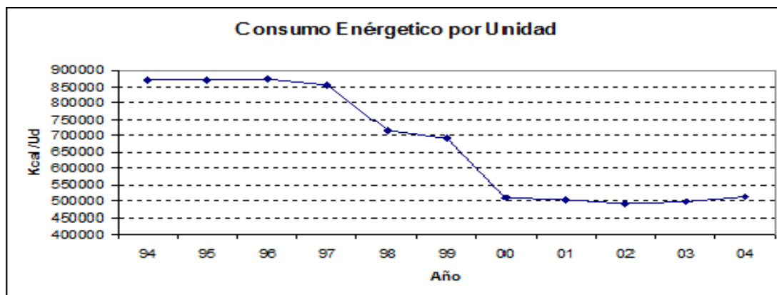
Gráfico 12 Comportamiento del índice energético Kcal/Unidad 94~04
