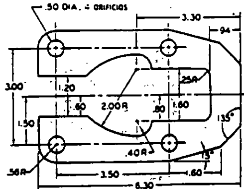
Fig. 2.94 Placa para carradura. Usando el plan A-2, dibuje a lápiz. Omita dimensiones y notas.
