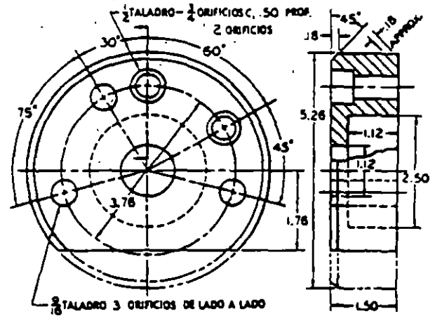
Fig. 2.90 Cubretapa. Usando el plan A-2, dibuje estas vistas a lápiz. Omite dimensiones y notas. Ver 17 B.
