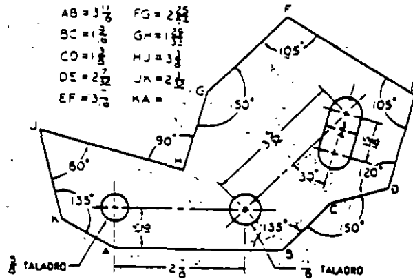
Fig. 2.92 Placa para esfuerzo cortante. Usando el plan A-2, dibuje con toda precisión a lápiz. De la longitud de KA. Omita las otras dimensiones y notas.
