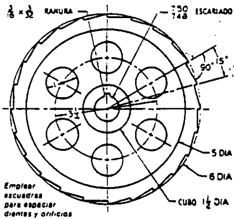
Fig. 2.93 Rueda dentada o de trinqueta. Empleando el plan A-2, dibuje a lápiz. Omita dimensiones y notas.
