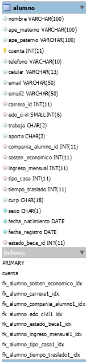
ILUSTRACIÓN 8 - TABLA ALUMNO
