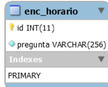
ILUSTRACIÓN 28 - TABLA HORARIO
