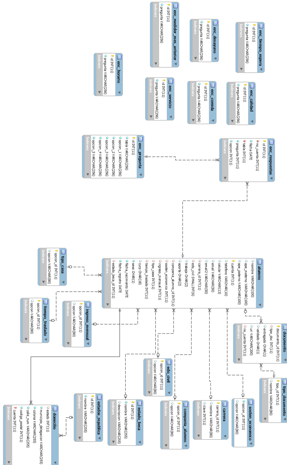
ILUSTRACIÓN 30 - DIAGRAMA ENTIDAD-RELACIÓN
