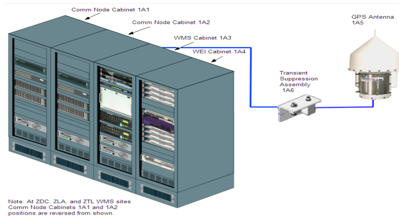
Figura 3.11. Gabinete con nodos de comunicaciones, WMS, WEI, y antena GPS.
