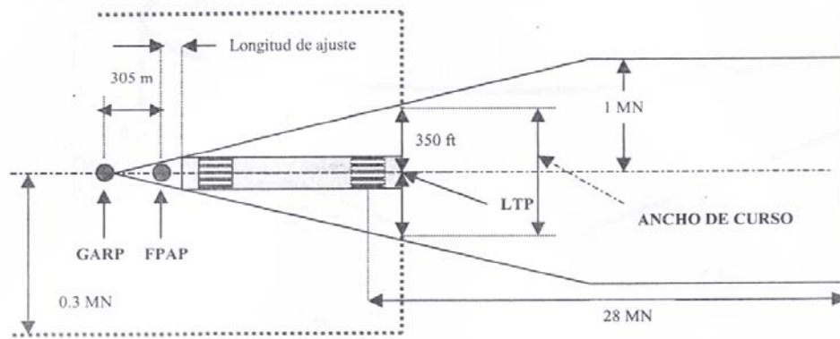
Figura 4.4. Diagrama de desviación lateral del sistema LAAS.
