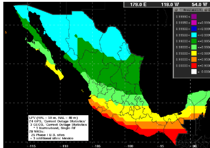
Figura 4.8. Disponibilidad de cobertura del sistema WAAS con 3 estaciones WRS para aproximaciones LPV (VAL – 50 m, HAL – 40 m) con 0.9 de probabilidad, arrojados por el estudio ionosférico en la mayor parte de la República Mexicana.
