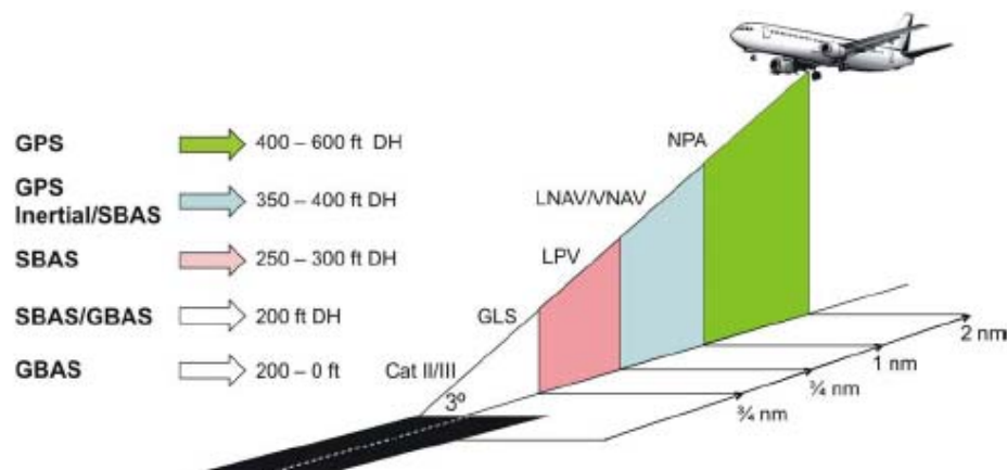
Figura 2.13. Definición de Alturas para aproximación a pista con GPS/WAAS.
