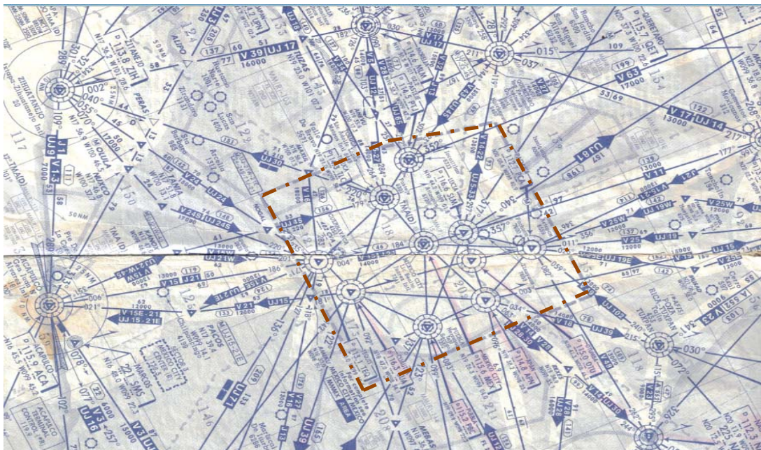
[15] Figura. 4.17. El tráfico aéreo confluye hacia el cuadro de aproximación terminal sobre el chequeo electrónico de los VOR circundantes al AICM.
