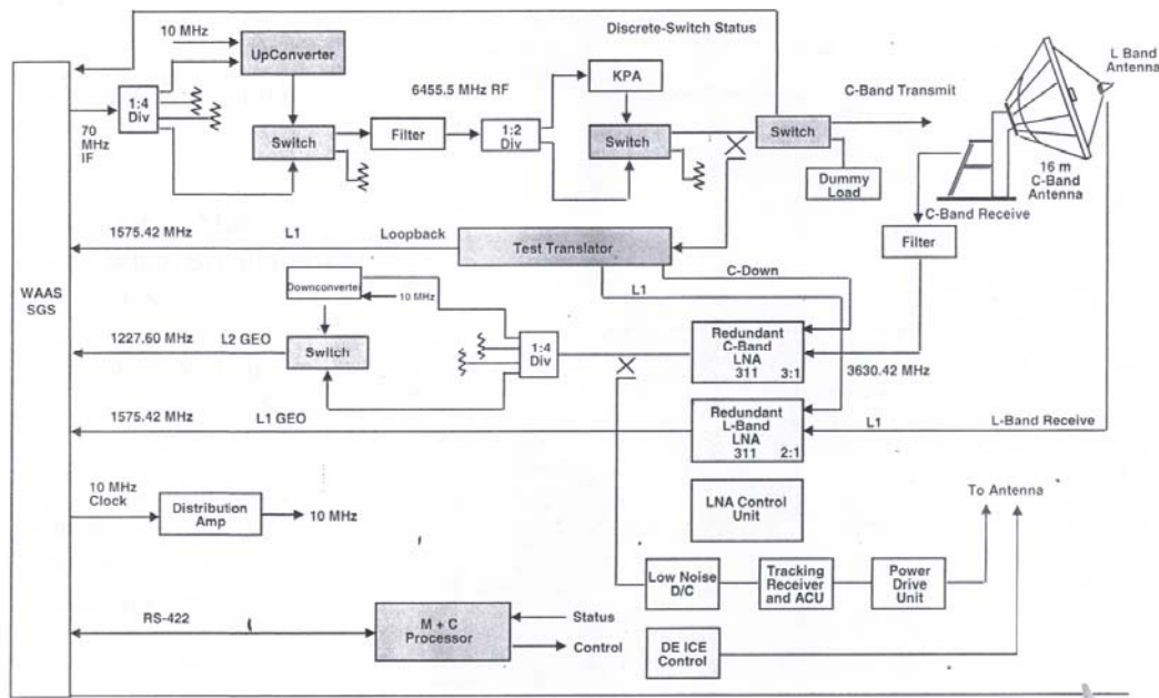
Figura 3.13. Diagrama de la circuitería del GUS para enlace de radio frecuencia.
