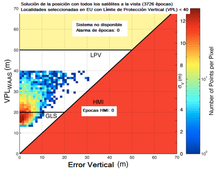
Figura 3.5. Carta triangular que muestra la distribución de los errores verticales de posición.
