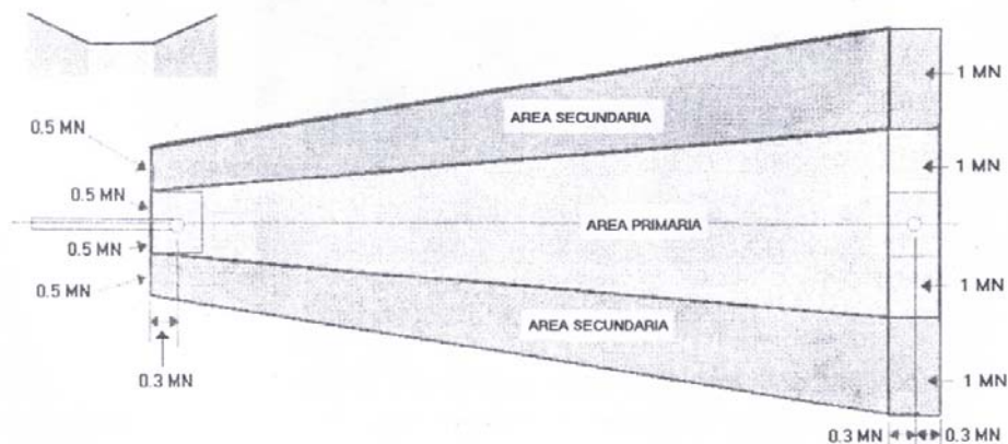
Figura 4.7. Áreas de protección para operación con aproximaciones GPS/WAAS/LAAS
