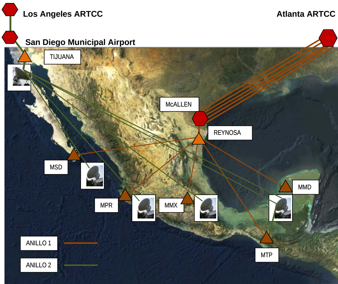
Figura 4.14. Anillos Metropolitanos de Interconexión con el Backbone de WAAS en E.U.
