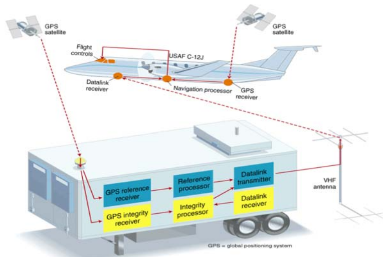
Figura 4.2. Diagrama de operación del sistema GPS/LAAS.
