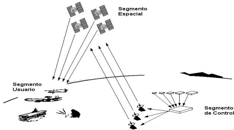
Figura 1.3. Sistema de posicionamiento satelital NAVSTAR.
