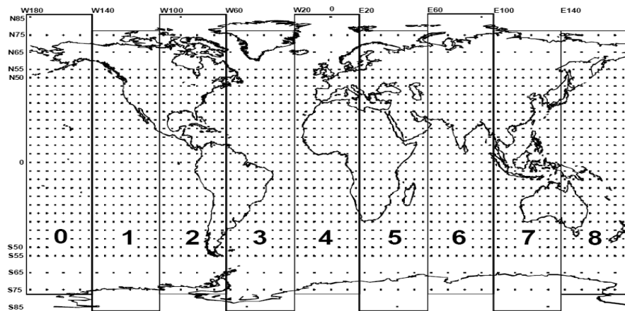
Figura 3.4. Red global de puntos ionosféricos predefinidos.
