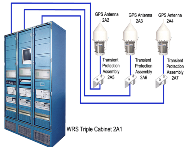
Figura 4.10. Elementos que conforman la estación de referencia con tres antenas GPS.
