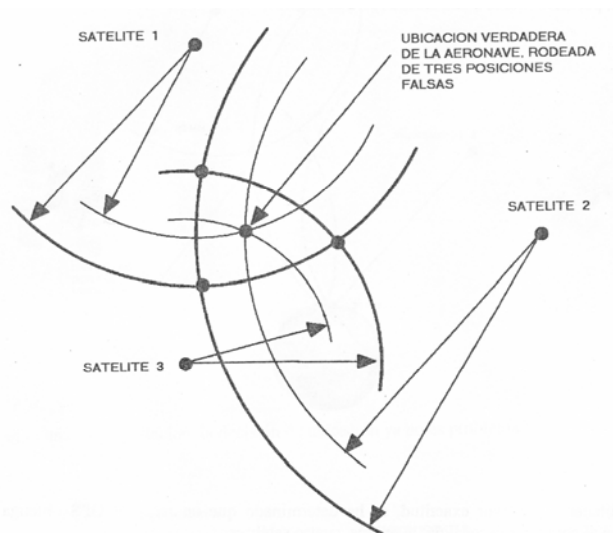
Figura 1.5. Ubicación verdadera de la aeronave, rodeada por tres posiciones falsas.
