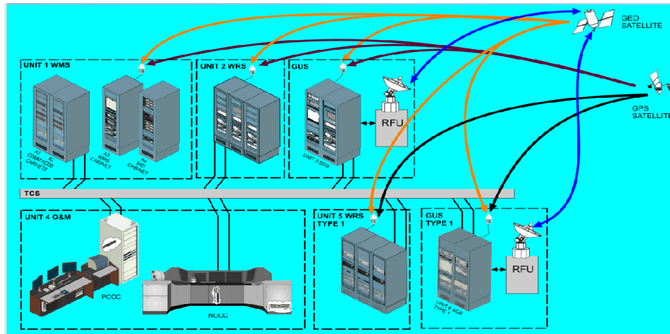
Figura 3.9. Interconexión entre los elementos del sistema WAAS.
