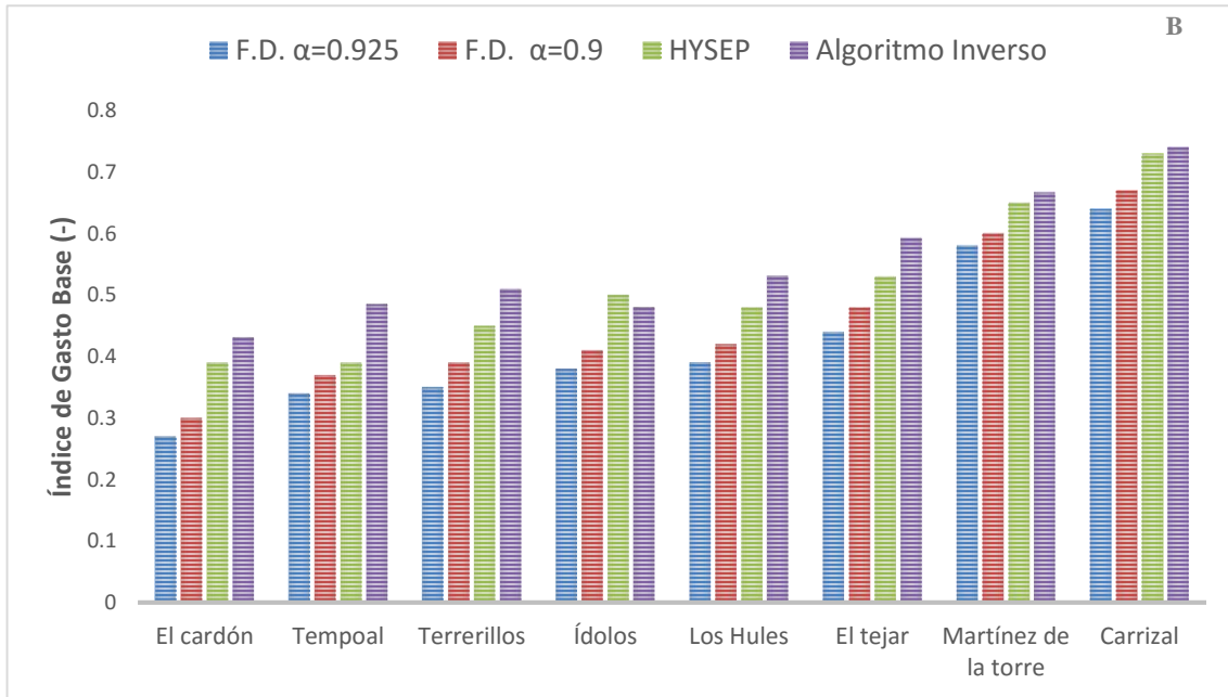
Ilustración 3.10 Recarga (A) e Índice de Gasto Base (B) estimados en las cuencas de la Sierra Madre Oriental
