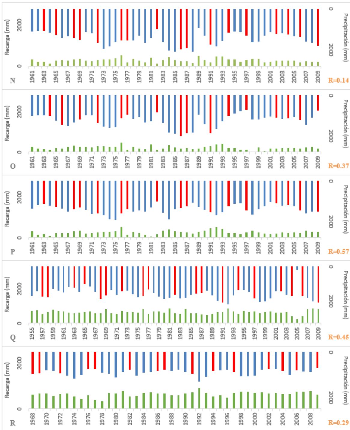
Ilustración 3.3 Recarga y precipitación para las cuencas de estudio Sierra Madre Oriental; (N) Los Hules, (O) El Cardón, (P) Terrerillos, (Q) Martínez de la Torre, (R) Carrizal.
