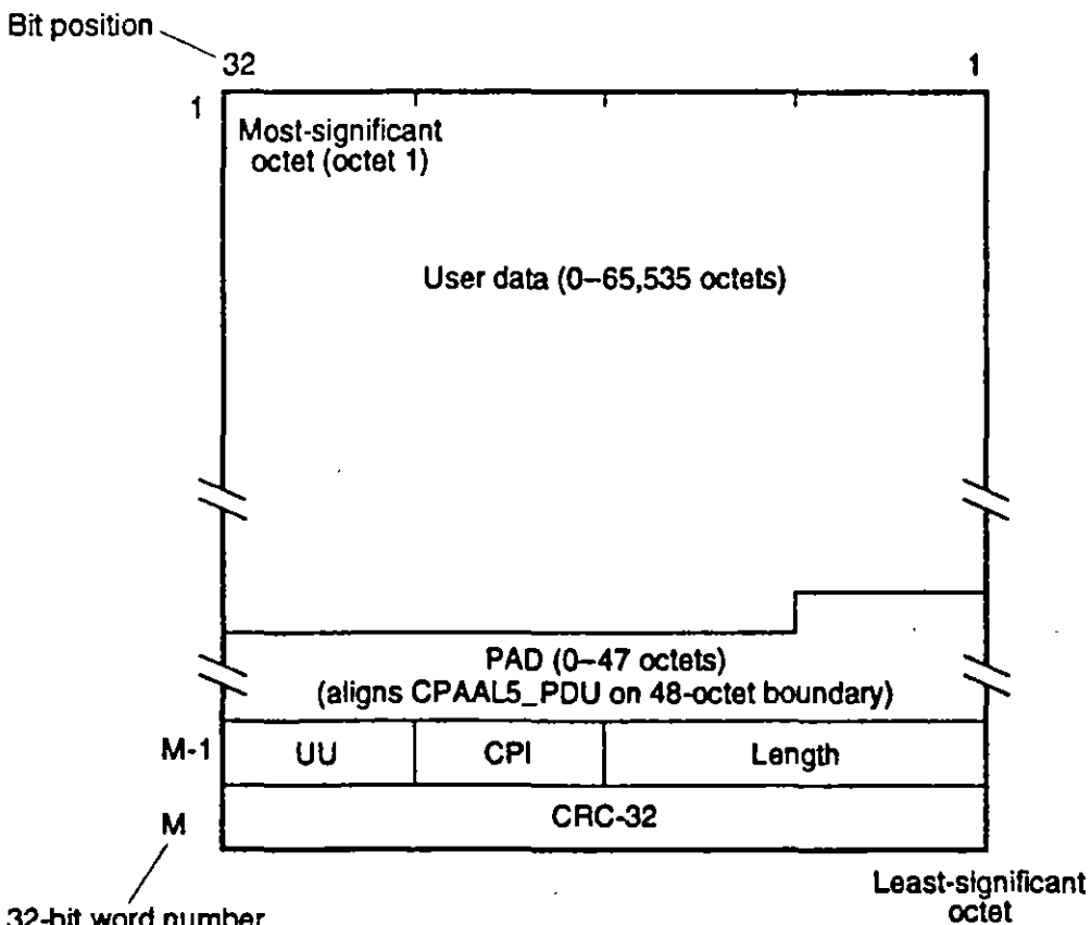
Figure 3.17 CPAAL5_PDU.
