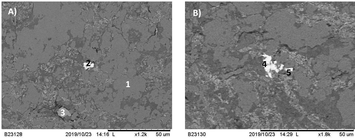
Fig. 5.2. A) Muestra tomada de la misma zona que la anterior, con matriz de la misma composición (1), en esta matriz se observa un cristal de monacita (2), y un cristal de ilmenita (3). B) En la matriz se aprecia otro cristal de monacita (4) y adyacente un zircón (5).
