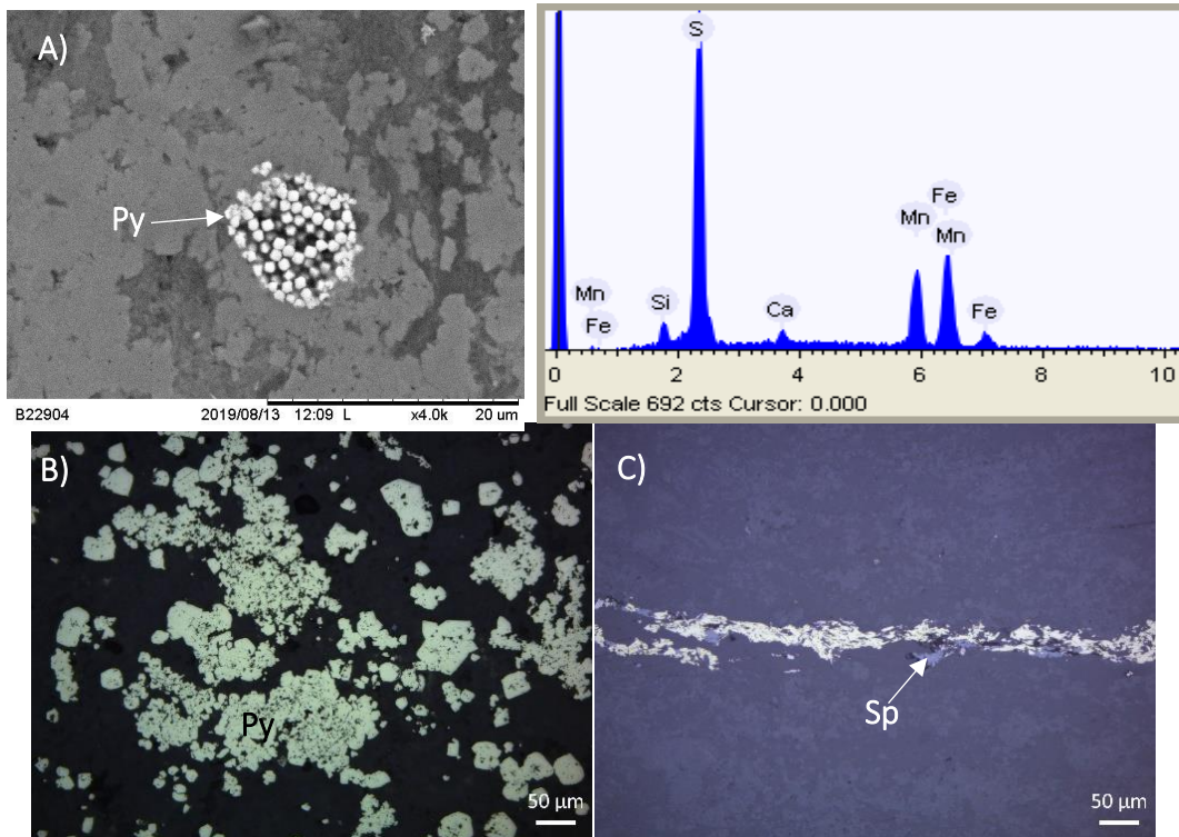
Fig. 5.14 Fotomicrografías de pirita. A) Framboides de pirita (Py). B) Pirita (Py) en cristales euhedrales y masivos. C) Vetilla de pirita con esfalerita (Sp).
