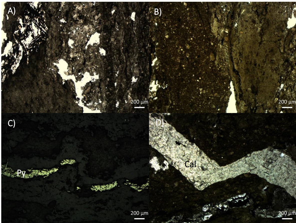
Fig. 3.8 Fotomicrografías de la muestra MOL-CMX-23 . A) Porosidad de la muestra. B) Cambio textural. C) Falla normal en vetilla de pirita. D) Deformación en vetilla de calcita.
