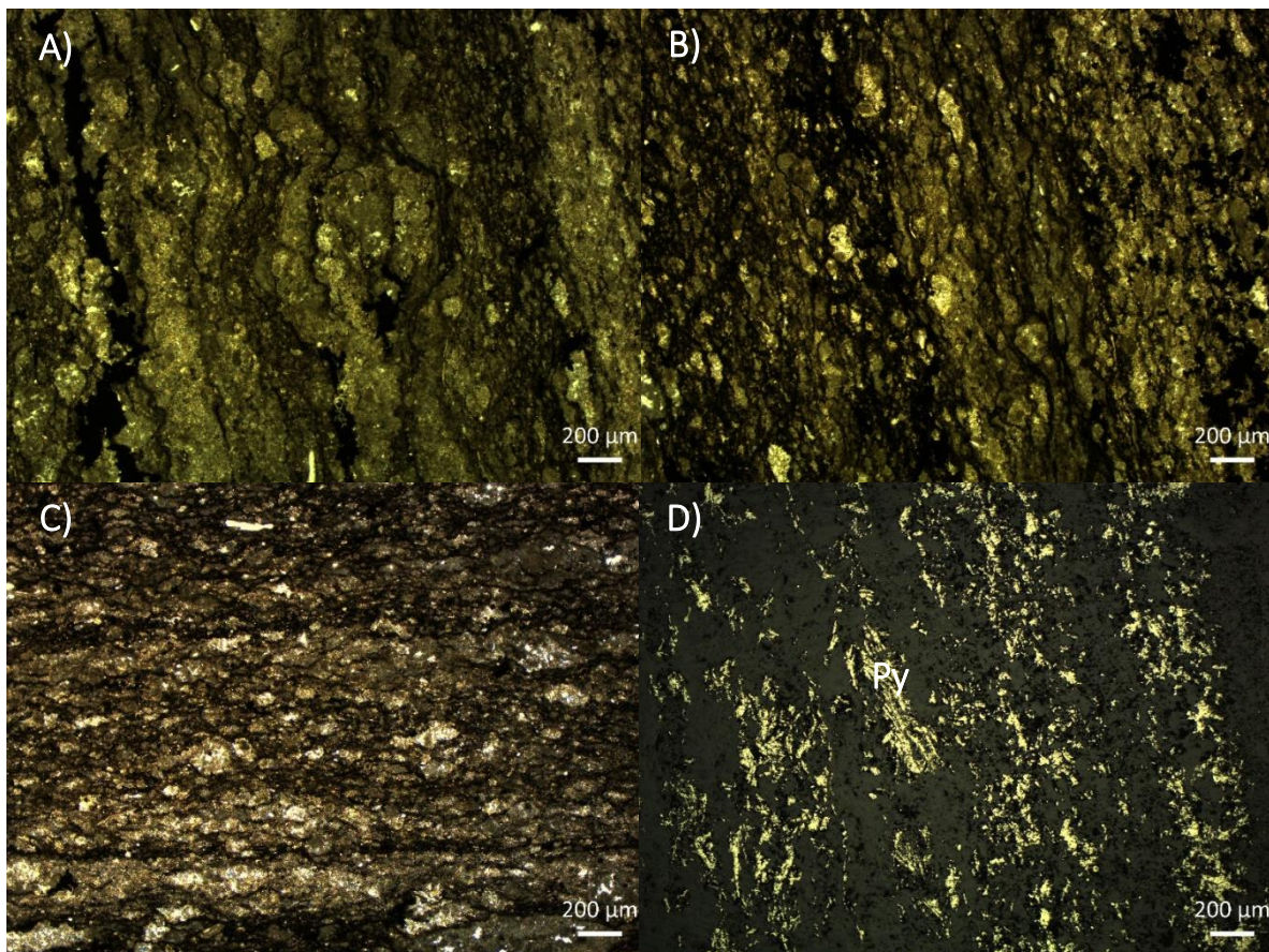
Fig. 3.5 Fotomicrografías de la muestra MOL-VII-15. A) Estructuras de carga. B) Laminación de la matriz. C) Cambios en la composición de la matriz. D) Marcasita tabular y acicular siendo reemplazada por pirita (Py).
