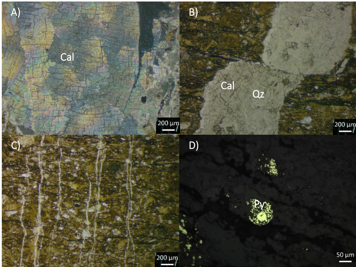
Fig. 3.26 Fotomicrografías de la muestra MOL-TAM-68. A) Fractura rellena de calcita (Cal), véase el crucero romboidal que muestra. B) Laminación de la matriz con una fractura rellena de cuarzo (Qz) y calcita (Cal) casi perpendicular a laminación, además de una falla. C) Matriz laminada con vetillas de calcita perpendiculares a ella. D) Framboides de pirita (Py) con y sin núcleo de pirita.
