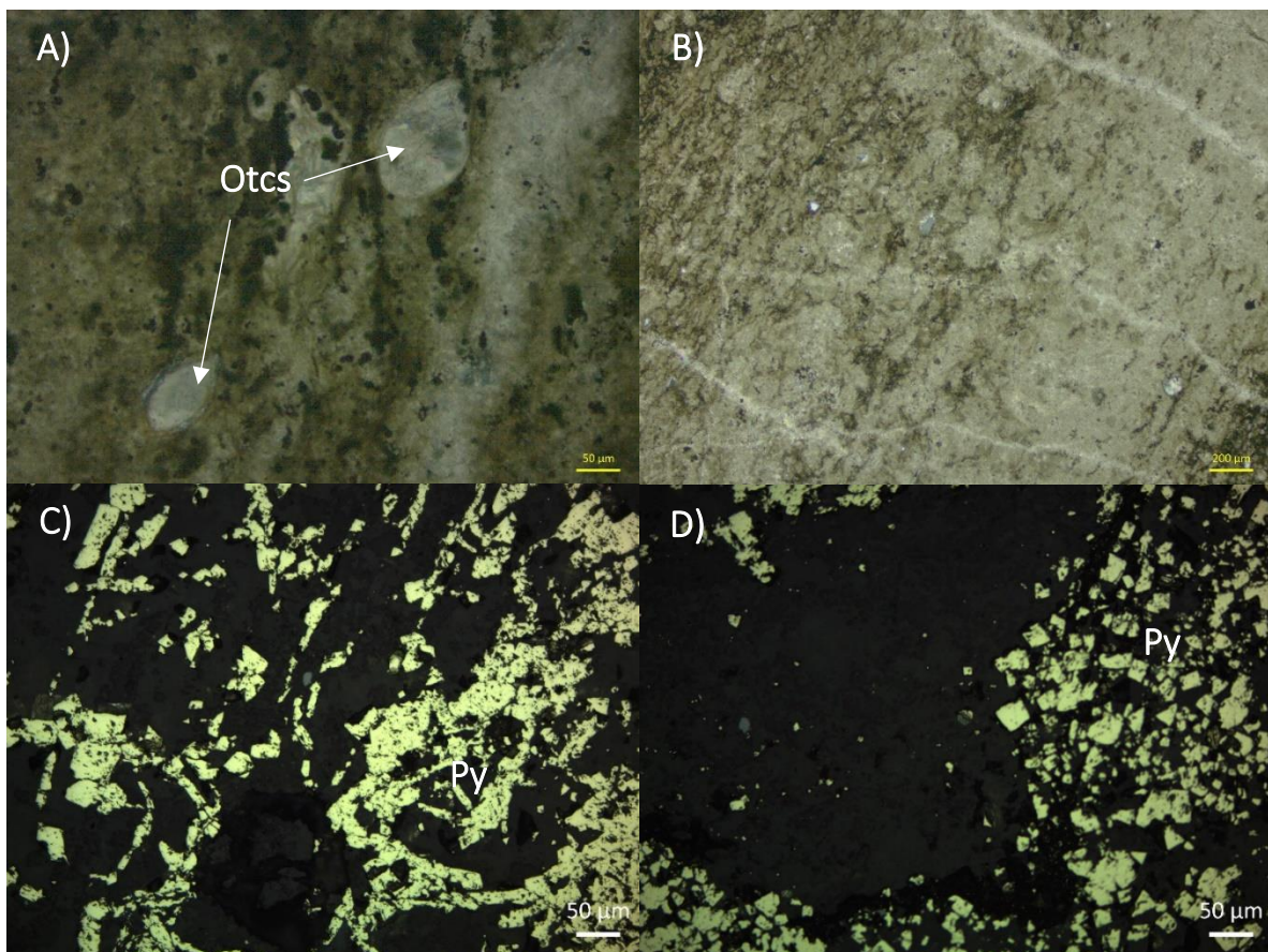
Fig. 3.17 Fotomicrografías de la muestra MOL-CMX-44. A) Ostrácodos (Otcs). B) Matriz carbonatada sin presencia de óxidos. C) Pirita (Py) reemplazando marcasita pseudobandeada. D) Pirita (Py) euhedral.
