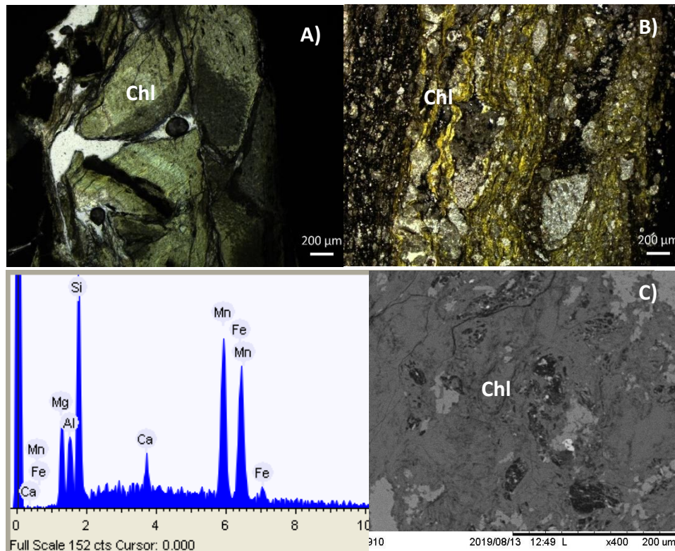
Fig. 6.5 Presencia de clorita en la zona del Bloque III y IV. A) Clorita en vetilla. B) Clorita en la matriz formando parte de la laminación. C) Micrografía y EDS de la clorita.
