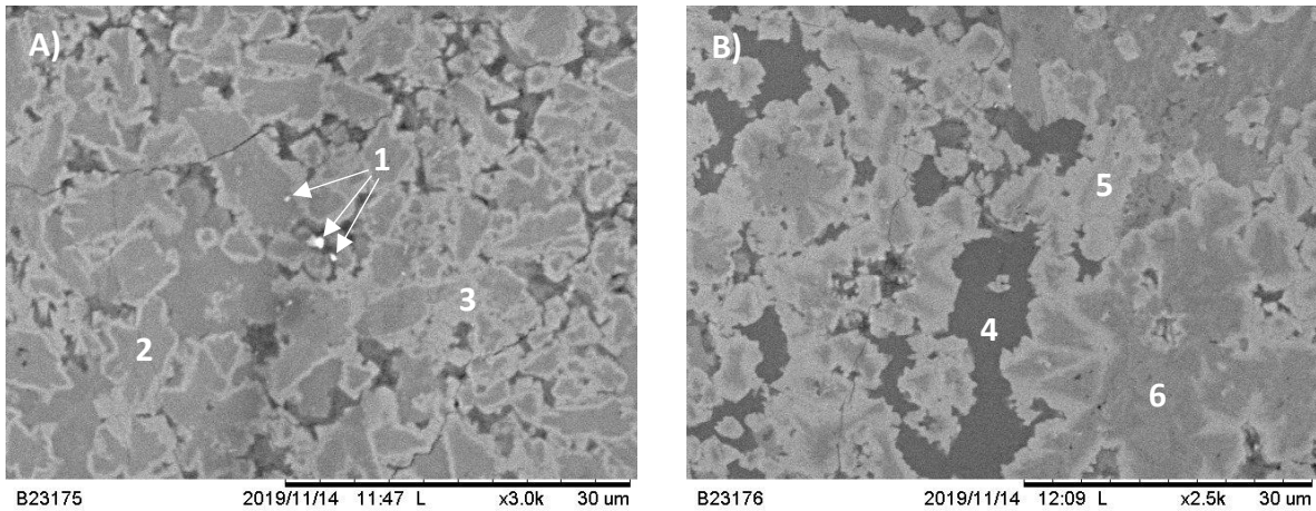
Fig. 5.9. A) Diseminado de microcristales de monacita (1) en una matriz que está conformada por calcita manganesífera (2) y calcita (3). B) Por otra parte tenemos una matriz conformada por abundante sílice (4), escaso manganeso (5) y calcita (6).
