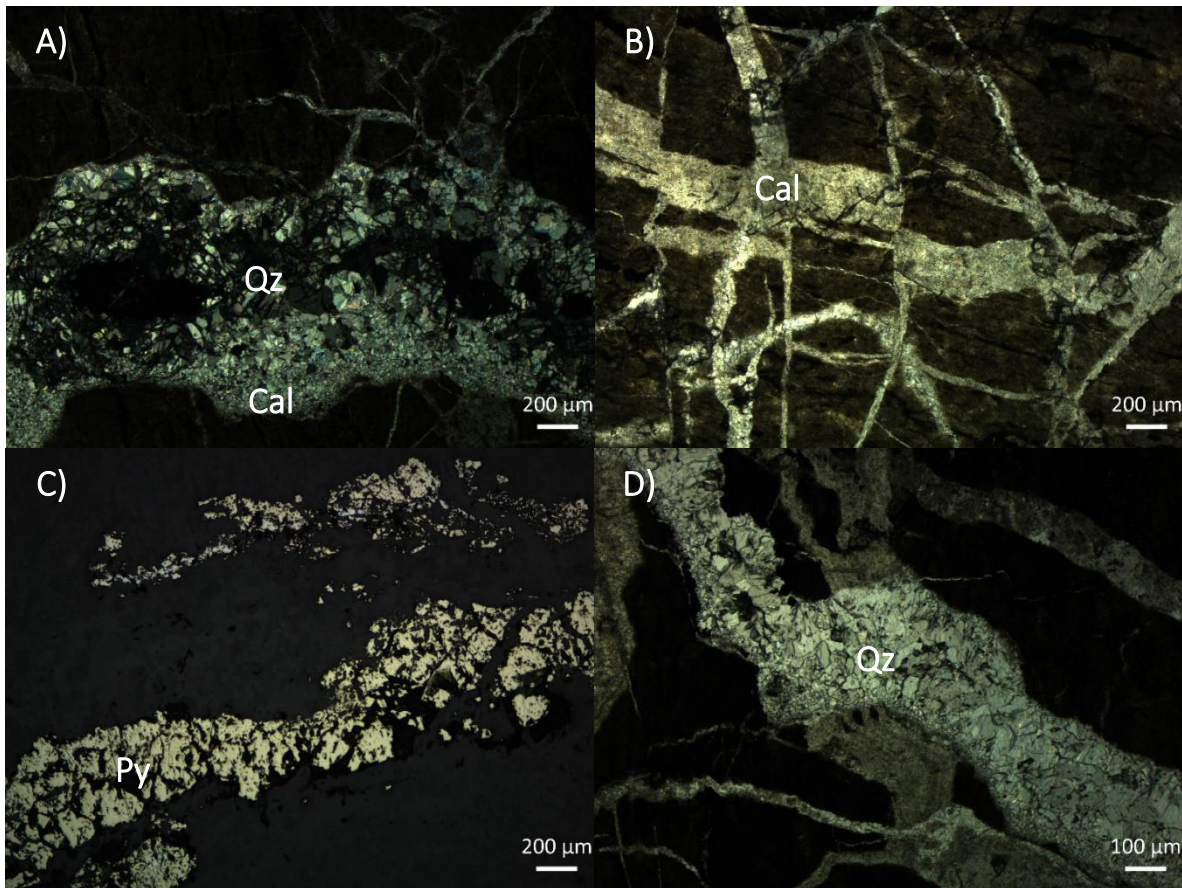
Fig. 3.9 Fotomicrografías de la muestra MOL-CMX-24. A) Vetilla rellena de calcita (Cal) en las orillas y cuarzo (Qz) al centro. B) Serie de fallas normales. C) Vetilla de pirita (Py). D) Vetilla de cuarzo (Qz).
