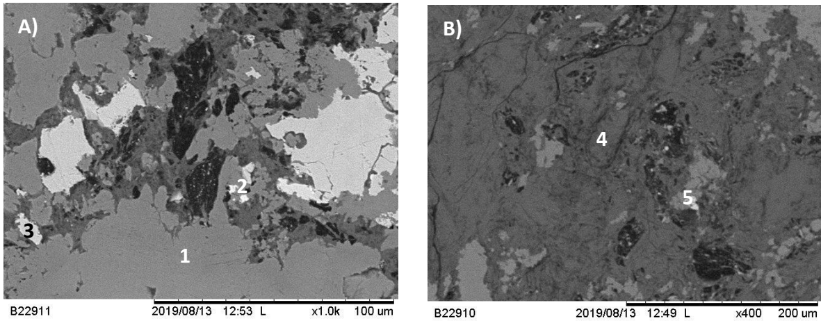
Fig. 5.1. A) Se observa una matriz clara (1) que presenta cristales de esfalerita (2) y de forma tabular una siegenita (3). B) En otra parte de la muestra se observa una matriz oscura (4) con zircón (5).
