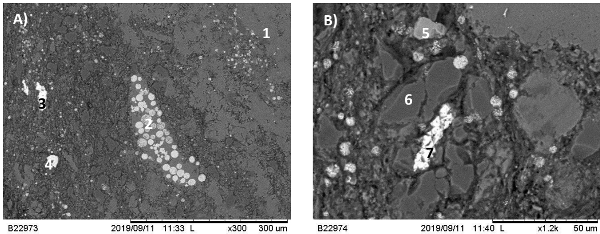
Fig. 5.6. A) Se aprecia una matriz clara totalmente carbonatada donde se observa un cristal de calcita (1), framboides de pirita (2), esfalerita (3) y zircón (4). B) En esta foto más detallada se observa un cristal de anatasa (5), un cristal anedral de cuarzo (6) y una esfalerita tabular (7).
