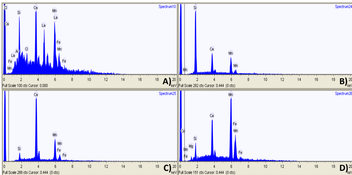
Fig. 5.9. A) Diseminado de microcristales de monacita (1) en una matriz que está conformada por calcita manganesífera (2) y calcita (3). B) Por otra parte tenemos una matriz conformada por abundante sílice (4), escaso manganeso (5) y calcita (6).
