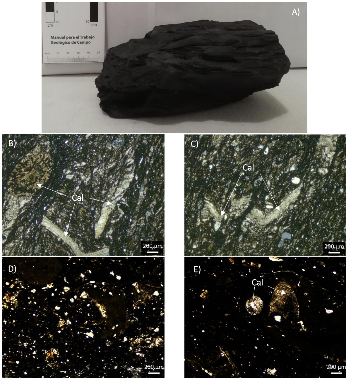
Fig. 5.7 Muestra de mano y fotomicrografías de la Formación Santiago. A) Limolita calcárea de la Formación Santiago, se aprecia laminada y ligeramente plegada. B) y C) Matriz de una limolita, podemos observar que presenta fragmentos plegados y una matriz un poco clara. D) y E) Matriz de una limolita que estuvo en contacto con un dique andesítico, hay presencia de fósiles y la matriz está más oscura, probablemente el dique quemó la materia orgánica de esta limolita.
