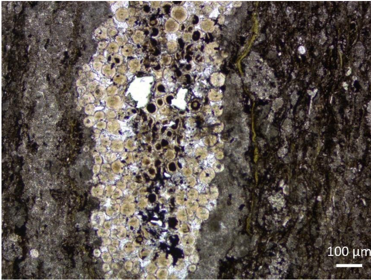
Fig. 5.26 Asociación de microfacies grainstone de ooides . Nótese que los ooides están micritizados ya que no muestran una estructura interna, están bien clasificados.
