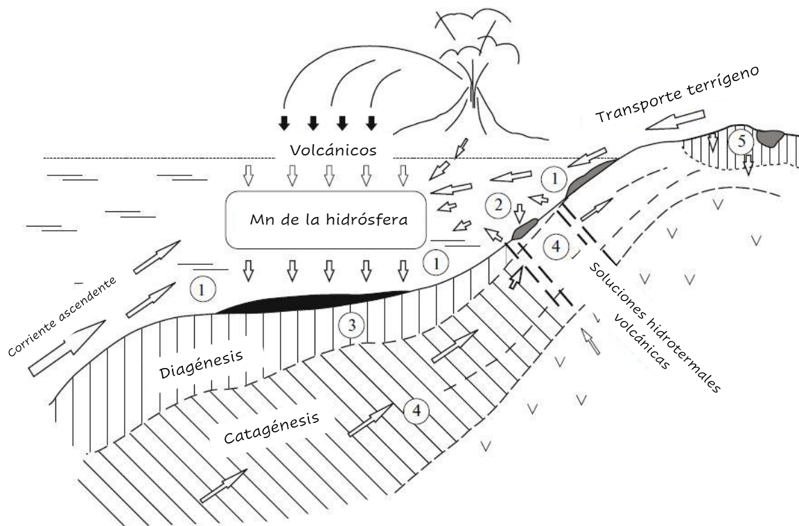
Fig. 2.2 Modelo para la formación de yacimientos de manganeso y sus principales fuentes. (1) Sedimentario; (2) Hidrotermal (Vulcanogénico, exhalativo-sedimentario); (3) Diagenético; (4) Catagénico (metasomático) y (5) Supergénico (costras erosionadas). Tomado de Kuleshov (2011)
