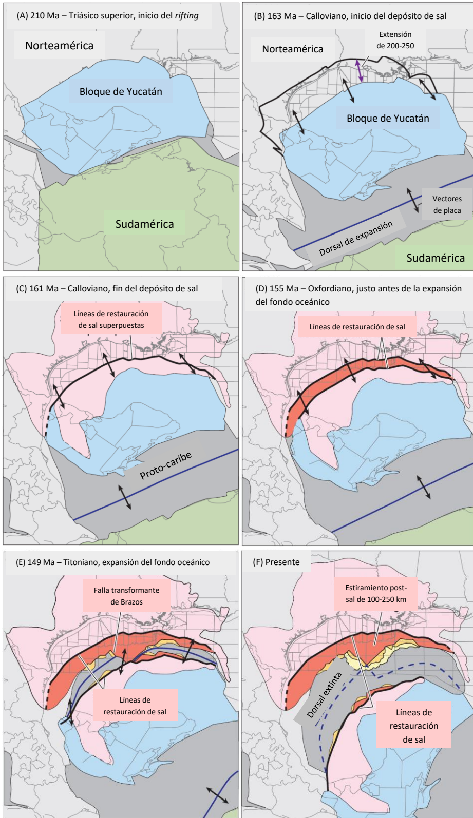
Fig. 4.1 Reconstrucción secuencial de las placas tectónicas tras la ruptura progresiva de Pangea. Modificado de Hudec et al. (2013).
