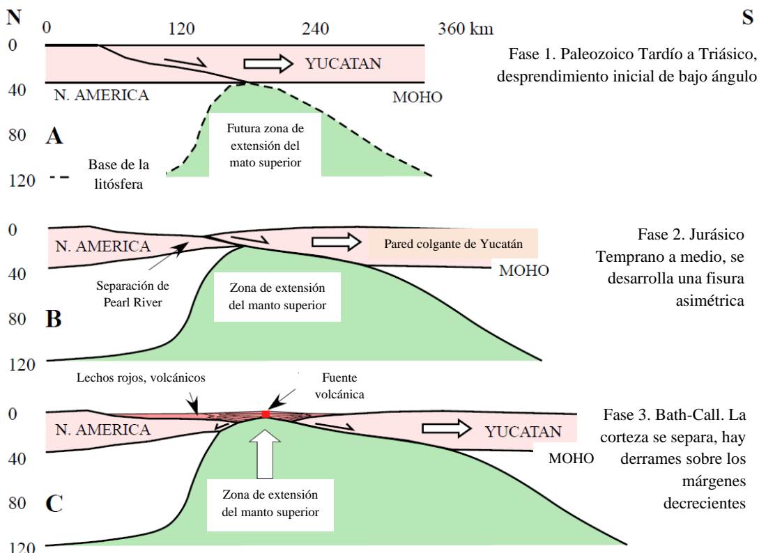
Fig. 4.5 A-C. Secciones transversales que muestran la evolución del Golfo de México desde el inicio del rifting hasta la formación de corteza proto-oceánica. Tomado de Pindell y Kennan (2007)
