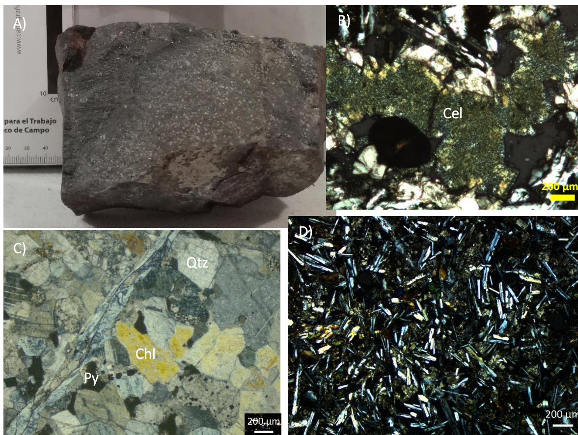
Fig. 5.8 Fotomicrografías de algunos intrusivos presentes en la mina Tetzintla. A) Monzonita con cristales visibles de cuarzo y calcita. B) Presencia de celadonita en uno de los intrusivos. C) Intrusivo cloritizado. D) Matriz con textura intersertal e intergranular.
