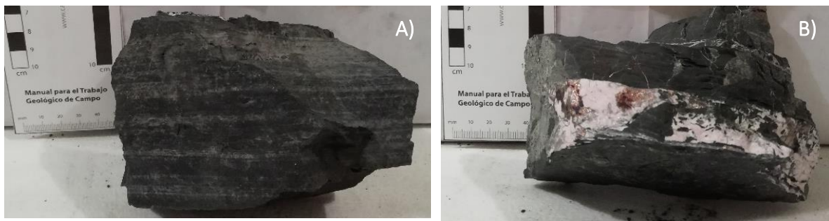
Fig. 5.9 Muestras representativas de la roca encajonante. A) Wackstone laminada, se observan láminas de pirita intercaladas con la matriz de carbonatos. B) Wackstone con vetilla de rodocrosita y pirrotita, la matriz se encuentra laminada.
