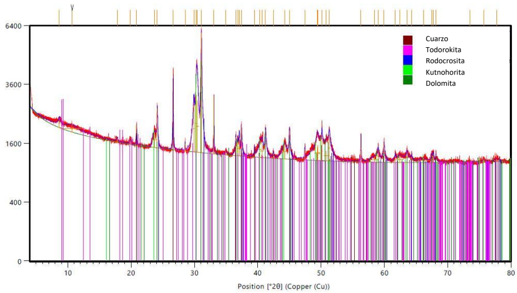
Fig. 5.2 Difractograma de la muestra MOL-IV-16
