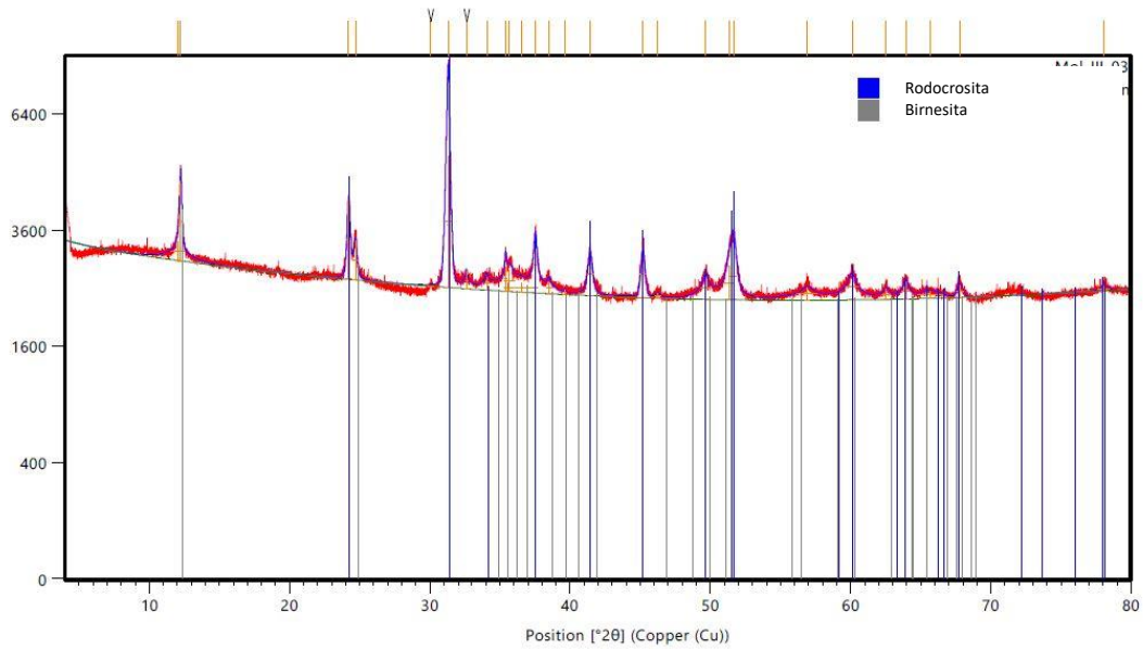
Fig. 5.1 Difractograma de la muestra MOL-III-03
