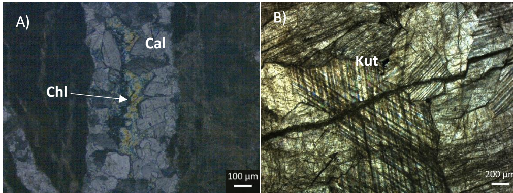
Fig. 5.18 Fotomicrografías de carbonatos. A) Veta de calcita (Cal), kutnohorita (Kut) con clorita (Chl) en el centro. B) Veta de calcita (Cal) y kutnohorita (Kut).
