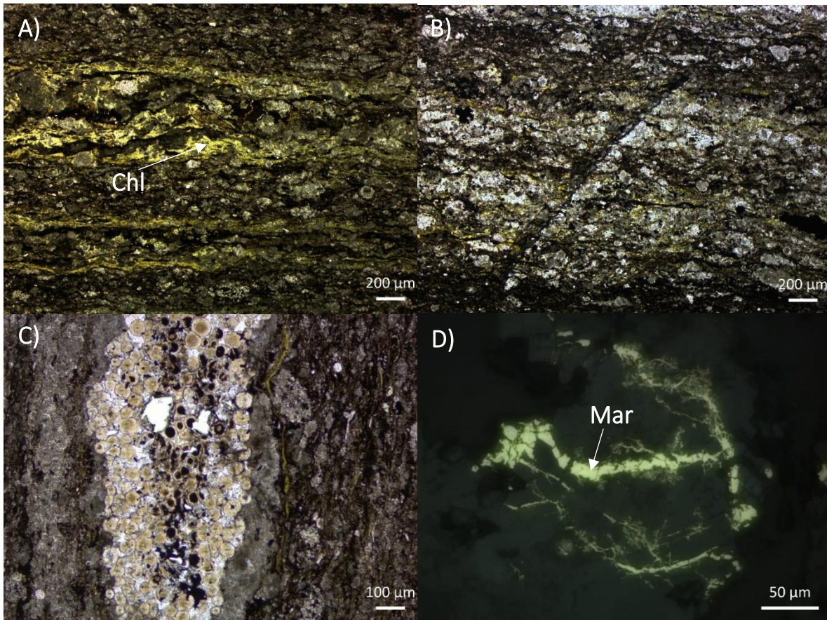
Fig. 3.4 Fotomicrografías de la muestra MOL-IV-10. A) Matriz laminada intercalada con clorita (Chl) y óxidos. B) Falla normal. C) Lente de un grainstone de ooides. D) Marcasita (Mar) siendo reemplazada por pirita.
