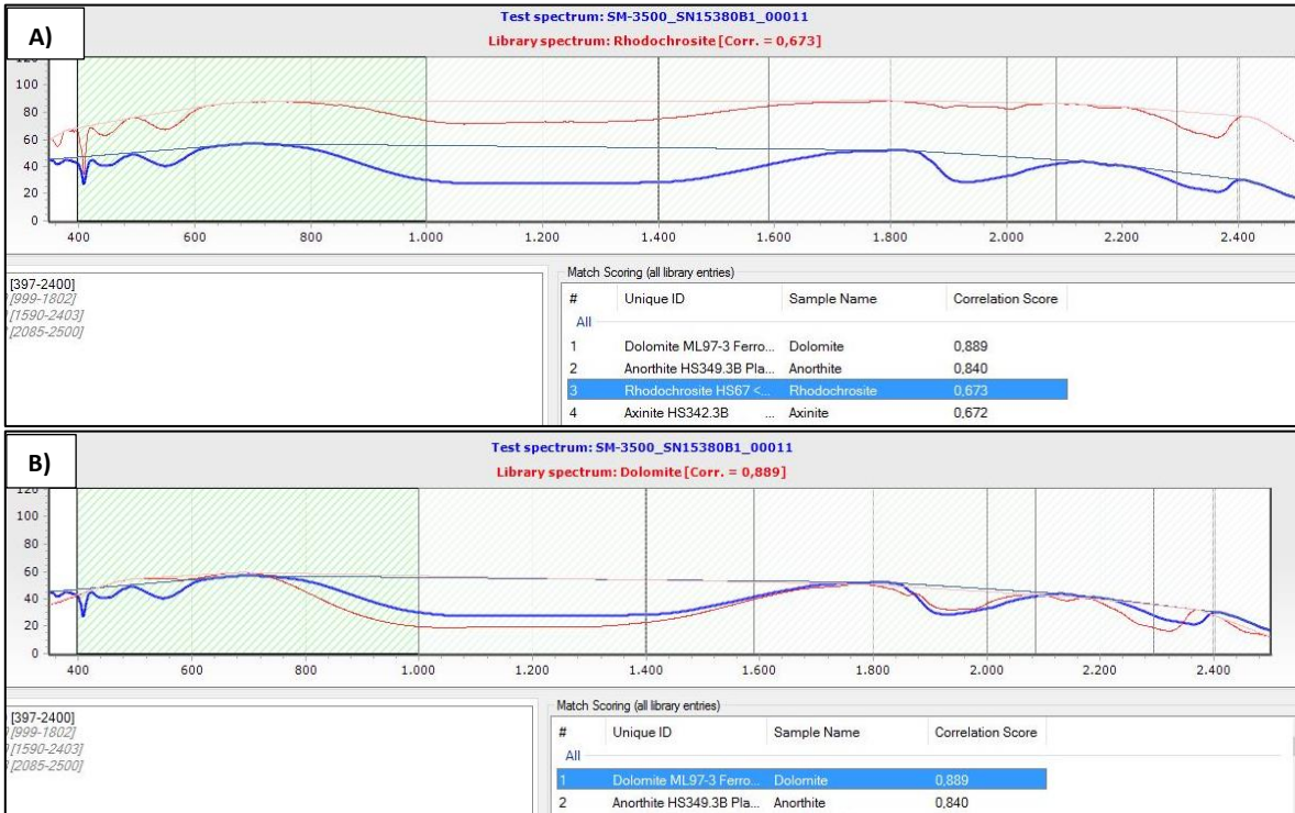
Fig. 3.1. Espectros infrarrojos de la muestra MOL-III-30. A) Rodocrosita. B) Dolomita
