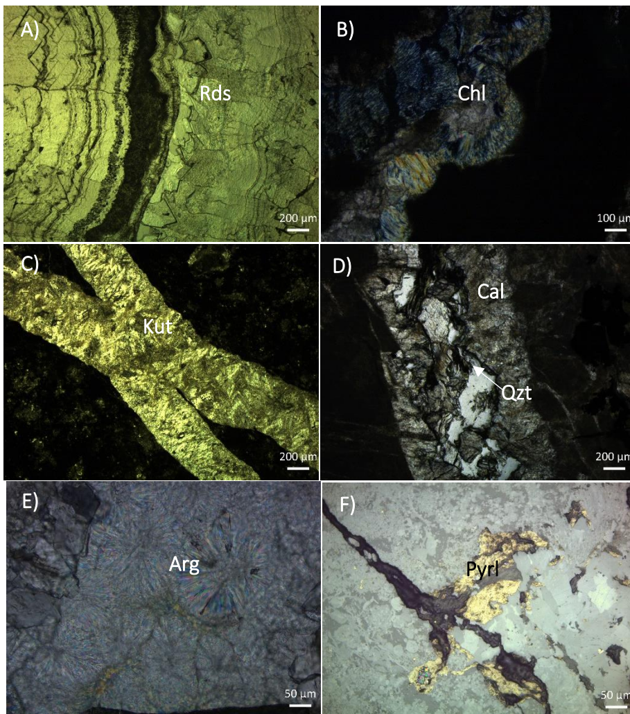
Fig. 5.12 Mineralogía del yacimiento. A) Rodocrosita (Rds) botroidal relleno una fractura, presenta una transición a kutnohorita. B) Vetilla de clorita (Chl) con nicoles cruzados. C) Vetilla de Kutnohorita (Kut). D) Vetilla de calcita (Cal) con cuarzo (Qzt) en el centro. E) Aragonito (Arg) asociado con calcita en vetilla. F) Pirolusita (PyrI) amorfa.
