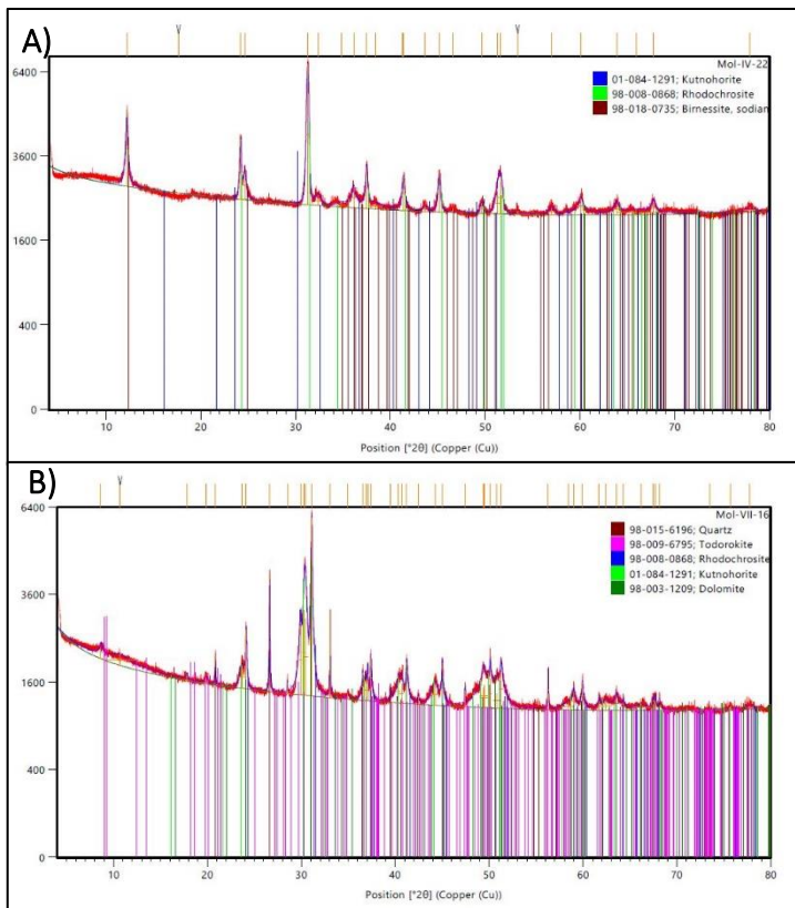
Fig. 5.19 Difractogramas de óxidos y carbonatos. A) Difractograma de una caliza de alta ley que contiene kutnohorita, rodocrosita y birnesita. B) El difractograma muestra a una caliza de baja ley que contiene cuarzo, todorokita, rodocrosita, kutnohorita y dolomita.
