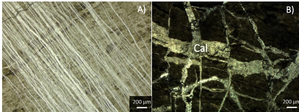
Fig. 5.22 Fotomicrografías de la unidad de cataclasita (Capa A). A) Wackstone con vetilleo de calcita. B) Mudstone con serie de fallas normales, las fallas están rellenas de calcita (Cal).
