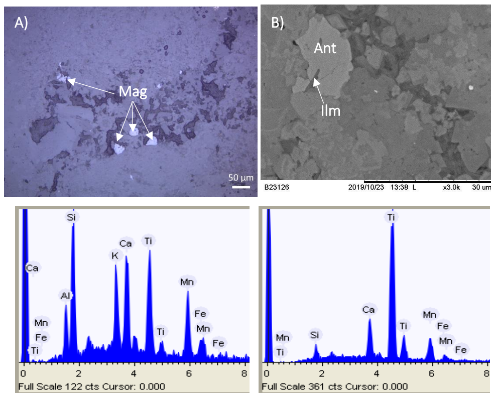
Fig. 5.17 Fotomicrografías y espectros EDS de óxidos. A) Cristales de magnetita (Mag) en matriz carbonatada. B) Cristal de anatasa (Ant) atravesado por un cristal tabular de ilmenita (Ilm).
