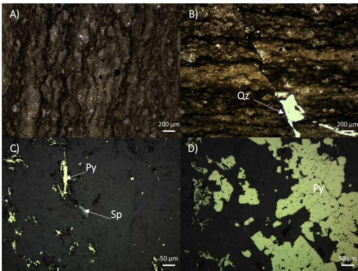
Fig. 3.11 Fotomicrografías de la muestra MOL-VII-29. A) Matriz carbonatada con finas laminaciones de óxidos de manganeso. B) Falla normal, con vetilla de cuarzo (Qz). C) Marcasita tabular reemplazada por pirita (Py) y esfalerita anhedral (Sp). D) Detalle de nódulo de pirita (Py) la pirita es euhedral, además, reemplazando marcasita.
