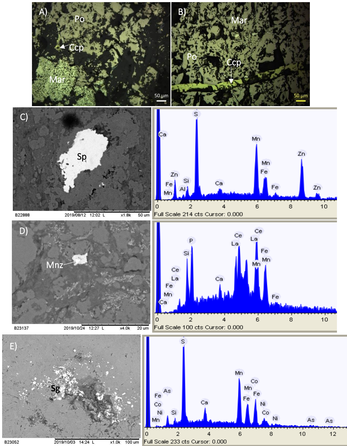
Fig. 5.13 Mineralogía de metálicos del yacimiento. A) Nódulo de pirita que contiene pirrotita (Po), calcopirita (Ccp), marcasita (Mar) y otros sulfuros. B) Lente de pirrotita (Po) con una microvetilla de calcopirita (Ccp). C) Esfalerita (Sp). D) Monacita (Mnz). E) Conjunto de sulfuros de Co y Ni, posible siegenita (Sg) con porcentajes de As (4% modal).
