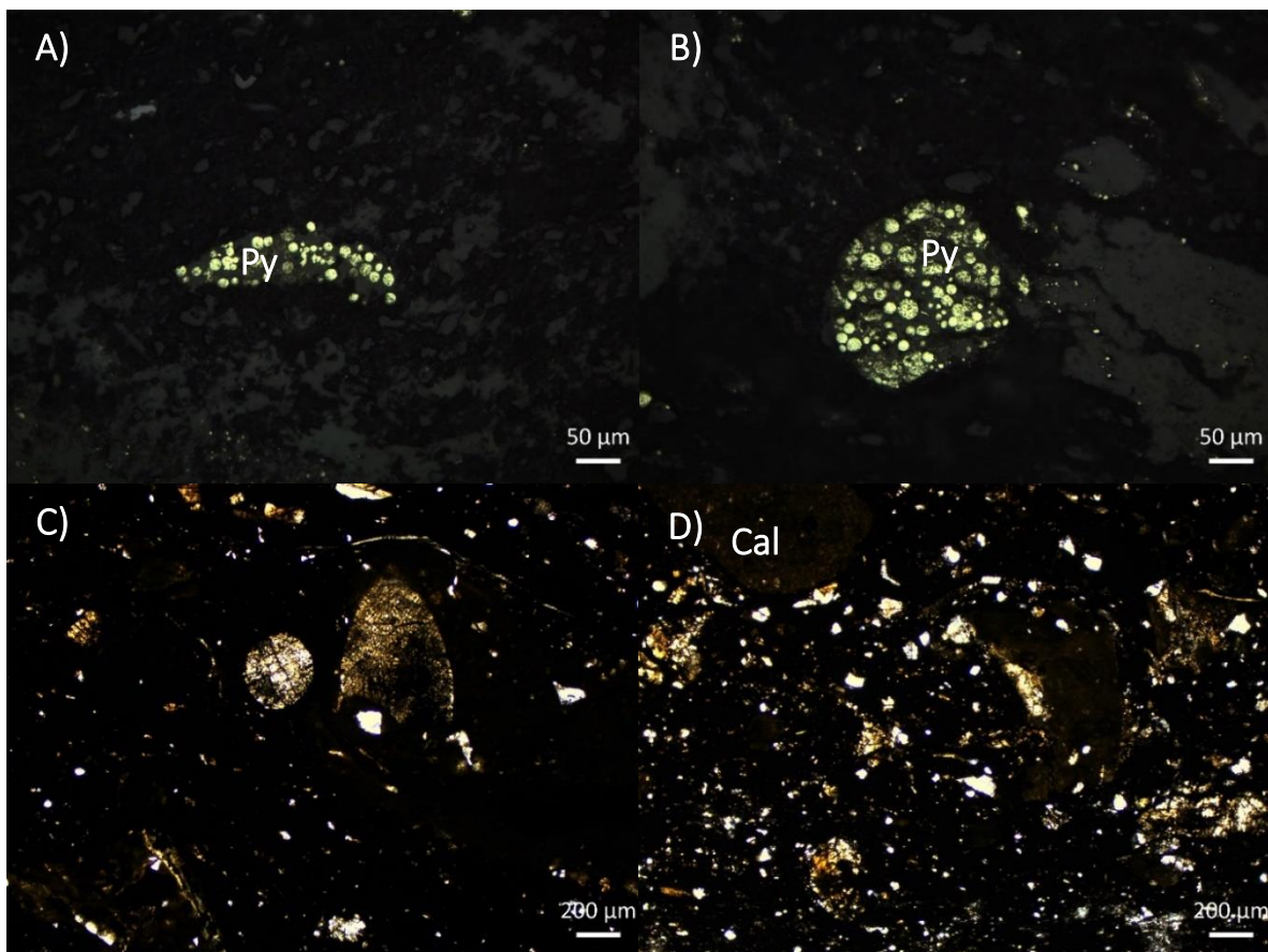
Fig. 3.13 Fotomicrografías de la muestra MOL-CMX-33. A) y B) Framboides de pirita. C) Fósil no identificado. D) Matriz de la roca con mucha materia orgánica con cristales de calcita (Cal) de gran tamaño (aprox. 600 \mu\text{m} ).
