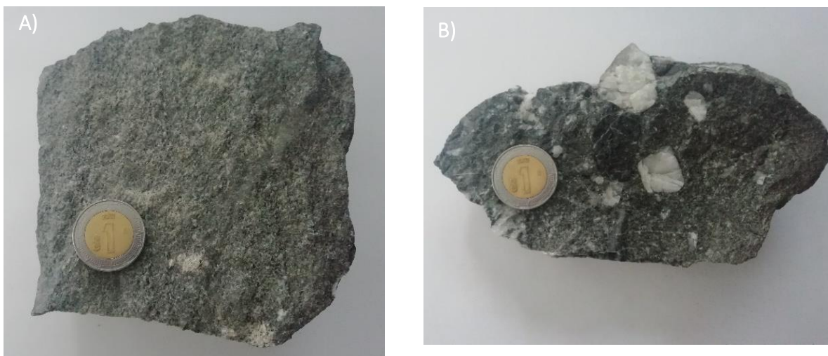
Fig. 5.4 Rocas de la Formación Huayacocotla. A) Arenisca de grano fino. B) Ortoconglomerado polimíctico, nótese los diferentes tamaños del cuarzo.
