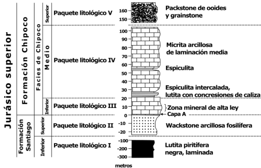
Fig. 4.3 Estratigrafía de la zona de Tetzintla. Tomado de Okita (1992)
