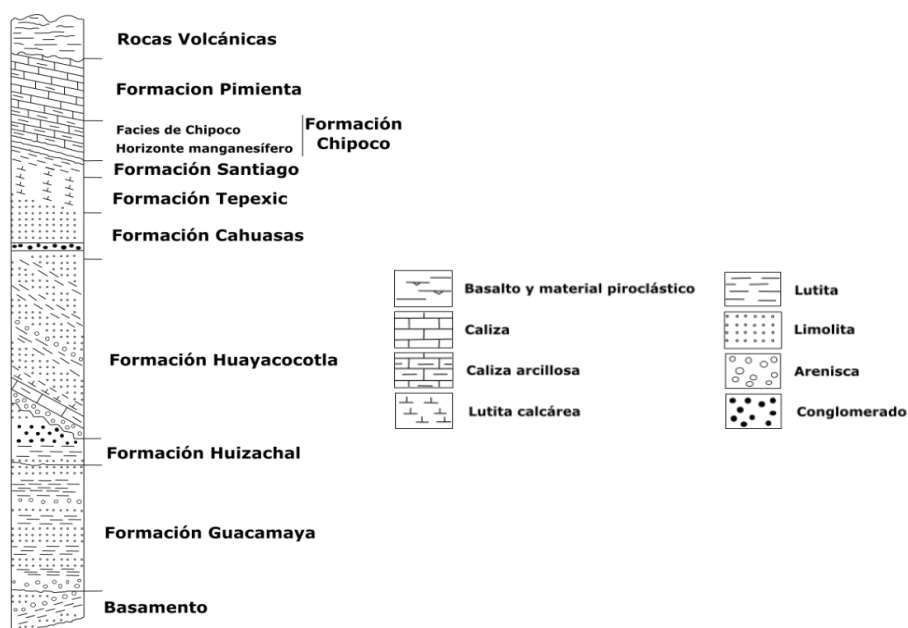
Fig. 4.2 Estratigrafía regional del Distrito manganesífero de Molango. Tomado de Okita (1992).
