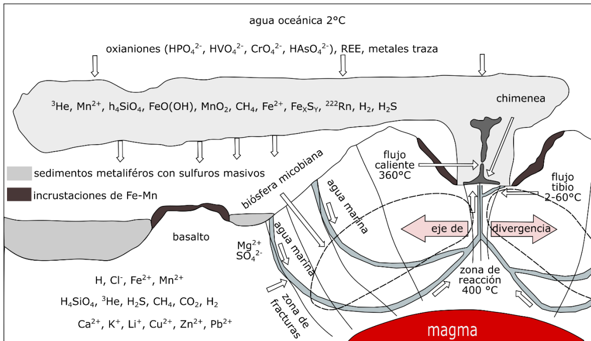
Fig. 2.3 Modelo para un sistema hidrotermal en una dorsal oceánica. Tomado de Pantoja-Alor y Gómez-Caballero (2004).
