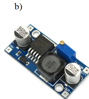
Figura 4.30: a) Diagrama eléctrico del convertidor Buck con el LM2596 b) PCB del convertidor
