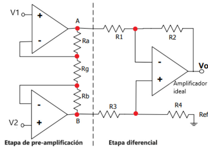
Figura 4.8: Amplificador de instrumentación basado en 3 Amplificadores operacionales.
