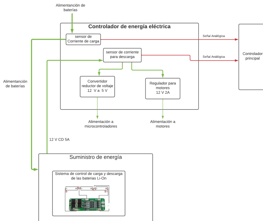
Figura 4.28: Diagrama de bloques del suministro y control de energía eléctrica.
