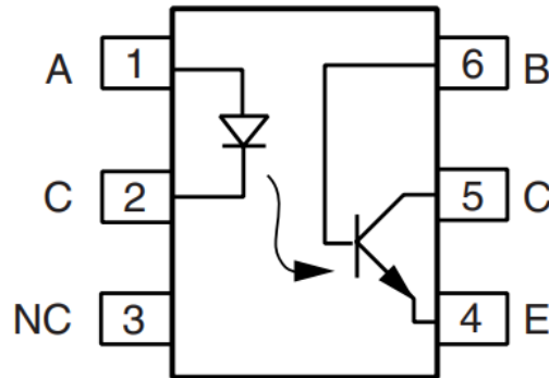
Figura 4.18: Opto-acoplador basado en un foto-transistor. Imagen recuperada de [9].
