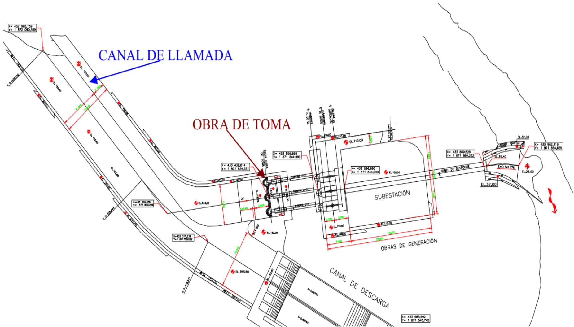
Figura 3.6: PLANTA DE LA LOCALIZACIÓN DE LA OBRA DE TOMA Y CANAL DE LLAMADA PARA LA OBRA DE GENERACIÓN,
