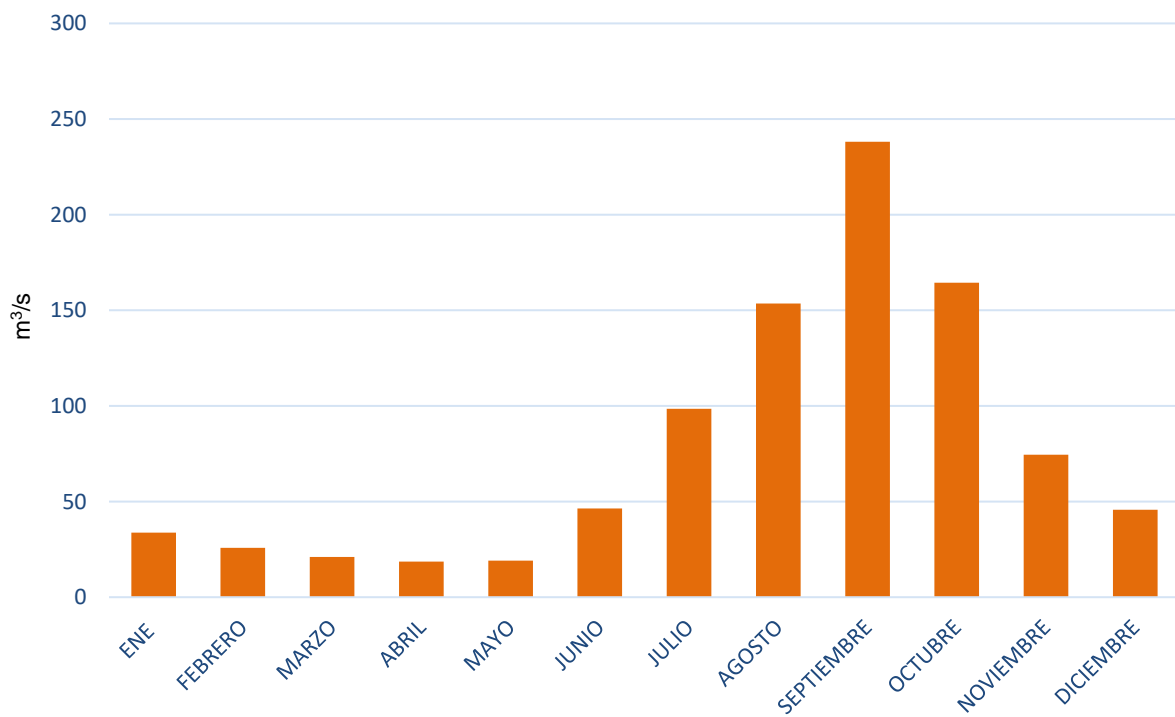
Figura 4.6: GASTOS MEDIOS MENSUALES DE LA E.H. EL PUENTE (1953 – 2007)
