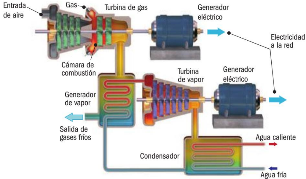
Figura 1.2: ESQUEMA DE UNA CENTRAL TERMOELÉCTRICA DE CICLO COMBINADO
