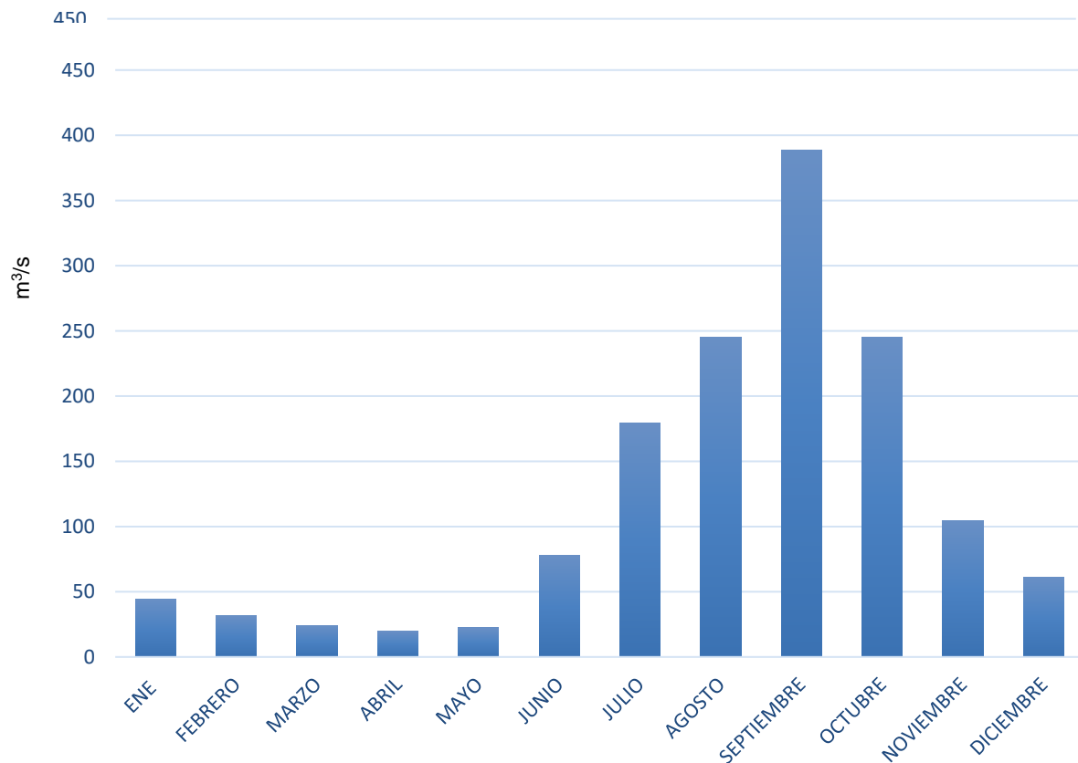
Figura 4.4: GASTOS MEDIOS MENSUALES DE LA E.H. LA PAROTA (1962 – 2003)
