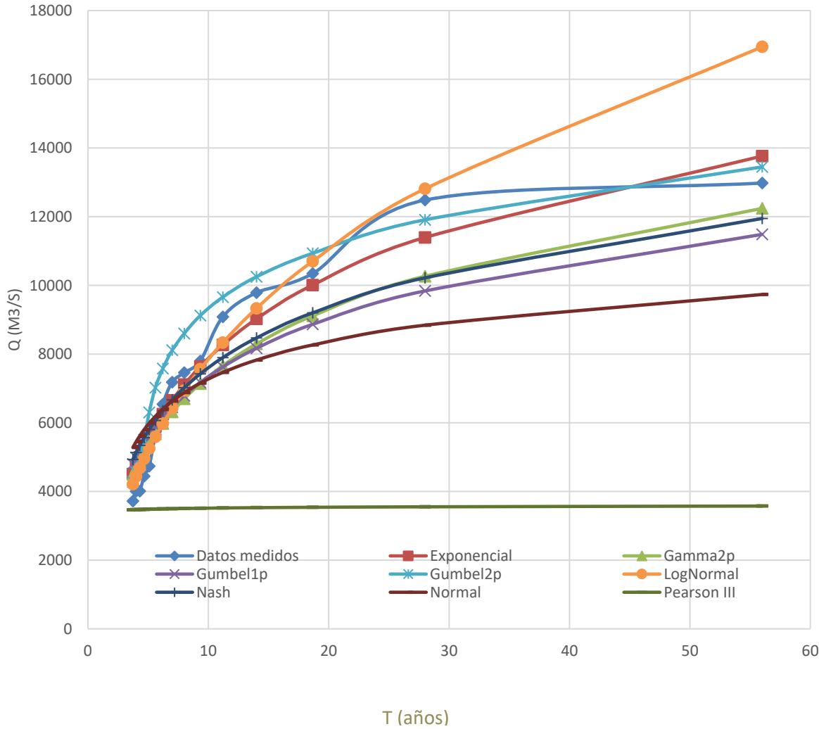
Figura 4.8: GRÁFICO CON LAS DIFERENTES DISTRIBUCIONES DE PROBABILIDAD ASOCIADOS A LOS GASTOS MÁXIMOS EN LAS ESTACIONES HIDROMÉTRICAS DE LA PAROTA, EL PUENTE Y AGUA SALADA
