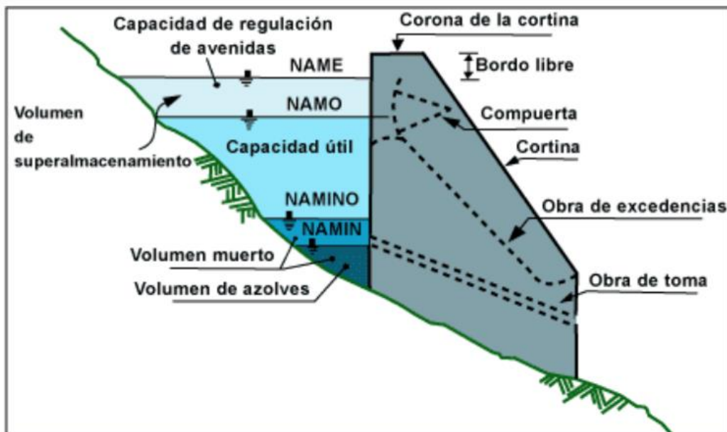
Figura 2.9: PRINCIPALES COMPONENTES DE UN VASO DE ALMACENAMIENTO
