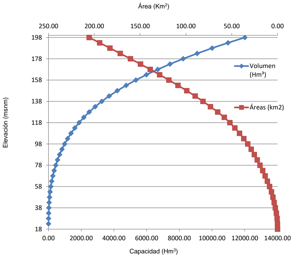
Figura 4.14: CURVA ELEVACIONES – ÁREAS – CAPACIDADES DEL EMBALSE CORRESPONDIENTE AL P.H. LA PAROTA
