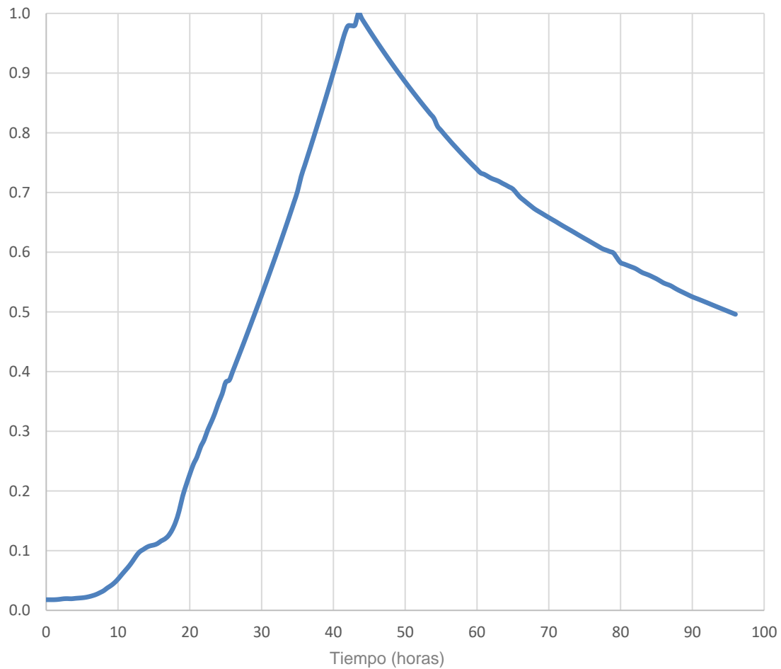
Figura 4.9: HIDROGRAMA UNITARIO DEL SITIO DEL P.H. LA PAROTA CON LOS REGISTROS DE LAS E.H. AGUA SALADA Y EL PUENTE
