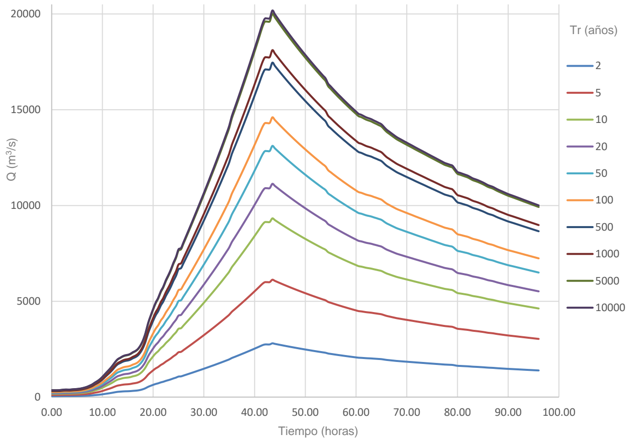
Figura 4.10: HIDROGRAMAS DE DISEÑO CORRESPONDIENTES A CADA PERIODO DE RETORNO DE LA DISTRIBUCION DE PROBABILIDAD DOBLE GUMBEL PARA EL SITIO DEL P.H. LA PAROTA
