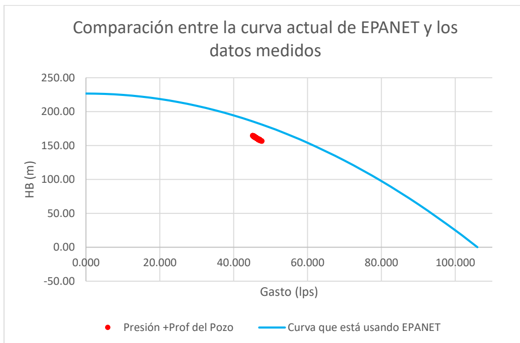
Gráfica 12 Comparación entre la curva actual de EPANET y los Datos medidos. Pozo BJ07 Miraflores
