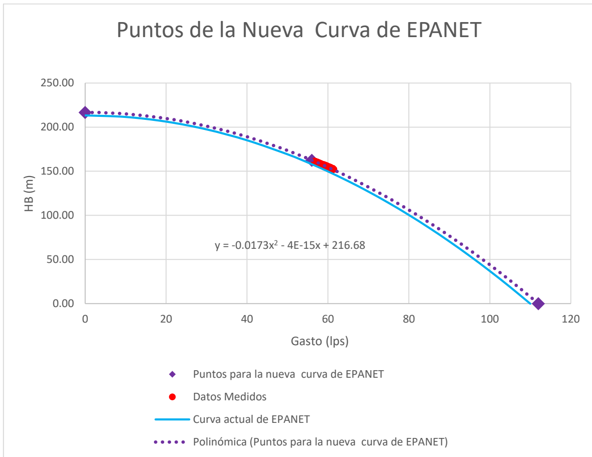
Gráfica 20 Curva nueva para EPANET. Pozo BJ23 en La Huerta
