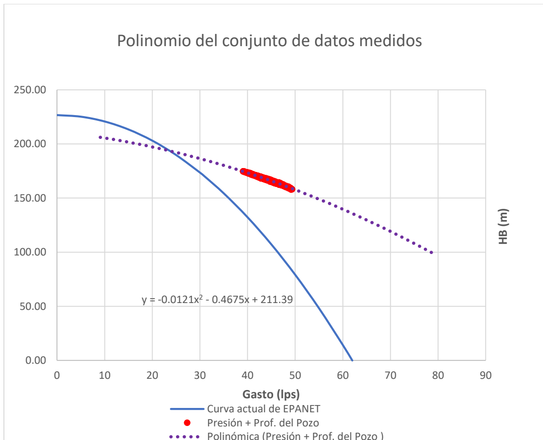
Gráfica 14 Curva polinómica y polinomio del conjunto de datos. Pozo BJ06 en Jardín Bombo
