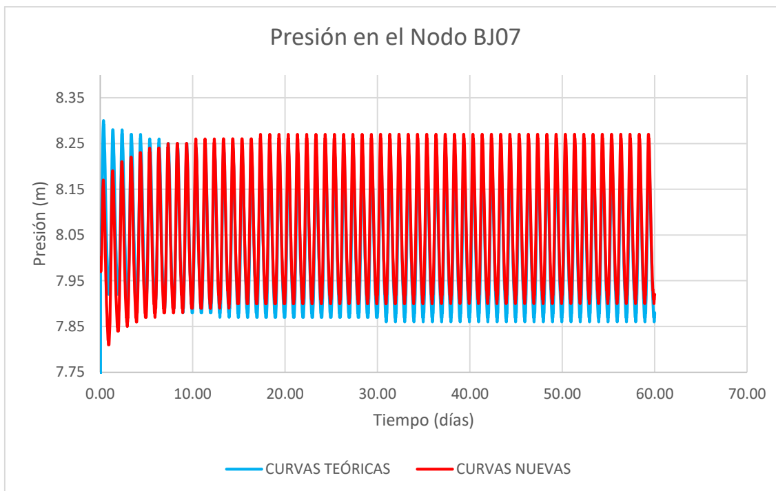
Gráfica 25 Presión en el nodo más cercano al pozo BJ07 en Miraflores
