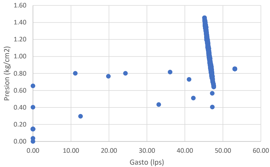
Gráfica 4 Datos medidos Pozo BJ07 en Miraflores
