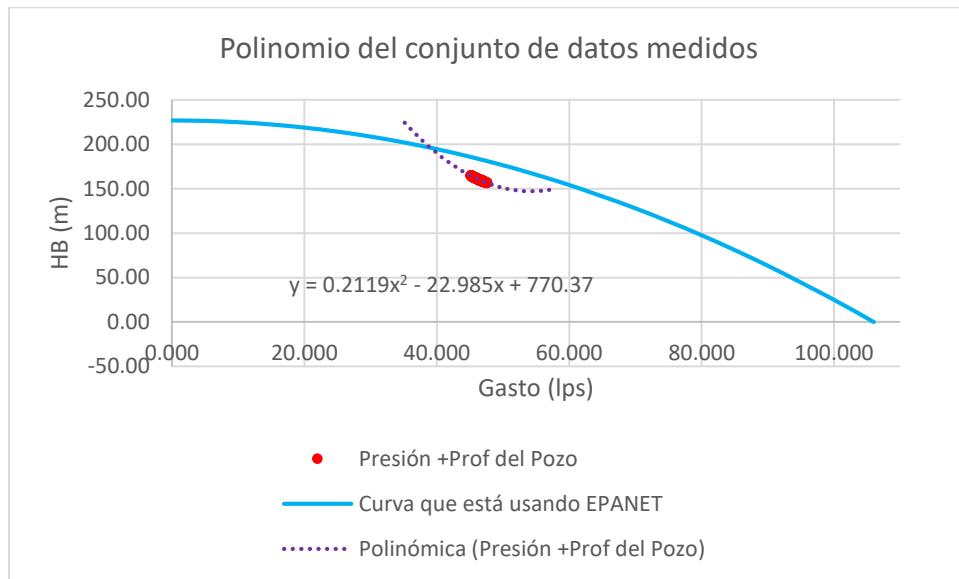
Gráfica 16 Curva Polinómica y polinomio del conjunto de datos. Pozo BJ 07 Miraflores.
