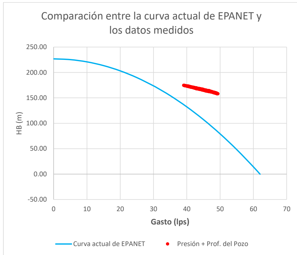
Gráfica 10 Comparación entre la curva actual de EPANET y los datos medidos. Pozo BJ06 Jardín Bombo.
