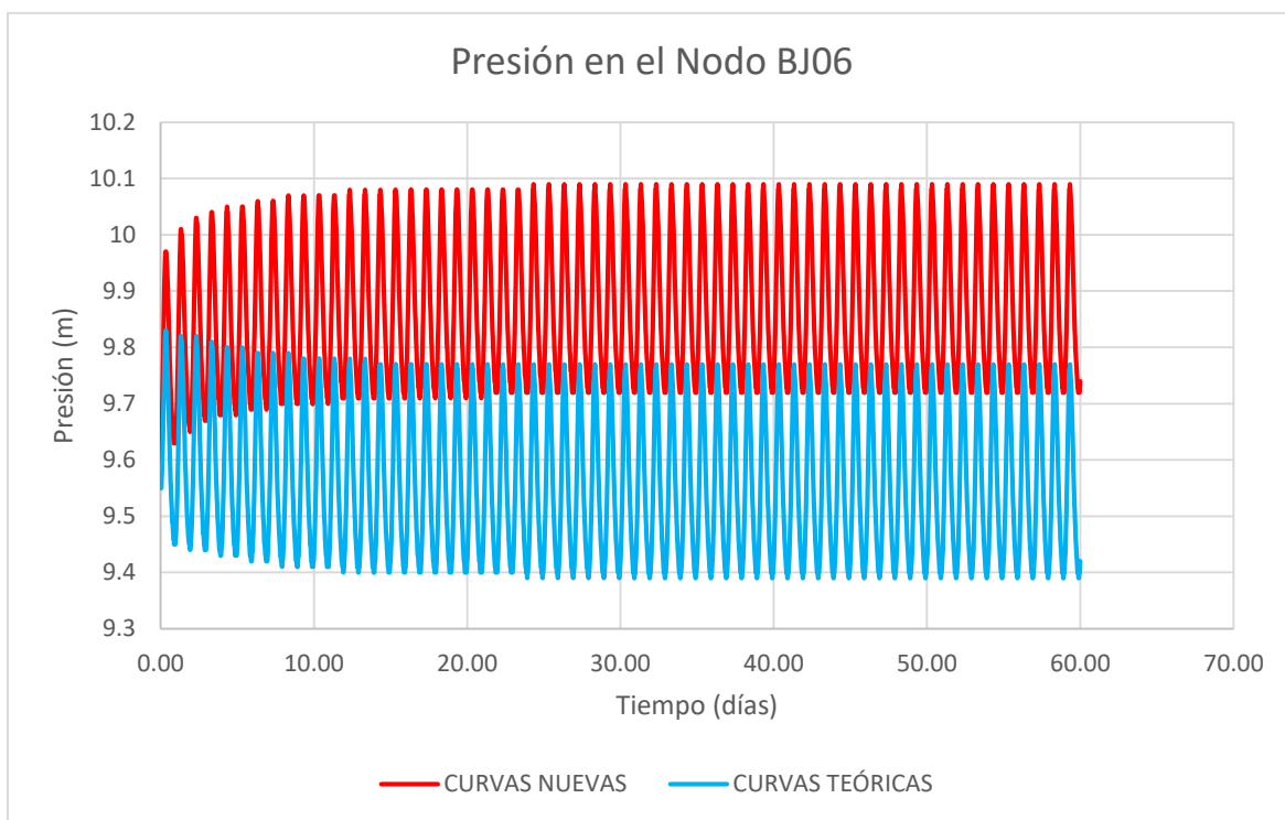
Gráfica 23 Presión en el nodo más cercano al pozo BJ06 Jardín Bombo.
