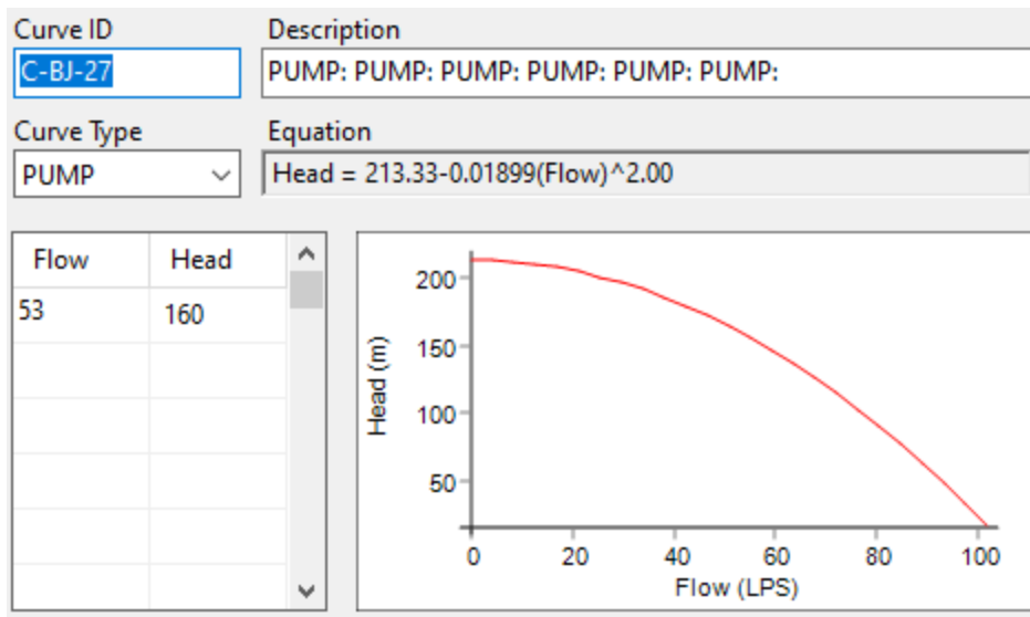
Imagen 16 Curva de la bomba pozo C-BJ-27 (Parroquia)
