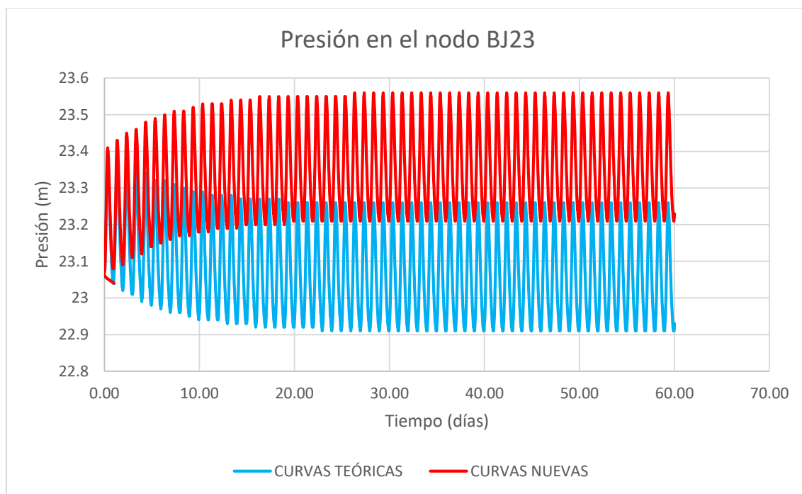
Gráfica 24 Presión en el nodo más cercano al pozo BJ23 en La Huerta
