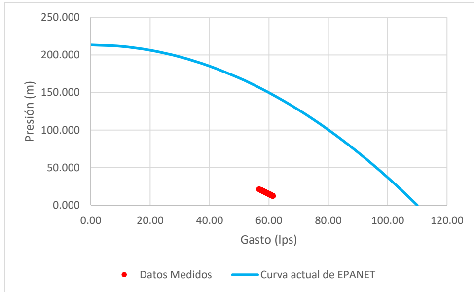
Gráfica 7 Comparativa datos medidos y curva actual. Pozo BJ23 en La Huerta
