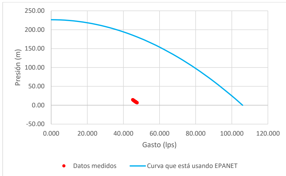
Gráfica 8 Comparativa datos medidos y curva actual. Pozo BJ06 Miraflores
