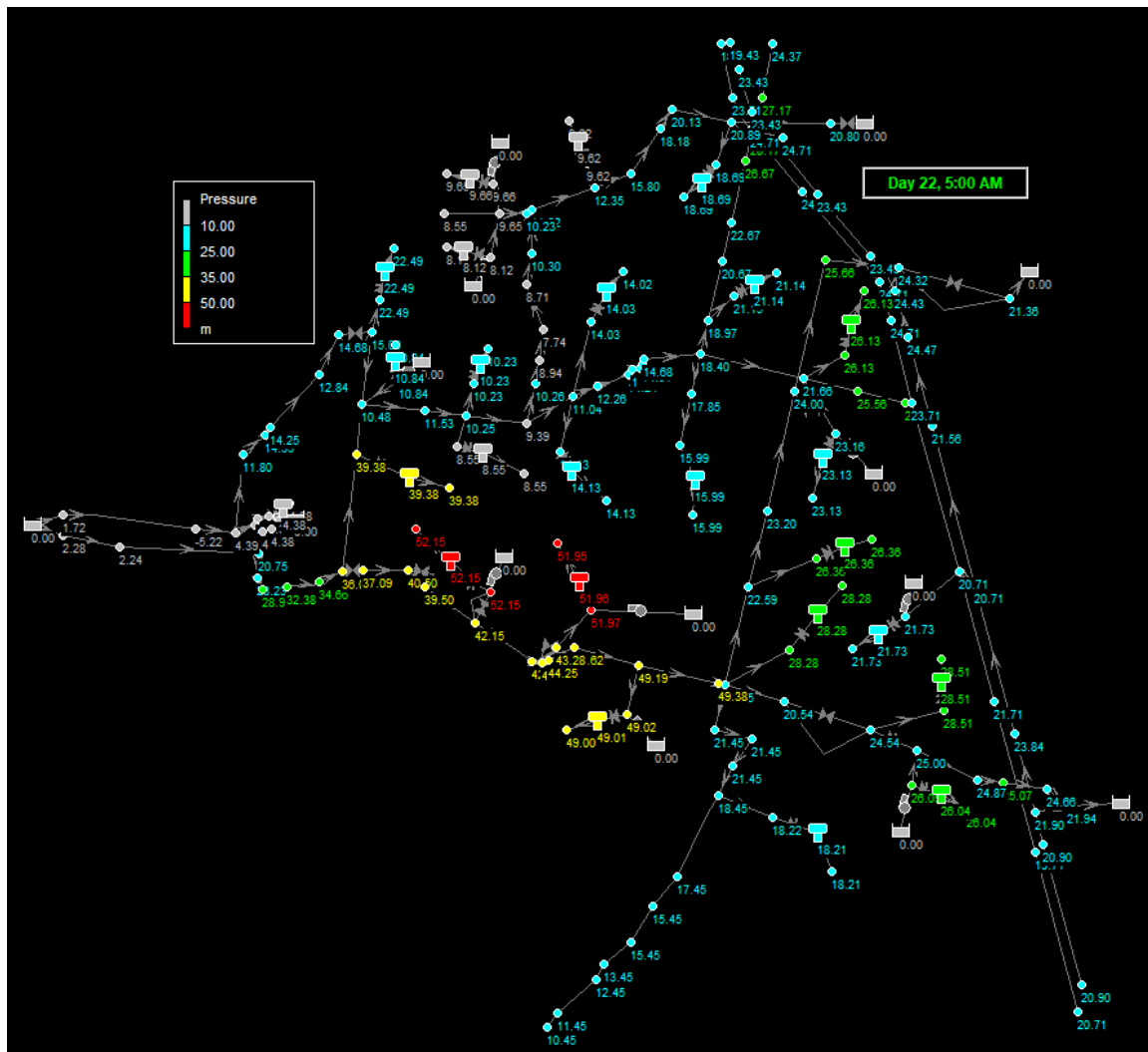
Imagen 21 Presiones cuando la red es estable a las 5:00hrs. Hora de menor demanda.
