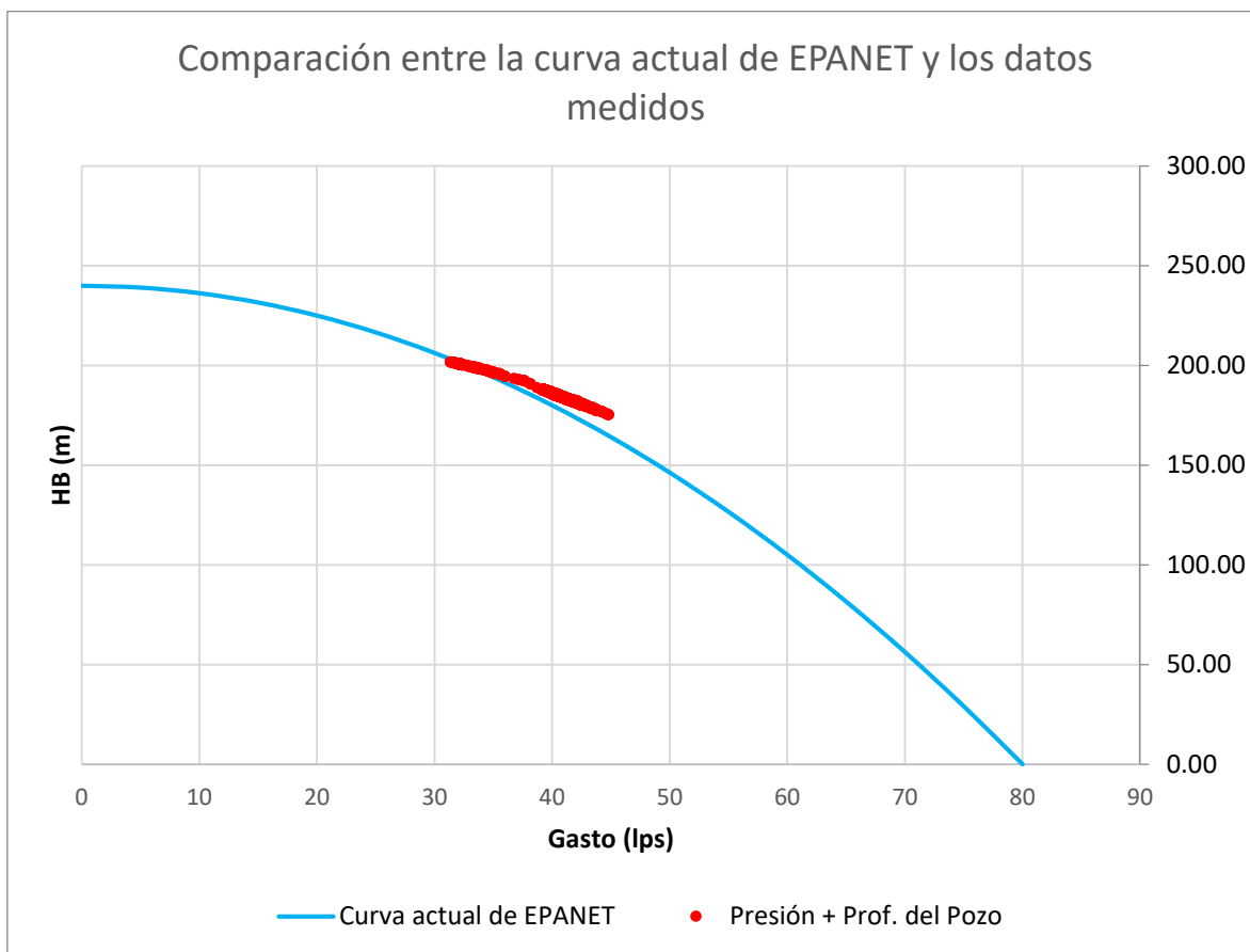
Gráfica 9 Comparación entre la curva actual de EPANET y los datos medidos. Pozo BJ03 Rosendo Arnaiz.
