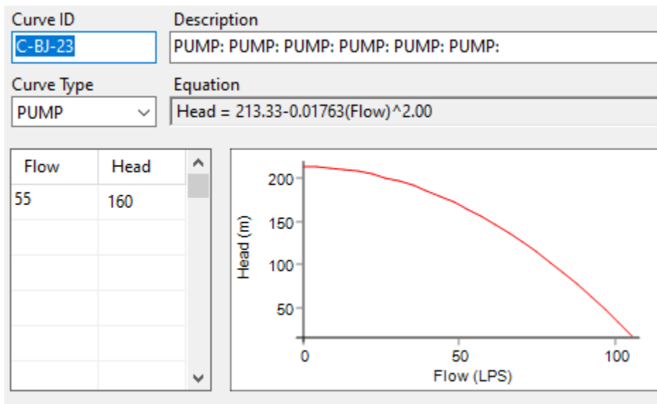
Imagen 15 Curva de la bomba pozo C-BJ-23 (La Huerta)
