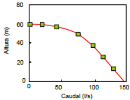
Imagen 7 Curva Multipunto
