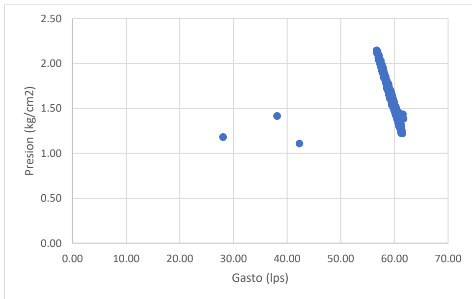
Gráfica 3 Datos medidos Pozo BJ23 en La Huerta
