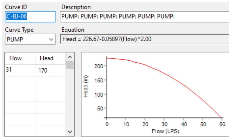
Imagen 10 Curva de la bomba pozo C-BJ-06 (Jardín Bombo)
