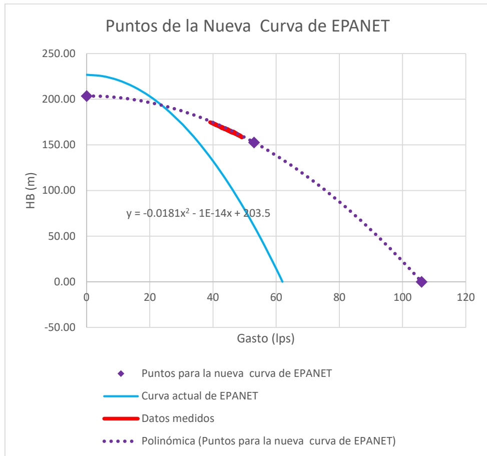
Gráfica 19 Curva nueva para EPANET. Pozo BJ06 en Jardín Bombo.
