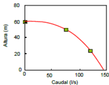
Imagen 6 Curva de tres puntos
