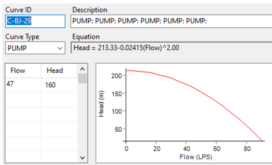
Imagen 17 Curva de la bomba pozo C-BJ-29 (Jardín Morelos)
