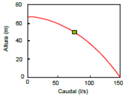
Imagen 5 Curva de un solo punto
