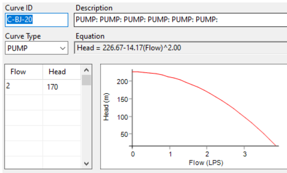
Imagen 13 Curva de la bomba pozo C-BJ-20 (Parroquia2)
