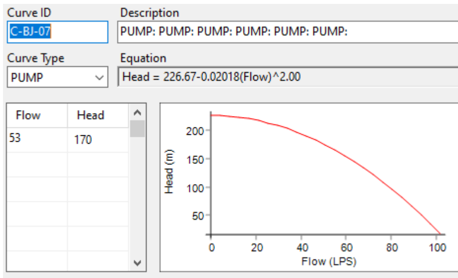
Imagen 11 Curva de la bomba pozo C-BJ-07 (Miraflores)
