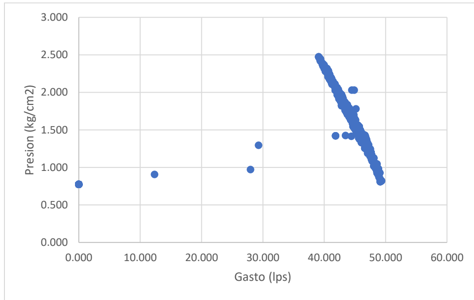
Gráfica 2 Datos medidos del pozo BJ06 en Jardín Bombo
