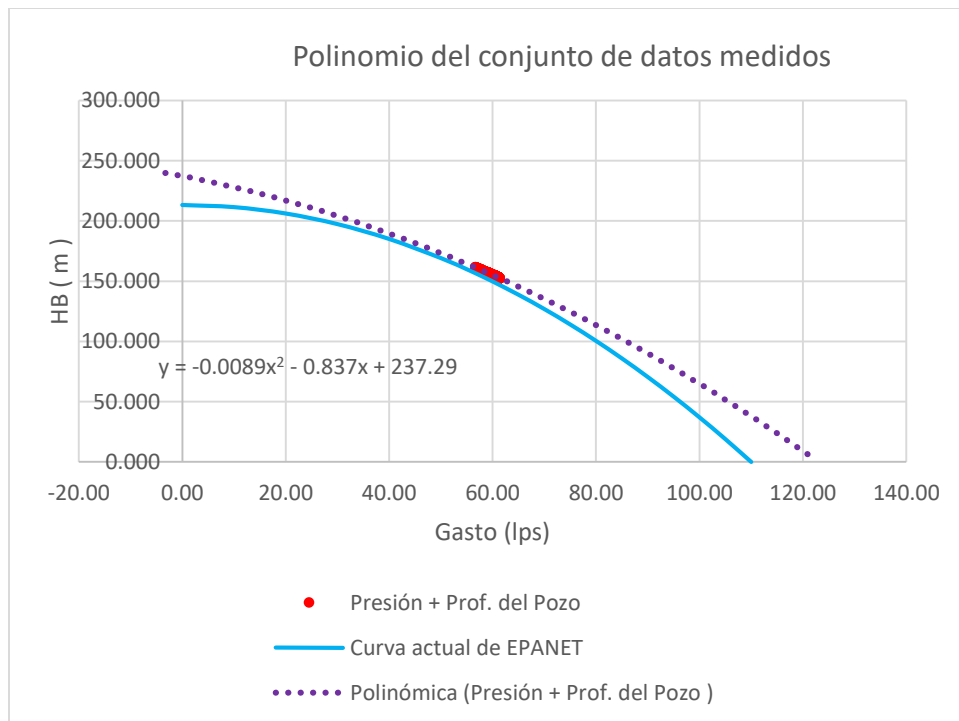
Gráfica 15 Curva polinómica y polinomio del conjunto de datos. Pozo BJ23 en La Huerta.
