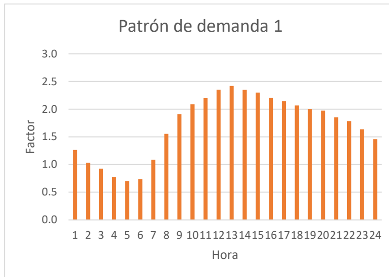
Imagen 3 Patrón de demanda 1
