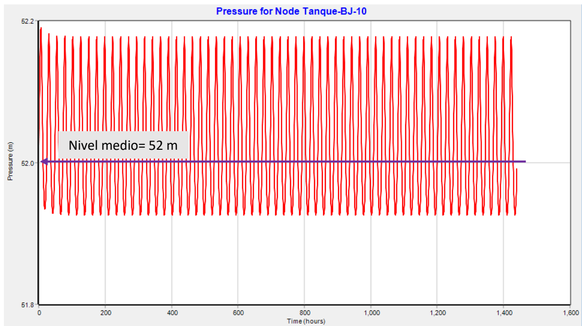
Imagen 18 Comportamiento del nivel de agua dentro del tanque.
