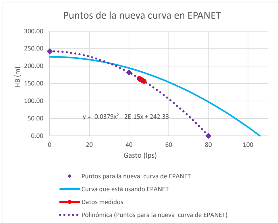
Gráfica 21 Curva nueva para EPANET. Pozo BJ07 en Miraflores.
