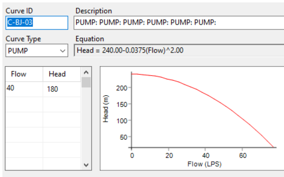
Imagen 9 Curva de la bomba pozo C-BJ-03 (Rosendo Arnaiz)
