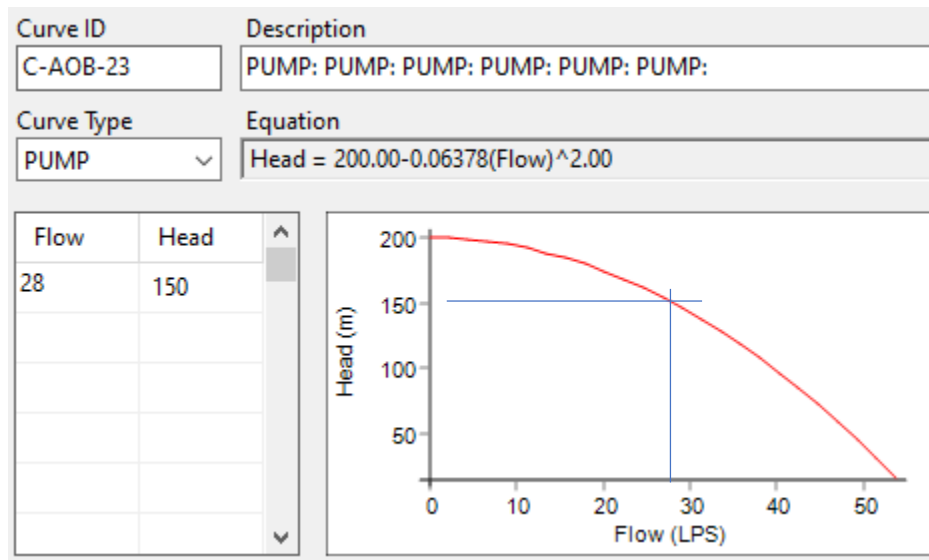
Imagen 8 Curva de la bomba pozo AOB-23 (Alonso XIII)
