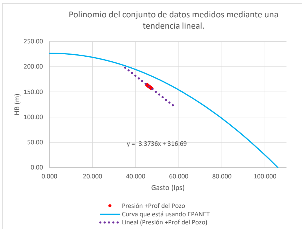
Gráfica 17 Polinomio de tendencia lineal del conjunto de datos. Pozo BJ 07 Miraflores.
