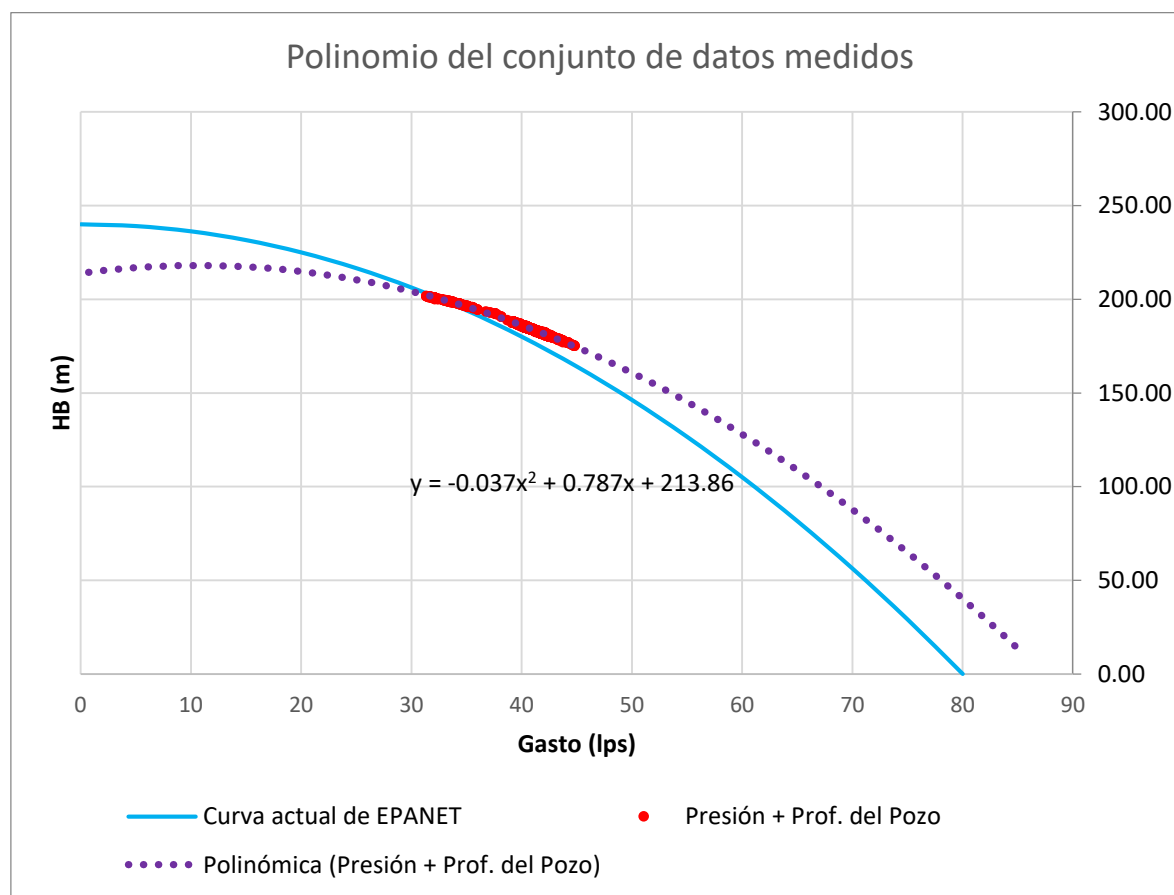
Gráfica 13 Curva polinómica y polinomio del conjunto de datos. Pozo (BJ-03) Ricardo Arnaiz
