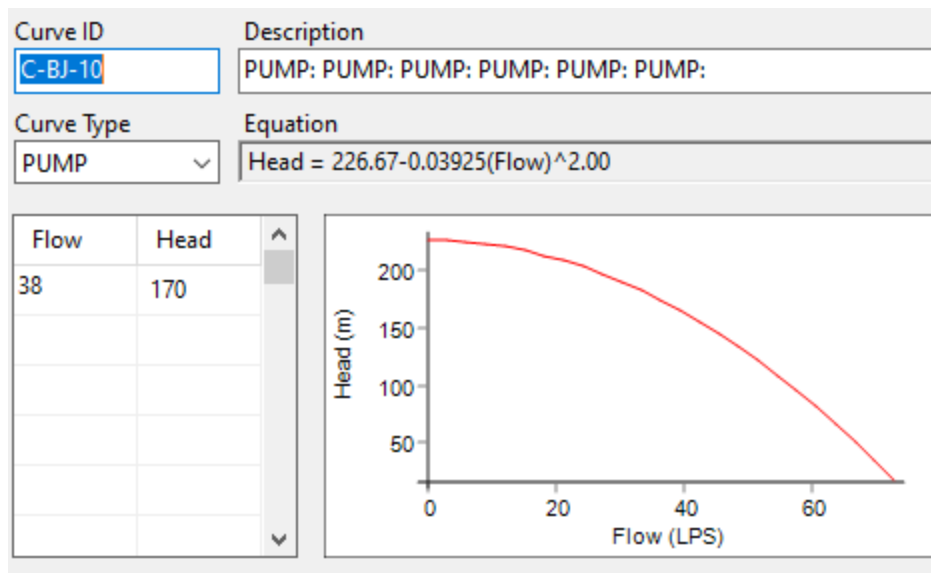
Imagen 12 Curva de la bomba pozo C-BJ-10 (La Campana)
