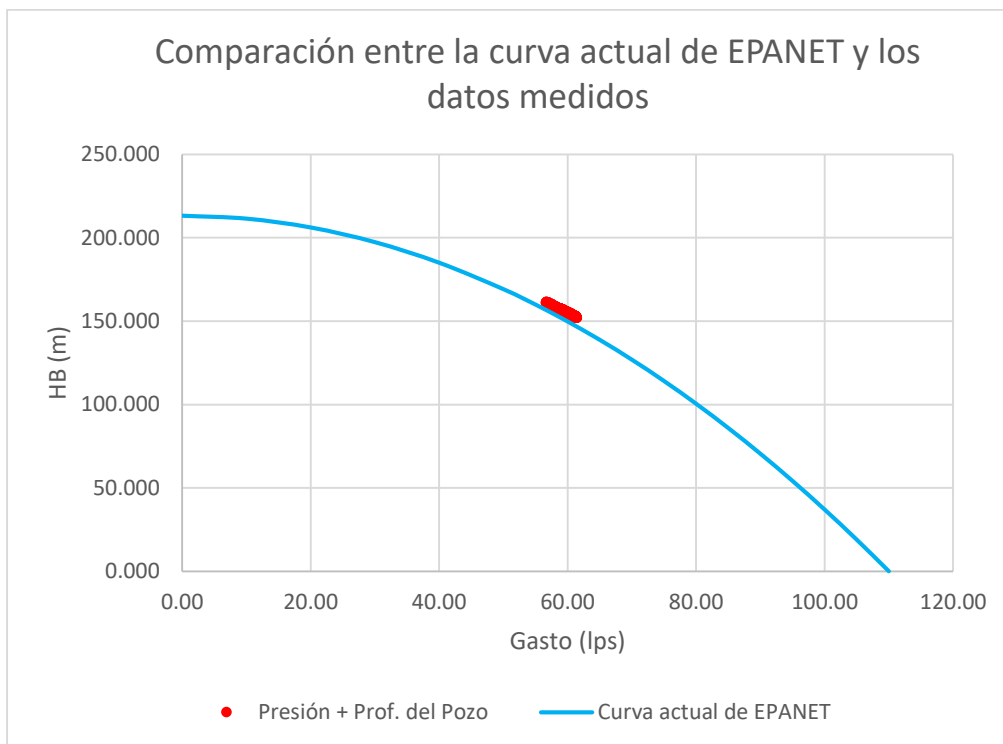
Gráfica 11 Comparación entre la curva actual de EPANET y los datos medidos. Pozo BJ23 La Huerta
