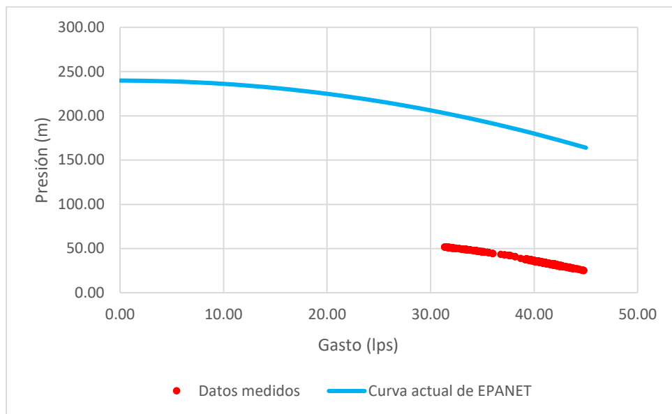
Gráfica 5 Comparativa datos medidos y curva actual. Pozo BJ03 en Rosendo Arnaiz
