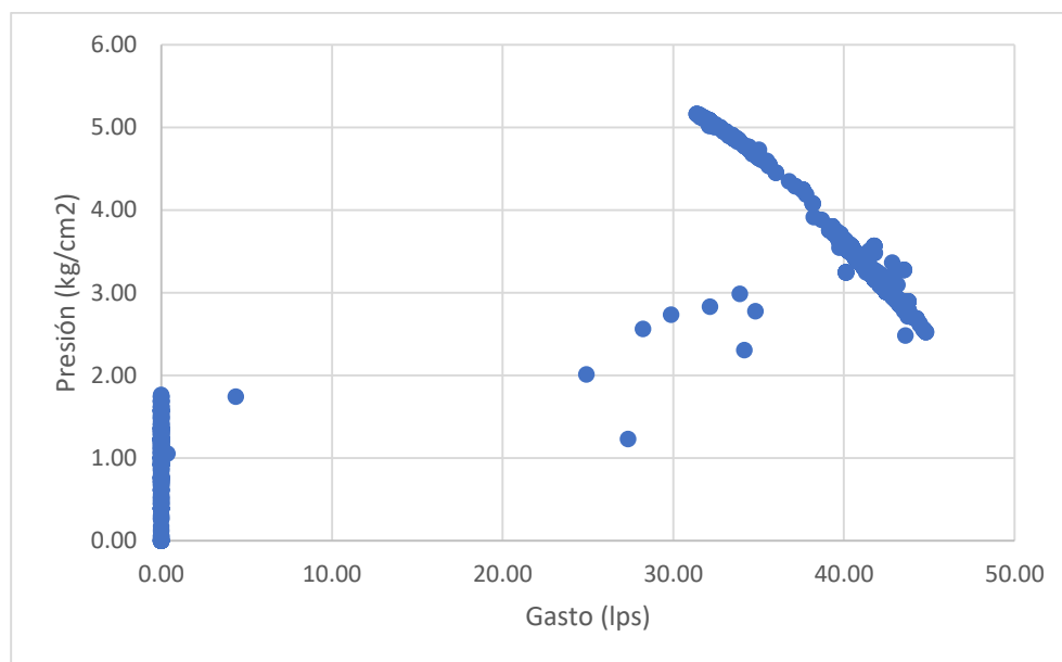
Gráfica 1 Datos medidos del Pozo BJ03 en Rosendo Arnaiz
