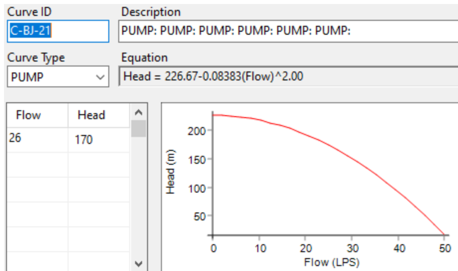
Imagen 14 Curva de la bomba pozo C-BJ-21 (Acacias)
