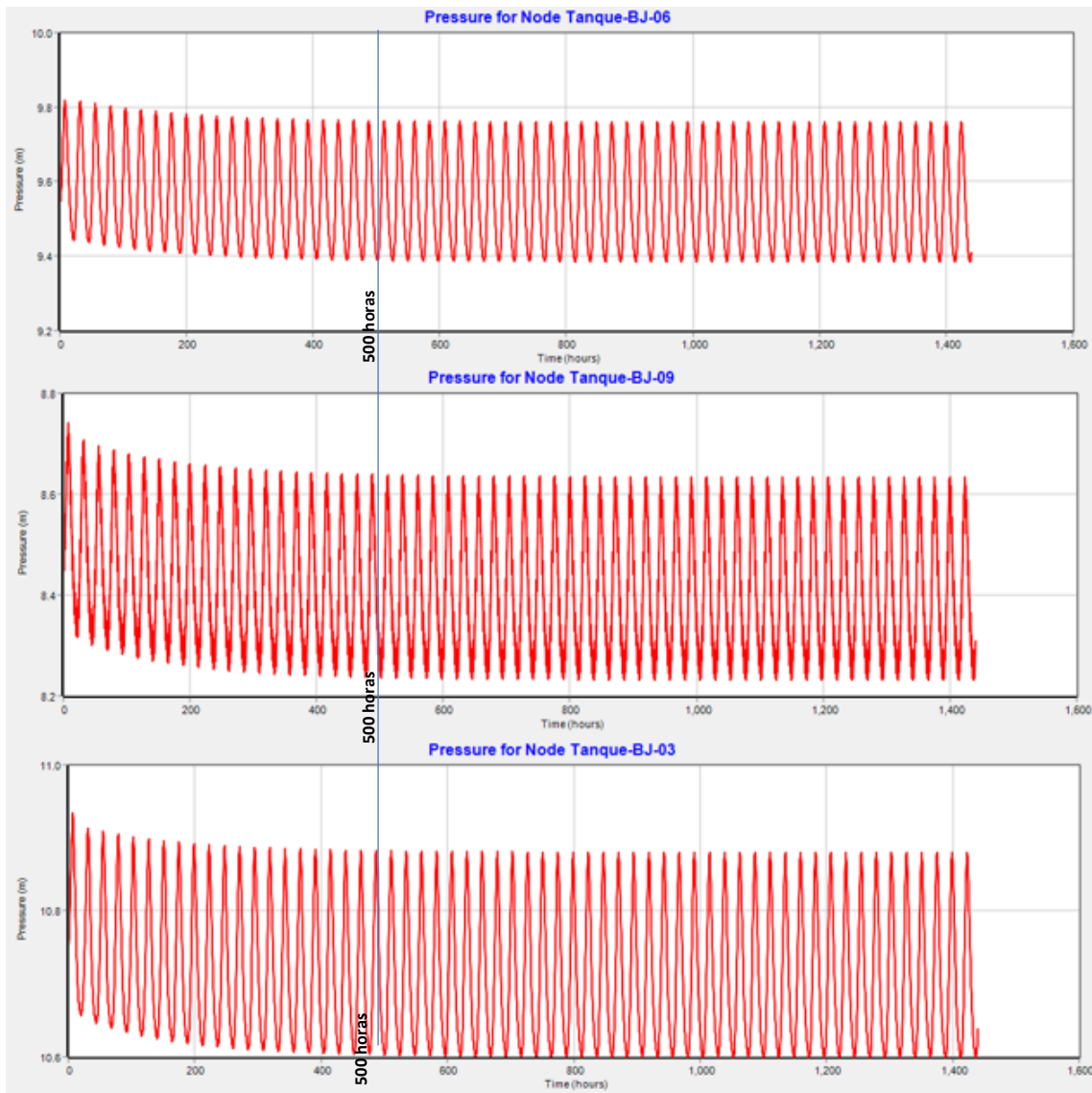
Imagen 20 Diferentes gráficas de la presión en diferentes tanques.
