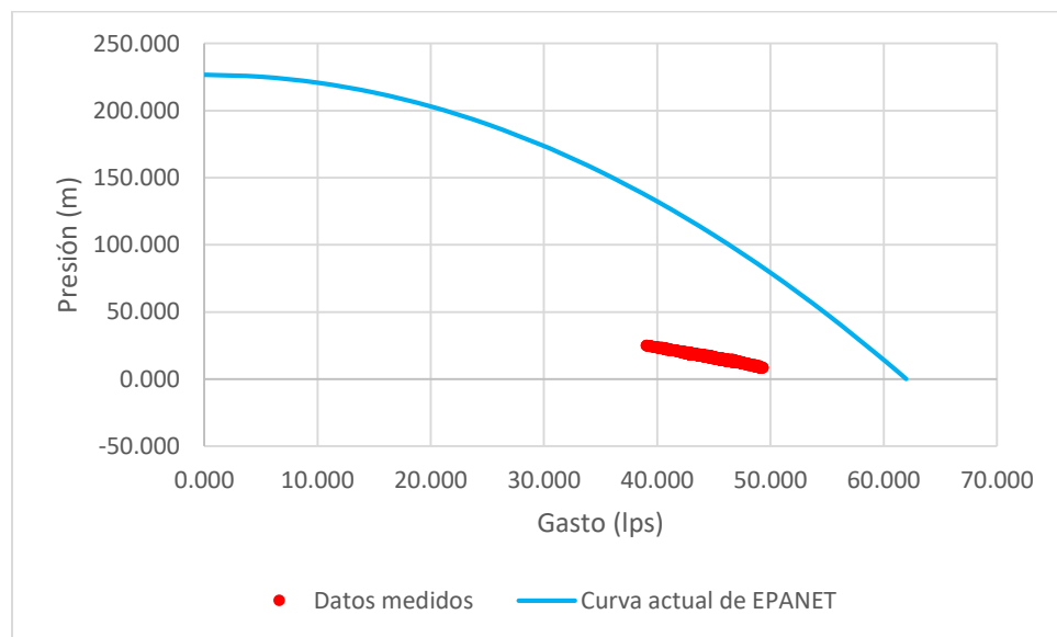
Gráfica 6 Comparativa datos medidos y curva actual. Pozo BJ06 Jardín Bombo.
