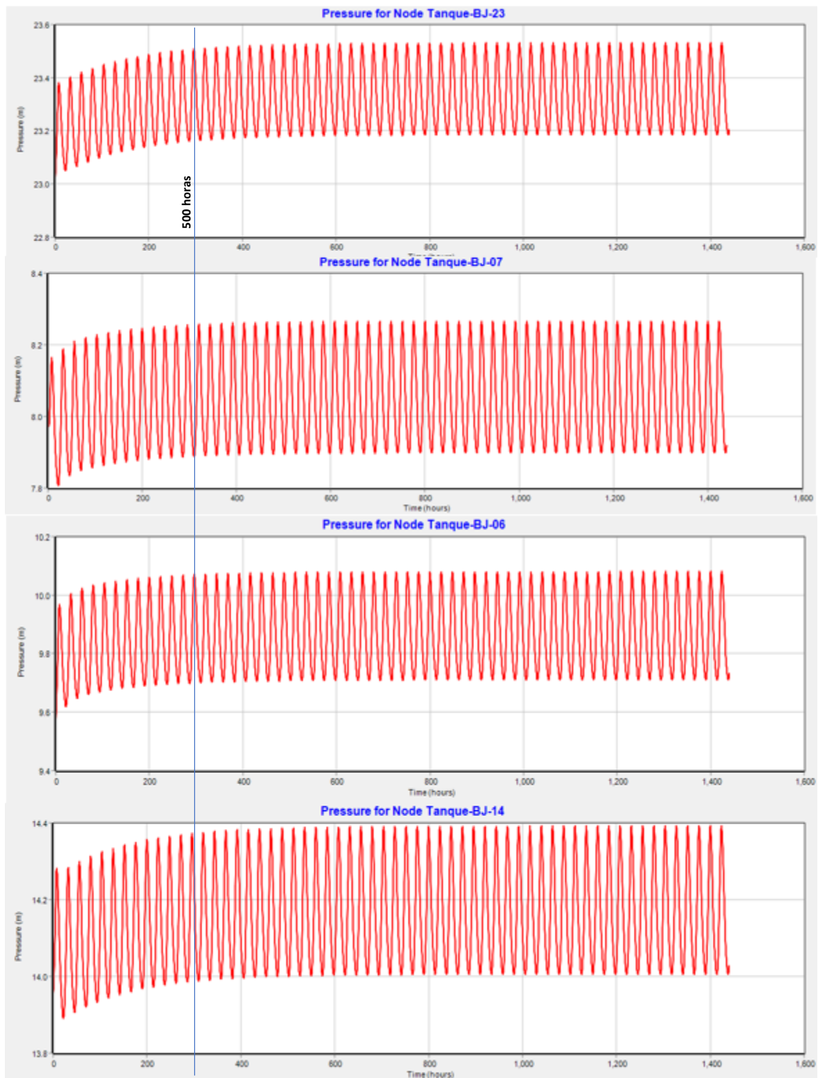
Imagen 24 Presiones en los tanques en los que más tarda en estabilizarse la red.
