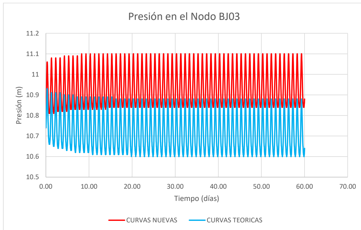
Gráfica 22 Presión en el nodo más cercano al pozo BJ03 Rosendo Arnaiz.
