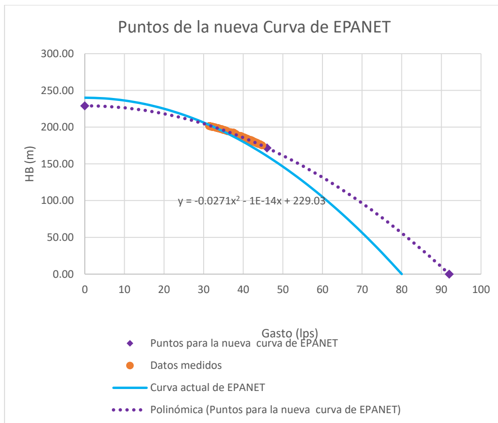
Gráfica 18 Curva nueva para EPANET. Pozo BJ03 en Rosendo Arnaiz
