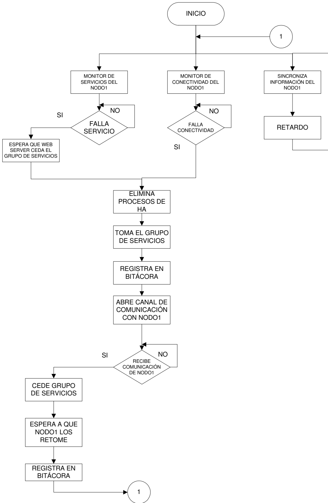
Figura 5.10 Diagrama de Flujo POLLUX
