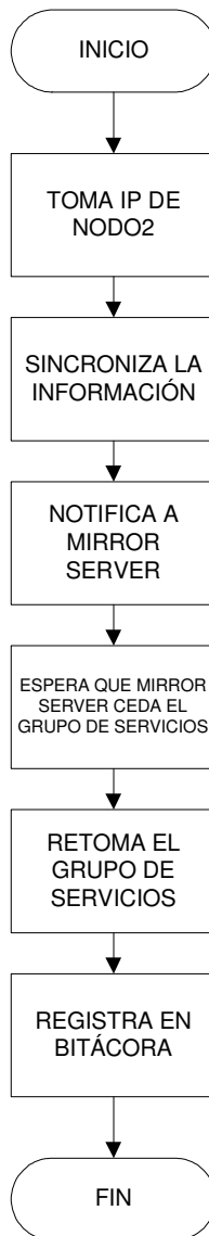
Figura 5.6 Diagrama de Flujo para RESTORE
