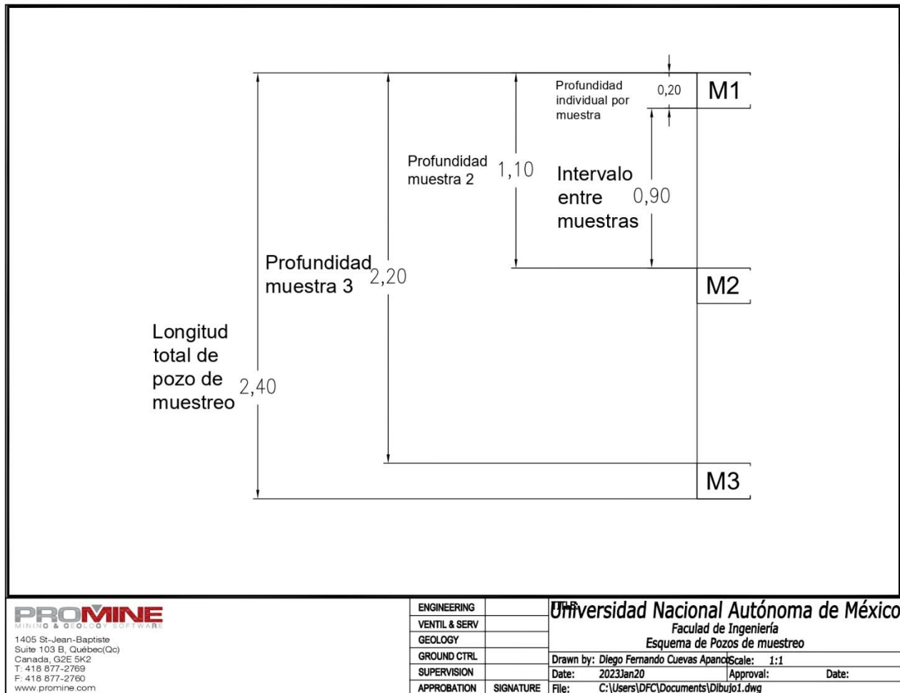
Figura 46. Esquema de pozo de muestreo.
