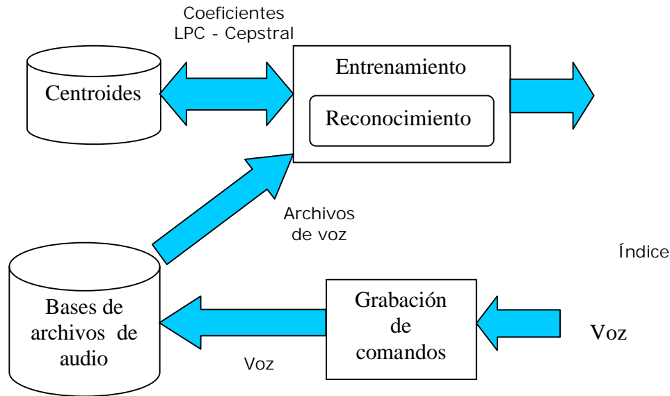
Fig. 4.1 b) Esquema general del entrenamiento de los comandos.
