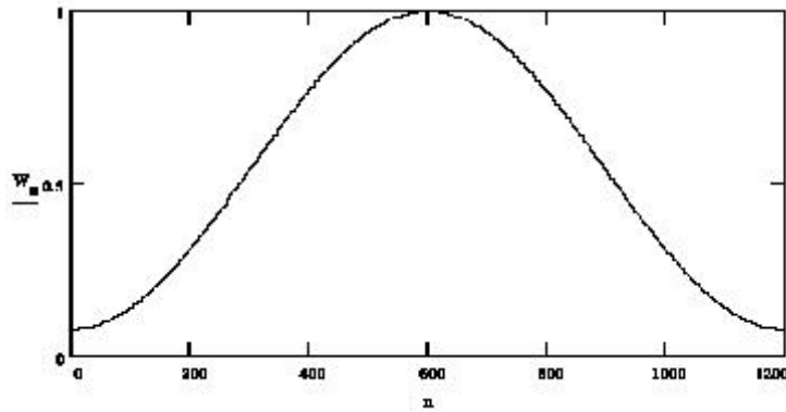
Fig. 1.6 Ventana de Hamming para 1200 muestras.
