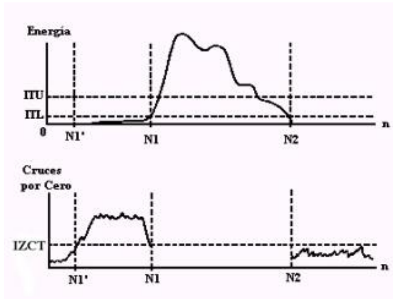
Fig. 1.5 Detección de inicio y fin de una señal de voz.
