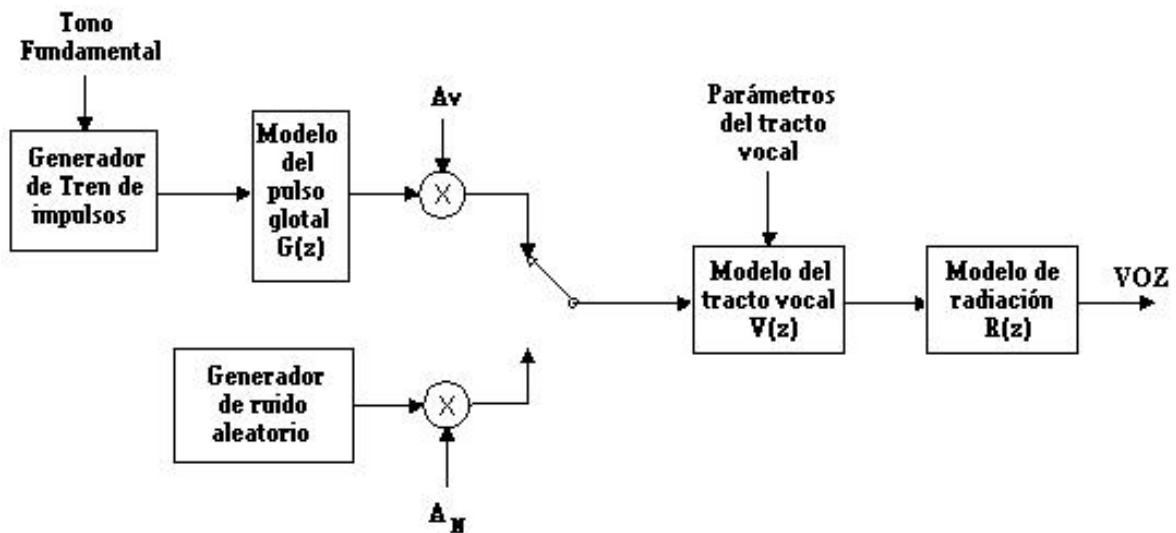
Fig. 1.3 Modelo digital para la voz.
