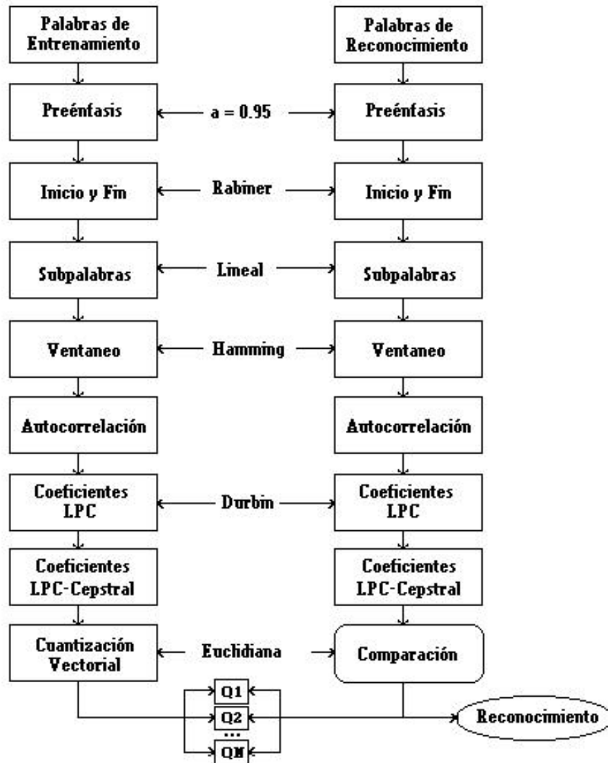
Fig. 1.4 Sistema de reconocimiento LPC-Cepstral.
